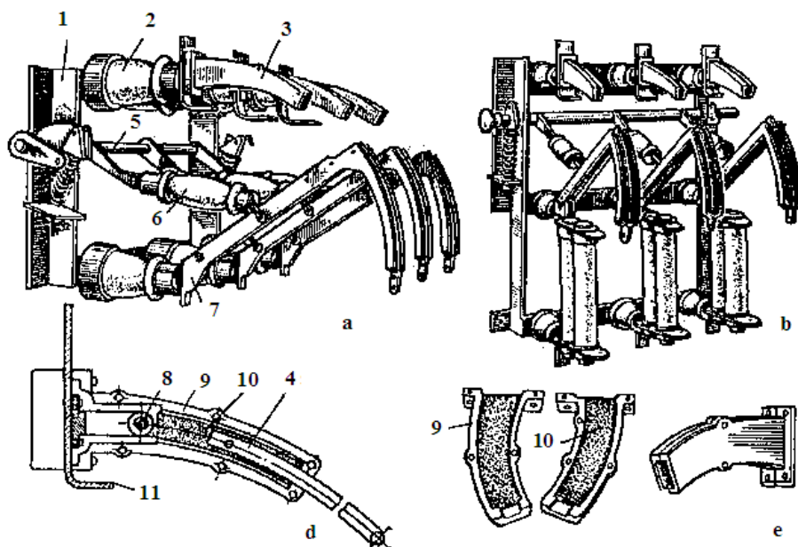
6.1-rasm. 6-10 kV ga yuklama o'chirgichlari: a) VN-16 (saqlagichlarsiz); b) VNP 16 (saqlagichli); d)- yon tomoni yig'ilgan yoy so'ndirish kamerasi; e)- yon tomoni va yig'ilgan kamera; 1- o'chirgich asosini o'rnatish metalli rama; 2-tayanch izolyator; 3-yoy so'ndirish kamerasi; 4-harakatlanuvchi pichoq kontakt; 5-yuritma o'qi; 6- harakatlanuvchi pichoqlarni tortgich; 7-harakatlanuvchi kontakt; 8- yoy so'ndirish harakatsiz kontakt; 9-yoy so'ndirish kamera ichki yuzasi; 10-organikshishali kiritma; 11- harakatsiz ishchi kontakt.
