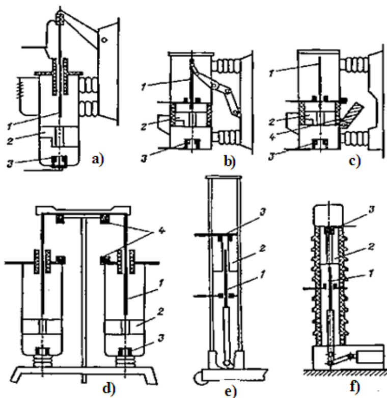
6.2-rasm. Kam moyli oʻchirgichlar konstruktiv sxemalari: 1- harakatlanuvchi kontakt; 2-Yoy soʻndirish kamerasi; 3- harakatsiz kontakt; 4- Ishchi kontakt.
