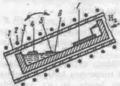
III 26-rasm. Nelson usuli bo'yicha suyuq epitaksiya uchun konteyner sxemasi:
