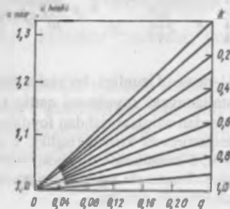
II 50-rasm. Choxralskiy yoki Brijmen usulida suyulmadan o'stirilgan kristallning tarkibi bir jins qismini aniqlash uchun nomogramma ( g -mazkur kristall qismini hosil qiluvchi suyulma ulushi, K -taqsimot koefitsienti).
