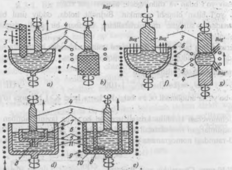
II.51-rasm. Uzunligi bo'yicha birday legirlangan kristallarni o'stirishda kristallanuvchi suyulmani qattiq (a, b), suyuq (d, e) va bug' (gaz) (f, g) fazalardan oziqlantirishdan foydalanadigan asosiy usullar:
