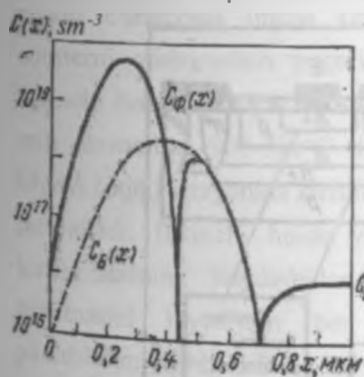
III.35-rasm. Ion legirlash usulida olingan n - p - n tuzilmali tranzistorlarda bor va fosfor taqsimoti.
