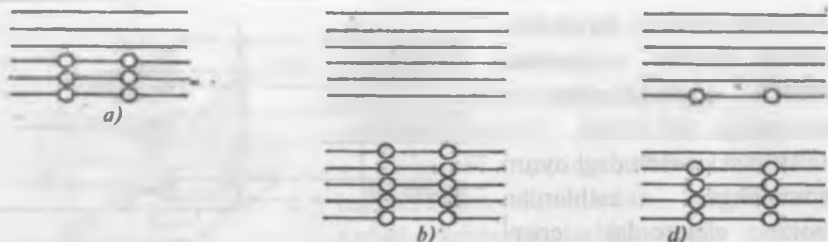
1.6—rasm. Energiya zonalarining elektronlar bilan to'ldiriliganligi hollari.
