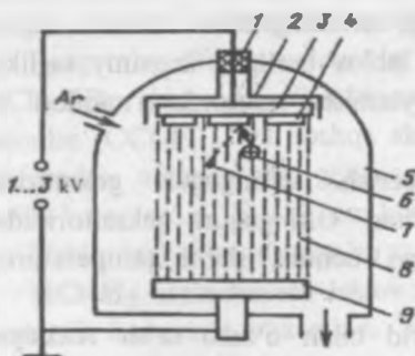
III 14-rasm. Vakuum kamerada ion-plazma yedirish jarayoni sxemasi:
