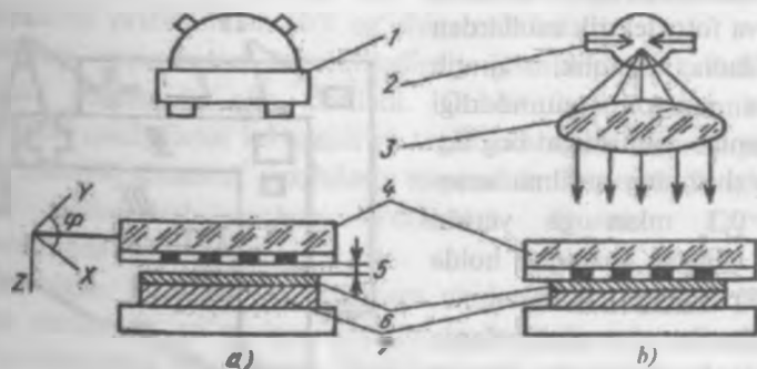
III. 47-rasm Kotaktli fotolitografiyada birga qo'shish (a) va ko'chirish (b) amali sxemalari:
