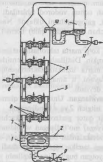
11.7—rasm. Rektifikatsion qurilma chizmasi.
