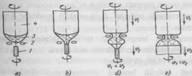
II.38-rasm Induktor diametri suyultiriladigan sterjen diametridan kichik bo'lgan holda tigelsiz zonaviy suyultirish usulida kristalni o'stirish jarayoni bosqichlari ( v_1 , v_2 — mos ravishda, sterjen va xamirturush harakati tezliklari): a -suyulma tomchisi hosil qilish; b -xamirturushni ho'llanishi; d -diametrni shakllantirish; e -o'zgarmas diametrli kristalni o'stirish.
