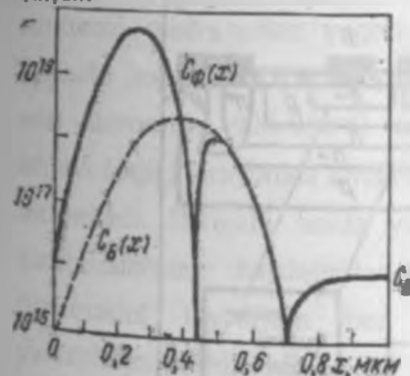
III.35-rasm. Ion legirlash usulida olingan n - p - n tuzilmali tranzistorida bor va fosfor taqsimoti.
