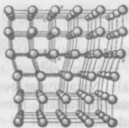
1.8—rasm. Kristalldagi chegaraviy dislokatsiya
