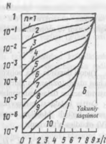
11.25—rasm. Ko'p qaytalangan zonaviy suyultirish usulida o'stirilgan kristall bo'yicha uchimovchan kirishma nazariy taqsimoti.
