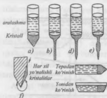
11.34-rasm Normal yo'nalgan kristallanish usulida kristallar o'stirishda qo'llaniladigan tigellar shakllari.
