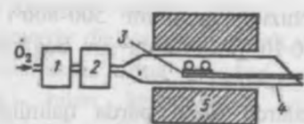
III 41-rasm Quruq kislorodda oksidlanish uchun qurilma sxemasi.
