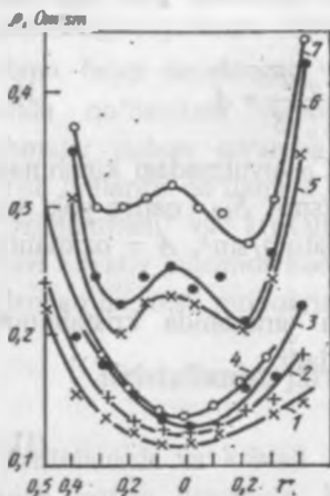
II 54-rasm. Aluminiiy kirishmasi kiritilgan kremniy monokristallarining ko'ndalang kesimi bo'yicha solishtirma elektr qarshilik taqsimoti:
