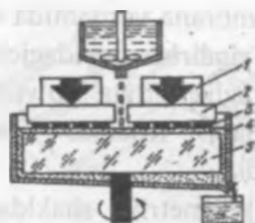
III.9-rasm. Tekislashda yarimo'tkazgich plastinkalar joylashishi: 1-yuk; 2-planshayba; 3-yarimo'tkazgich plastinkalar, 4-abraziv suspenziya; 5-tekislagich.
