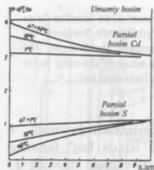
11 47-rasm. Nostexiometrik \text{CaS} tarkiblovchilarning parsial bosimlari hisoblangan qiymatlarining (turli \Delta T lar uchun) manbagacha masofaga bog'liqligi.
