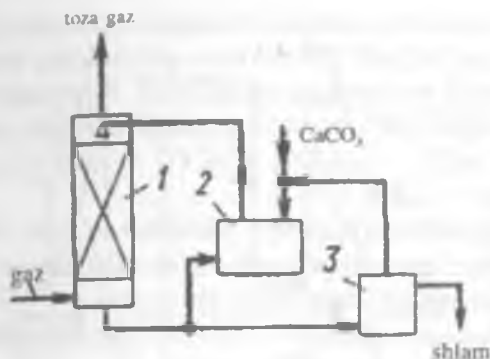
9.2- rasm. Oltingugurt anhidridini ohakli suv yordamida tozalash texnologik sxemasi:
