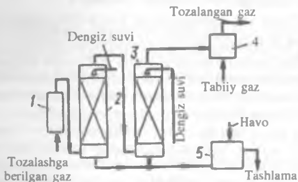
9.1- rasm. Oltingugurt angidridini dengiz suvi yordamida tozalash texnologik sxemasi:
