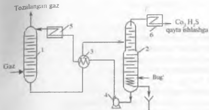
11.3-rasm. Gaz tarkibidagi H_2S va CO_2 larini monoetanolin eritmasi yordamida tozalash texnologik sxemasi:
