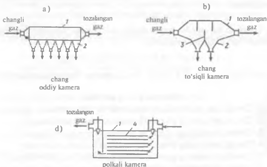
5.1-rasm. Chang tindirish kameralari:
