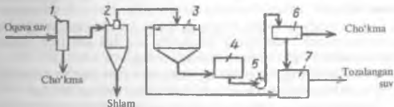
17.11-rasm. Sentrifugali oqova suv tozalash texnologik sxemasi: 1-reshtoka; 2-gidrosiklon; 3-zichlashtirish apparati; 4,7-sig'im; 5-nasos; 6-sentrifuga.
