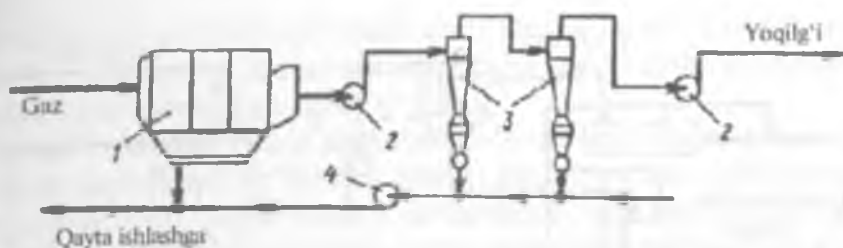
7.1-rasm. Changlarni rekuperatsiya qilish qurilmasi: 1-elektrofiltr; 2-nasos; 3-siklon; 4-haydagich.
