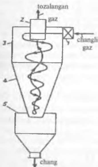
5.4-rasm. Siklonda gaz harakati:
