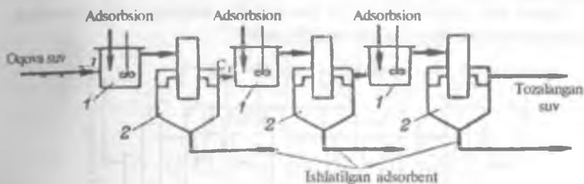
18.10-rasm 1. Adsorbtsion qurilmaning sxemasi:
