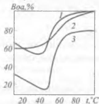
10.1-rasm. Tutun gazlarini azot oksidlaridan tozalash darajasining turli oksidlanish darajasidagi ( NO_a = [NO_2]/[NO+NO_2] ) haroratga bog'liqligi:
