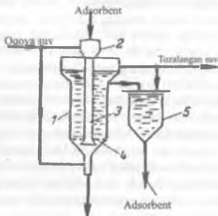
18.13-rasm. Mavhum qaynash rejimida ishlovchi silindrik bir yarusli adsorberning sxemasi:
