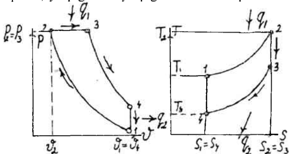
33-rasm. P=\text{const} boʻlganda issiqlik keltiruvchi siklning P - V diagrammasi
