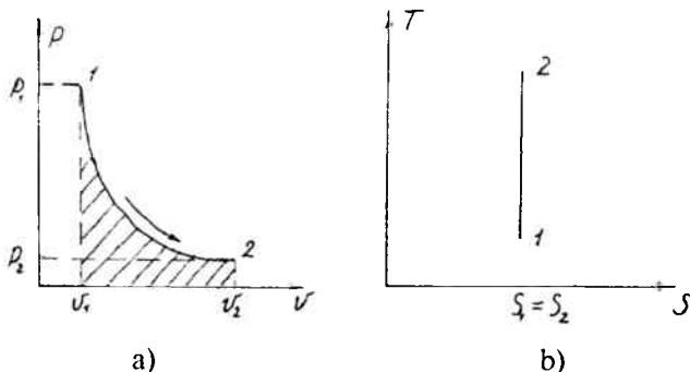
9-rasm. a) adiabatik jarayonning P - V diagrammasi; b) adiabatik jarayonning T - S diagrammasi.
