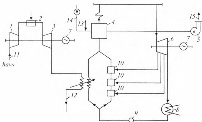
6.4- rasm. Bug' sikli ustiga gaz sikli qurilgan BGQ ning sxemasi: 1—kompressor; 2—yonish kamerasi; 3—gaz turbinasi; 4—bug' qozoni; 5—tutun tortkich; 6—bug' turbinasi; 7—elektr generatori; 8—kondensat; 9—ta'minlash nasosi; 10—regenerativ isitkichlar; 11—havo olish; 12—gazlar atmosferaga; 13—qozonga yoqilg'i berish; 14—havo berish; 15—tutun gazlari atmosferaga.
