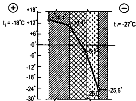
2.3-rasm. Tashqi to'siq konstruksiyadagi harorat chizig'i.
