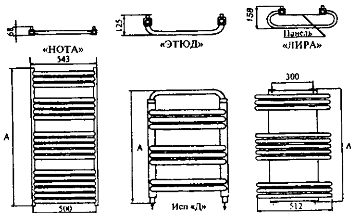
4.8-rasm. Sochiq quritgich radiatorlar
