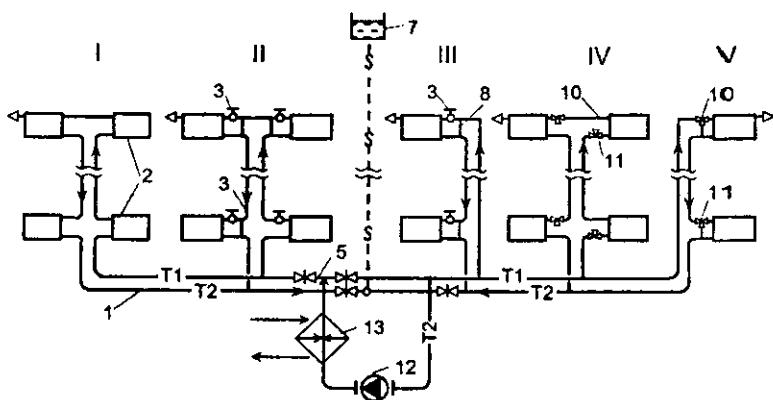
6.8, b-rasm. Quyidan taqsimlanuvchi bir quvurli va «II» harfi shaklidagi tirkaklari turli konstruksiyali tirkakli isitish tizimlari: I – to'g'ri oqimli tirkak; II va III – siljirilgan va oxiri «II» shaklida ulangan tirkak; IV-V – to'g'ri oqimli boshqariluvchi tirkak
