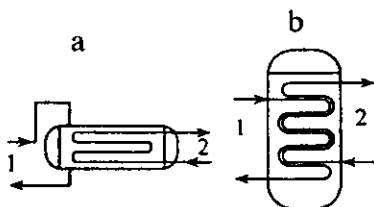
15.2-rasm. Bog'liq bo'lmagan issiqlik yig'uvchi moslamaning isitish tizimi konturiga bog'liq (a) va bog'liq bo'lmagan (b) sxemasi: 1 – isituvchi kontur; 2 – isitish tizimi konturi
