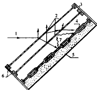
15.9-rasm. Yassi quyosh kollektori. 1 – quyosh nurlari; 2 – shishali yuza; 3 – kollektor qobig'i (korpusi); 4 – issiqlik qabul qiluvchi (plastina); 5 – issiqlikdan izolyatsiyalovchi qatlam; 6 – shishani o'rnatish uchun moslama; 7 – issiqlik qabul qiluvchining uzun to'laqlin nurlanishi
