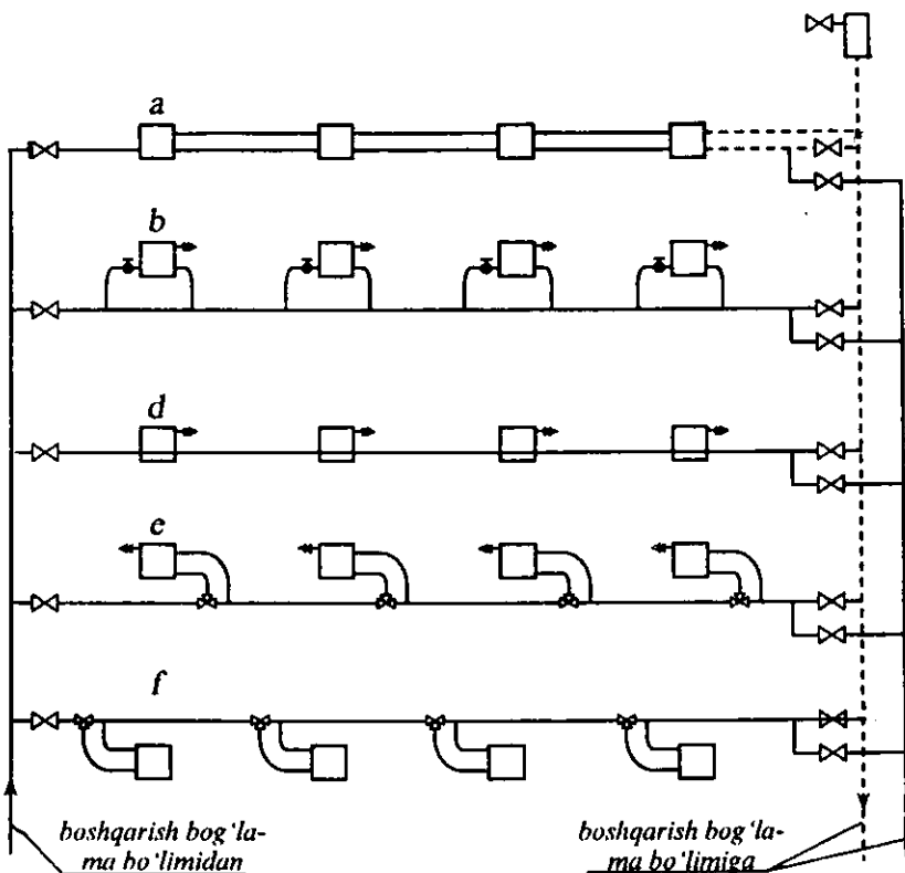
1.6-rasm. Sun'iy harakatlanuvchi suv bosimi ta'sirida ishlaydigan bir quvurli gorizontal isitish tizimlarining prinsipial sxemasi: a) issiq suvni to'g'ridan-to'g'ri to'liq miqdorda isitish asbobi orqali o'tish uslubi; b) birlashtiruvchi uzatma orqali isitish asboblarning ulanish uslubi; d) to'g'ridan-to'g'ri isitish asbobiga ulanish uslubi; e) boshqariluvchi, to'g'ridan-to'g'ri plintusgardishli ulash uslubi; f) to'g'ridan-to'g'ri, boshqariluvchi, deraza tagiga ulanuvchi gorizontal o'rnatilgan isitish asboblari
