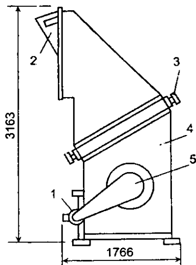
10.4-rasm. Polga o'rnatilgan havo retsikulyatsiyali STA-300M rusumli agregat: 1 – elektrodvigatel; 2 – havo qopqog'i; 3 – havo isituvchi uskuna; 4 – uskuna; 5 – g'ilofga o'ralgan tasmali uzatma
