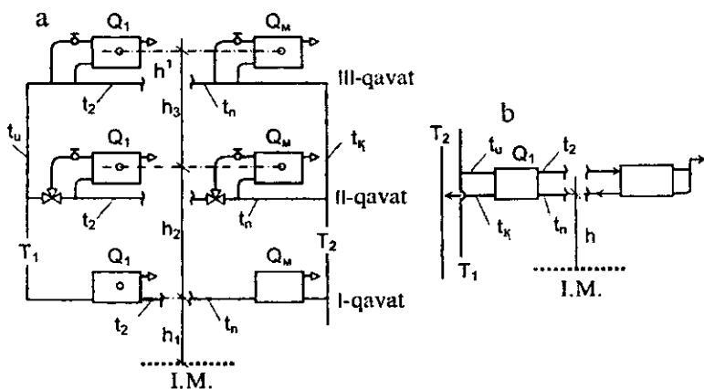
7.6-rasm. Gorizontalar o’rnatilgan bir quvurli issiq suv bilan ishlaydigan isitish tizimining sxemasi
