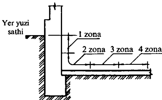
3.2-rasm. Pol maydonida sarf bo'layotgan issiqlik miqdorini aniqlash uchun qabul qilingan sxema
