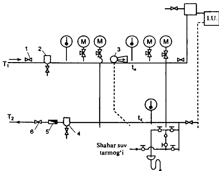
6.2-rasm. Yuqori haroratli issiqlik quvuriga bevosita bog'liq bo'lib ulangan isitish tizimining prinsipial sxemasi
