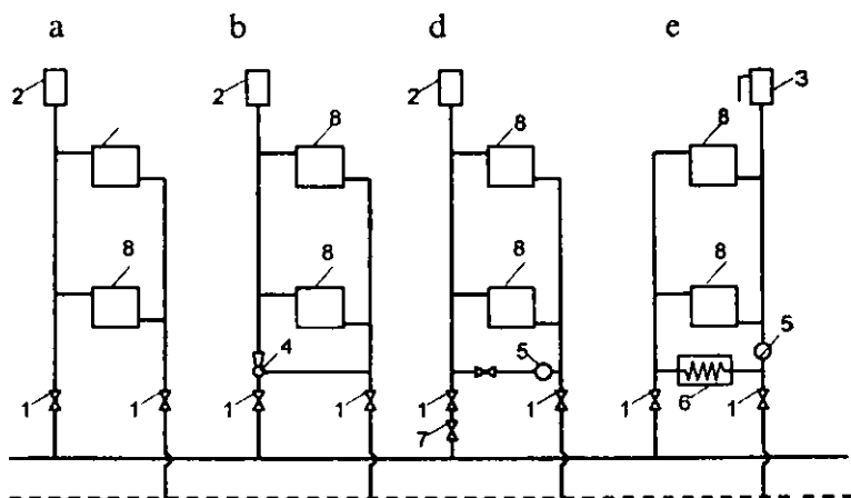
6.1-rasm. Issiqlik qurilmalarining issiqlik tashuvchi quvurlariga ulanishi: a – bevosita ulanish sxemasi; b – elevator bog'lami bilan birgalikda aralashtirilish usuli bilan ulanishi; d – ulanish quvurida nasoslarning o'rnatilishi; e – issiq suv hosil qilish uchun o'rnatilgan qurilma bilan ulanish sxemasi; 1 – o'chirgich (zadvijka); 2 – havo yig'uvchi uskuna; 3 – kengaytiruvchi idish; 4 – suv elevatori; 5 – nasoslar; 6 – issiqlik hosil qiluvchi uskuna; 7 – bir tomonlama o'tkazuvchi klapan; 8 – isitish asbobi
