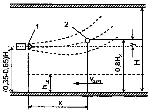
10.5-rasm. Isitilgan havo oqimining xona balandligi bo'yicha tarqalishi: 1 – isituvchi agregat; 2 – kritik ko'ndalang kesimda havo harakatining ko'rinishi
