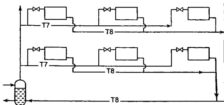
15.4-rasm. Gorizontal ikki quvurli past haroratli bug'li isitish tizimining umumiy ko'rinishi
