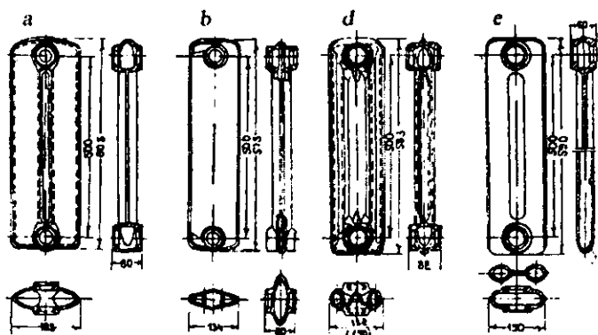
4.3-rasm. Turli isitish asboblarning shakli: a – «Польза» radiatori; b – «Гусенический» radiatori; d – «Москва-132» radiatori; e – ЛОП-150 nomli radiator
