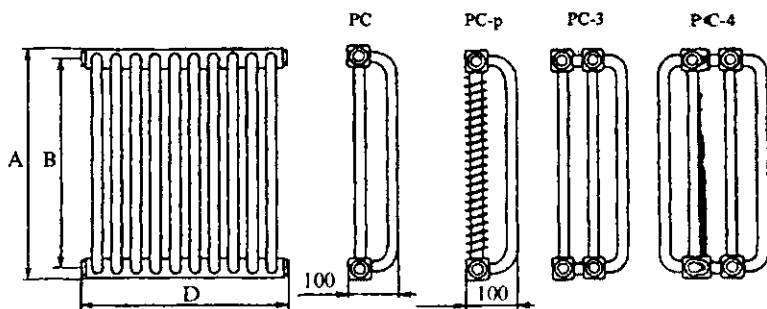
4.7-rasm. Po'lat quvurli radiatorlar
