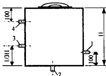
6.10-rasm. Kengaytirish sig'iriga ulanuvchi quvurlar: 1 – kengaytiruvchi quvur uchun ; 2 – probkali patrubka; 3 – nazorat qilishga mo'ljallangan quvur; 4 – ortiqcha issiq suvni chiqarish quvuri
