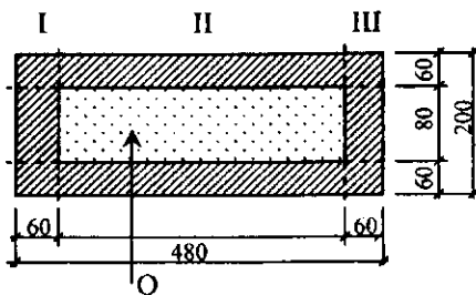
2.1-rasm. Bo'shlig'i yengil material bilan to'ldirilgan betondan iborat kichik blok
