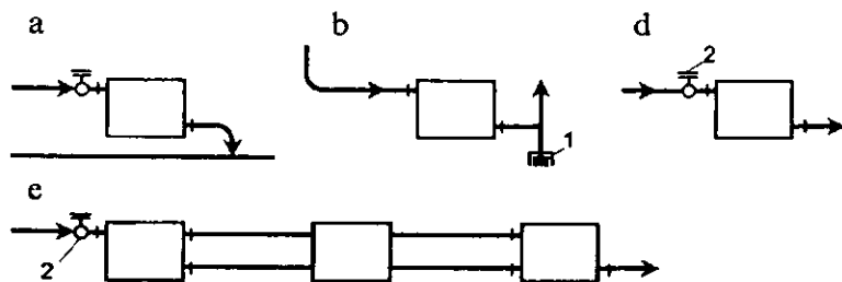
5.9-rasm. Issiqlik tashuvchining isitish tizimida yuqoridan pastga harakatlanganda quvurlarni isitish asboblari har tomonlama ulanishi
