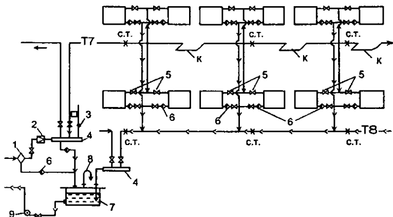
9.7-rasm. Kondensat va magistral bug' quvurlarining halqali harakatda bo'lgan ikki quvurli isitish tizimining sxemasi: 1 – bug' dan ajralayotgan suv kondensatini ajratuvchi uskuna; 2 – bug' bosimini pasaytiruvchi uskuna; 3 – ortiqcha bosim ta'sirini kamaytiruvchi moslama; 4 – tarqatuvchi kollektor; 5 – bug' miqdorini boshqaruvchi jo'mrak; 6 – kondensat ajratuvchi uskuna; 7 – kondensat idishi; 8 – havo quvuri; 9 – kondensat nasos; x – siljimas tirgak
