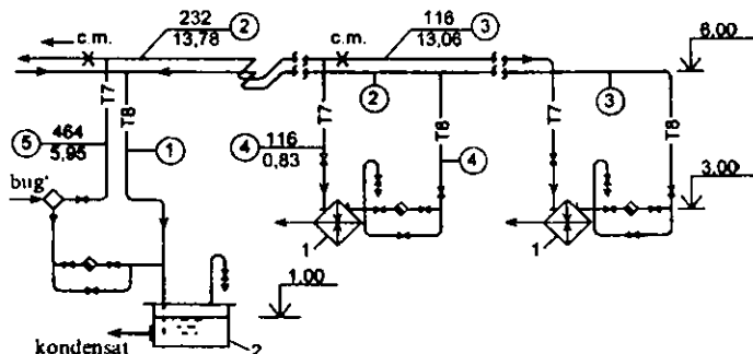
9.12-rasm. Yuqori bosim ta'sirida ishlaydigan isitish tizimining (kondensat idishi yopiq) hisobiy sxemasi
