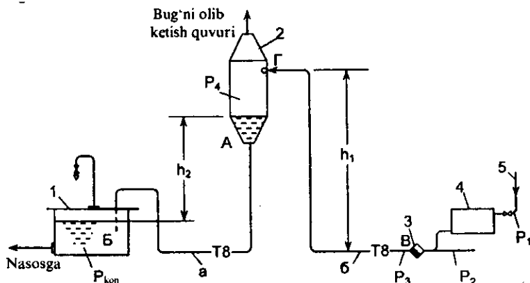
9.13-rasm. Bosim ta'siri ostidagi (a) va ikki fazali (b) kondensat uzatuvchining sxemasi: 1 – kondensat idishi; 2 – separator idish; 3 – kondensatorni olib ketuvchi; 5 – bug' uzatuvchi
