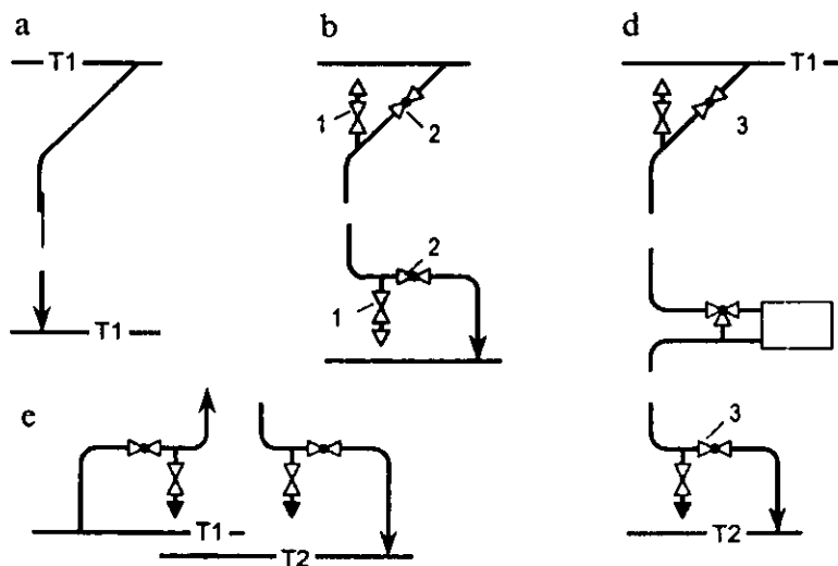
5.4-rasm. Tirgaklarni uzatuvchi va qaytaruvchi quvurlarga ulanish sxemalari
