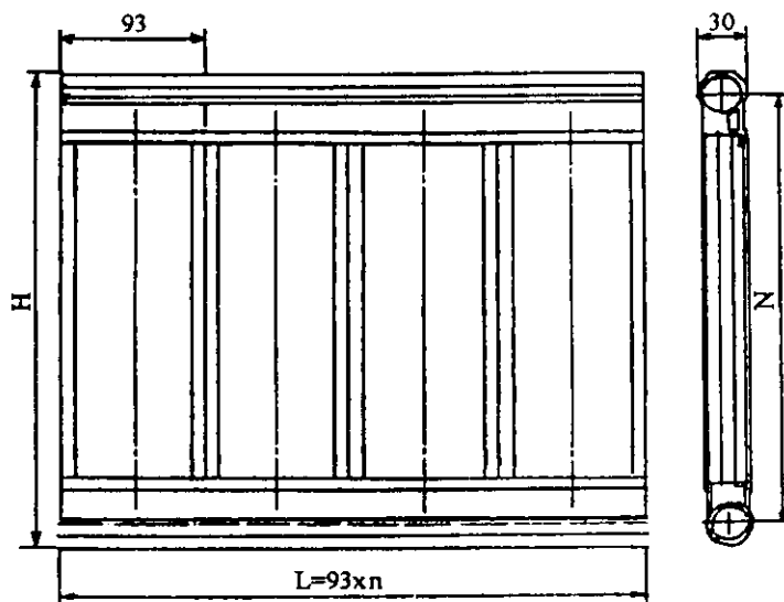
4.9-rasm. «СИАЛКО» markali radiator
