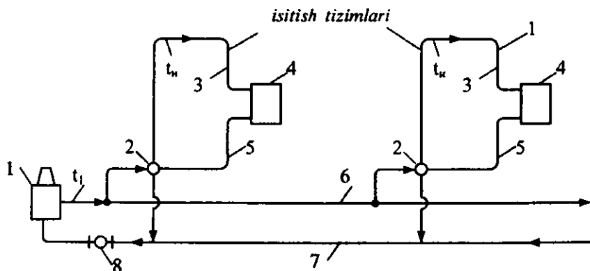
1.2-rasm. Tuman miqyosidagi isitish tizimining sxemasi: 1 – birlamchi issiqlik uzatuvchi; 2 – mahalliy issiqlik bo'limi; 3 va 5 – uzatuvchi va qaytuvchi quvurlar; 4 – isitish asboblari; 6 va 7 – magistral uzatuvchi va qaytaruvchi quvurlar; 8 – sirkulyatsion nasos
