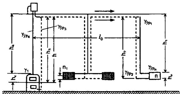
7.9-rasm. Turar joy binolaridagi isitish tizimining uzatuvchi va teskari magistral quvurlarining ship tagida o'rnatilishi
