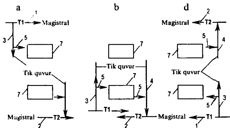
5.1-rasm. Isitish markazidan vertikal issiqlik tarqatish tizimi: a – yuqoridan tarqatuvchi; b – pastdan uzatuvchi; d – «to'ntarilgan» vertikal quvurlarda suv harakati
