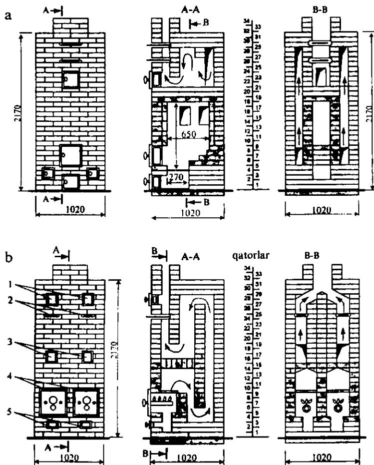
12.4 a, b – rasm. Qattiq yonilg'i bilan ishlaydigan pechlarning o'txonalarini ikkiga bo'lib ularning tashqi o'lchamini o'zgartirmasdan gaz bilan ishlaydigan o'txonalarga aylantirish: a – o'zgartirilmasdan oldingi ko'rinishi; b – o'zgartirilgandan keyingi ko'rinishi; 1 – kengaytirilgan choklar; 3 – tozalash uchun ajratilgan joy; 2 – olovdon hilini boshqarish uchun o'rnatilgan o'chirgich; 4 – gaz mash'ala dastasi (gorelka); 5 – ikkilamchi havoni boshqarish uchun o'rnatilgan eshikcha (darcha)
