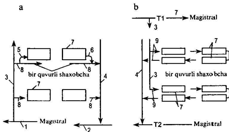
5.2-rasm Pastdan (a) va yuqoridan (b) uzatuvchi suvli gorizontal isitish tizimlari: 1, 2 - uzatuvchi va qaytaruvchi magistral; 3 va 4 – uzatuvchi va qaytaruvchi irgak; 5 va 6 – uzatuvchi va qaytaruvchi ulama; 7 – isitish asboblari; 8 – bir quvurli shaxobcha; 9 – bifilyar tarmoq
