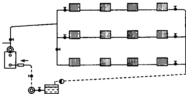
9.9-rasm. Bir quvurli gorizontall joylashgan to'liq to'g'ri harakatli va yo'lma-yo'lakay bug' kondensat harakati ta'sirida ishlaydigan bug'li isitish tizimining sxemasi
