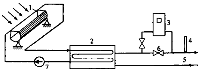
15.8-rasm. Parabolotsilindrik konsentratli va suyuq issiqlik yig'uvchi moslamali past haroratli isitish tizimi: 1 – parabolotsilindrik konsentrat; 2 – suyuqlikli issiqlik akkumulyator; 3 – qo'shimcha issiqlik manba; 4 – termometr; 5 – isitish tizimi konturi; 6 – boshqaruvchi jo'mrak; 7 – uyurmaviy nasos
