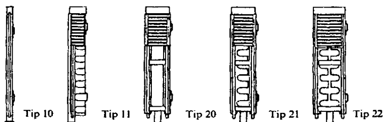
4.6-rasm. PCB-3 markali po'lat panelli radiatorlar
