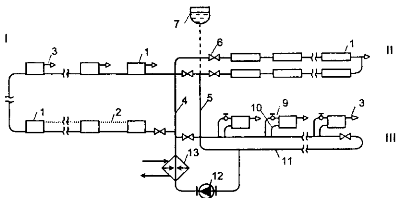
7.5-rasm. Bir quvurli gorizontaal (ko'ndalang) isitish tizimidagi isitish asboblarni taqsimlovchi magistral quvurlarga turli xil ulash sxemalari: I - gorizontaal (ko'ndalang) quyidan yuqoriga harakat qiluvchi isitish tizimi; II - quyidan yuqoriga harakat qiluvchi bifilyar isitish tizimi; III - oxirida birlashtiruvchi quvur bo'limi. 1 - isitish asbobi; 2 - havo quvuri; 3 - havo jo'mragi; 4 - taqsimlovchi tirgak; 5 - qaytuvchi tirgak; 6 - jo'mrak; 7 - kengaytiruvchi idish; 8 - konvektorlar; 9 - jo'mrak; 10 - tirgak; 11 - teskari magistral quvur; 12 - nasos; 13 - issiqlik almashgich (qozon)
