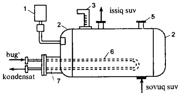
6.6-rasm. Maxsus sig'imli issiqlik almashtiruvchi uskunalar
