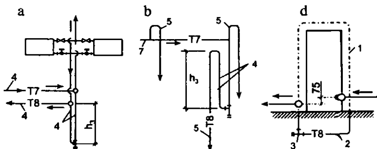
9.6a, b, d-rasm: 1 – havo quvuri; 2 – eshik ostidan izolyatsiya qilib o'tkazilgan quvur; 3 – uchtalik tiqindon; 4 – suv zulfini; 5 – kalach; 6 – kondensat tirgak
