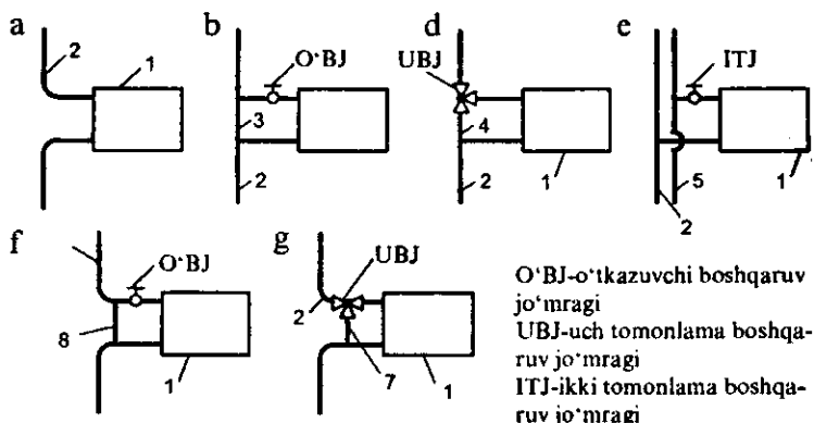
5.7-rasm. Bir (a-d) va ikki (e) quvurli vertikal isitish tizimida quvurlarning isitish asboblari bir tomonlama ulanishi: 1 - isitish asboblari; 2 - bir quvurli tirgaklar, 3 - o'qi siljiltilmagan birlashtiruvchi tirgaklar; 4 - o'qli aylanma uchastkasi; 5 va 6 - ikki quvurli tirgaklarda isitish tizimlariga issiqlik uzatuvchi va qaytaruvchi quvurlar; 7 - o'qdan siljiltilgan tutashtiruvchi quvur; 8 - siljiltilmagan tutashtiruvchi quvur
