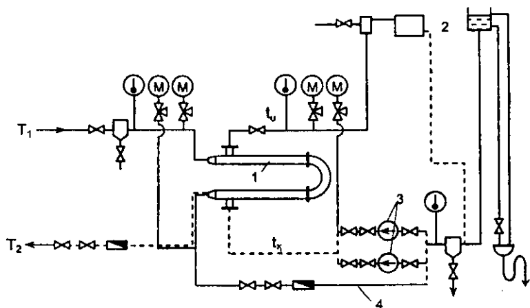
6.4-rasm. Yuqori haroratli issiqlik tashuvchi quvurlarga isitish tizimining «Bog'liq bo'lmagan holda» ulanish sxemasi
