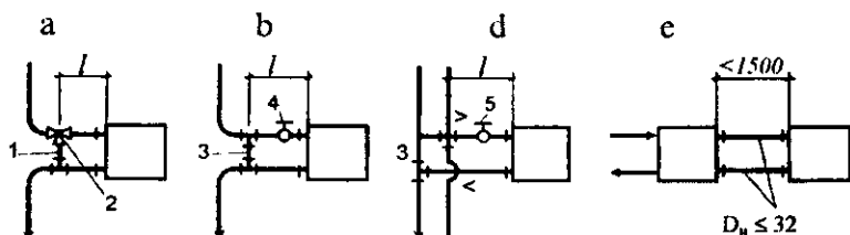
5.8-rasm. Bir quvurli (a,b), ikki quvurli (d) va yuqoridan uzatuvchi tirkaklarga isitish asboblarning ulanishi: 1 – tirkak o'qidan siljirilgan uzatma; 2 – UBJ; 3 – tirkak o'qidan siljirilgan uzatma; 4 – O'BJ; 5 – IBJ
