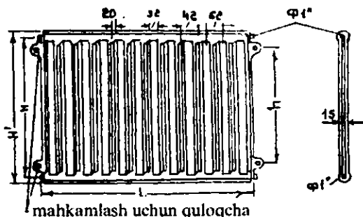
4.13.-rasm. Quyma po'lat tunukadan yasalgan radiator
