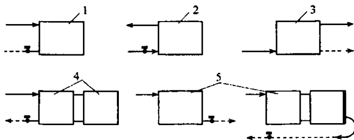
4.18-rasm. Isitish asbobining issiqlik quvurlariga ulanishi: 1 – yuqoridan pastga; 2 – pastdan yuqoriga; 3 – pastdan pastga; 4 – radiatorlarning bir-biri bilan ilgakli ulanishi; 5 – radiatorlarga quvurlarning har tomonlama ulanish ushlari
