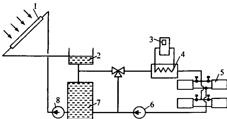
15.10-rasm. Avtomatlashtirilgan yassi kollektorlar bilan jihozlangan quyosh energiyasi bilan isitiladigan past haroratli suvli isitish tizim sxemasi: 1 – yassi quyosh kollektorlari; 2 – kengaytiruvchi sig'im; 3 – qo'shimcha issiqlik manbai; 4 – issiqlik almashtiruvchi uskuna; 5 – isitish asboblari; 6, 8 – uyurmaviy nasoslar; 7 – issiqlik yig'uvchi moslama (sig'im)
