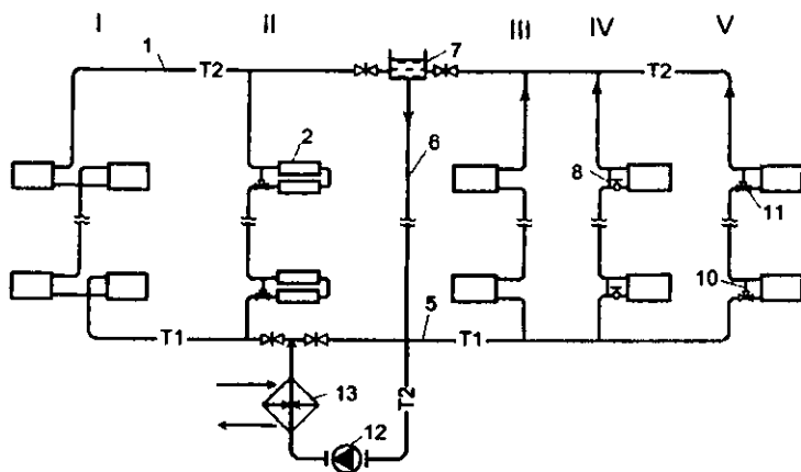
6.8, e – rasm. Quyidan taqsimlanuvchi ikki quvurli yuqoridan (a) va quyidan taqsimlanuvchi tirgaklari turli konstruksiyali isitish tizimining markaziy issiqlik tarmog'iga ulanishi: 1 va 2 uzatuvchi T1 va qaytuvchi T2 magistral quvurlar; 3 va 4 – uzatuvchi va qaytuvchi tirgaklar; 5 – isitish asbobi; 6 – jo'mrak UBJ; 7 – bosh tirgak; 8 – kengaytirish sig'imi; 9 – havo quvurlari; 10 – havo jo'mragi; 11 – kengaytirish sig'imini qaytuvchi magistral quvur bilan birlashtiruvchi quvur; 12 – nasos; 13 – issiqlik generatori
