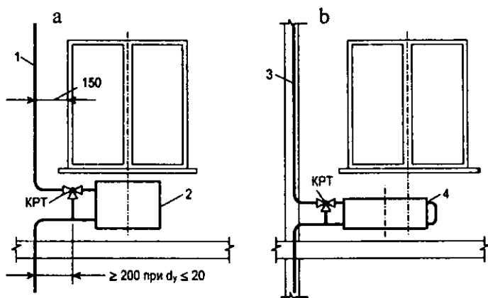
5.3-rasm. Ko'p qavatli binolarda vertikal o'rnatilgan bir quvurli suvli isitish tizimning tuzilishi (isitish asbobi oldida uch tomonlama boshqaruvchi jo'mrak o'rnatilgan): a – tirgakning deraza yonida joylashuvi (deraza va radiator o'qlari mos tushgan); b – isitish asbobining tirgak tomon siljirilgan holati; 1 – tirgak, 2 – radiator, 3 – devor ichiga qurilgan tirgak, 4 – konvektor
