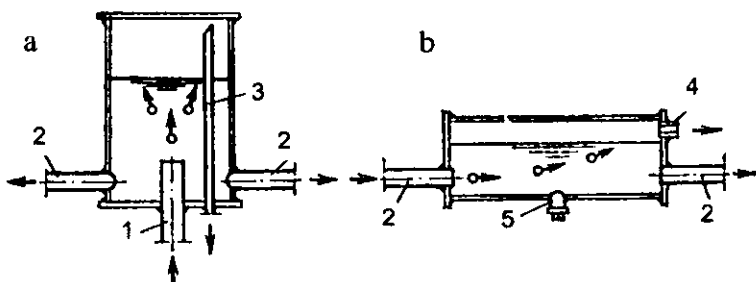
5.17-rasm. To'g'ri oqimli havo yig'uvchi uskunalar: 1 – bosh tirgak; 2 – magistral quvurlar; 3 – diametri 15 mm bo'lgan havo chiqaruvchi quvur;
