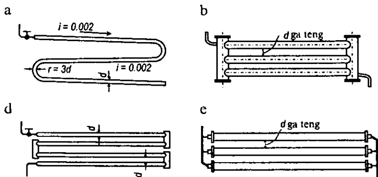
4.16-rasm. Sirti silliq quvurlardan yasalgan isitish asboblari: a – bir xil diametrli quvurdan egilib tayyorlangan; b, d – bir xil diametrli quvurdan payvandlash yo'li bilan tayyorlangan; e – silliq quvurlar uch qator qilib terilib tayyorlangan
