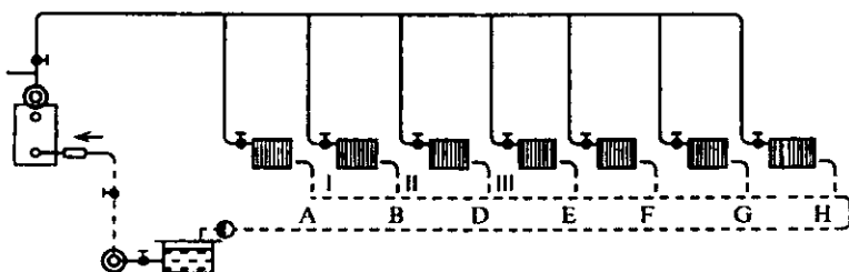
9.7-rasm. Kondensat va magistral bug' quvurlarining halqali harakatda bo'lgan ikki quvurli isitish tizimining sxemasi: 1 – bug' dan ajralayotgan suv kondensatini ajratuvchi uskuna; 2 – bug' bosimini pasaytiruvchi uskuna; 3 – ortiqcha bosim ta'sirini kamaytiruvchi moslama; 4 – tarqatuvchi kollektor; 5 – bug' miqdorini boshqaruvchi jo'mrak; 6 – kondensat ajratuvchi uskuna; 7 – kondensat idishi; 8 – havo quvuri; 9 – kondensat nasos; x – siljimas tirgak
