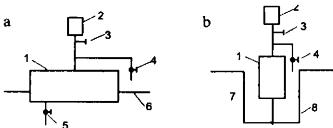
5.20 - rasm. Havo yig'uvchi uskunalar va vantuzlarning o'rnatilishi: 1 - havo yig'uvchi moslama; 2 - vantuz; 3 - ta'mirlash va taftish davrida ishlatiladigan vantuzning jo'mragi; 4 - qo'l bilan ishlatiladigan jo'mrak; 5 - havo yig'uvchi moslamaning suv chiqaruvchi quvuri; 6 - magistral quvur; 7 - havo harakati yo'li; 8 - sirtmoq shaklidagi quvur
