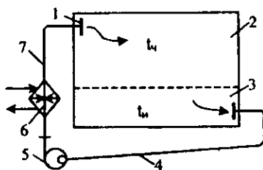
1.13-rasm. Markazlashtirilgan havoli isituvchi qurilmaning sxemasi: 1 – havo tarqatuvchi panjara; 2 – isitiladigan xona; 3 – ishchi maydon; 4 – qaytuvchi havo quvuri; 5 – havo so'rg'ich parrak; 6 – kalorifer; 7 – issiq havo quvuri
