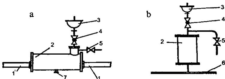
5.18-rasm. Havo yig'uvchi va havo yig'ib chiqaruvchi uskunalar: 1 – magistral quvur; 2 – havo yig'uvchi uskuna; 3 – havo yig'uvchi quvurlarning moslamasi; 4 – jo'mraklar; 5 – havo jo'mragi; 6 – havo yig'uvchi quvur; 7 – cho'kindi chiqaruvchi moslama
