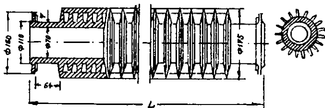
4.15-rasm. Qovurg'ali cho'yandan quyilgan quvur shaklidagi isitish asbobi: a – yotiq holatda o'rnatilgan turi; b – tik holatda o'rnatilgan turi
