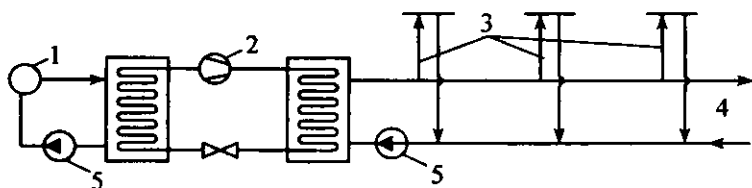
15.12-rasm. Issiqlik nasoslari yordamida geotermal suv haroratini ko'tarib markazlashtirilgan isitish qurilmalarida ishlatilgach, qaytayotgan suvni yana yer tagiga yuborish sxemai: 1 – issiq suv chiqaradigan quduq; 2 – issiqlik almasigan; 3 – issiqlik iste'molchilari; 4 – geotermal issiq suv quvurlari; 5 – uyurmaviy nasoslar
