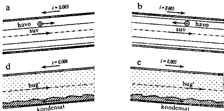
5.6-rasm. Isitish asboblari issiqlik tashuvchining harakat yo'nalishi hamda taklif qilingan va ruxsat etilgan qiyalik darajasi: a va b – yuqoridan tarqatiluvchi issiq suvli isitish qurilmalarida; d va e – issiqlik tashuvchi bug' bo'lgan holda
