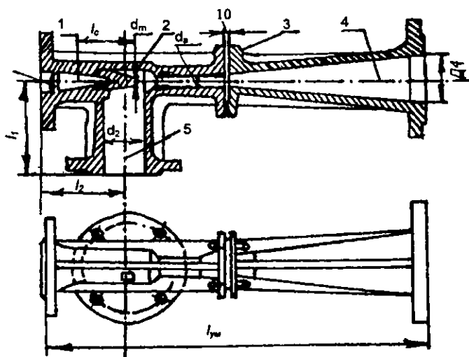
6.3-rasm. Issiq suv aralashmasini hosil qiluvchi elevator
