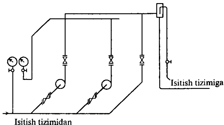
7.7 - rasm. Issiqlik tashuvchini harakatga keltiruvchi nasoslarning isitish tizimiga ulanishi
