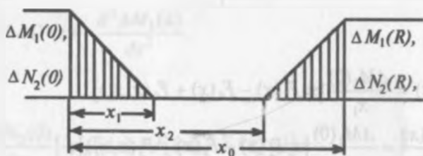
4.1- chizma. Eguvchi moment va balqa kuchlarining noxiziqli komponentlari o'zgarishi.
