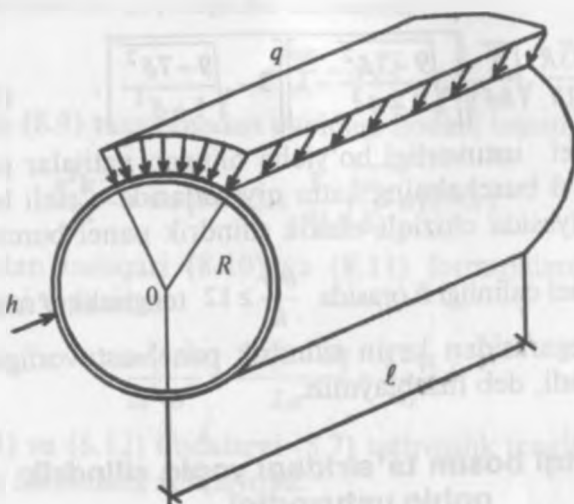
5.9- chizma. Tashqi bosim ta'sirida bo'lgan silindrik qobiq.
