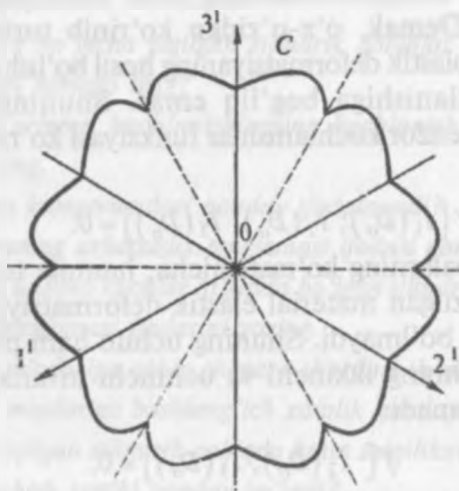
3.1- chizma. Plastiklik egri chizig'i.
