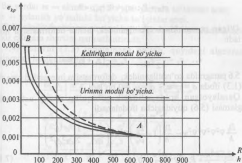
5.6- chizma. O'qqa simmetik to'lqin hosil bo'lganda kritik deformatsiyaning qobiq nisbiy qalinligiga bog'liqlik grafigi.
