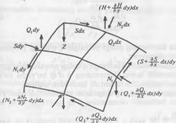
5.1- chizma. Qobiqning o'rta sirtiga ta'sir etuvchi zo'riqishlar.
