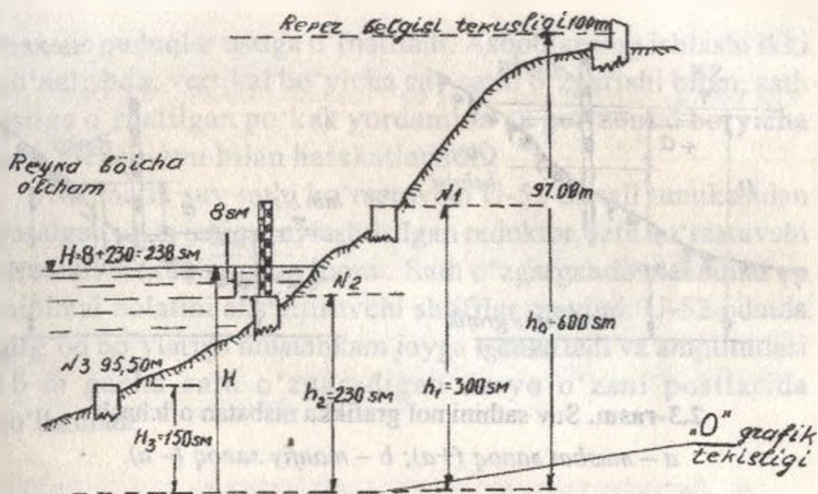
2.2-rasm. Qoziqli gidrologik postda o'lganadigan suv sathi balandligining belgilari va sanoqlari chizmasi
