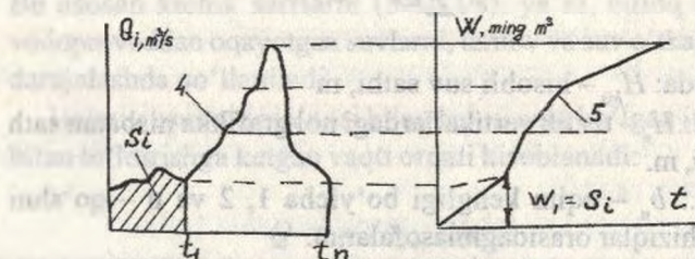
2.24-rasm. Suv sarfi gidrografi (4) va oqim hajmi grafigi (5)
