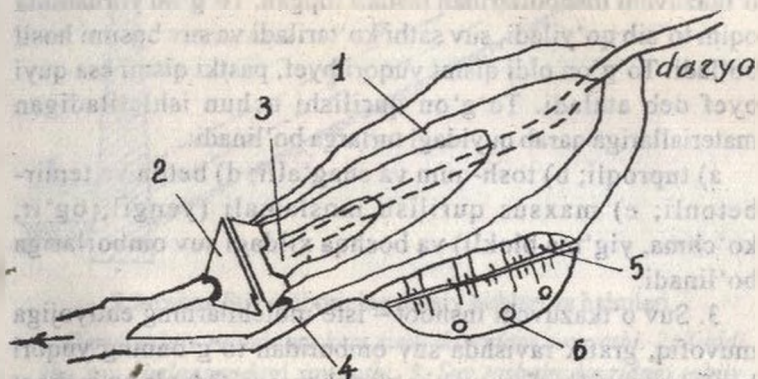
3.8-rasm. Suv ombori va uning inshootlari
