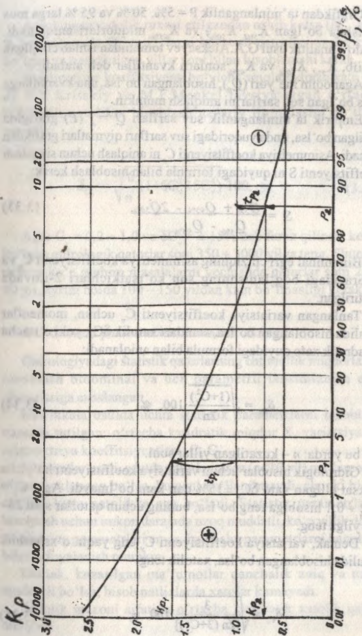
3.3-rasm. C_v=0,3 va C_s=2C_v ga teng bo'lganda ta'minlanganlikning analitik egri chizig'ining ko'rinishi.
