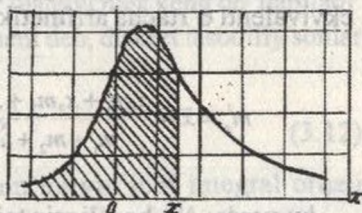
3.2-rasm. Tasodifiy sonlarning taqsimlanish egri chizig'i
