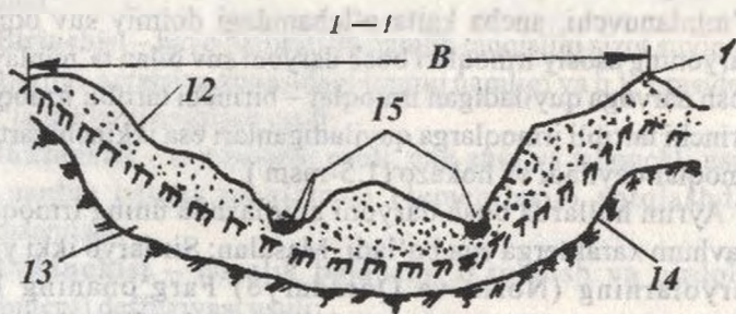
1.6-rasm. Havzaning ko‘ndalang kesimi
