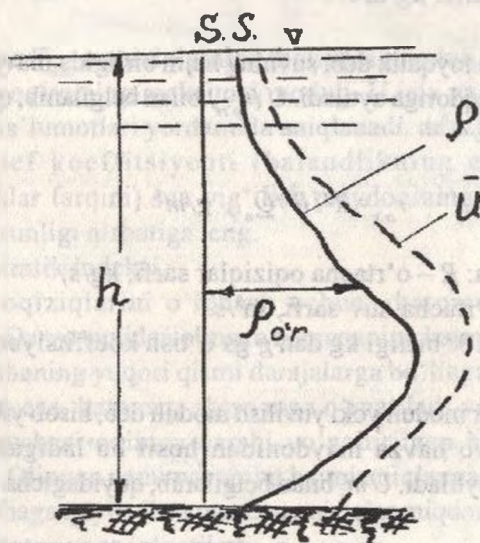
2.27-rasm. Oqizqlarni chuqurlik bo'yicha taqsimlanishi:
