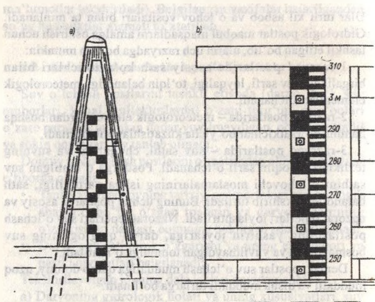
2.1-rasm. Reykali postlar:
