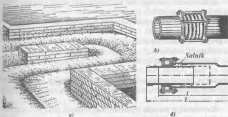
9-rasm. Issiqlik tarmoqlarida ishlatiladigan kompesatorlar:
