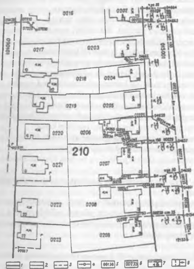
2-rasm. 1:500 masshtabdagi suvo'tkazgich kadastr planining sxemasi.
