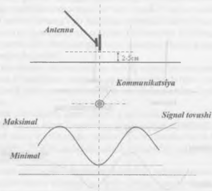
47-rasm. «Kommunikatsiyani» minimum signali bo'yicha qidirish sxemasi.
