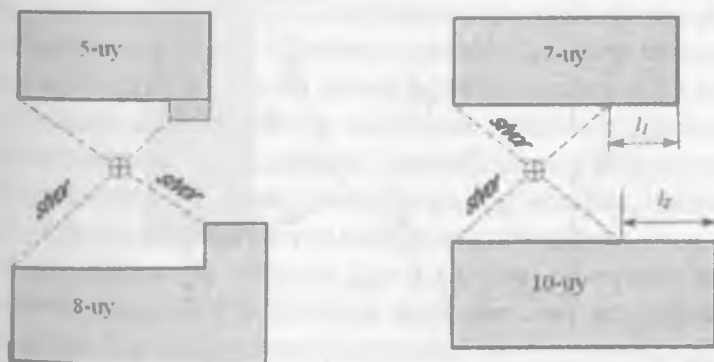
31-rasm. Kanalizatsiya qudug'ining stvorlar usulida planga olish sxemasi.
