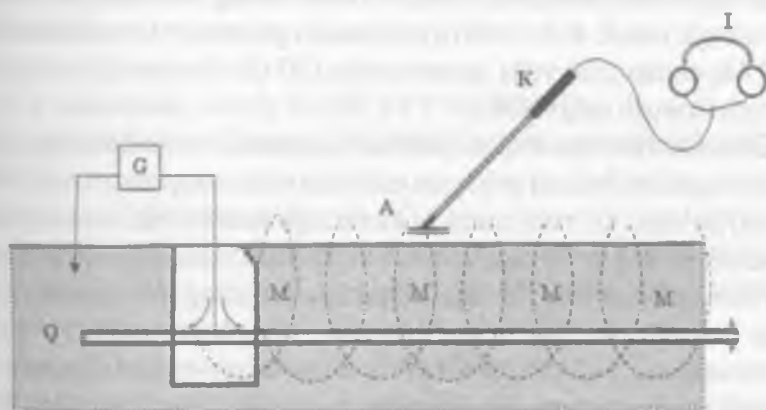
44-rasm. To'ko'tkazuvcn yerosti kommunikatsiyalarini aniqlash sxemasi
