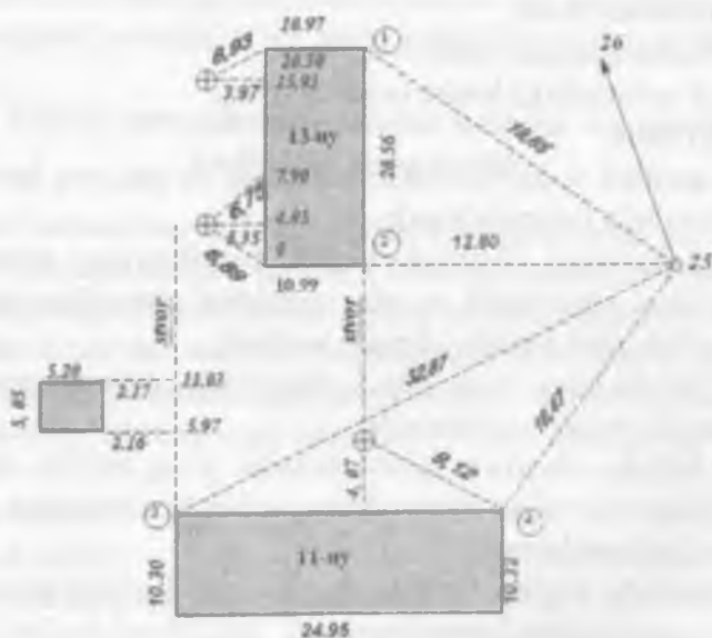
17-rasm. Turli usullarda gorizontol planga olishning abrisi.
