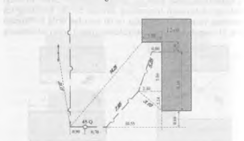
32-rasm. Gazo'tkazgich tarmoq trassasini kombinatsiya usulida planga olish sxemasi.
