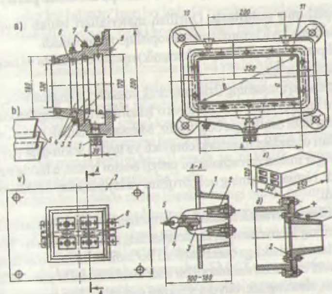
27-rasm. Lentasimon presslarning mundshtuklari: a-normal konstruksiyali mundshtuk, b-ichki qoplama, v-to'rt teshikli mundshtuk, g-4 ta teshikli g'isht, d-bug' bilan isitiladigan mundshtuk, l-po'lat list, 2-nasadka, 3-kernlar, 4-kern tutgich,
