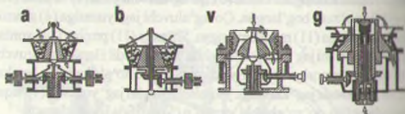
5-rasm. Konussimon maydalagichlar: a - yuqori tayanchli harakatlanuvchi valli, b - quyi tayanchli harakatlanuvchi valli, v - harakatlanuvchi valli, g - gidravlik amortizatori.
