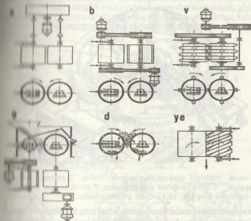
8-rasm Valli maydalagich: a-yuzasi tekis valli, b- yuzasi notekis valli, v- yuzasi tish bilan qoplangan valli, g - tekis-notekis valli, d - teshik valli, ye - vint yuzaga ega valli.
