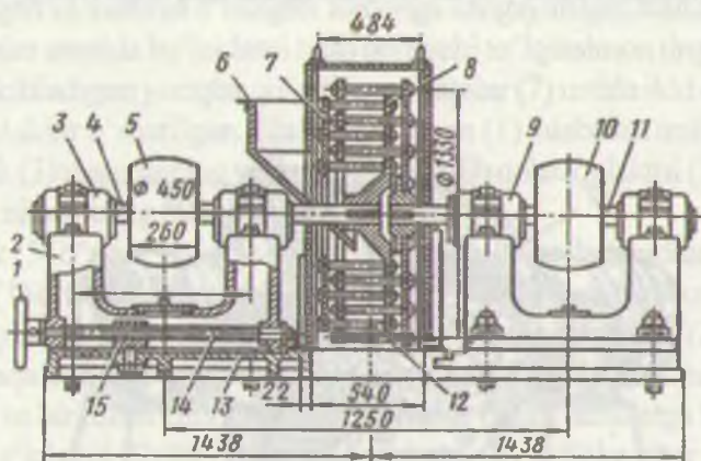
15-rasm. Ikki rotorli dezintegrator: 1 - maxovik, 2 - ustun, 3,9 - podshipnik, 4,11 - o'q, 5,10 - shkiv, 6 - qabul qiluvchi quti, 7 - po'lat disk, 8 - halqa, 12 - maydalovchi jismlar billar, 13 - tayanch plita, 14 - vint, 15 - gayka.
