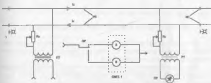
Рис. 5. Схема рельсовой цепи при отсутствии подвижной единицы.
