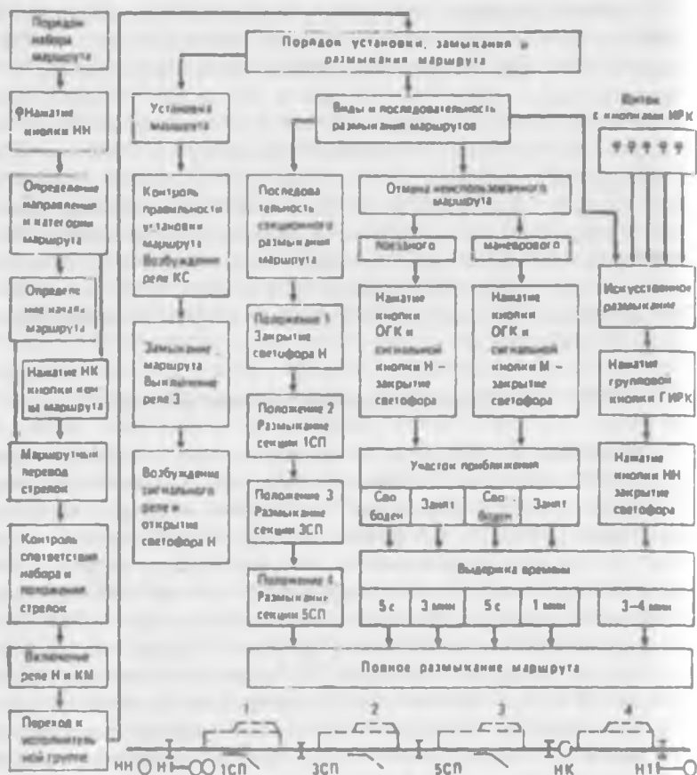
Рис. 9. Схема режимов работы БМРЦ.
