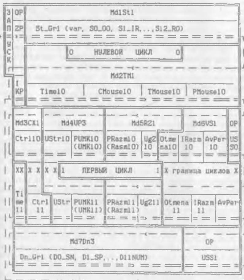
Рис. 21. Структурная схема программы компьютерной централизации.
