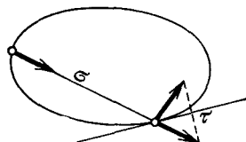
Рис. 261. Бильярдное преобразование как произведение двух инволюций
