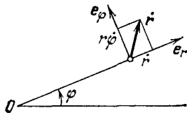
Рис. 29. Разложение вектора \dot{\mathbf{r}} по базису e_r, e_\varphi
