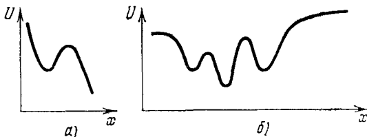
Рис. 11. Потенциальная энергия
