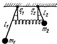
Рис. 84. Связанные маятники
