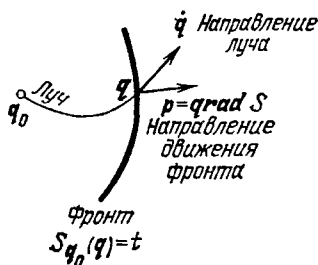
Рис. 195. Направление луча и направление движения фронта
