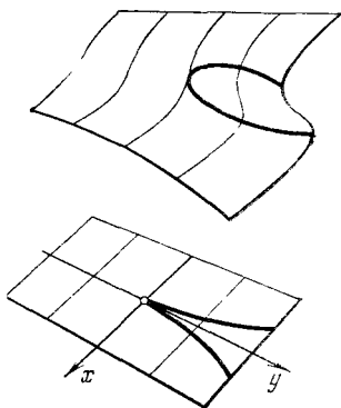
Рис. 245. Сборка Уитни
