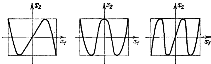
Рис. 24. Многочлены Чебышева
