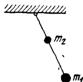
Рис. 87. Предельный случай маятников, связанных бесконечно жесткой пружиной
