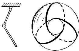
Рис. 191. Периодическое движение двойного маятника
