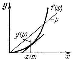
Рис. 43. Преобразование Лежандра
