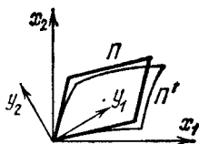
Рис. 159. Независимость внешней производной от системы координат
