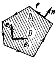
Рис. 152. Ориентация границы
