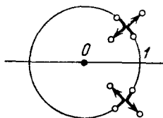
Рис. 178. Поведение кратных собственных чисел при малом изменении симплектического преобразования
