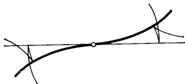
Рис. 264. Эволюенты кубической параболы
