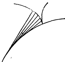
Рис. 252. Особенность эволюенты гладкой кривой
