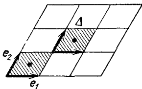
Рис. 216. К задаче 7
