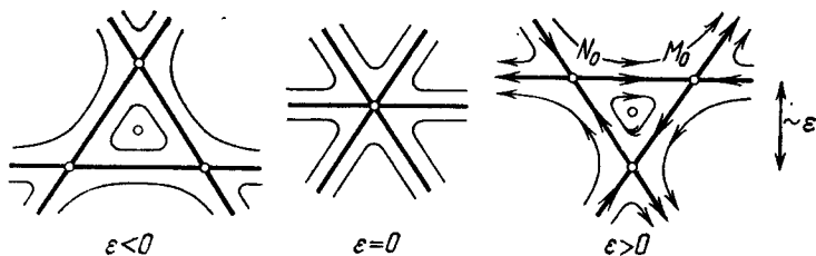
Рис. 239. Прохождение резонанса 3 : 1
