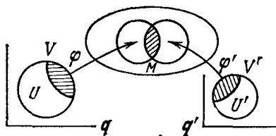
Рис. 56. Совместные карты
