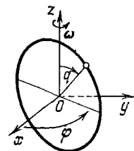
Рис. 68. Бусинка на вращающейся окружности
