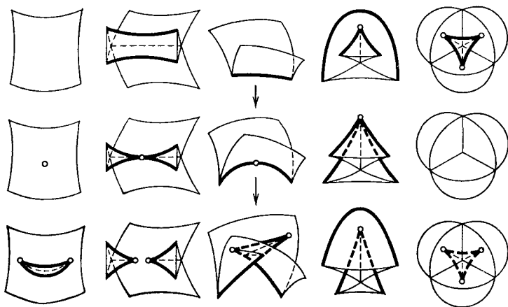
Рис. 258. Типичные перестройки волновых фронтов
