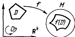
Рис. 150. Сингулярный k -мерный полиэдр
