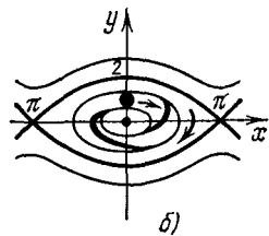
Рис. 15. Действие фазового потока на круг
