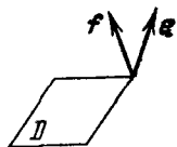
Рис. 174. Косоортogonalное дополнение
