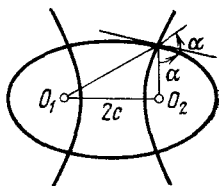
Рис. 204. Эллиптические координаты
