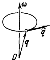
Рис. 105. Угловая скорость
