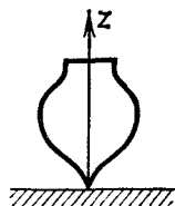
Рис. 129. Спящий волчок
