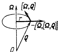
Рис. 108. Центробежная сила инерции
