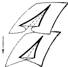
Рис. 263. Раскрытый ласточкин хвост
