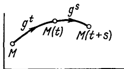
Рис. 14. Фазовый поток
