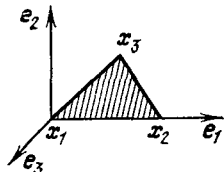
Рис. 112. Конфигурационное многообразие твердого тела
