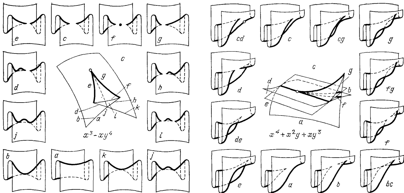
Рис. 260. Двадцать четыре вида двух поверхностей
