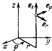
Рис. 145. К задаче 13
