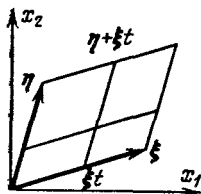
Рис. 158. К теореме о внешней производной
