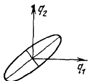
Рис. 85. Потенциальная энергия сильно связанных маятников
