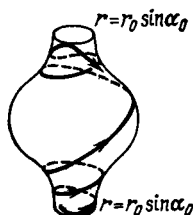
Рис. 67. Геодезические на поверхности вращения
