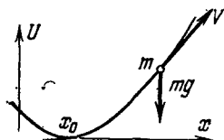
Рис. 77. Бусинка на проволоке
