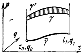
Рис. 187. Принцип наименьшего действия в фазовом пространстве
