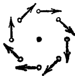
Рис. 27. Непотенциальное поле
