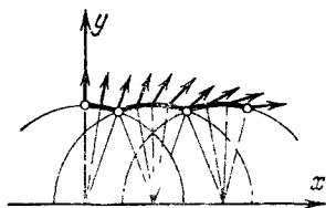
Рис. 232. Параллельное перенесение на плоскости Лобачевского
