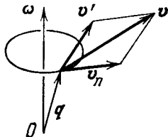
Рис. 106. Сложение скоростей
