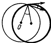
Рис. 36. Орбита, близкая к круговой
