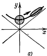
Рис. 15. Действие фазового потока на круг
