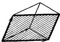
Рис. 136. Ориентированная площадь — 2-форма
