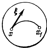
Рис. 157. Интеграл по
