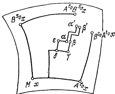
Рис. 171. Криволинейный четырехугольник |убеа
