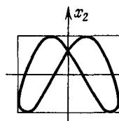
Рис. 23. Серия фигур Лиссажу с \omega = 2
