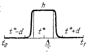
Рис. 42. Построение функции h
