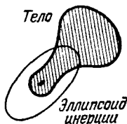
Рис. 116. Эллипсоид инерции
