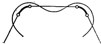
Рис. 262. Кратчайший путь в обход препятствия
