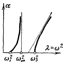
Рис. 86. Зависимость собственных частот от жесткости пружины
