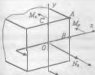
65-rasm. Buralish, cho'zilish va egilish bir bo'lganda kuchlanishlarni hisoblash modeli.
