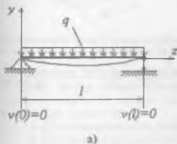
48-rasm. Chegaraviy shartlarga misollar: a) ikki tayanchli; b) konsol balka.
