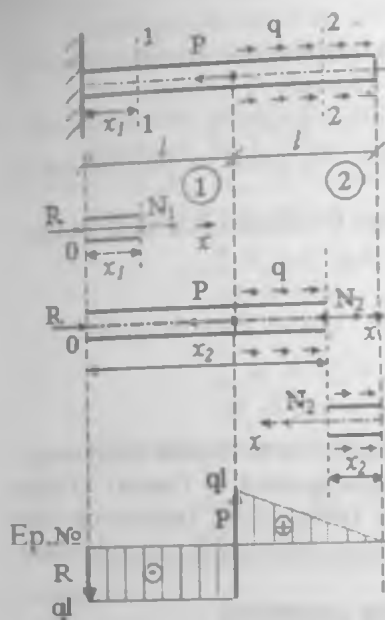
4-rasm. Cho'zilish-siqilishda normal kuchlar epyurasini qunsh
