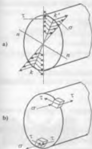
64-rasm. Valning kuchlangan holati: a) kuchlanishlar epyurasi; b) kuchlanishlar taqsimoti
