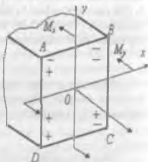
61-rasm. Momentlar ta'siri bo'yicha ishoralarni qo'yish
