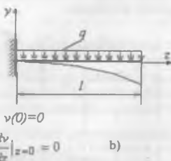
48-rasm. Chegaraviy shartlarga misollar: a) ikki tayanchli; b) konsol balka.
