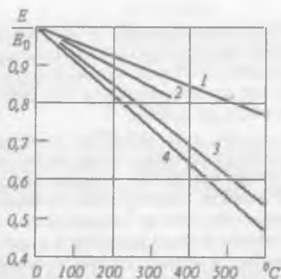
32-rasm. Elastiklik modulining temperaturaga bogʻliqligi.
