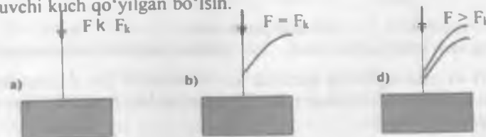
67-rasm. Sterjenlarda a) ustuvor; b) bevarq; d) noustuvor muvozanat holatlari.
