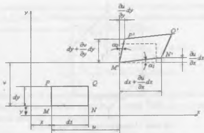
21-rasm. Yassi deformatsiya.
