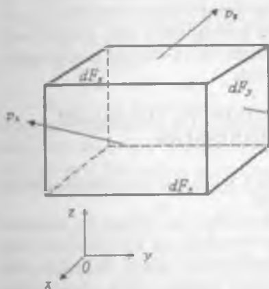
14-rasm. Cheksiz kichik parallelepipedning muvozanat holati
