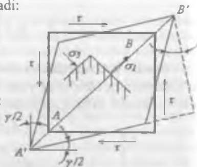
23-rasm. Yassi siljish deformatsiyasi.
