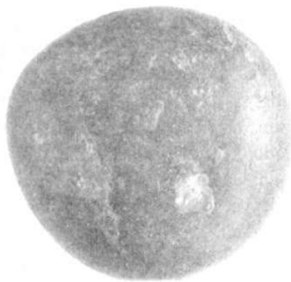
53- rasm. Fosforit.
