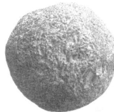
18- rasm. Fosforit.
