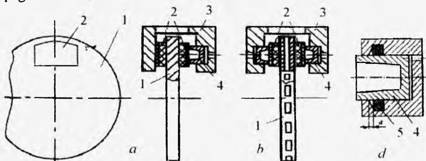
89-rasm. Ochiq tipdagi diskli tormoz.
