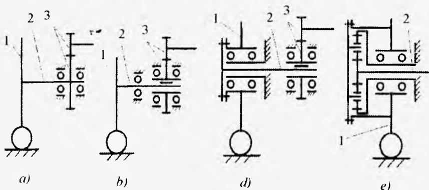
53-rasm. Yarim o'qlarning yuklanishi bo'yicha xillari.
