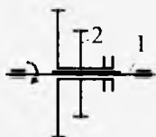
Shlitsali o'q bilan siljivchi shlitsali silindrsimon shesterniyalar bloki (karetk). 1-shlitsali o'q; 2-siljivchi shlitsali silindrsimon shesterniyalar bloki yoki karetk.
