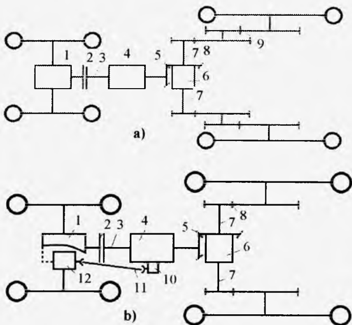
10-rasm. Modernizatsiyalashgan traktorlar transmissiyasining birinchi an'anaviy sxemasi:
