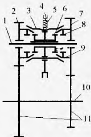
26-rasm. Sinxronizator o'rnatilgan shesternyali ilashishning sxemasi: 1-birlamchi o'q; 2,7-erkin o'tirgan shesternyalar; 3-qisuvchi halqa; 4-yo'naltiruvchi qurilma; 5-prujinali cheklagich; 6-sinxronizatorning tishli muftasi; 8-tishli toji; 9-gubchak; 10-ikkilamchi o'q; 11-qo'zg'almas shesternyalar.
