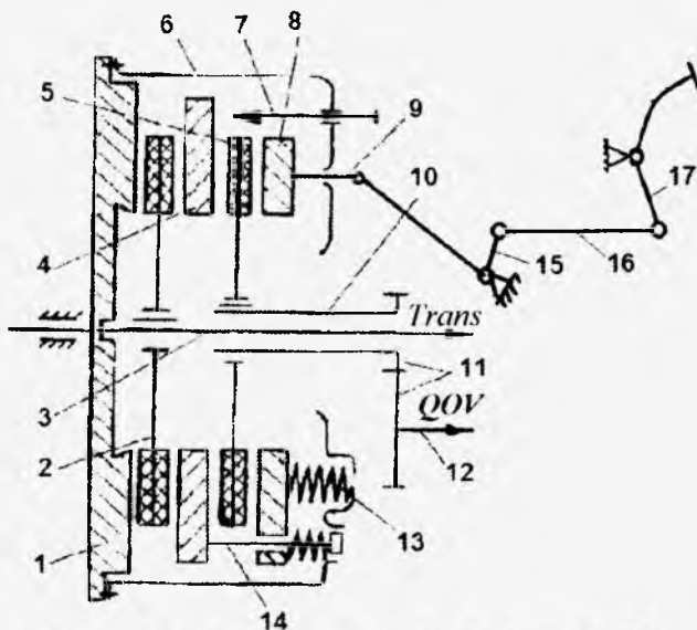
19-rasm. Birgalikda boshqariladigan ilashish muftasining sxemasi: 1-maxovik; 2-ilashish muftasini asosiy yetaklanuvchi disk; 3-ilashish muftasining o'qi; 4-o'rtadagi yetakchi disk; 5-QOV' muftasini yetaklanuvchi disk; 6-qobig'; 7-o'rtadagi yetakchi diskni qaytishini cheklovchi vint; 8-qisuvchi disk; 9-tortqi-qaytargich; 10-QOV'ni g'ovak vali; 11-QOV'ning shesternyali uzatmasi; 12-QOV'ning o'qi; 13-qisuvchi prujina; 14-prujinali tortqi; 15-ikki yelkali richag; 16-tortqi; 17-tepki.
