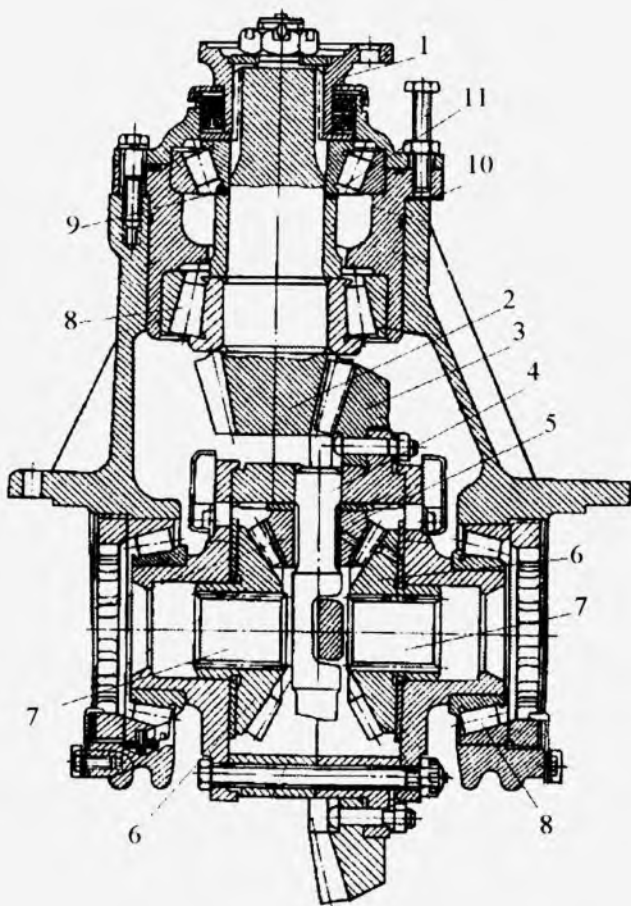
48-rasm. Bir juftli bosh (markaziy) uzatmaning tuzilishi.
