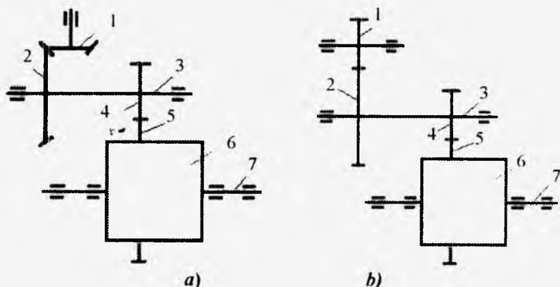
49-rasm. Ikki juftli bosh (markaziy) uzatmaning kinematik sxemasi:
