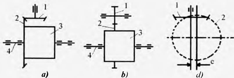
47-rasm. Bir-pog'onali bosh (markaziy) uzatmaning kinematik sxemalari.
