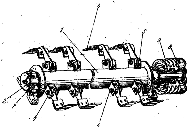
11.3-rasm. Rotorning umumiy ko'rinishi: 1-truba; 2-stapfa; 3-quloqcha; 4-bolt; 5-tayanch vtulkalar; 6-pichoq; 7-podshipnik; 8-o'zdirish muftasi; 9-yurituvchi shkiv
