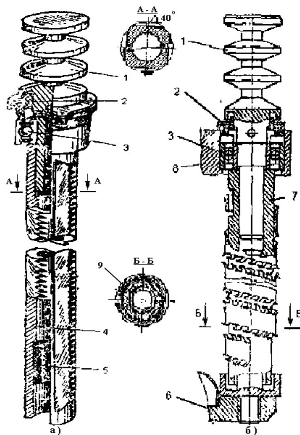
14.4-rasm. Vertikal shpindellar: a)yaxlit; b)tarkibiy; 1-rolik;
