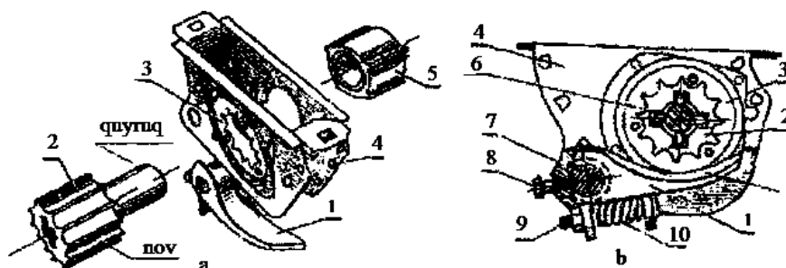
5.2-rasm. Novli-g'altakli ekish apparati: 1-apparat klapani; 2-novli g'altak; 3-rozetka; 4-apparat korpusi; 5-aylanmaydigan mufta; 6-apparatlar vali; 7-klapani ochish valiki; 8-mahkamlash bolti; 9-rostlash bolti; 10-prujina
