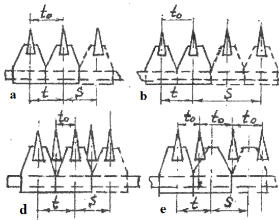
10.2-rasm. Segment - barmoqli qirqish apparatlarining turlari: a-bir yo'l o'tadigan pichoqli; b-ikki yo'l o'tadigan pichoqli baland qir-qish; d-past qirqish; e-o'rtacha qirqish apparatlari; t -segmentlar qadami; t_0 -barmoqlar (yoki qarshi qirqish plastinalari) qadami; S - pichoq yo'li
