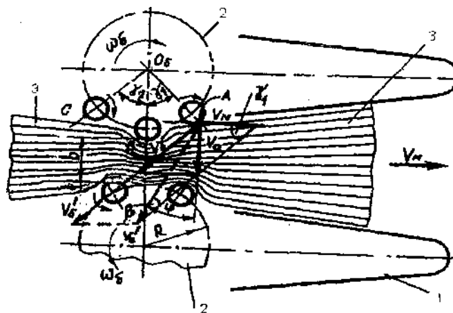
14.5-rasm. G'ozapoyalar shpindel bilan A nuqtada uchrashadi. G'ozapoyalar shpindel barabanlar ta'sirida ish tirqishiga faol tortilishi uchun A nuqtaning v_a absolyut tezligi v_m mashina tezligiga qarshi yo'nalgan bo'lishi lozim. Absolyut tezlik baraban v_b va mashina v_m tezliklarining geometrik yig'indisiga teng:
