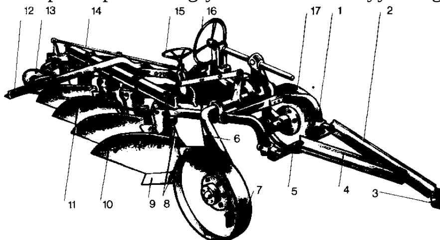
2.1-rasm. PP-5-35 rusumli tirkalma plug: 1 - rama; 2 - bo'ylama tortqi; 3 - ilgak; 4 - kashak; 5 - ko'ndalang planka; 6 - egat g'ildiragining o'qi; 7 - egat g'ildiragi; 8 - chimqirqar; 9 - lemex; 10 - ag'dargich; 11 - cho'zish plankasi; 12 - borona uchun tirkalma; 13 - orqa g'ildirak; 14 - tortqi plankasi; 15 - egat g'ildiragi mexanizmi; 16 - dala g'ildiragi mexanizmi; 17 - dala g'ildiragi
