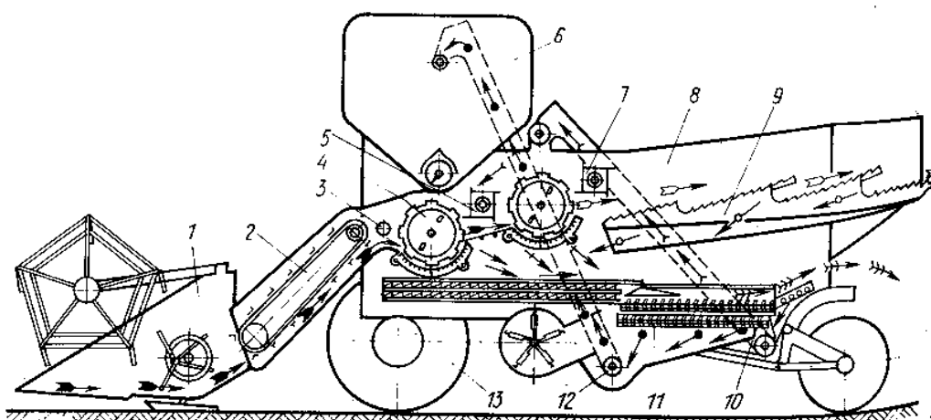
12.1-rasm. SKD-6 “Sibiryak” g’alla yig’ish kombaynining sxemasi:
