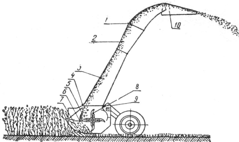
18.2-rasm. Rotorli oʻtoʻrgich-maydalagichining texnologik ish jarayoni sxemasi 1;2-nov seksiyasi; 3-yoʻnaltiruvchi truba; 4-rama; 5-qarshilik plastinasi; 6-pichoq; 7-yoʻnaltiruvchi toʻsiq; 8-rotorli baraban; 9-ketingi toʻsiq; 10-diffuzor
