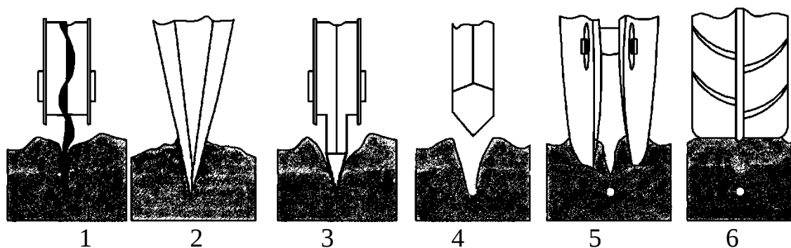
8.2-rasm. CASE-1200 pnevmatik seyalkaning texnologik ish jarayoni sxemasi: 1 – yerni kesish va tor egat ochish; 2 – egat ochish; 3 – egat tubini zichlash; 4 – urug' o'tkazish; 5 – urug'larni ko'mish; 6 – tuproqni zichlash
