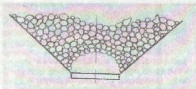
1.10- rasm. Bunkerning chiqaruvchi tuynugi ustidagi gumbaz.
