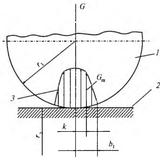
57-rasm. Qarshilik koeffitsientini aniqlash sxemasi:
