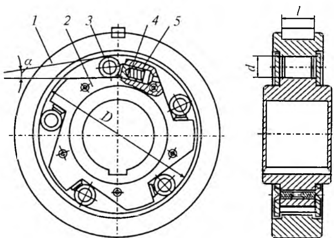
43-rasm. Rolikli to'xtatgichlar.
