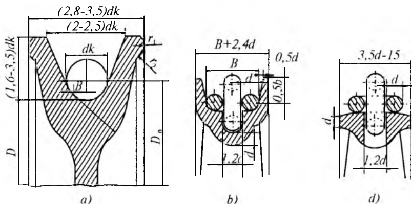
21-rasm. Yo'naltiruvchi bloklar gardishining shakli.
