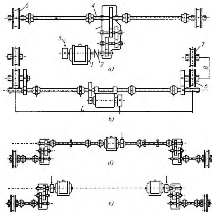
60-rasm. Ko'priqli kran siljitish mexanizmining sxemalari: a — sekinyurar valli; b — o'rta tezlik bilan harakatlanuvchi valli; d — tezyurar valli; e — alohida yuritmal.
