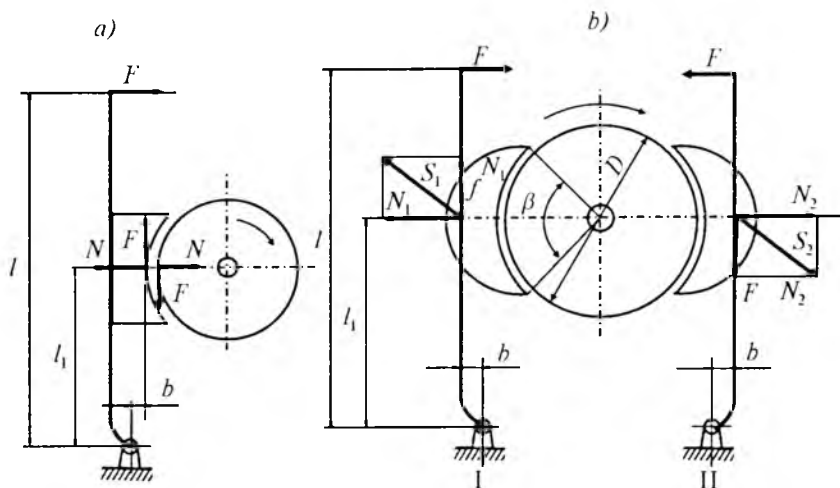
45-rasm. Kolodkali tormozlar sxemasi.
