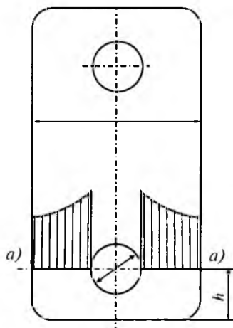
32-rasm. Oзма jag'ining hisobiy sxemasi.
