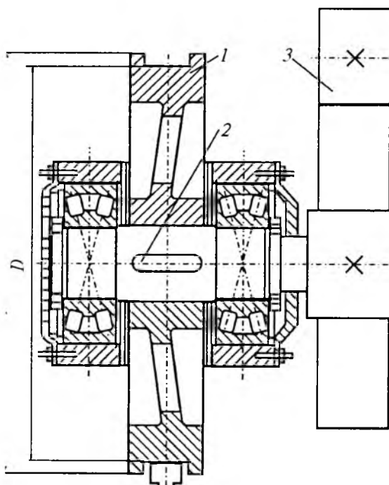
55-rasm. Yuruvchi g'ildirak: 1 — g'ildirak; 2 — val; 3 — tishli uzatma.
