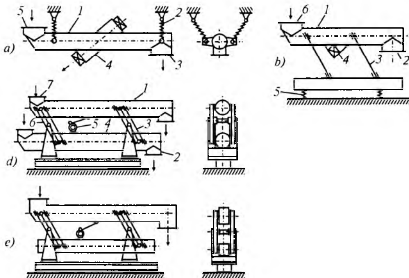
130-rasm. Vibratsion konveyerlar.
