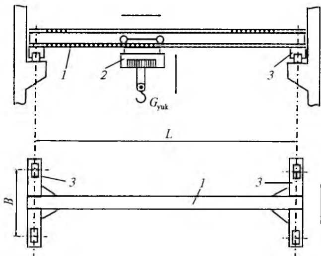
11-rasm. Tayanchga o'rnatilgan kran balka:
