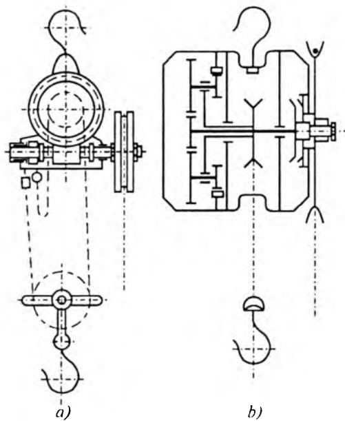
73-rasm. Dastaki tal sxemasi: a — chervyakli uzatmali; b — tishli uzatmali.
