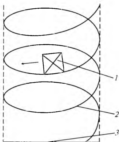
83-rasm. Vintsimon gravitatsion qurilmada yuk tushirish sxemasi: 1 — yuk; 2 — vintsimon qurilmaning ishchi qismi; 3-yuk to'xtatish qismi.
