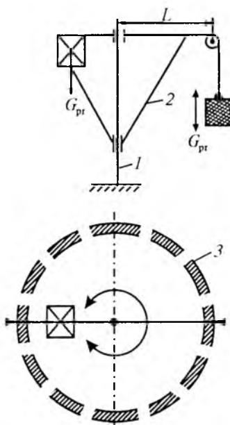
10-rasm. Qulochi o'zgarmas to'liq aylanuvchi strelali kran:
