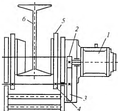
77-rasm. Mashina yuritmal siljitish mexanizmi kinematik sxemasi.
