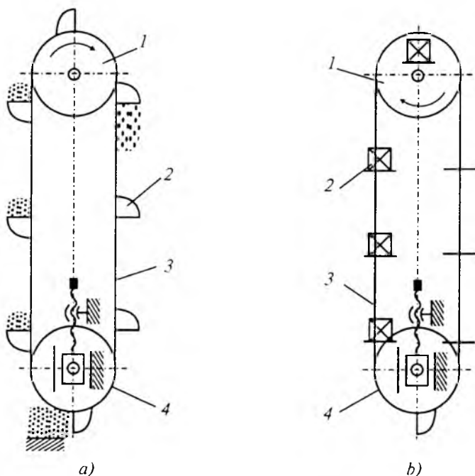
98-rasm. Elevator sxemasi.
