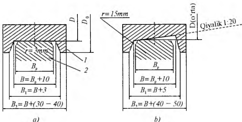
56-rasm. Yuruvchi g'ildirak:
