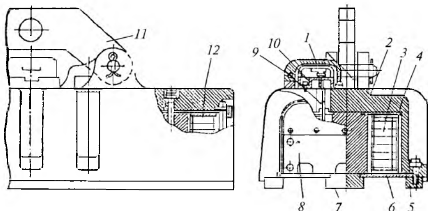
40-rasm. To'g'ri to'rtburchakli elektromagnit.
