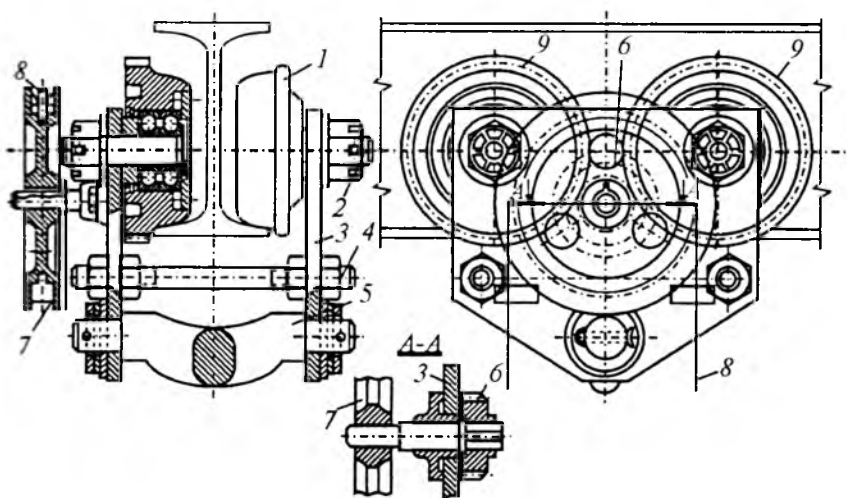
75-rasm. Dastaki siljitish mexanizmli tal aravachasi.
