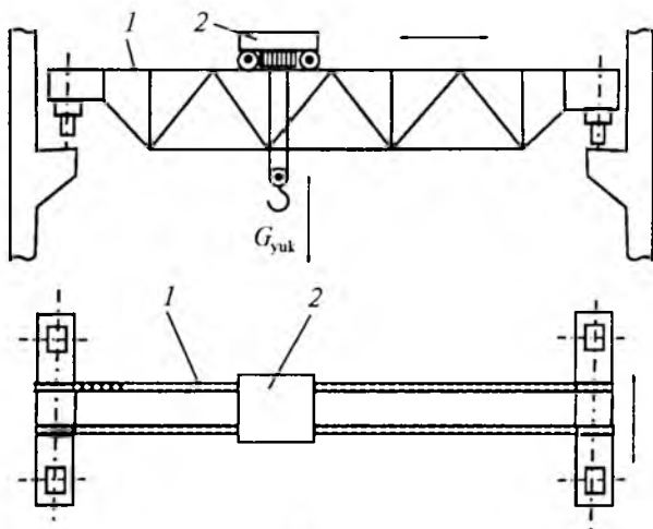
13-rasm. Ko'prikli kran sxemasi: 1 — asosiy balka — ko'prik; 2 — aravacha.
