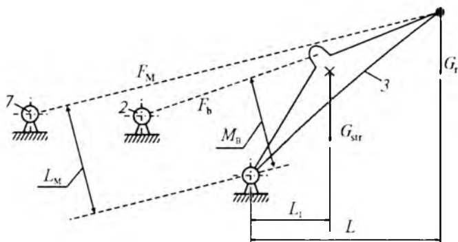
68-rasm. Kran qulochini o'zgartiruvchi kuch miqdorini aniqlash sxemasi:
