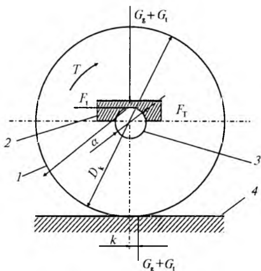
58-rasm. Siljishga qarshilikni aniqlash sxemasi:
