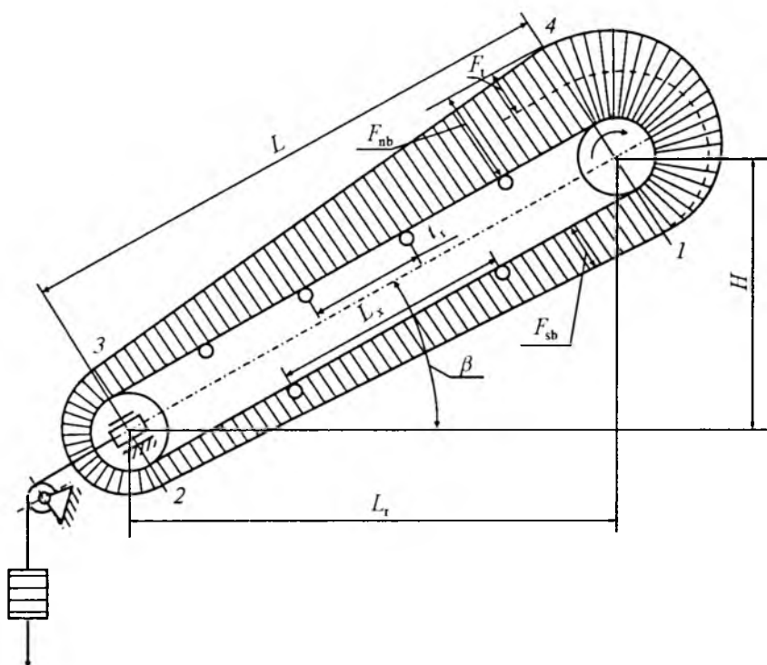
III-rasm. Tasmali konveyerni hisoblash sxemasi.
