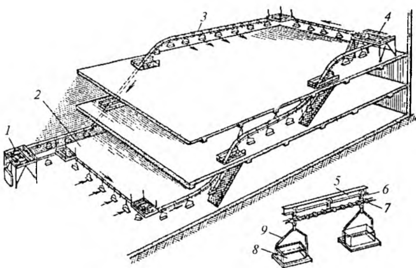
117-rasm. Osm konveyer sxemasi:
