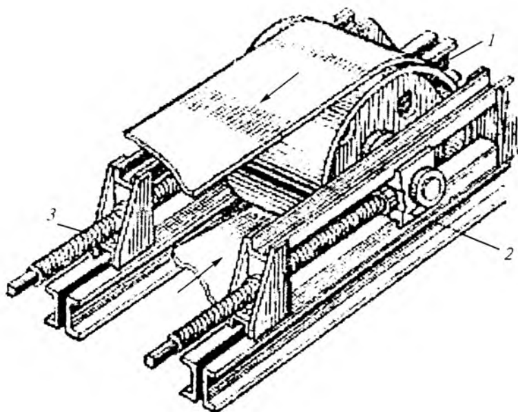
105-rasm. Vintli taranglovchi qurilma.
