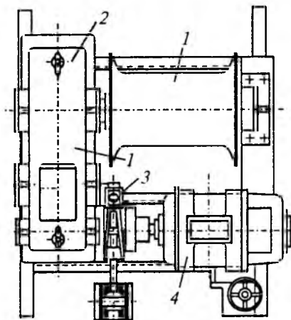
72-rasm. Elektr yuritmalı lebyodkalar.
