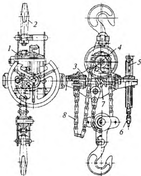
74-rasm. Chervyakli uzatmali tal.
