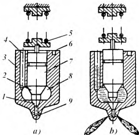
8.10- rasmi. Yopiq forsunkaning ishlash sxemasi:
