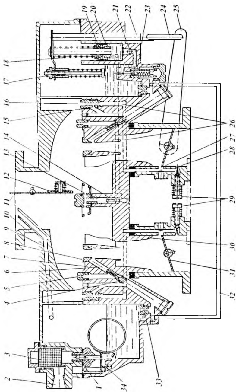
7.1-расм. К-88 А карбураторни схемаси.
