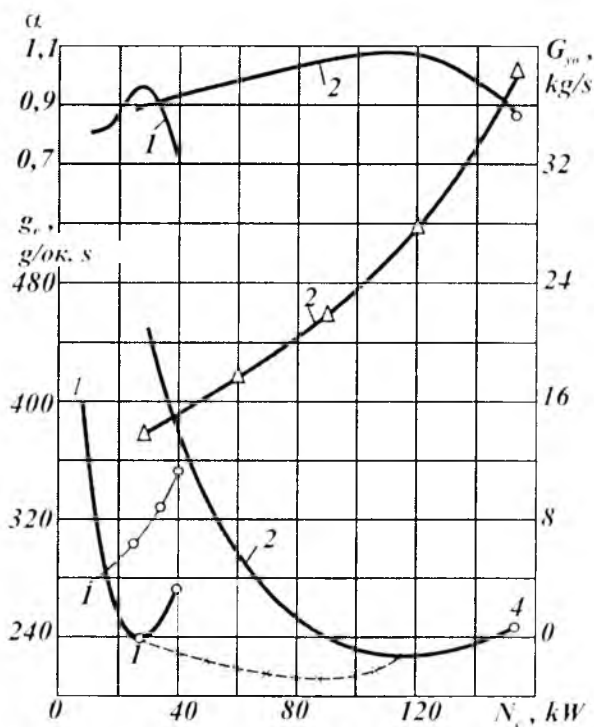
10.5-rasm. 3ИЛ-130 dvigateling yuklama tavsiflari.
