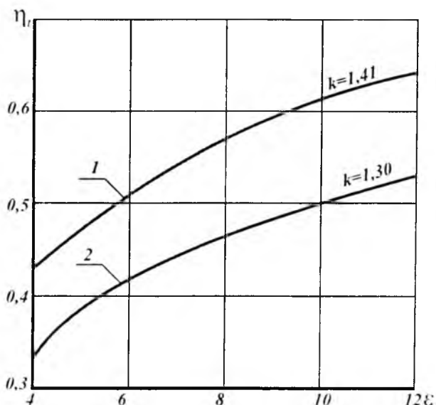
2.3-rasm. Issiqlik V = \text{const} da beriladigan sikl uchun \eta_t ning \epsilon ga bog'liqlik grafigi ( k ning ikki qiymati uchun).
