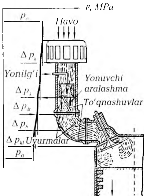
5.1-rasm. Karburatorli dvigatelning kiritish sistemi bo'ylab zaryad harakatining sxemasi.
