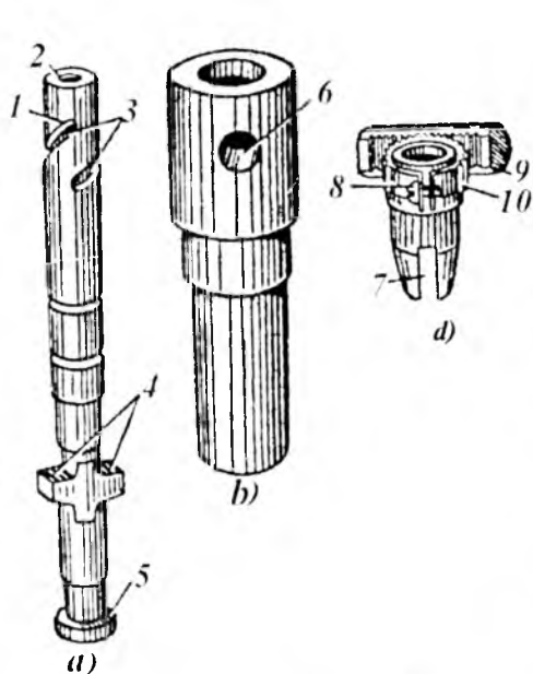
8.2-rasm. ЯМ3-236 dizeli yonilg'i nasosi seksiyasining detallari: a – plunjer; b – gilza; d – vtulka va reyka.
