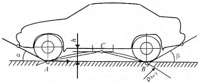
8.1-rasm. Yo'l to'siqlaridan o'ta olishning geometrik o'lchamlarini aniqlash.
