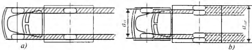
8.2-rasm. Oldingi va orqa g'ildiraklar izining mos kelish koefitsiyentini aniqlash.
