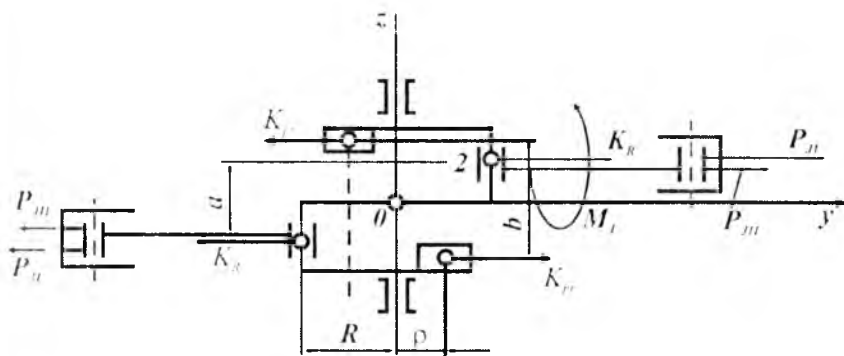
13.1-rasm. Ikki silindrlı dvigatellarnı muvozanatlash.
