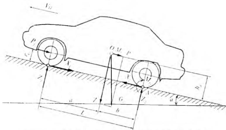
7.1-a rasm. Avtomobilning qiya tekislik bo'ylab harakati.
