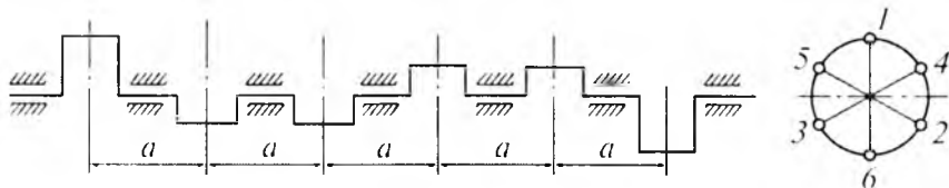
13.6-rasm. Olti silindrli dvigatelni muvozanatlash (krivoshiplari orasidagi burchak 60^\circ ).
