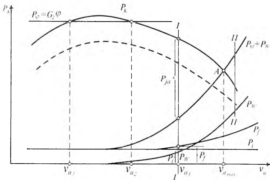
3.1-rasm. Avtomobilning kuchlar balansi grafiği.
