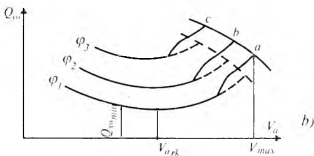
5.1-rasm. Avtomobilning yonilg'i tejamkorligini aniqlash.
