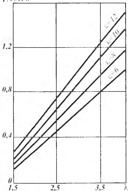
2.4-rasm. \epsilon ning har xil qiymatlari uchun p , bosimning \lambda ga bog'liqligi.
