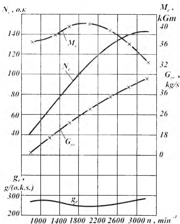
10.2-rasm. 3ИЛ-130 dvigatelining tashqi tezlik tavsifi.
