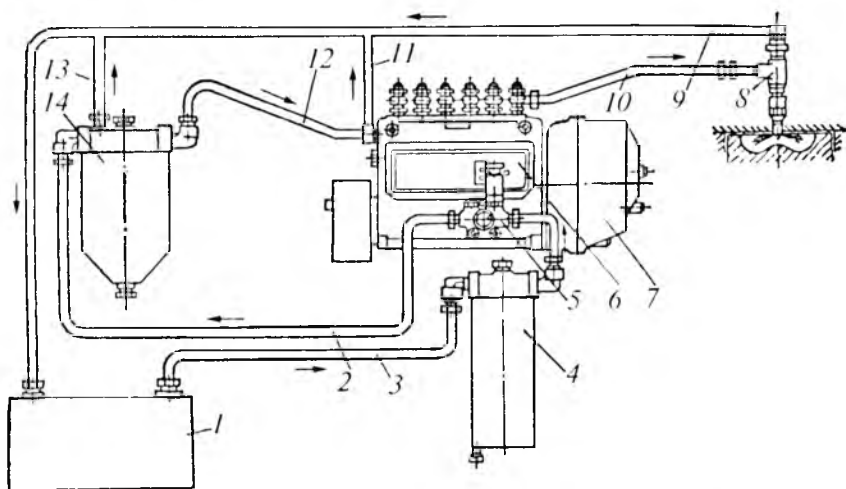
8.1-rasm. ЯМЗ-236 dizelni yonilg'i bilan ta'minlash tizimi.
