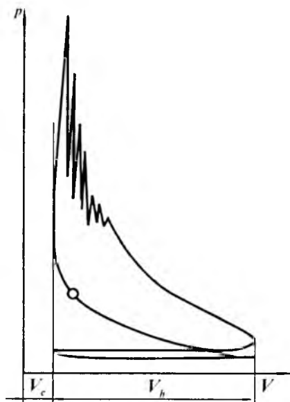
5.9-rasm. Detonatsiyali yonish diagrammasi.
