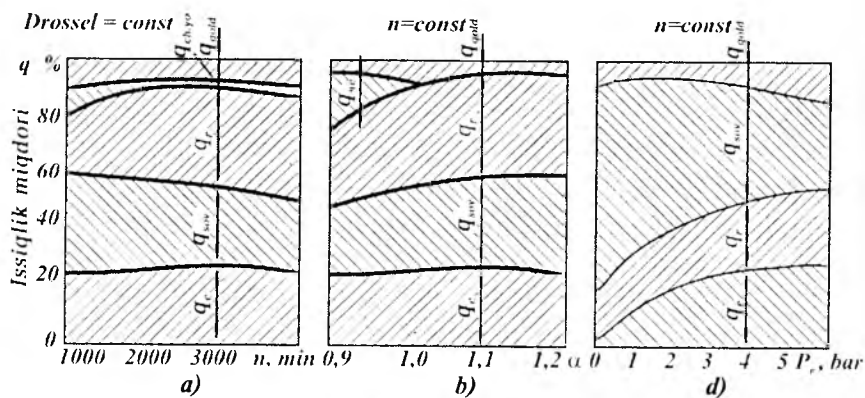
6.6-rasm. Dvigatelnig issiqlik balansi:
