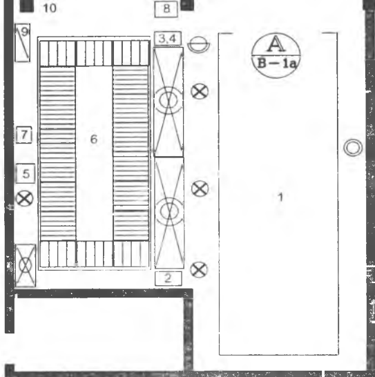
2.4.21- rasm. «Maxsutrans» avtokorxonasi bo‘yoqchilik ustaxonasining rejasi.
