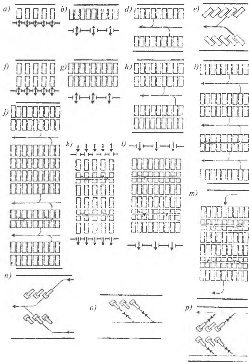
2.4.28- rasm. Saqlash mintaqalarida avtomobillarni o'rnashtirish usullari.
