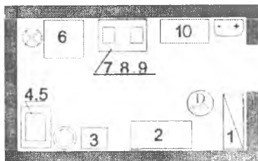
2.4.13- rasmi. «Maxsustrans» avtokorxonasi elektrtexnik ustaxonasi rejasi.
