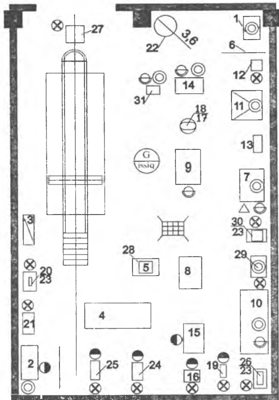
2.4.17- rasm. «MaxsuTrans» avtokorxonasi issiqlik ustaxonasining rejasi.
