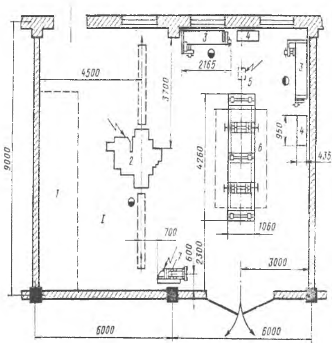
2.4.23- rasm. 500 ta yuk avtomobili uchun ATK duradgorlik ustaxonasining rejasi:
