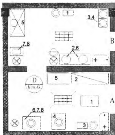
2.4.14- rasm. «Maxsustrans» avtokorxonasi akkumulator ustaxonasining rejası.
