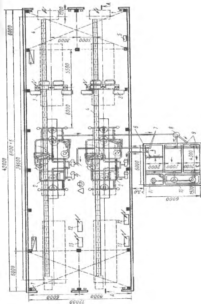
2.4.5- rasm. Avtobuslarga kundalik xizmat ko'rsatish mintaqasining rejası:
