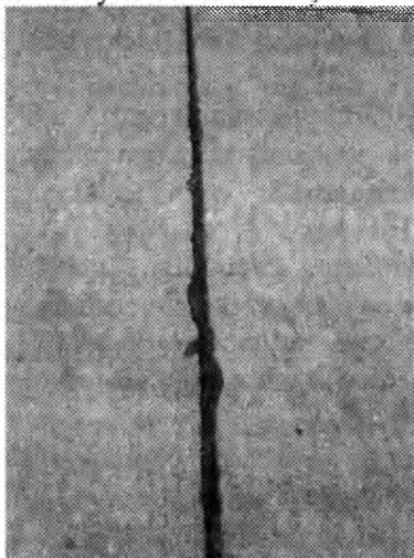
4.36-rasm. Issiq ob-havoda siqilish choklaridagi mastikaning qoplama yuzasiga chiqib qolishi
