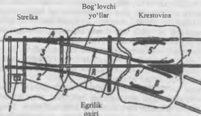
5.38-rasm. Oddiy strelkali o'tkazgich chizmasi: 1-o'tkazuvchi mexanizm; 2, 4-rama relslari; 3-ayri yo'naltirgich (отрпак); 5,8-kontrrelslar; 6-usovik; 7-krestovina; 9-o'tkazgich bruslari (shpallari).
