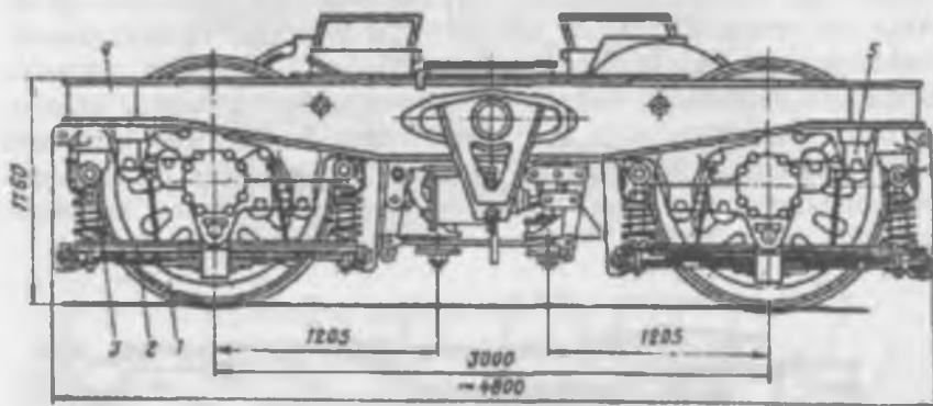
8.5-rasm. VL80 K aravacha shakli: 1 - o'ildirak jufti; 2 - reszorlar; 3 - vintsimon prujina; 4 - telejkaning yon ramasi; 5 - kronshteyn.
