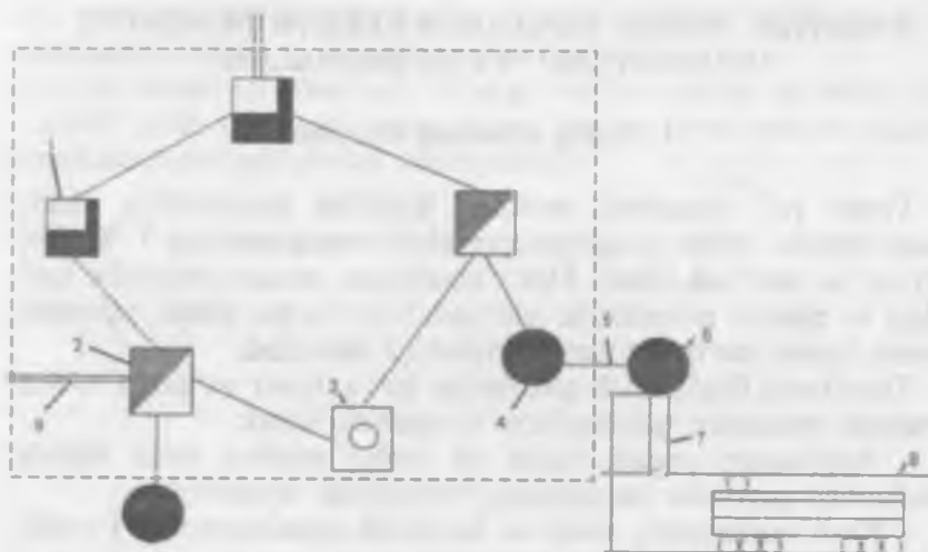
7.1-rasm. Elektrlashgan temir yo'llarda elektr ta'minotining prinsipial chizmasi: 1-issiqlik elektr stantsiyasi; 2- gidroelektrstansiya; 3- atom elektr stantsiyasi; 4-nohiiaviy transformator nimstantsiyasi; 5- yuqori kuchlanishli tuman liniyasi; 6-tortuvchi nimstansiya; 7- ta'minot liniyasi; 8-kontakt tarmog'i; 9-energiya tizimlarini bog'lovchi liniya.
