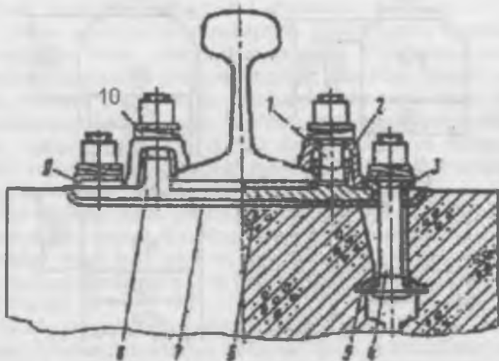
5.31-rasm. Temir - beton shpallar uchun KB rusumidagi ajratma mahkamlagich: 1 — klemmali prujinali bolt; 2 — klemma; 3 — ajratib turuvchi vtulka; 4 — belgilovchi (zakladnoy) bolt; 5 — anker shayba; 6 — taglik; 7 — rezina taglik; 8 — metall taglik; 9 — yassi shayba; 10 — ikki vintli prujinali shayba.
