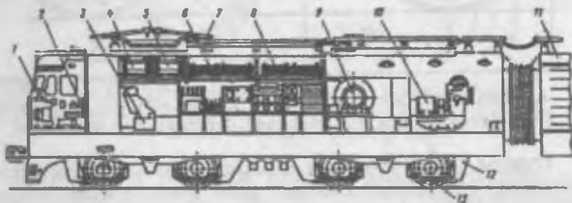
8.4-rasm. VL10 elektrovozida jihozlarning joylashtirilishi: 1 — boshqaruv pult; 2 — mashinist o'rindig'i; 3 — tezkor ishlovchi uzgich; 4, 5 — induktiv shunt va rezistorlarning balkalari; 6, 8 — ulash rezistorining bloki; 7 — tok qabul qilgich; 9 — motor-ventilator; 10 — motor-kompressor; 11 — elektrovoz ikkinchi bo'limining kuzovi; 12 — tortish elektr dvigateli; 13 — g'ildirak jufti.
