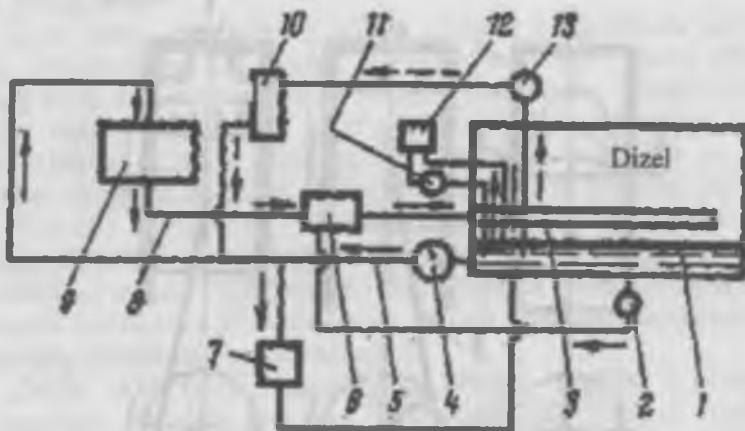
8.12-rasm Dizelni moylash tizimi: 1-dizel poddoni; 2- moy haydash nasosi; 3-moy tarqatgich kollektori; 4-markaziy sirkulyatsiya nasosi; 5-issiqlik moy quvuri; 6-moyni dag'al tozalash filtri; 7-moyni oliy tozalovchi filtri; 8-sovutilgan moy quvuri; 9-muzlatgich; 10-moy isitgich; 11-sentrifuga nasosi; 12-sentrifuga; 13-moyni isitgich orqali haydovchi nasos.
