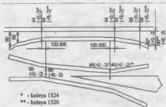
T3-rasm. Krestovinaga nisbatan kontrrelsning joylashish chizmasi va uning asosiy tarkibi oʻlchamlari.
