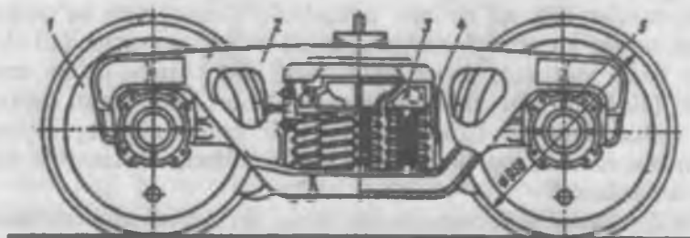
10.12-rasm. 1 - g'ildiraklar; 2 - aravachaning yon tomon quyma po'lat korobkasi; 3 - ressor komplekti; 4 - tebranishlarning ponali so'ndirgichlari; 5 - bukxa.
