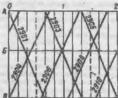
14.3-rasm. Ikki yo'li grafik.
