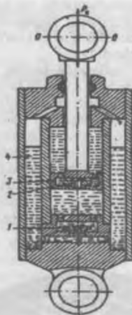
10.10-rasm. Gidravlik so'ndirgichning prinsipial chizmasi.
