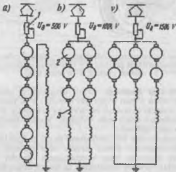
8.7-rasm. Olti o'qli elektrovozda tortish elektr dvigatellarining ulanishi: a-ketma-ket; b-ketma-ket-parallel; v-parallel; 1-ishga tushiruvchi rezistor; 2-tortish elektr dvigateli yakori; 3-qo'zg'atuvchi cho'lg'am.
