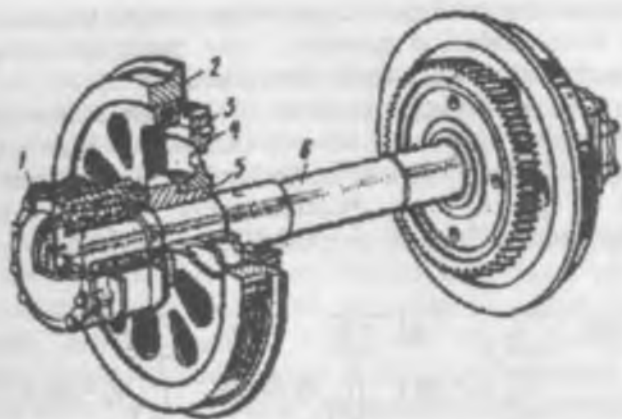
8.6-rasm Elektrovozning g'ildirak jufti: 1 — buksa; 2 — bandaj; 3 — shestemyali o'ildirak gardishi; 4 — shestemyali o'ildirak markazi; 5 — o'ildirak markazi; 6 — o'ildirak o'qi.
