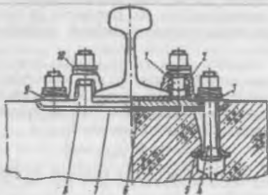
5.33-rasm. Temir-beton shpallarga relsni ajraladigan KB turidagi biniktirgichlar bilan qotirish: 1-klemmpli bosib turuvchi bolt; 2-klemma; 3-izolyatsiyalovchi vtulka; 4-bostirma bolt; 5-anker shayba; 6-qistirma; 7-rezina taglik; 8-metall taglik; 9-yassi shayba; 10-ikki o'ramli prujinali shayba.
