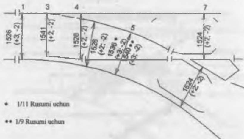
T2,b-rasm. 1524 mm li yoʻl uchun oʻlchov joylari: 1 – ramali rels ulanmasi; 2 – ramali rels burilish egrisining boshlanish joyi; 3 – strelka ayrilarining uchi; 4 – ayrilar oʻzagi; 5 – oʻtkazgich egrisining oʻrtasi; 6 – oʻtkazgich egrisining oxiri; 7 – krestovina.
