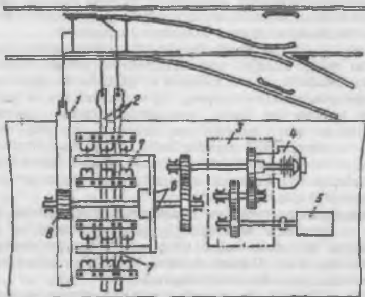
11.12-rasm. Elektrli markazlashtirilgan strelkali o'tkazgich: 1- ishchi tortish o'qi; 2 - tig'li yo'naltirgich holatini belgilovchi moslama; 3 - reduktor; 4 - friksion mufta; 5 - elektr dvigatel; 6 - avtoullovchi richag; 7 - avtoulagich; 8 - tishli uzatgich.
