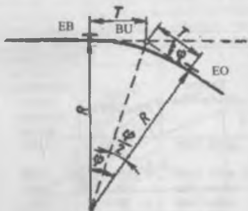
4.4-rasm. Aylanma egrilikning to'zilishti: EB - egrilik boshlanishi; EO - egrilik oxiri; BU - burilish cho'qqisi; R - egrilik radiusi; \varphi - burilish burchagi.
