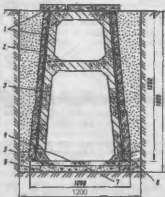
5.5-rasm. Rom rusumidagi temir-beton yopiq ariqcha: 1-temir-beton plitalar; 2-xandaqni qum qatlam bilan qoplanishi; 3-10×10 sm o'lehamli temir-beton ramalar; 4-sement qoplama; 5-bo'shliqlarni beton bilan to'ldirilishi; 6-qum-shchebenli asos-qatlam; 7-betonli asos-qatlam; 8-2,5 sm diametrlı drenaj tuynukchalari.
