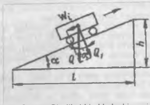
4.5-rasm. Qiyalikni hisoblash chizmasi.
