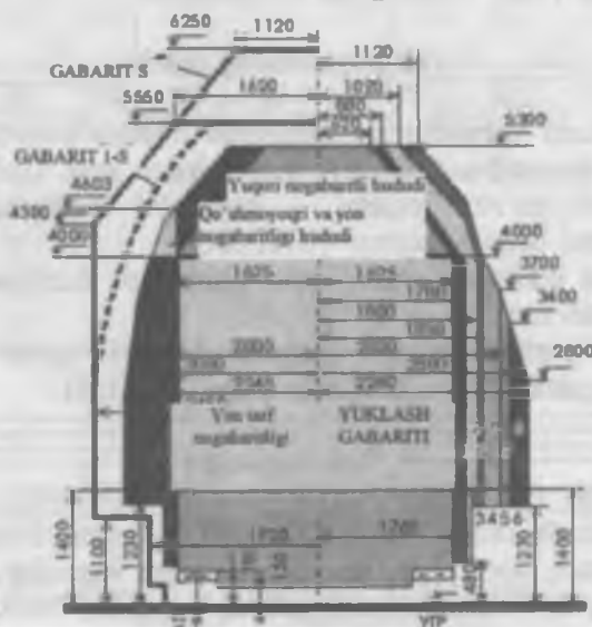
T12-rasm. Harakat tarkibi gavariti.
