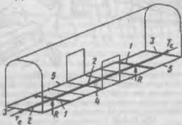
10.13-rasm. Vagon ramasi va kuzovining chizmasi.
