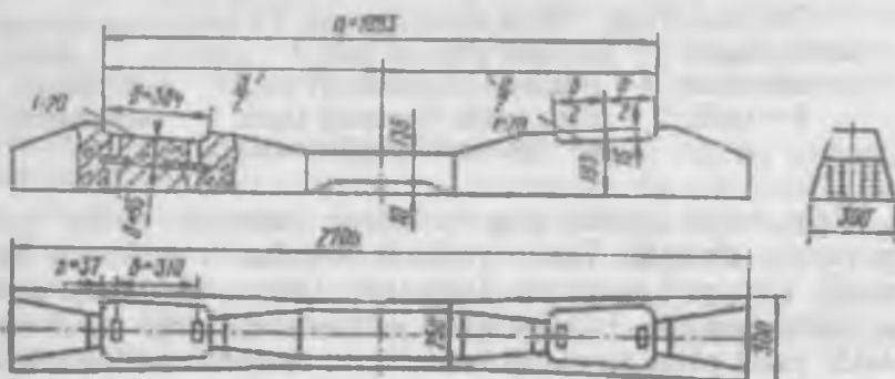
5.3-rasm. Temir - beton shpalla.
