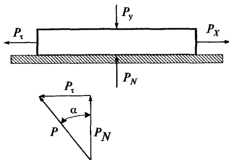
Рис. 2.8. Схема действия сил при трении скольжения
