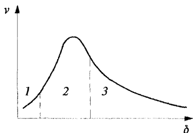
Рис. 2.21. Зависимость скорости атмосферной коррозии \delta от толщины пленки влаги \delta на поверхности металла:
