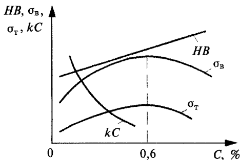
Рис. 4.7. Зависимость механических свойств сталей от содержания углерода
