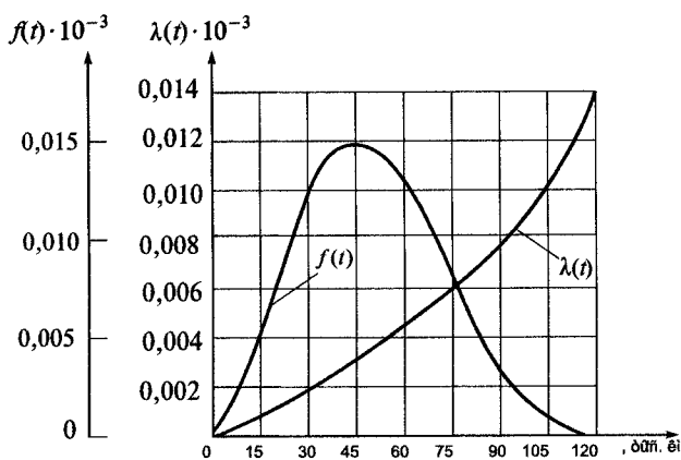
Рис. 6.15. Графики плотности распределения f(t) и интенсивности отказов \lambda(t) ведомых дисков сцепления
