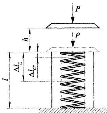
Рис. 2.5. Схема ударного эксплуатационного нагружения
