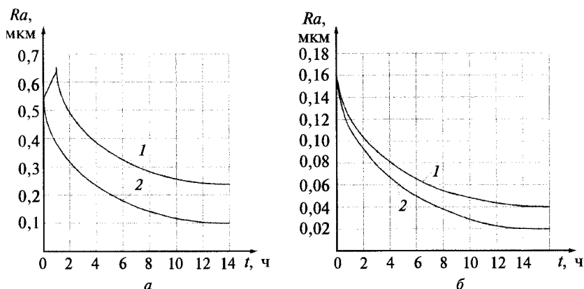
Рис. 4.10. Изменение шероховатости деталей цилиндропоршневой группы в процессе обкатки двигателя:
