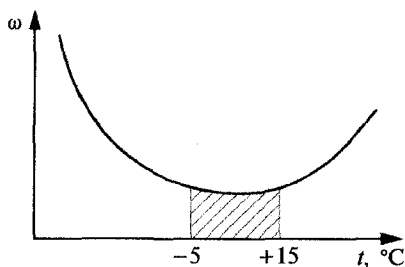
Рис. 4.12. Зависимость количества отказов автомобиля от температуры окружающего воздуха t, ^\circ\text{C}
