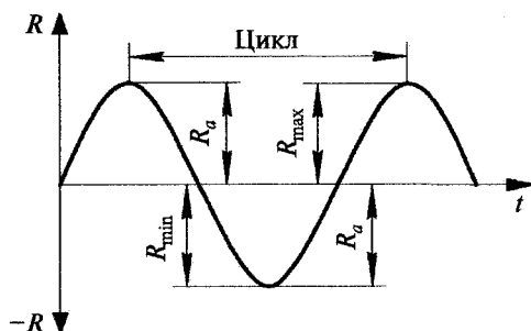
Рис. 2.16. Схема симметричного циклического нагружения
