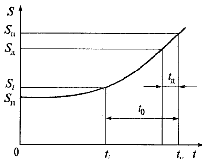
Рис. 8.19. Схема определения периодичности диагностирования по частной реализации диагностического параметра
