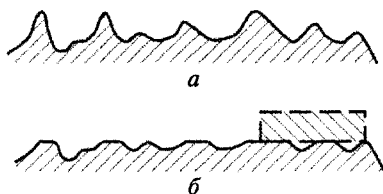
Рис. 2.11. Схема преобразования технологического рельефа поверхности (а) в эксплуатационный (б)
