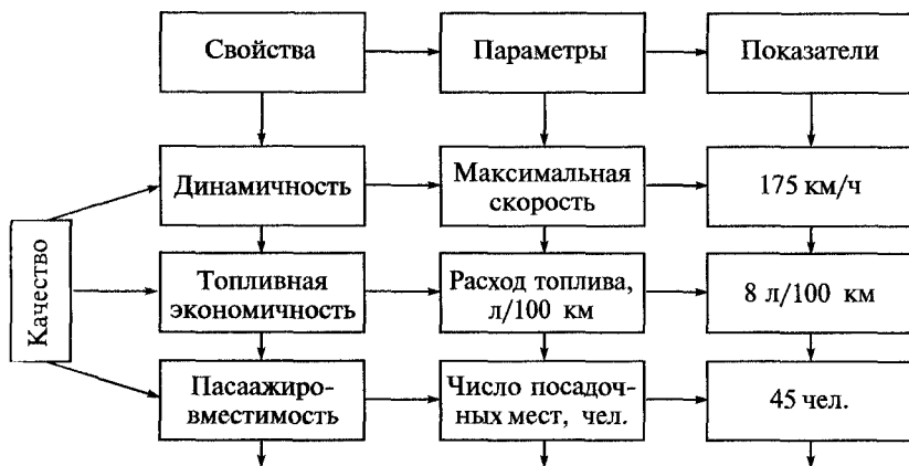
Рис. 1.2. Структура понятия качества автомобиля
