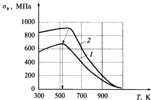
Рис. 2.19. Зависимость напряжений прочности \sigma_b от температуры: 1 — углеродистая сталь 45; 2 — легированная сталь 40Х
