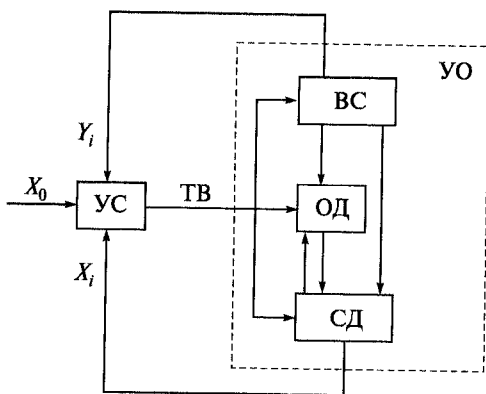
Рис. 8.21. Схема управления техническим состоянием объекта в эксплуатации: УС — управляющая система; ВС — внешняя среда; УО — управляемый объект; ОД — объект диагностирования; СД — средства диагностирования; ТВ — технические воздействия
