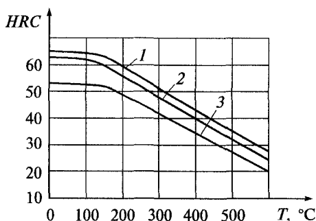
Рис. 7.11. Зависимость твердости материала стальных деталей с различным содержанием углерода C от температуры отпуска: 1 — C = 0,8\% ; 2 — C = 0,6\% ; 3 — C = 0,35\%
