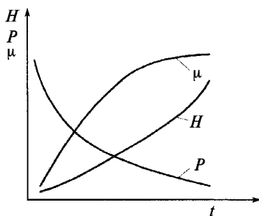
Рис. 3.4. Зависимость наработки до возникновения усталостного выкрашивания от твердости металла H , эксплуатационного нагружения P и вязкости смазочного материала \mu
