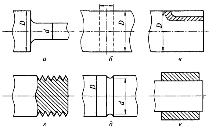
Рис. 2.17. Примеры концентраторов внутренних напряжений:
