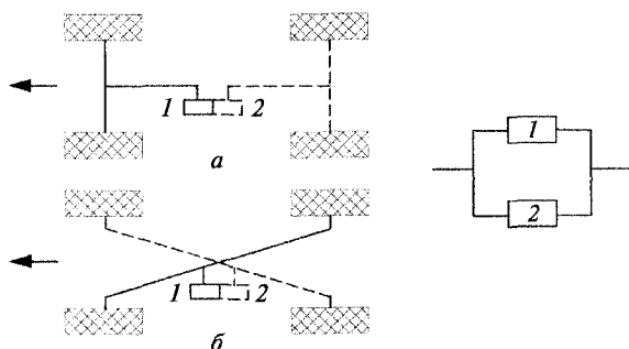
Рис. 7.6. Схемы тормозных систем с осевым ( а ) и диагональным ( б ) разделением контуров:
