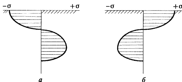
Рис. 2.13. Типичные эпюры остаточных напряжений I рода в поверхностном слое детали после механической обработки
