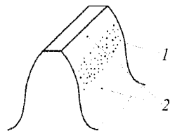
Рис. 3.12. Изнашивание зуба шестерни: 1 — зона наибольшего изнашивания; 2 — зона усталостного изнашивания
