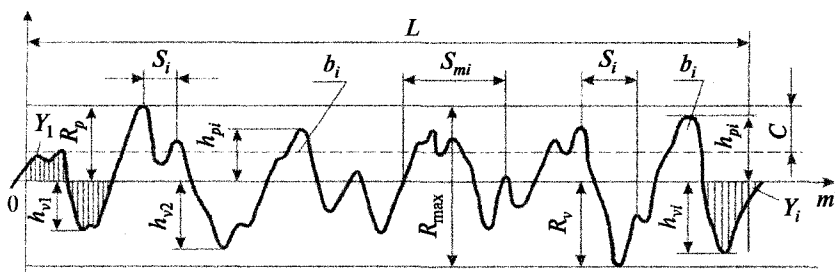
Рис. 4.9. Профилограмма поверхности для определения шероховатости
