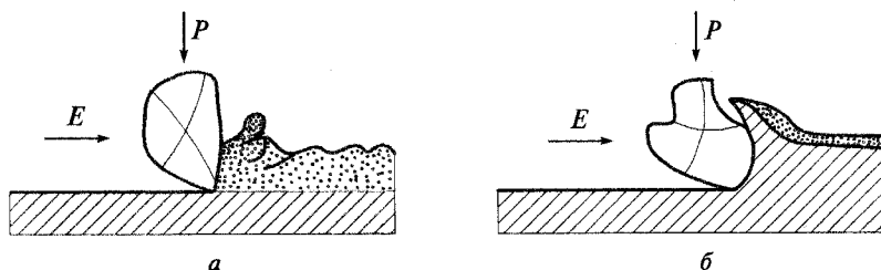
Рис. 3.2. Формы абразивного изнашивания: а — механохимическая; б — механическая
