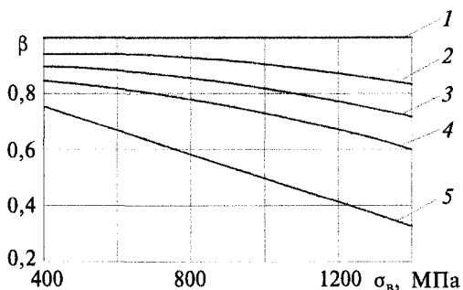
Рис. 2.18. Зависимость коэффициента качества поверхности \beta от предела прочности стали \sigma_b и вида обработки поверхности:
