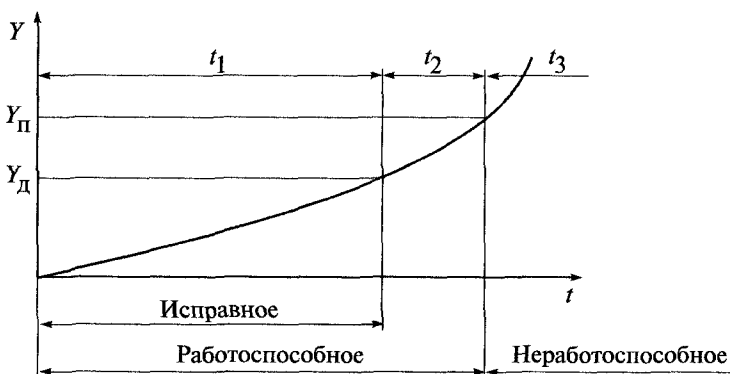
Рис. 8.4. Схема развития постепенного отказа:
