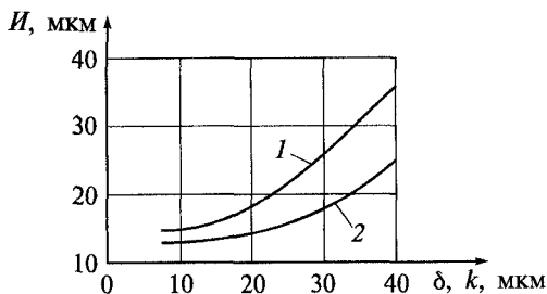
Рис. 7.10. Зависимости износа H от овальности \delta (1) и конусности k (2) гильз цилиндров
