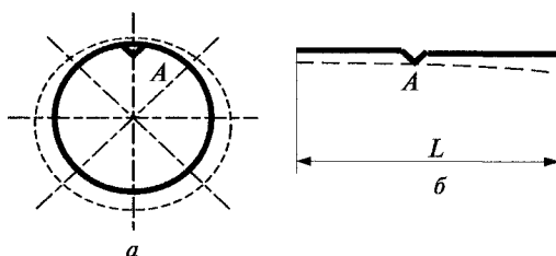
Рис. 3.14. Совмещение профилограмм:
