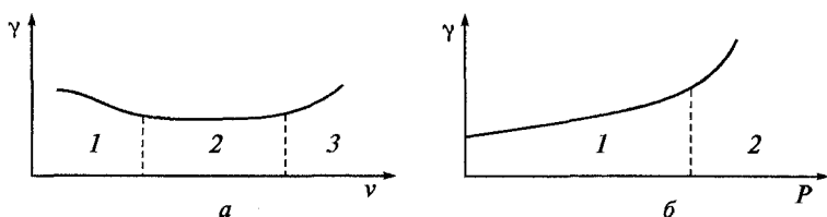
Рис. 4.1. Зависимости скорости изнашивания \gamma от скорости относительного скольжения v и давления P на поверхности трения
