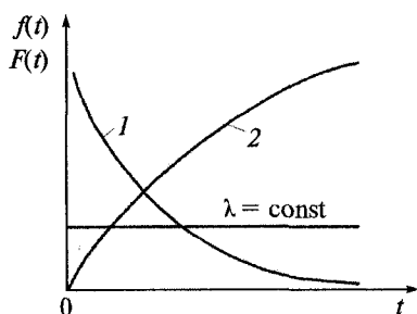
Рис. 6.2. Дифференциальная (1) и интегральная (2) функции экспоненциального распределения
