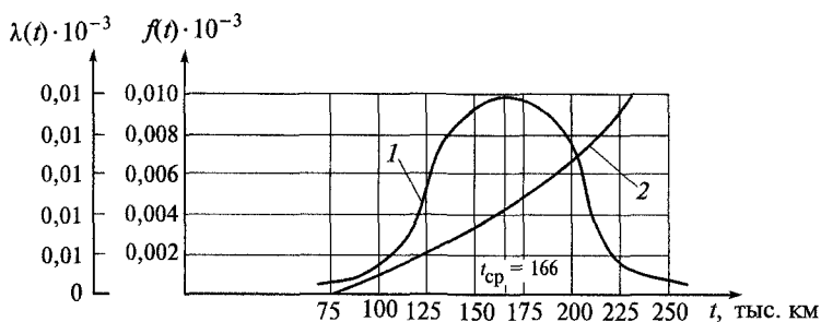
Рис. 6.12. Графики плотности распределения (1) и интенсивности отказов (2) вкладышей шеек коленчатого вала
