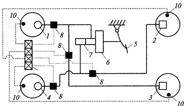
Рис. 5.2. Принципиальная схема тормозной системы автомобиля ВАЗ-21703-01-018:
