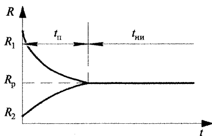
Рис. 3.8. Изменение шероховатости поверхностей за период приработки
