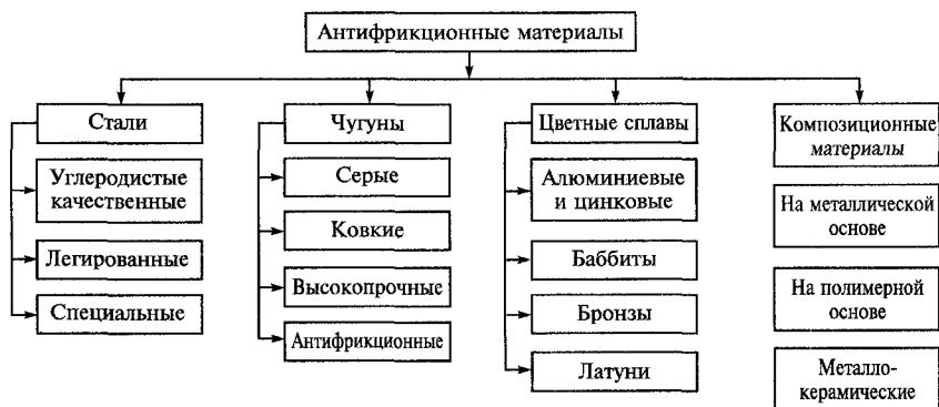
Рис. 7.2. Антифрикционные материалы, используемые в узлах трения
