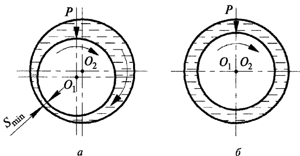
Рис. 4.4. Схема формирования масляного клина в подшипнике скольжения коленчатого вала:
