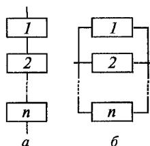
Рис. 5.1. Схемы соединения конструктивных элементов:
