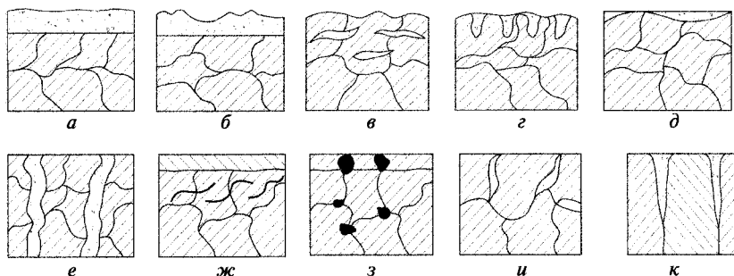
Рис. 2.22. Виды коррозии:
