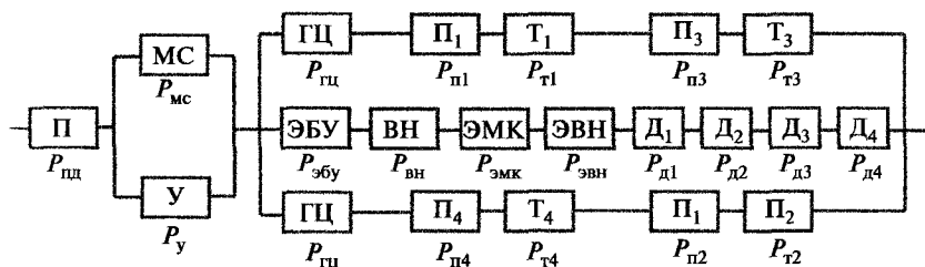
Рис. 5.3. Структурная схема двухконтурной тормозной системы автомобиля ВАЗ-21703-01-018:
