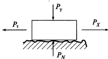
Рис. 2.2. Схема взаимодействия поверхностей при их относительном перемещении: P_t — сила трения; P_y — нормальная сила (сила прижатия); P_x — осевая сила перемещения; P_N — нормальная сила реакции силового нагружения
