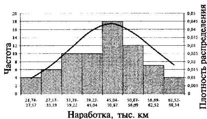
Рис. 5.10. Гистограмма распределения отказов подшипника верхней опоры телескопической стойки ПП
