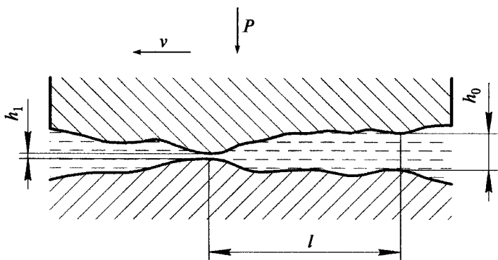
Рис. 4.5. Схема элементарного гидродинамического клина, возникающего в зоне трения:
