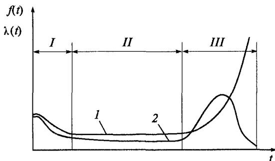
Рис. 1.5. Типичные зависимости интенсивности \lambda(t) — 1 и плотности вероятностей f(t) — 2 по наработке t
