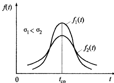
Рис. 6.3. Графическая интерпретация нормального распределения
