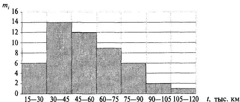
Рис. 6.13. Гистограмма распределения отказов ведомых дисков сцепления автомобилей
