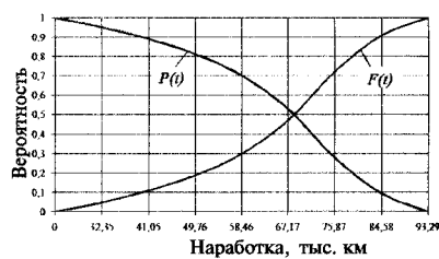
Рис. 5.13. Интегральные функции отказа F(t) и безотказной работы P(t) телескопической стойки
