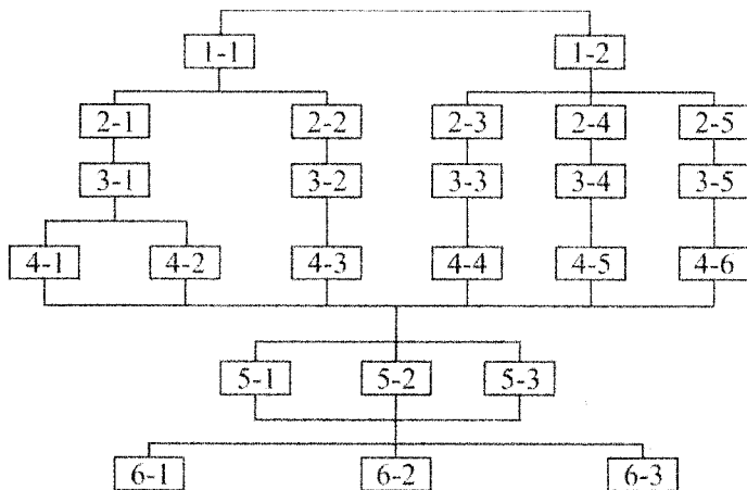
Рис. 8.15. Блок-схема структурно-следственных связей рулевого управления переднеприводного автомобиля семейства ВАЗ:
