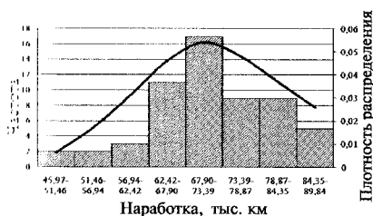
Рис. 5.14. Гистограмма распределения наработок на отказ подшипника ступицы ПП
