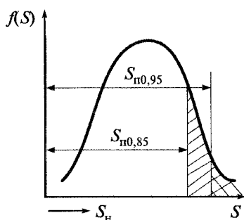
Рис. 8.16. Схема определения предельных нормативов диагностических параметров
