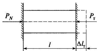
Рис. 2.3. Схема возникновения температурного напряжения детали
