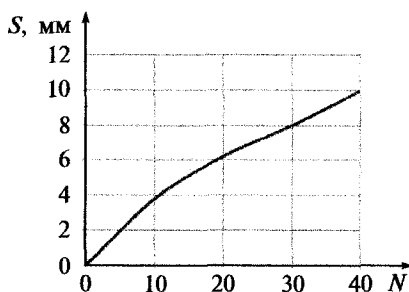
Рис. 5.17. Распространение подпленочной коррозии на передних дверях легкового автомобиля:
