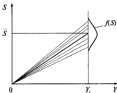
Рис. 8.12. Распределение результатов измерения диагностического параметра S_i
