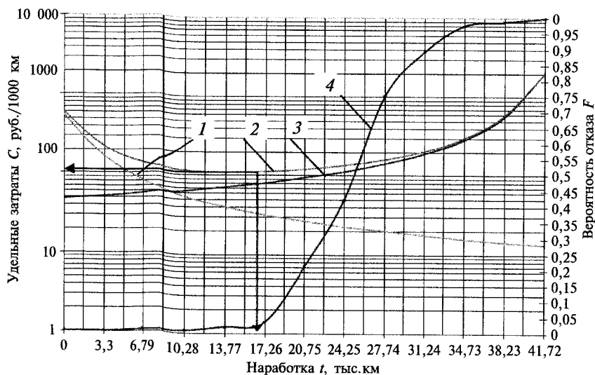
Рис. 8.20. Определение периодичности технических воздействий экономико-вероятностным методом:
