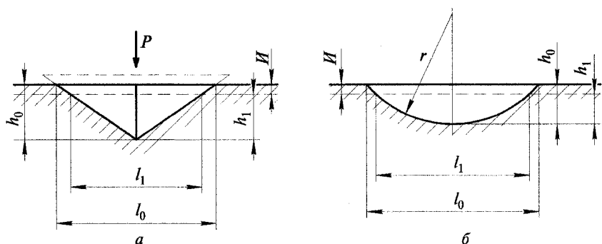
Рис. 3.15. Схема измерения износа методом искусственных баз:
