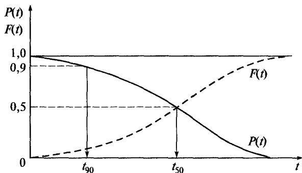
Рис. 1.4. Изменение вероятности безотказной работы P(t) и отказа F(t) по наработке t
