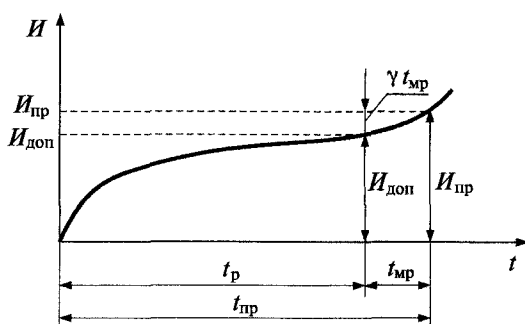
Рис. 3.10. Схема определения допустимого износа
