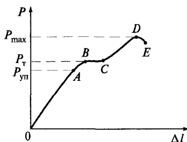
Рис. 2.12. Диаграмма зависимости «деформация—нагрузка»
