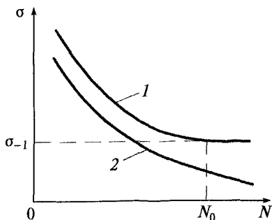
Рис. 2.14. Кривая выносливости: 1 — сталей; 2 — цветных металлов
