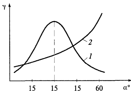
Рис. 3.3. Зависимость интенсивности гидро- и газобразивного изнашивания \gamma от угла атаки \alpha абразивных частиц:
