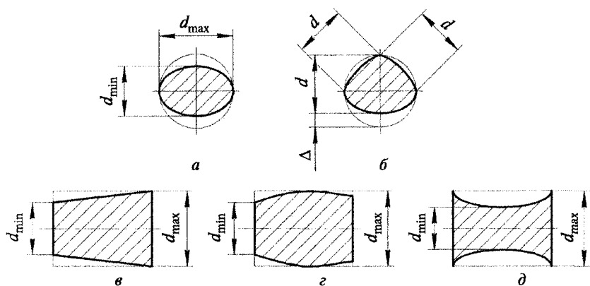
Рис. 4.8. Отклонение формы цилиндрических поверхностей:
