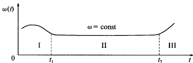
Рис. 1.6. Изменение параметра потока отказов \omega по наработке t
