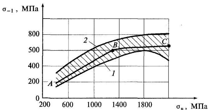
Рис. 2.15. Зависимости между пределами выносливости \sigma_{-1} и прочности \sigma_B стальных образцов
