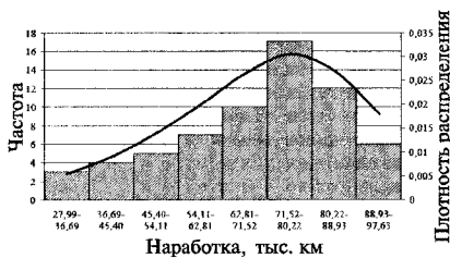
Рис. 5.12. Гистограмма распределения наработок на отказ телескопической стойки ПП
