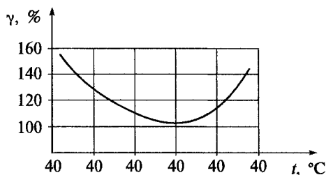
Рис. 4.2. Изменение интенсивности изнашивания цилиндров двигателя (расстояние 8 мм от верхней плоскости блока) в зависимости от температуры масла в камере t
