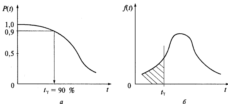
Рис. 1.7. Схема определения \gamma -процентного ресурса
