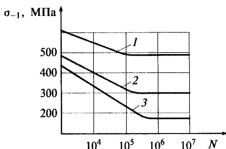
Рис. 2.20. Кривая выносливости образцов из стали 20Х13 с коррозионными повреждениями:
