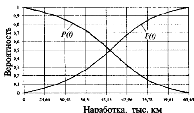
Рис. 5.11. Интегральные функции отказа F(t) и безотказной работы P(t) подшипника верхней опоры
