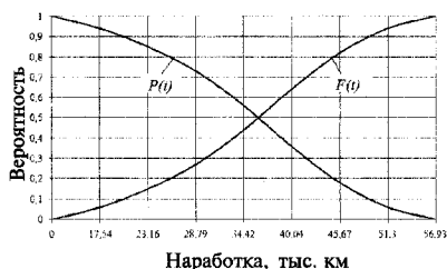
Рис. 5.9. Интегральные функции отказа F(t) и безотказной работы P(t) шарового шарнира
