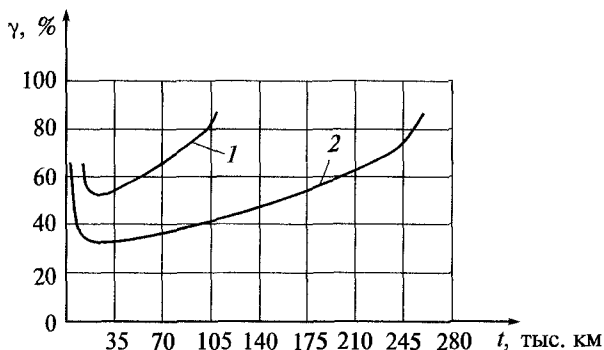
Рис. 8.1. Кривые изнашивания хромированного поршневого кольца: 1 — на минеральном масле; 2 — на синтетическом масле; \gamma — относительный износ
