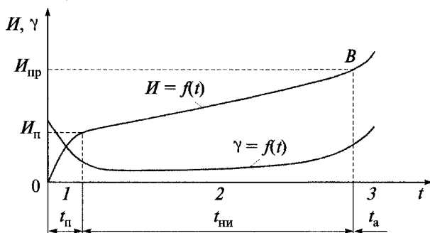
Рис. 3.7. Кривая изнашивания деталей машин:
