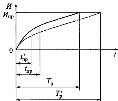
Рис. 7.4. Схема изменения процесса изнашивания в результате изменения геометрической формы
