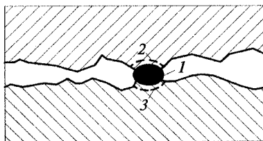
Рис. 3.5. Схема образования схватывания контактирующих поверхностей: 1 — локальный участок схватывания; 2, 3 — линии границ разрушения металлических связей
