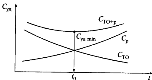
Рис. 8.7. Зависимость затрат на ТО и ремонт от периодичности ТО
