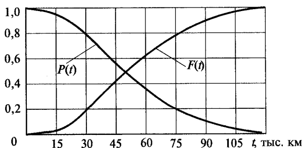
Рис. 6.14. Графики вероятностей отказа F(t) и безотказной работы P(t) ведомых дисков сцепления
