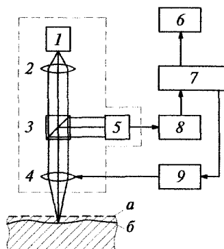
Рис. 3.13. Схема прибора для бесконтактного измерения профиля рабочей поверхности детали:
