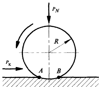
Рис. 2.9. Схема контакта рабочих поверхностей при трении качения
