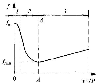
Рис. 4.6. Зависимость коэффициента трения от режима работы сопряжения
