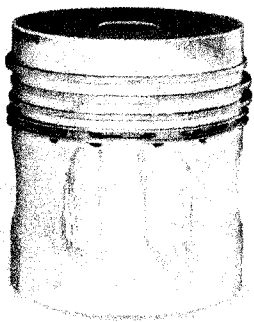
Рис. 8.2. Задирь на юбке поршня из алюминиевого сплава при работе с недостаточным количеством масла
