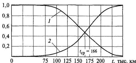
Рис. 6.11. График функции вероятности безотказной работы (1) и вероятности отказов (2)
