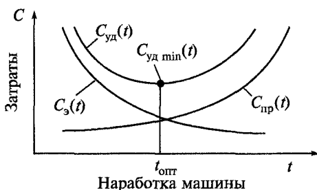
Рис. 1.1. Схема обоснования оптимального уровня надежности машины
