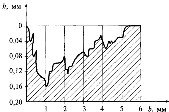
Рис. 2.23. Очаг коррозионного разрушения на крыле автомобиля: h и b — глубина и ширина каверны
