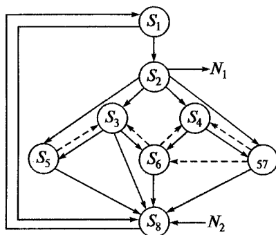
Рис. 1.8. Обобщенный граф возможных состояний автомобилей
