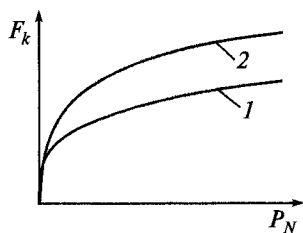
Рис. 2.10. Зависимость фактической площади контакта F_k от нагрузки P_N для деталей с различной поверхностной твердостью:
