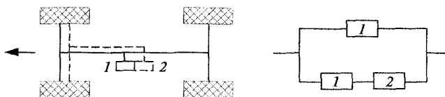
Рис. 7.7. Схема тормозной системы с резервированием переднего контура: 1 — контур, объединяющий первую секцию главного тормозного цилиндра и тормозные механизмы всех колес; 2 — контур, объединяющий вторую секцию главного тормозного цилиндра и тормозные механизмы передних колес
