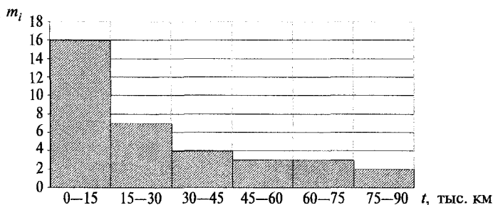
Рис. 6.8. Гистограмма распределения наработок элементов системы освещения до отказа
