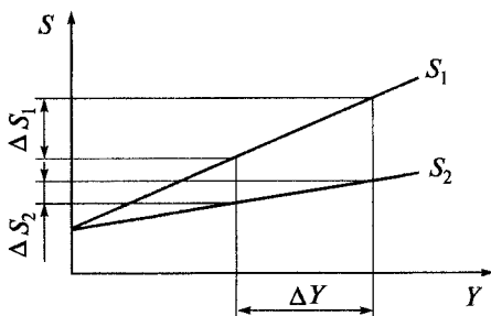
Рис. 8.13. Схема определения чувствительности диагностических параметров
