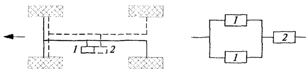
Рис. 7.8. Схема тормозной системы с резервированием переднего контура и одного из цилиндров задних колес:
