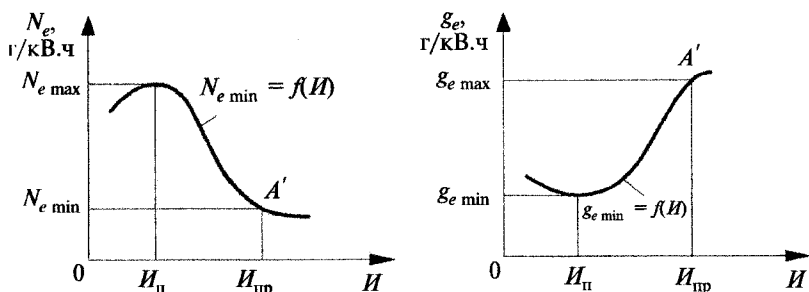
Рис. 3.9. Графики изменения эффективной мощности N_e и удельного расхода топлива g_e от степени износа двигателя
