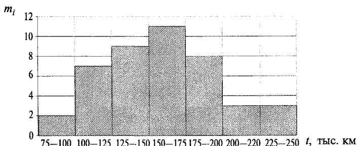
Рис. 6.10. Гистограмма распределения отказов вкладышей коренных шеек коленчатого вала по наработке
