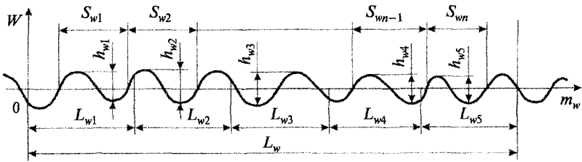
Рис. 4.11. Профилограмма поверхности для определения волнистости
