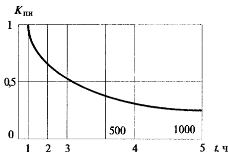
Рис. 3.16. Изменение концентрации продуктов изнашивания двигателя в масле: 1 — новый двигатель; 2 — после наработки 100 ч; 3 — после наработки 300 ч; 4 — после наработки 600 ч; 5 — после наработки 1000 ч
