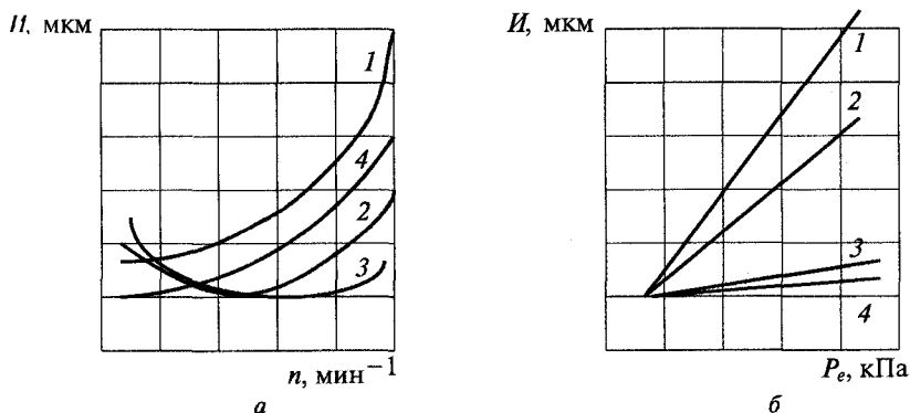
Рис. 4.13. Влияние частоты вращения коленчатого вала n и среднего эффективного давления P_e на износ деталей двигателей 3МЗ:
