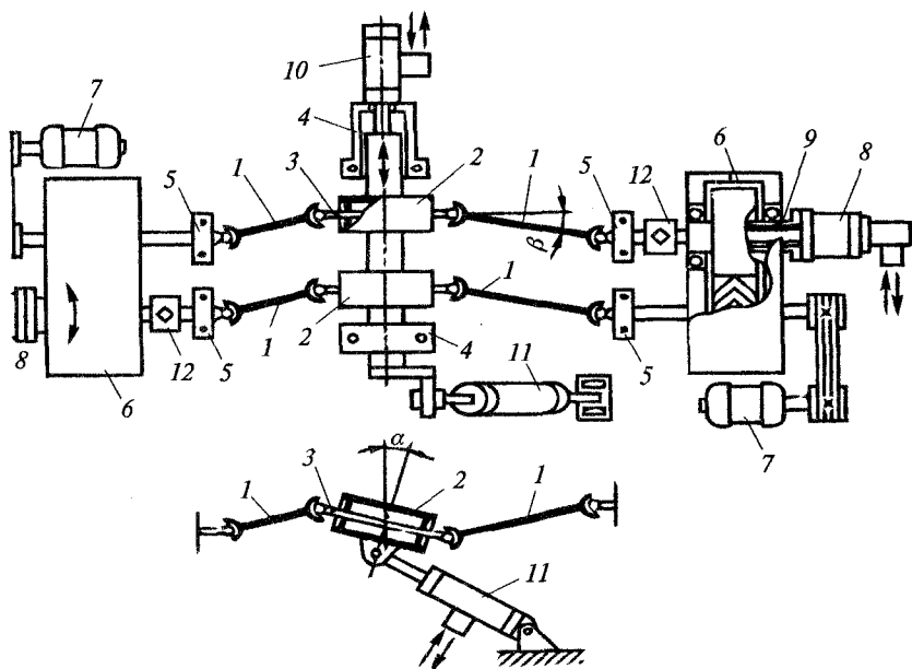
Рис. 5.16. Схема стенда для испытаний карданных валов с программным регулированием вращательных нагрузок, вертикальных и горизонтальных углов передачи момента:
