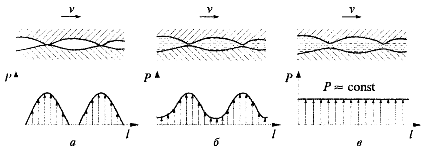
Рис. 4.3. Схематичное изображение основных видов трения:
