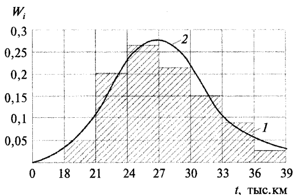
Рис. 6.6. Гистограмма 1 и теоретическая кривая распределения 2 значений наработки свечей зажигания до отказа
