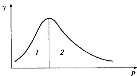
Рис. 3.6. Зависимость интенсивности изнашивания при фреттинг-коррозии от давления на поверхности трения
