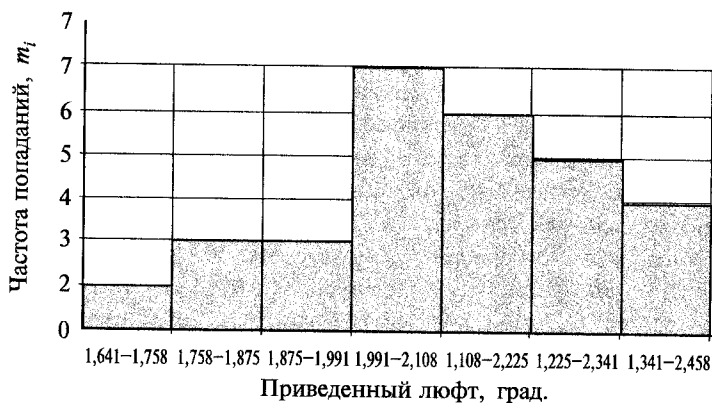
Рис. 8.17. Гистограмма распределения значений люфта \alpha_{pm} , град.
