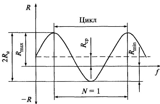
Рис. 2.6. Схема циклического нагружения:
