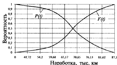
Рис. 5.15. Интегральные функции вероятности отказа F(t) и безотказной работы P(t) подшипника ступицы ПП
