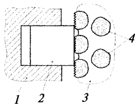
Рис. 7.3. Схема взаимодействия поршневого кольца с рабочей поверхностью цилиндра: 1 — поршень; 2 — поршневое кольцо; 3 — цилиндр блока из алюминиевого сплава; 4 — кристаллы кремния
