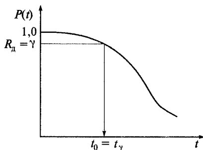
Рис. 8.5. Определение периодичности ТО по допустимому уровню безотказности
