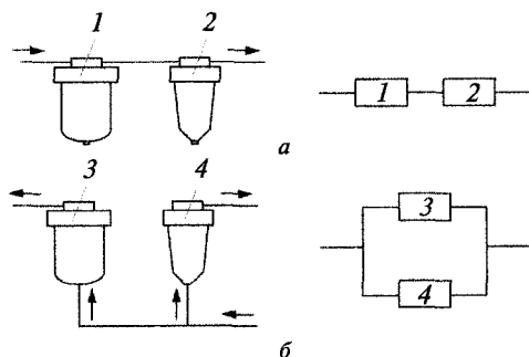
Рис. 7.5. Схемы соединения фильтров:
