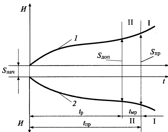
Рис. 3.11. Схема определения допустимого зазора в сопряжении:
