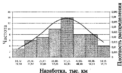
Рис. 5.8. Гистограмма распределения наработок шарового шарнира рычага ПП
