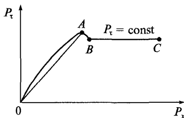
Рис. 2.7. Схема изменения силы трения P_\tau при переходе от состояния покоя к движению:
