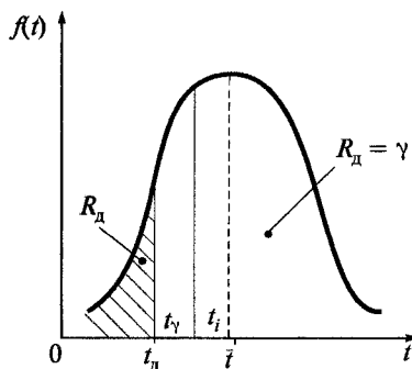
Рис. 8.18. Схема определения оптимальной периодичности диагностирования по допустимой вероятности безотказной работы
