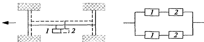
Рис. 7.9. Схема тормозной системы с общим резервированием:
