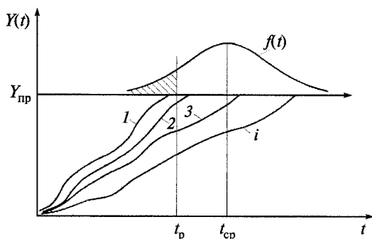
Рис. 8.3. Схема формирования отказа изделия
