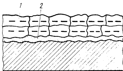
Рис. 9.4. Схема соединения частиц присадочного металла между собой и подслоем:
