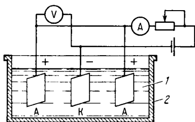
Рис. 10.8. Схема установки для нанесения гальванических покрытий: 1 — электролит; 2 — ванна; А — анод; К — катод
