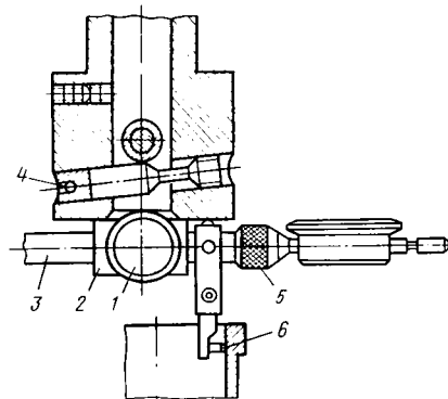
Рис. 4.3. Резцовая головка станка 2А78Н с приспособлениями для центрирования гильз: 1—винт; 2—колодка; 3—рычаг; 4—шариковая оправка; 5—гайка; 6—упор рычага
