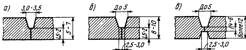
Рис. 7.16. Разделка сквозных трещин
