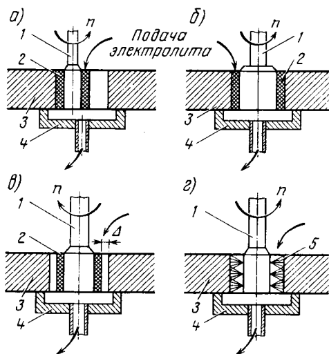
Рис. 10.14. Схема осаждения металла контактным способом: 1 — анодная головка; 2 — тампон; 3 — деталь; 4 — сборник электролита; 5 — щетка; n — частота вращения; \Delta — зазор между тампоном и деталью
