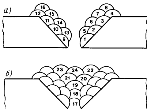
Рис. 7.17. Схема сварки трещин способом отжигающих валиков: а — обварка кромок разделки; б — наложение соединительных валиков; 1 — 24 — последовательность наложения валиков
