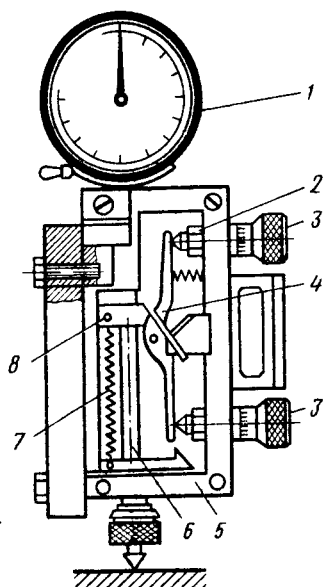
Рис. 2.1. Электроконтактный предельный преобразователь модели 228:
