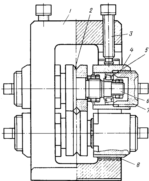
Рис. 5.10. Роликовая волока
