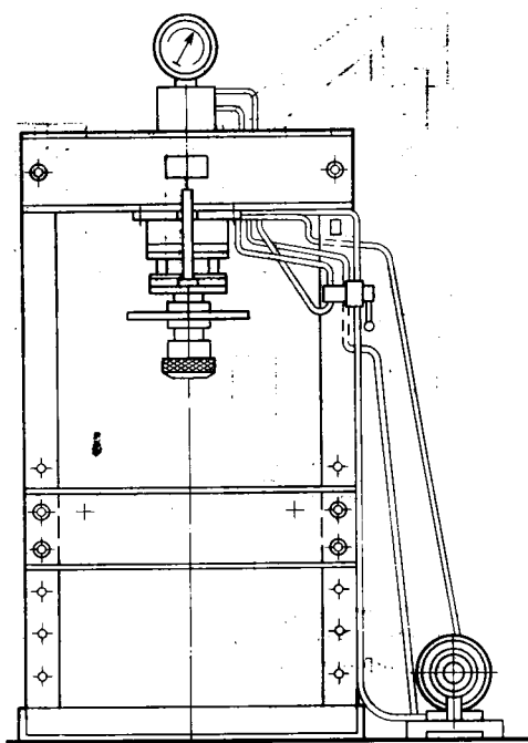
Рис. 6.23. Универсальный гидравлический пресс модели 2135-1
