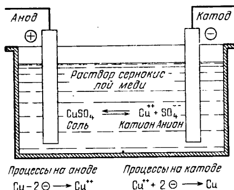
Рис. 10.2. Схема гальванического процесса
