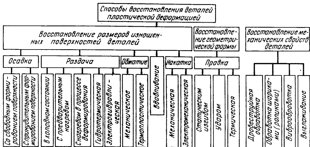
Рис. 6.2. Классификация способов восстановления деталей пластической деформацией
