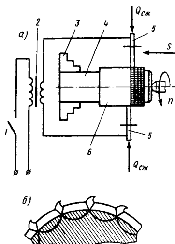
Рис. 8.1. Схема электроконтактной приварки ленты на деталь типа вал (а) и перекрывания сварочных точек (б): 1 — прерыватель тока; 2 — трансформатор; 3 — патрон для крепления детали; 4 — восстанавливаемая деталь; 5 — роликовые электроды; 6 — привариваемая лента
