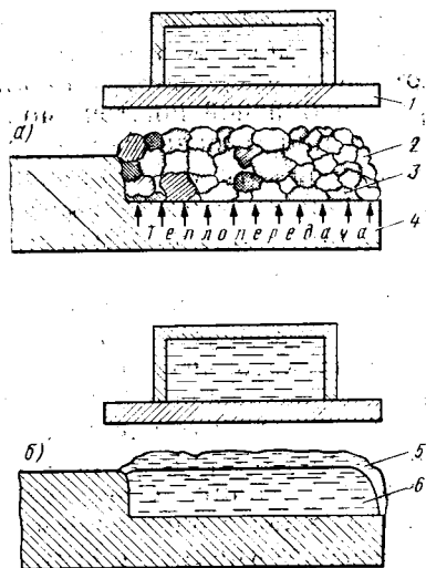
Рис. 8.9. Схема способа индукционной наплавки порошкообразной шихтой:
