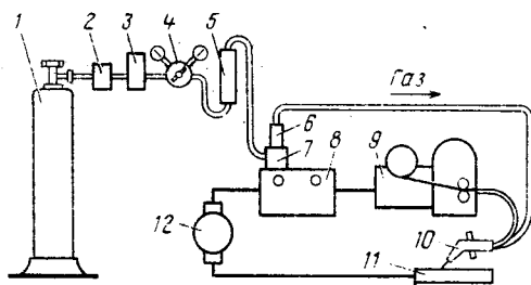
Рис. 7.10. Схема установки для сварки (наплавки) в среде \text{CO}_2 :
