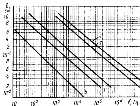
Рис. 2.15. Номограмма для определения глубины \delta проникновения вихревых токов (по данным А. Л. Дорофеева): 1 — титановый сплав ВТ3; 2 — нержавеющая сталь 1Х18Н9Т; 3 — АК6; 4 — медь; 5 — высоколегированная сталь
