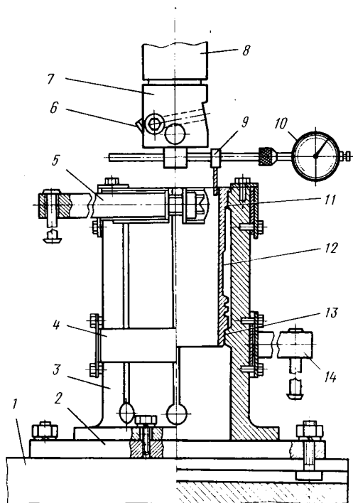
Рис. 5.16. Приспособление для центровки и закрепления гильзы цилиндров на столе расточного станка:
