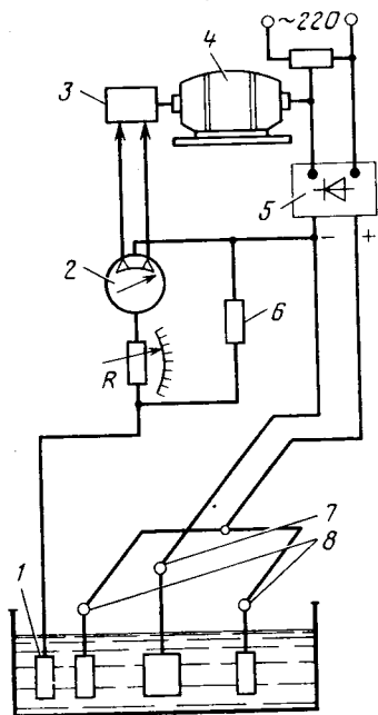
Рис. 10.19. Схема установки автоматического регулирования плотности тока: 1 — датчик; 2 — гальванометр; 3 — блок управления; 4 — двигатель; 5 — селеновый выпрямитель; 6 — шунт; 7 — катод; 8 — анод
