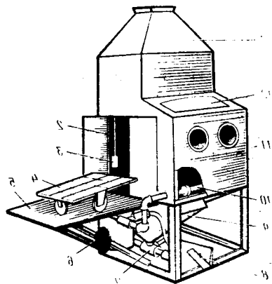
Рис. 1.8. Установка для очистки деталей косточковой крошкой
