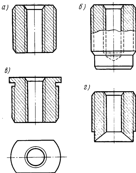
Рис. 5.7. Основные типы свертышей:
