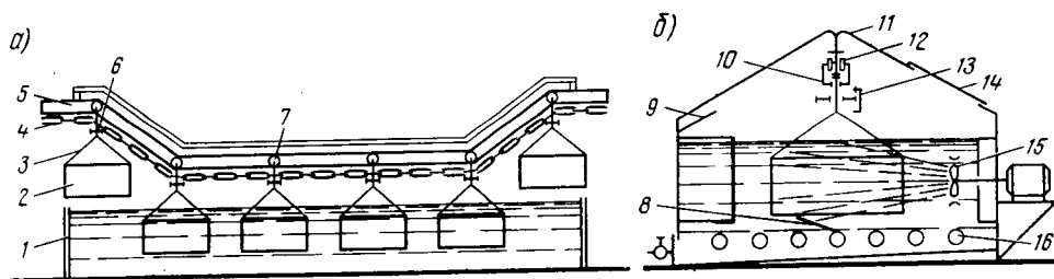
Рис. 1.7. Конвейерная моечная машина КМ-4:
