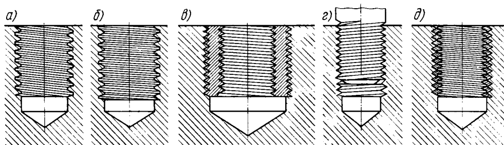
Рис. 5.6. Способы ремонта резьбовых соединений:
