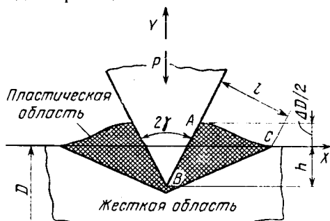
Рис. 6.15. Схема для определения усилия высадки металла при электромеханическом способе накатывания поверхностей:
