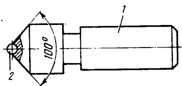
Рис. 6.22. Алмазная гладилка: 1 — оправка; 2 — алмаз
