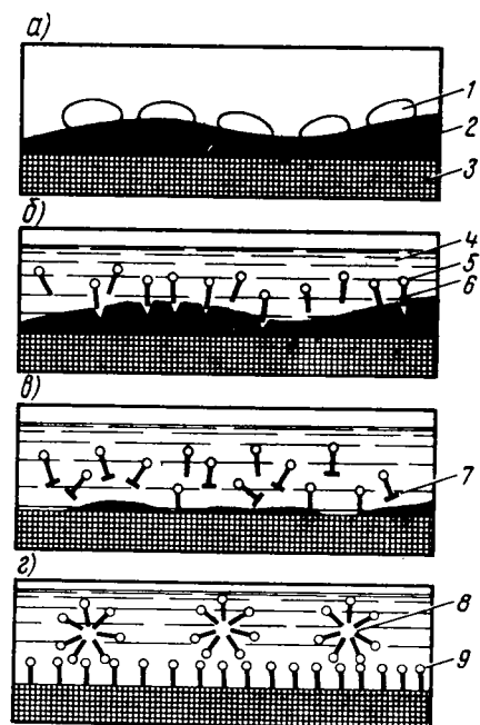
Рис. 1.3. Схема моющего процесса:
