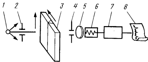
Рис. 2.12. Схема радиометрического метода контроля:
