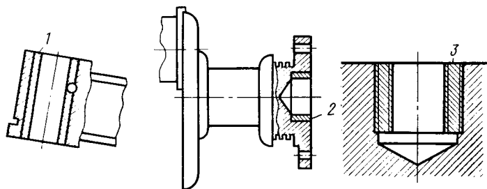
Рис. 5.1. Дополнительные ремонтные детали (ДРД): 1 и 2 — втулки; 3 — ввертыш
