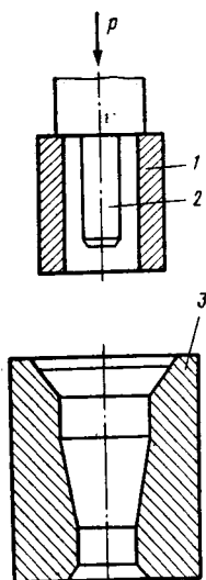
Рис. 6.7. Восстановление втулок обжатием: 1 — втулка; 2 — пуансон; 3 — матрица
