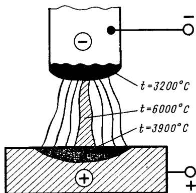
Рис. 7.1. Распределение температуры t в сварочной дуге
