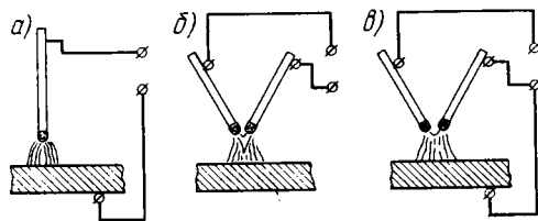
Рис. 7.2. Виды сварочных дуг: а — прямого действия; б — косвенного действия; в — комбинированного действия (трехфазная)
