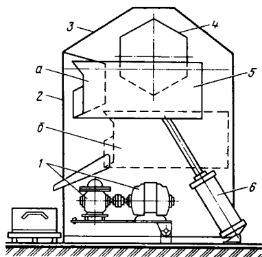
Рис. 1.9. Установка для мойки мелких деталей во вращающемся барабане: а и б — соответственно крайнее верхнее и крайнее нижнее положения ванны
