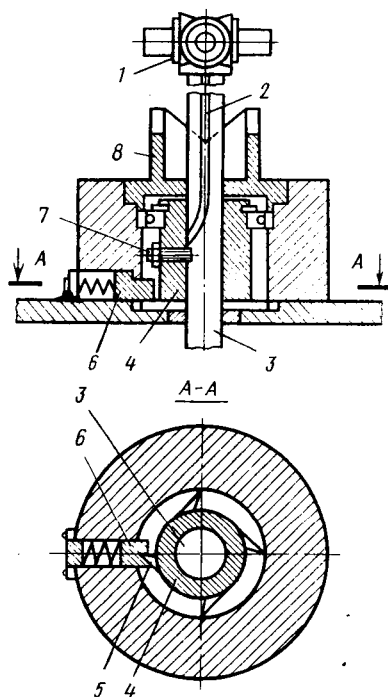
Рис. 6.26. Механизм фиксации и поворота крестовин на 90^\circ
