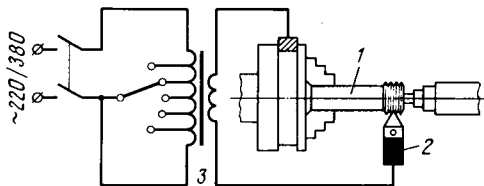
Рис. 6.13. Схема электромеханического способа накатывания деталей
