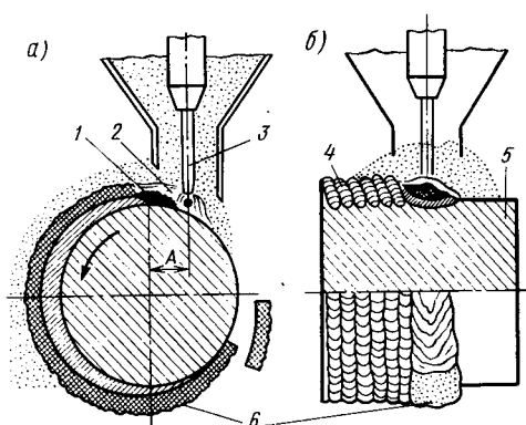
Рис. 7.5. Схема наплавки под слоем флюса: а — поперечный разрез; б — продольный разрез; 1 — ванна расплавленного металла; 2 — расплавленный флюс; 3 — электродная проволока; 4 — наплавленный слой металла; 5 — деталь; 6 — шлаковая корка; А — смещение электродной проволоки с зенита
