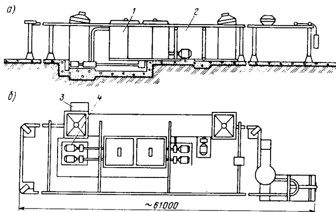
Рис. 1.6. Моечная установка ОМ-4267:
