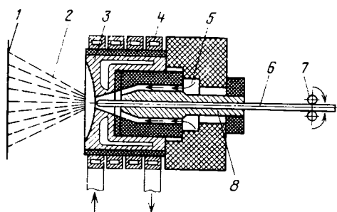
Рис. 9.9. Распылительная головка высокочастотного устройства для напыления: 1 — напыляемая поверхность; 2 — газометаллическая струя; 3 — концентратор тока; 4 — индуктор ТВЧ; 5 — воздушный канал; 6 — проволока; 7 — подающие ролики; 8 — направляющая втулка
