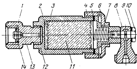
Рис. 7.12. Осушитель углекислого газа: 1 — винт; 2 — решетка; 3 — сетка; 4 — гайка; 5, 9 и 14 — прокладки; 6 — крышка; 7 — пружина; 8 и 13 — штуцера; 10 — болт; 11 — поглотитель влаги; 12 — корпус
