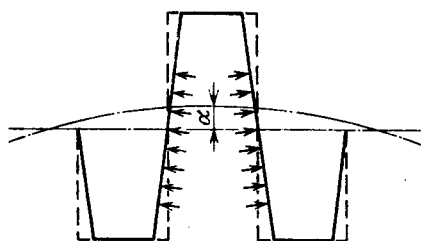
Рис. 6.20. Правка коленчатого вала местным наклепом:
