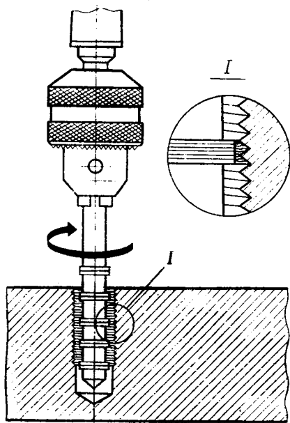
Рис. 5.14. Очистка резьбовых отверстий от грязи ершом
