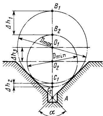
Рис. 12.1. Влияние угла призмы на точность установки
