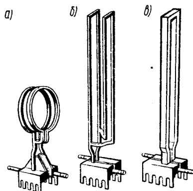
Рис. 8.7. Индукторы для нагрева наружных наплавляемых поверхностей: а — с двумя витками, соединенными параллельно; б — прямоугольный; в — петлевой
