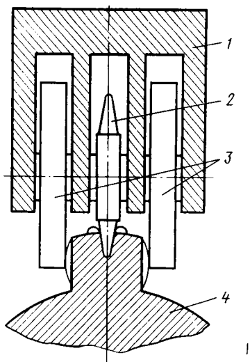
Рис. 6.10. Восстановление шлицев вдавливанием:
