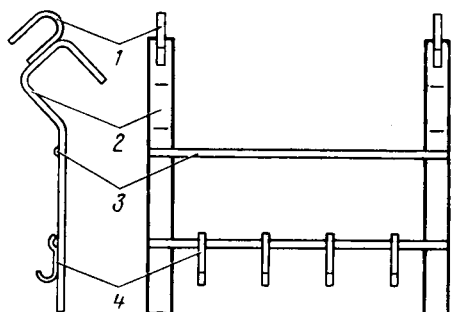
Рис. 10.16. Подвесочное приспособление: 1 — ручка-крючок, приваренная к подвесному крюку; 2 — подвесной крюк; 3 — ручка-перекладина, приваренная между подвесными крюками; 4 — крючки-контакты для подвески деталей
