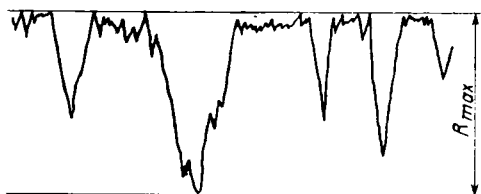
Рис. 4.7. Профиль участка гильзы при плоско- вершинном хонинговании
