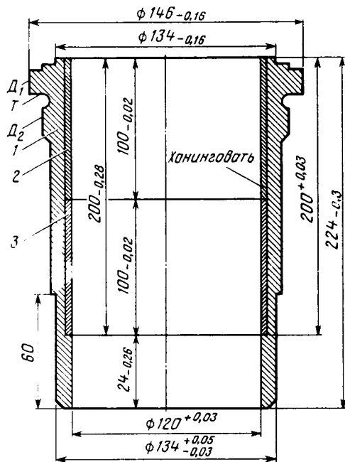
Рис. 5.24. Геометрические размеры гильзы цилиндров КамАЗ-740, восстановленной под номинальный размер: D_1 , D_2 , T — посадочные поверхности гильзы цилиндров; 1 — гильза цилиндра; 2 и 3 — соответственно верхняя и нижняя облицовочные пластины
