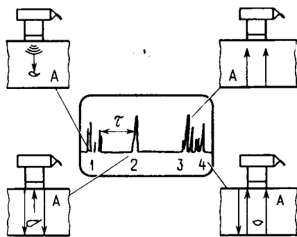
Рис. 2.10. Схема акустического контроля объекта А по методу отраженного излучения: 1 — начальный импульс; 2 — импульс от дефекта; 3 — донный импульс; 4 — многократно отраженные импульсы; \tau — временной интервал
