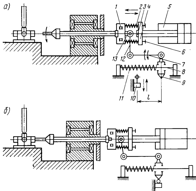
Рис. 6.27. Принципиальная схема путевого датчика установки УВК-1: а — исходное положение; б — положение при окончании процесса раздачи
