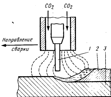
Рис. 7.8. Схема сварки (наплавки) в среде углекислого газа:
