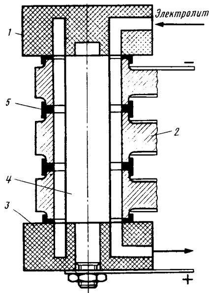
Рис. 10.13. Восстановление нижних головок шатунов железнением в проточном электролите:
