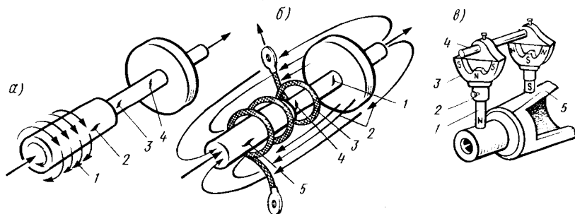
Рис. 2.11. Способы намагничивания деталей:
