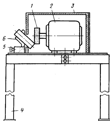
Рис. 6.34. Приспособление для полирования наружных фасок пальцев
