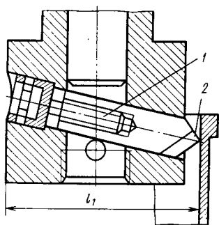
Рис. 4.4. Регулировка винта резца
