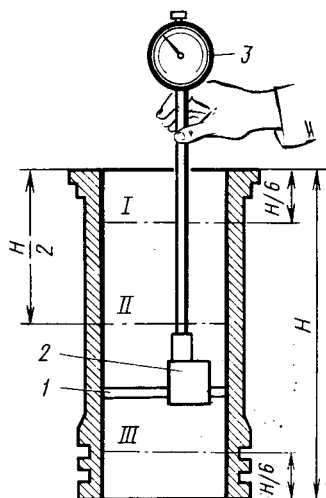
Рис. 2.4. Схема измерения диаметра гильзы цилиндра
