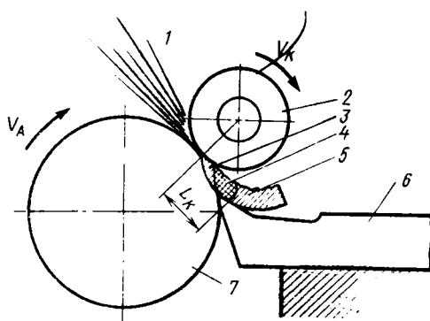
Рис. 12.4. Схема абразивно-лезвийного способа обработки:
