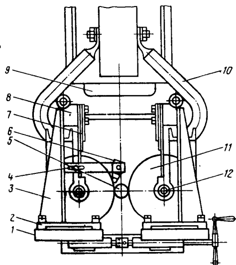
Рис. 8.2. Головка ГКН-Р1 для электроконтактной приварки проволоки: 1 — суппорт; 2 — основание; 3 — кронштейн; 4 — планка; 5 — восстанавливаемая деталь; 6 — направляющий мундштук; 7 — рессора; 8 — опора; 9 — трансформатор; 10 — токоведущие шины; 11 — сварочные ролики; 12 — ось
