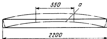
Рис. 6.21. Стальной брус квадратного сечения ( 30 \times 30 мм), выправленный газопламенным методом
