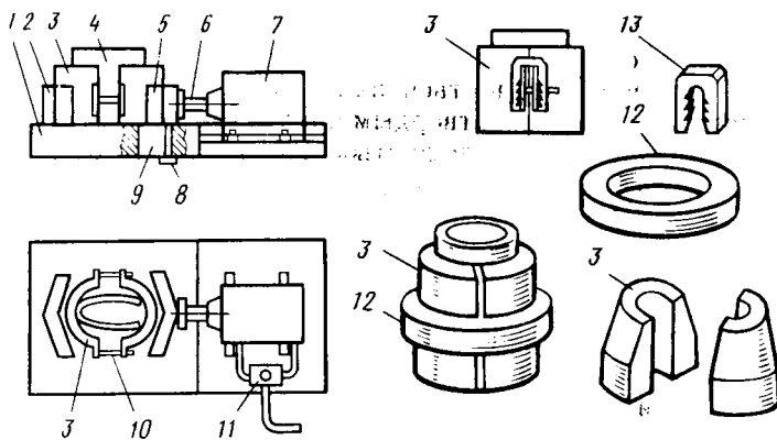
Рис. 5.22. Механизированная пресс-форма для свертывания пластин в цилиндр: 1 — плита приспособления; 2 — неподвижный упор полукольца пресс-формы; 3 — полукольцо пресс-формы; 4 — пластина, предварительно свернутая; 5 — подвижный упор полукольца пресс-формы; 6 — шток пневмоцилиндра; 7 — направляющий болт штифта; 8 — направляющий штифт подвижного полукольца; 9 — направляющий штифт подвижного полукольца; 10 — направляющий штифт подвижного полукольца; 11 — рычажок с тройником; 12 — кольцевой замок пресс-формы; 13 — накидной замок пресс-формы
