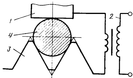
Рис. 8.3. Восстановление резьбы электроконтактной приваркой проволоки: 1 — роликовый электрод; 2 — трансформатор; 3 — витки резьбы; 4 — присадочная проволока
