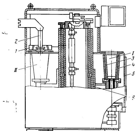
Рис. 6.28. Схема установки ОР-11301 для термопластичного обжата гильз цилиндров: I позиция — загрузка, выгрузка гильз; II позиция — рабочая
