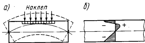
Рис. 6.19. Правка наклепом: а — направление изгиба детали; б — эпюра остаточных напряжений. Пунктиром показано конечное состояние детали
