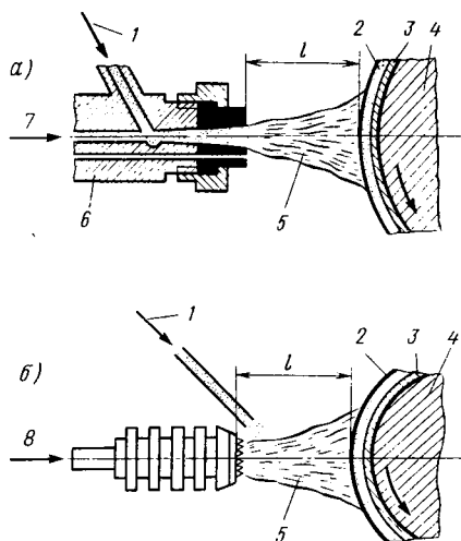
Рис. 9.3. Принципиальная схема подачи порошка при газопламенном напылении: а — инжекцией струи кислорода; б — силами гравитации; 1 — подача порошка; 2 — напыленный слой; 3 — подслой; 4 — деталь; 5 — факел пламени; 6 — горючая смесь; 7 — транспортирующий газ; 8 — подача рабочего газа; l — дистанция напыления
