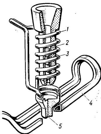
Рис. 8.13. Схема наплавки жидким сплавом толкателей автомобильных двигателей:
