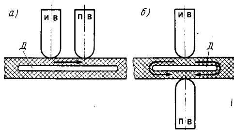
Рис. 2.17. Принципиальная схема одно- и двустороннего велосимметрического контроля:
