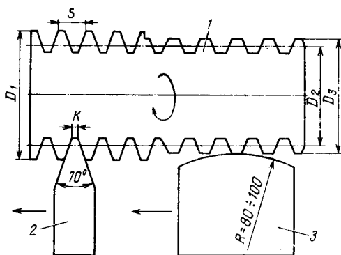
Рис. 6.14. Схема накатывания и сглаживания деформированной поверхности детали:
