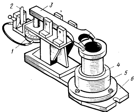
Рис. 4.2. Приспособление для установки и крепления гильз: 1—пневматический привод; 2—кран управления; 3—рычаг; 4—центрирующее кольцо; 5—корпус; 6—основание
