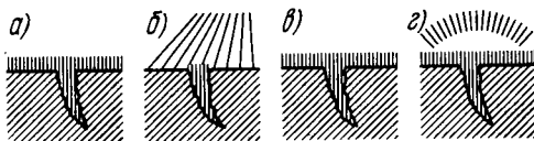
Рис. 2.13. Схема капиллярной дефектоскопии: а — нанесение индикаторной жидкости; б — удаление излишков жидкости; в — нанесение проявляющей смеси; г — наблюдение индикаторного рисунка
