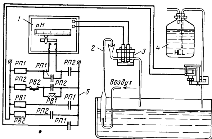
Рис. 10.20. Схема автоматического регулирования кислотности (pH) электролита: 1 — pH-метр; 2 — аэролифт; 3 — датчик; 4 — бутылка с кислотой; 5 — автоматический регулятор
