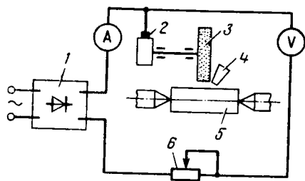
Рис. 12.5. Схема электрохимического шлифования
