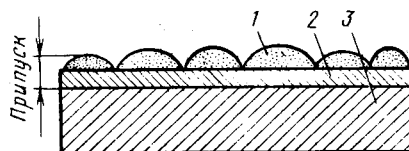
Рис. 12.3. Схема разреза восстанавливаемой детали с образованным на ней припуском и дефектным слоем:
