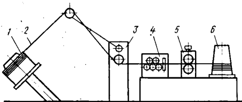
Рис. 5.9. Волоочильный стан для получения ромбической проволоки: 1 — установочный барабан; 2 — проволока; 3 — устройство для аварийной остановки стана; 4 — правильное устройство; 5 — роликовая волока; 6 — приемный барабан
