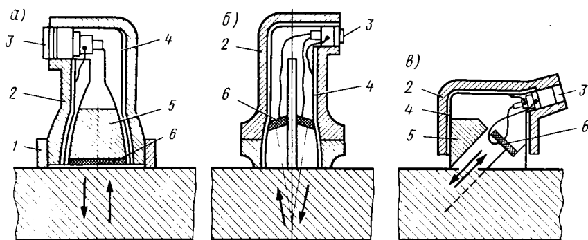
Рис. 2.6. Конструкция нормального (а), раздельно-совмещенного (б) и наклонного (в) искателей: 1 — протектор; 2 — корпус; 3 — штепсельный разъем; 4 — экран; 5 — демпфер; 6 — пьезопластина. Стрелками обозначают направление ультразвукового сигнала
