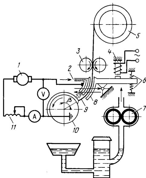
Рис. 7.14. Схема установки для вибродуговой наплавки:
