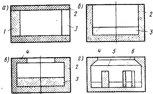
Рис. 10.5. Ячейки для получения равномерных покрытий на плоских деталях: а — двухэлектродная; б — одноэлектродная; а — с выравнивающими козырьками; б — с непроводящими вставками; 1 — анод; 2 — непроводящий экран; 3 — катод; 4 — козырек; 5 — непроводящая вставка; 6 — трубчатая непроводящая вставка
