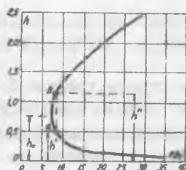
Рис. 11.3. График прыжковой функции \Pi(h)
