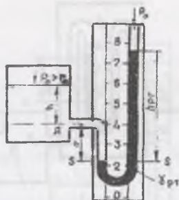
Рис. 2.4. U-образный ртутный манометр
