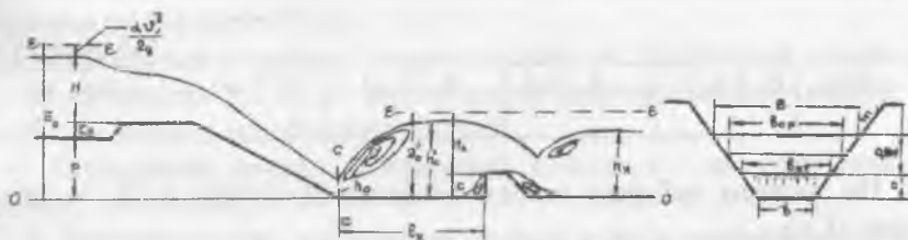
Рис. 15.2. Водобойная стенка
