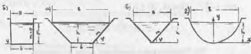
Рис. 9.2. Примеры поперечного сечения канала
