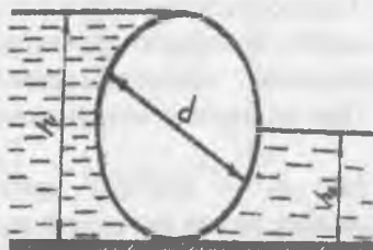
Рис. 4.2. Примеры построения тела давления
