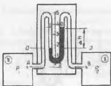
Рис. 2.8. Дифференциальный манометр
