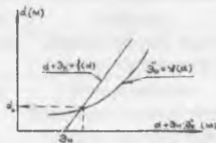
Рис. 15.4. Определение теоретической глубины колодца
