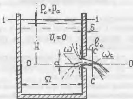
Рис. 8.1. Истечение жидкости из малого отверстия в атмосферу
