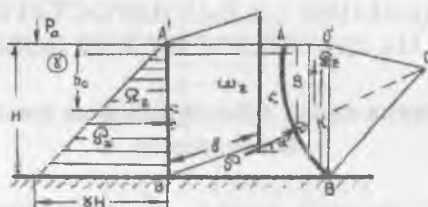
Рис. 4.1. Эпюра давления на цилиндрическую поверхность ABC а) б) в)
