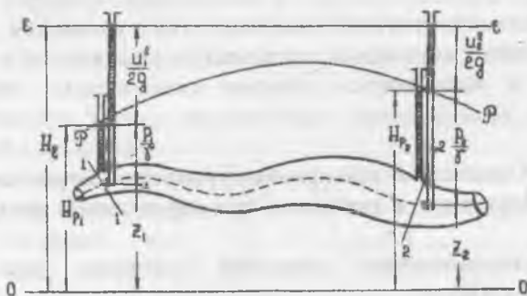
Рис. 5.1. Геометрическая интерпретация уравнения Бернулли для идеальной жидкости
