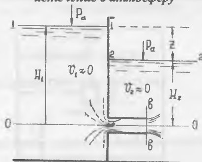
Рис. 8.6. Истечение под уровень через насадок
