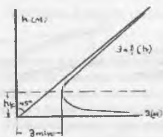
Рис. 10.5. График удельной энергии сечения
