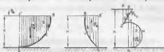
Рис. 4.1. Эпюра давления на цилиндрическую поверхность ABC а) б) в)
