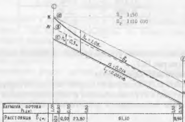
Рис. 10.7. Построение кривой свободной поверхности по способу Б.А.Бахметева
