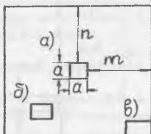
Рис. 8.3. К вопросу о типе сжатия струй
