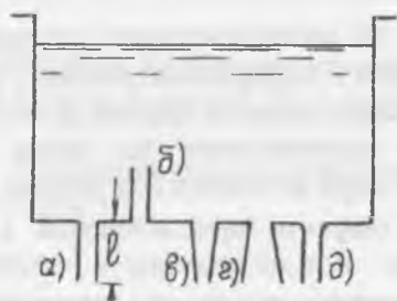
Рис. 8.4. Типы насадков
