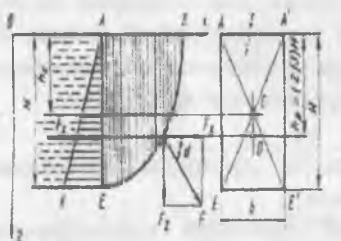
Рис. 4.2. Примеры построения тела давления
