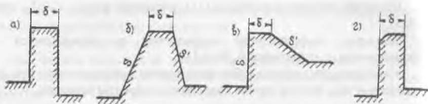
Рис. 12.7. Водосливы практического профиля
