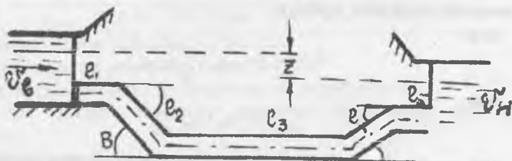
Рис. 6.2. Схема дюкера
