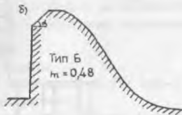
Рис. 12.6. Водосливы практического профиля криволинейного очертания
