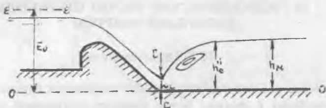
Рис. 14.4. Прыжок в сжатом сечений
