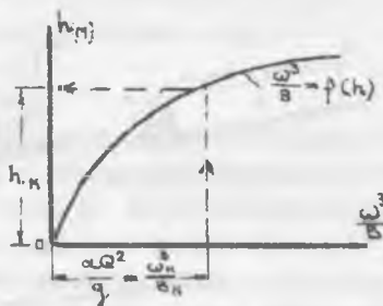
Рис. 10.6. Определение критической глубины
