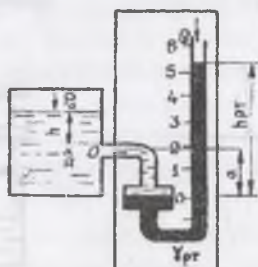
Рис. 2.7. Чашечный мановакуумметр
