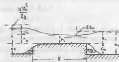
Рис. 12.3. Подтопленный водослив с широким порогом
