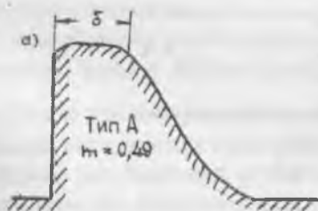
Рис. 12.6. Водосливы практического профиля криволинейного очертания
