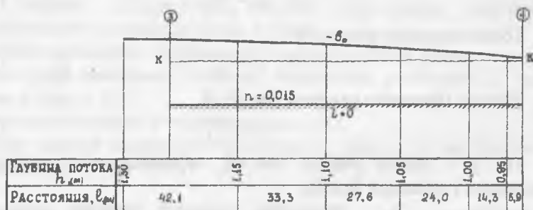
Рис. 10.8. Построение кривой свободной поверхности по способу В.И. Чарнамского
