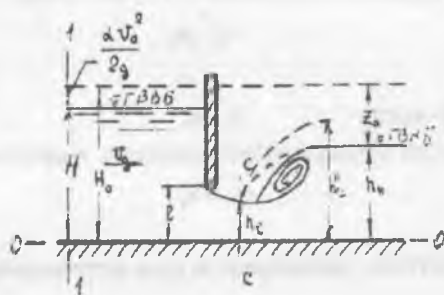
Рис. 13.1. Свободное истечения из-под щита
