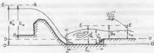
Рис. 15.1. Водобойный колодец
