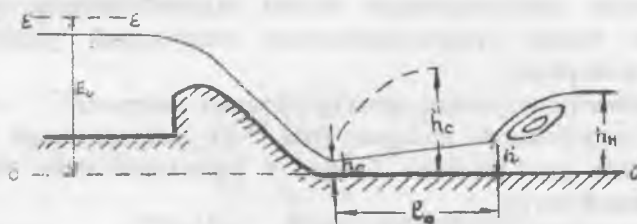
Рис. 14.5. Сопряжение бьефов при помощи отогнанного прыжка
