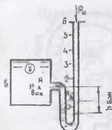
Рис. 2.5. U-образный вакуумметр
