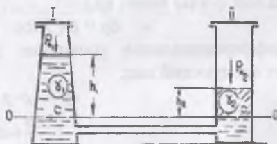
Рис. 2.2. К закону сообщающихся сосудов
