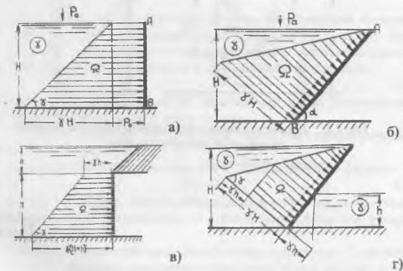
Рис. 3.1. Эпюра гидростатического давления
