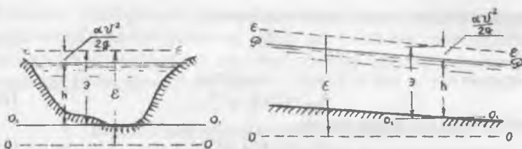
Рис. 10.4. К определению удельной энергии сечения \mathcal{E}
