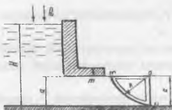
Рис. 4.3. Сила давления на круговую поверхность
