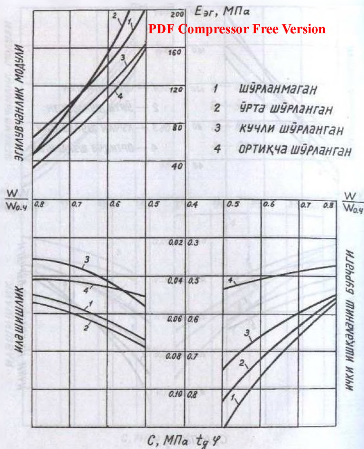
51-расм. Турли даражадаги шўрланган тупроқлар учун K_3=1,05 ҳолатидаги E_{\text{г}} , C_{\text{га}}=f(W/W_{0.4}) боғланишларини мужассамлаштирган график
