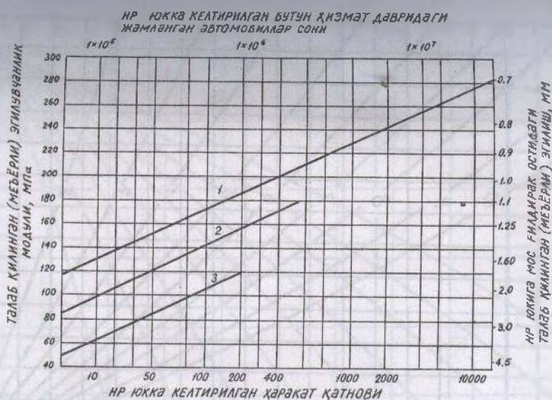
73-расм. Талаб қилинган (ноқулай ҳолатли) букилишни ва ноқулай ҳолатдаги ҳаракат қатновига боғлиқ (хунлик) НР автомобилига келтирилган йўл тўшамасининг этигувчанлик модулини аниқлаш графиги: 1—мукамал турдаги қоп- ламаларда; 2—енгил турдаги қопламаларда; 3—ўткинчи турдаги қопламаларда
