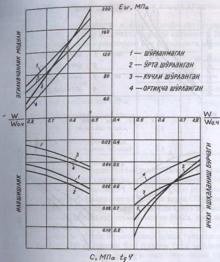
50-расм. Турли даражада шўрланган тупроқлар учун K_3=1,0 ҳолатидаги E_{\alpha, C} tg\alpha=f(W/W_{0.4}) боғланишларни мужассамлаштирган график
