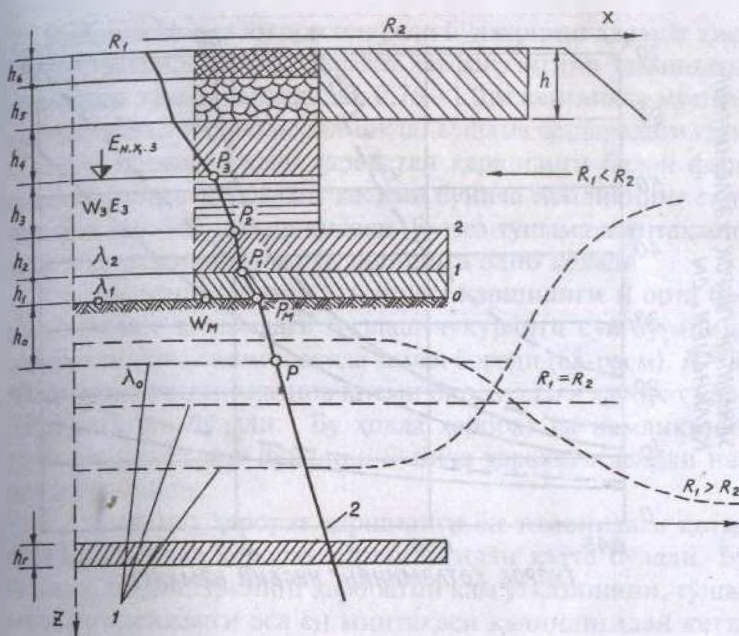
68-расм. Сув-ҳарорат тартибини ҳисобга олиб лойиҳаланган йўл тушамасининг қатламлари: 1—музлаш чегараси; 2—туйинган сув буғининг эгилувчанлик чизиғи; h_1 — W_m ҳолатида K_1=0,98-1,0 гача зичланган тупроқ; h_1 —буғ тўсқич қатлам; h_2 —ҳарорат тўсқич; h_3 —сув ва совуққа кам чидамли қатлам; h_4 — h_6 тушама асосининг қатламлари ва қопламаси; h_5 —сув тўсқич қатлам
