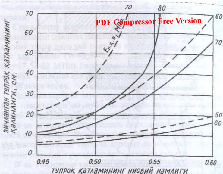
69-расм. Зичланган тупроқ қатлам қалинлигини унинг қурилиш вақтидаги намлиги ва қабул қилинаётган E_{н.х.з.} га боғлаб топish учун номограмма (узлуксиз чизиклар — огир саз тупроқлар ва чангли қум тупроқлар учун қирқимдилари — огир чангсимон саз тупроқлар ва ёпишқоқ тупроқлар учун).
