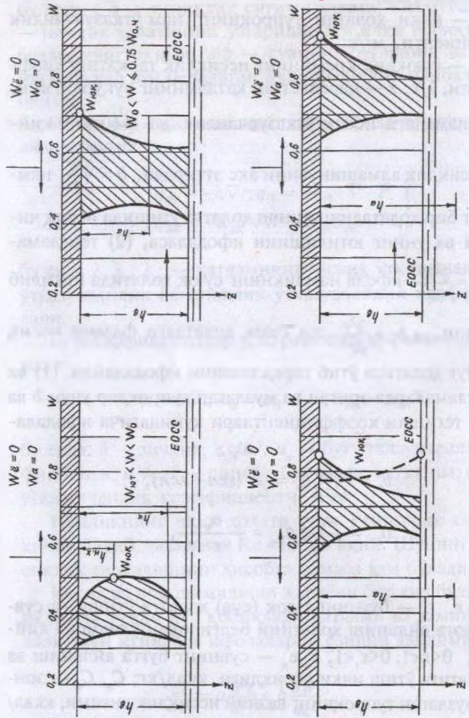
11-расм. Курғоқчилик туманларида йўл қобиғининг сув-ҳарорат тартибини ажратиш: I— дифузион тартиб; II—дифузион тартиб; III—геологик намсилжишли тартиб; IV—гидрогеологик нам силжишли тартиб
