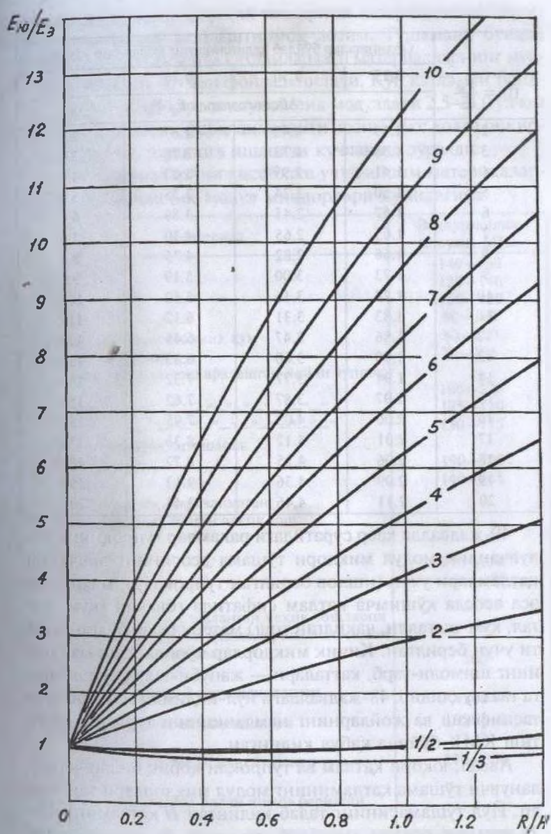
75-расм. E_1/E_9=0,4 ҳолатида нокир йўл тўшамасини ҳисоблаш учун номограмма
