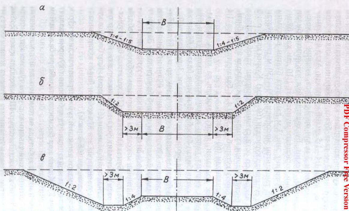
60-расм. Учар қумларда йўлнинг ўйма ҳолатидаги қўндаланг қиёфалари: а—2 м гача чуқурликда; б—2 м дан чуқур супачали; в—2 м дан чуқур кўтарма қўринишда
