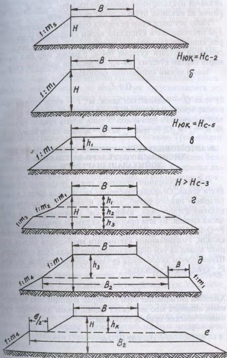
64-расм. Қўтарма ҳолатидаги тупроқ қобиғининг кўндаланг қиёфали кўримлари
