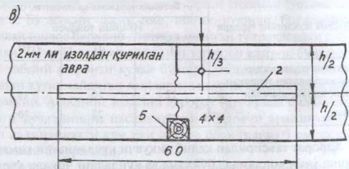
3-расм. Чокларнинг тузилиши: а—кеңгайишдаги; б—сиғилишдаги; в—алдамчи сиқилиш чоки. 1—сеймон бетон; 2—пўлат даста; 3—дастани битум билан ёғлаш; 4—чокни махсус қоримша билан тўлдириш; 5—ёғоч пайраҳали қатлам; 6—кийдиргич; 7—кийдиргич қиринди ёки каноп жуни билан тўлдириш
