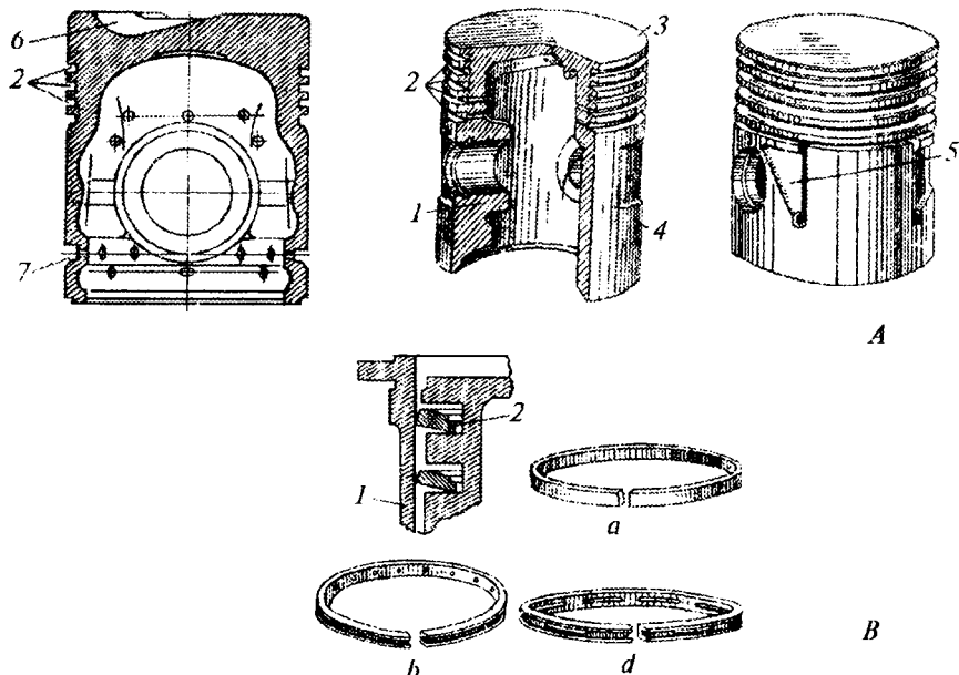
3.4-rasm. Porshen (A): 1 — bobishka; 2 — halqa ariqchalari; 3 — tubi; 4 — yo'naltiruvchi qism; 5 — kesik; 6 — diffuzor osti o'yig'i; 7 — moy o'tadigan teshiklar; va porshen halqalari (B): 1 — silindr; 2 — konussimon qirgimli halqa; a — kompression halqa; b, d — moy sidirgich halqalari
