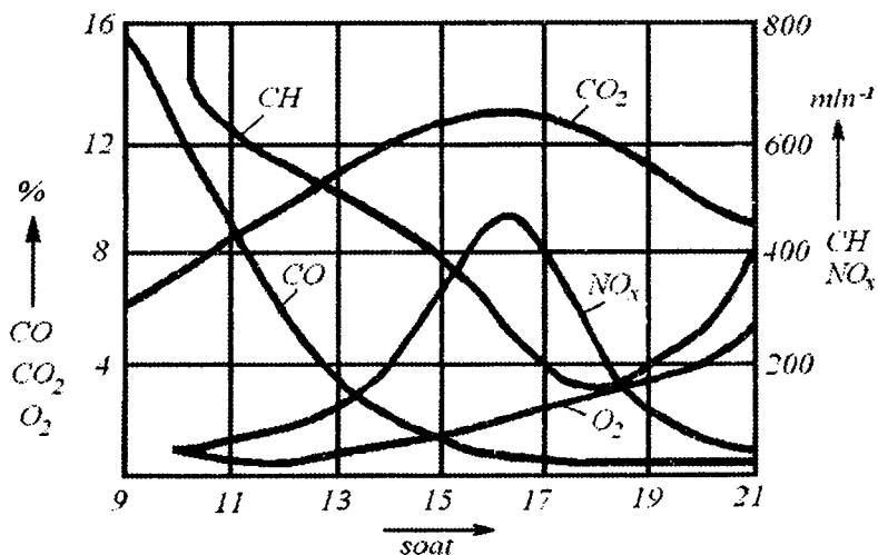
28.2-rasm. Kun mobaynida emissiya tarkibining o'zgarish grafigi
