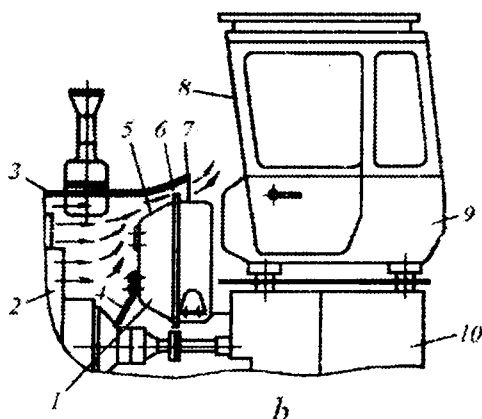
28.4-rasm. Kabinani traktorda joylashtirish:
