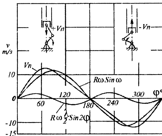
14.3-rasm. Porshen tezligi grafigi
