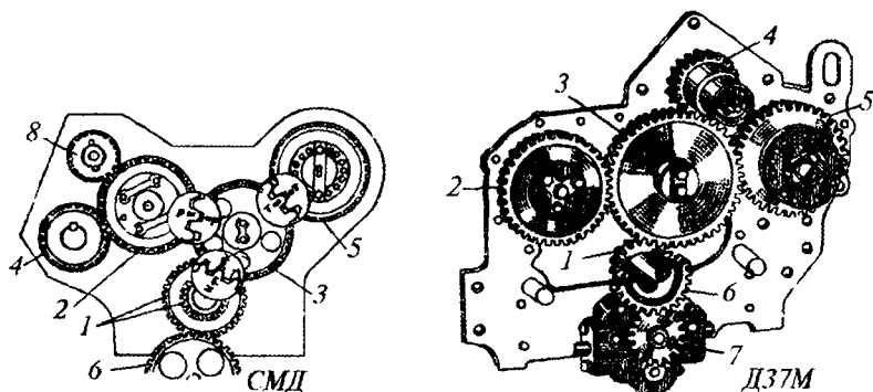
4.6-rasm. Taqsimlash shesternalarining joylashtirish sxemasi:
