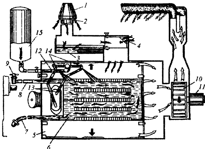
28.7-rasm. MT3-80 traktori mikroiklimni mo'tadillash tizimi sxemasi:
