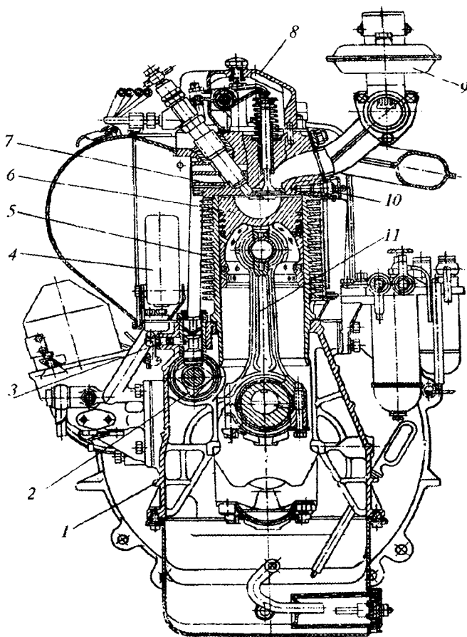
2.13-rasm. Havo bilan sovitiladigan to'rt taktili dizel motorining ko'ndalang qirqimi:
