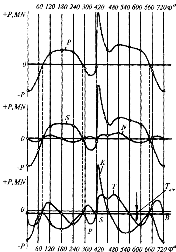
14.7-rasm. Tirsakli val burilishi burchagi boʻyicha P , N , S , K va T kuchlar grafiklarini qurish
