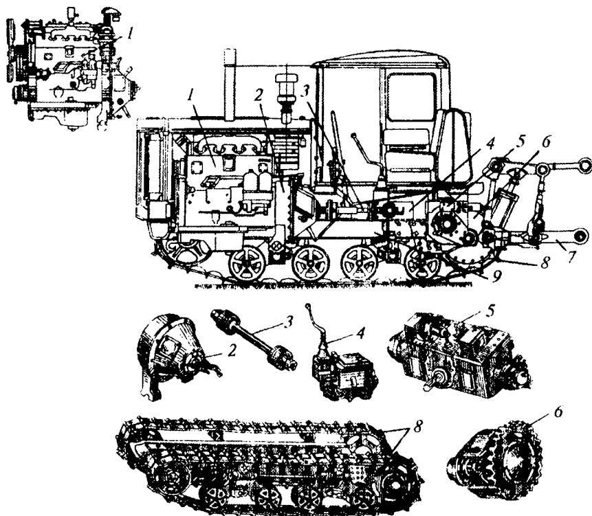
1.1-rasm. O'rmalovchi zanjirli traktorning umumiy ko'rinishi va asosiy mexanizmlari:
