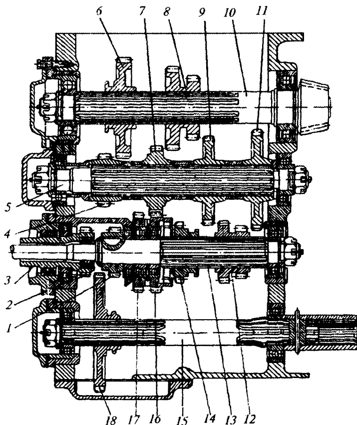
17.10-rasm. Bir necha juft shesternasi ilashadigan uzatmalar qutisining tuzilishi (TT3-100 K.11):
