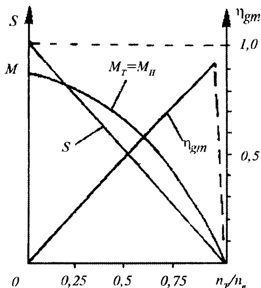
15.5-rasm. Gidromuftaning tashqi tavsifi
