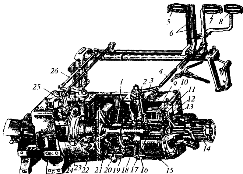
18.11-rasm. O'rmalovchi zanjirli traktorning (JT-75) ketingi ko'prigi:
