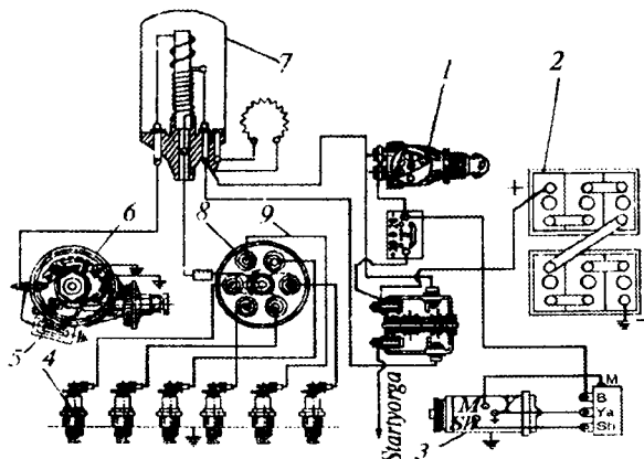
11.9-rasm. Olti silindrli motor batareyali yondirish tizimining sxemasi:
