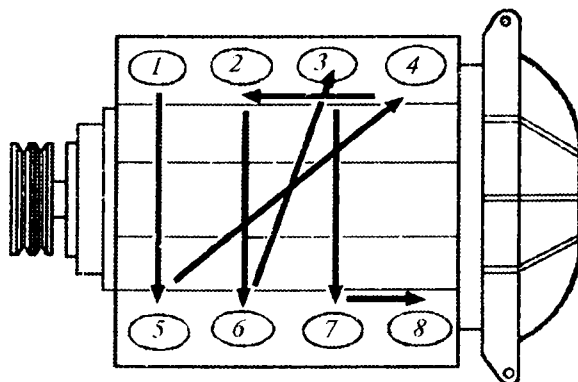
2.11-rasm. Sakkiz silindrlı motor silindrlarining joylashtirilishi va ishlash tartibi
