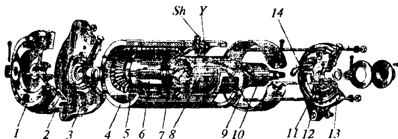
11.7-rasm. O'zgarmas tok generatori:
