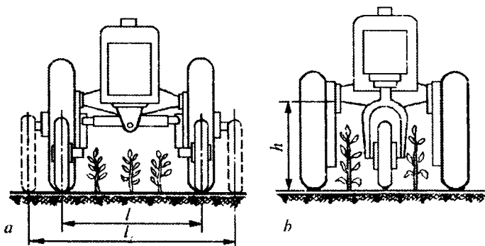
19.3-rasm. G'ildirakli traktorlar koleyasi (a) va agrotexnika masofasi (b)
