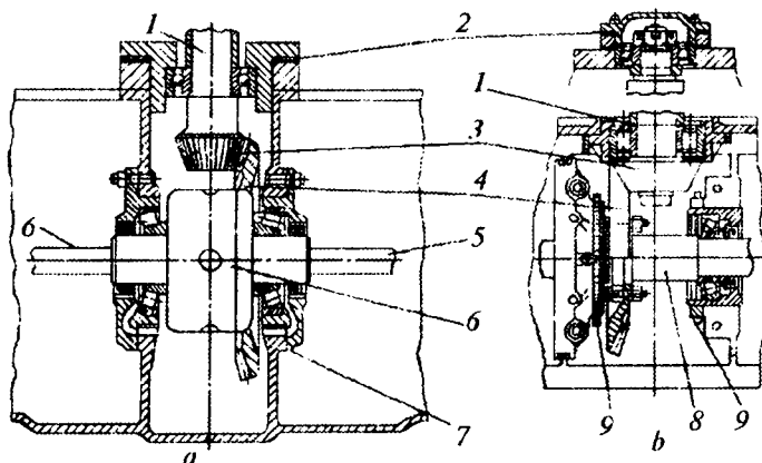
18.2-rasm. Traktorning asosiy uzatmalari:
