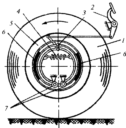
20.10-rasm. Kolodkali tormozning ishlash sxemasi:
