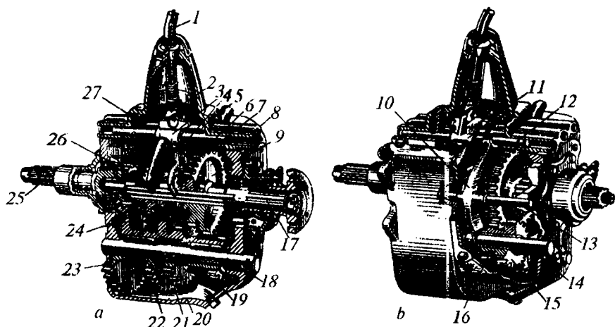
17.9-rasm. To'g'ri uzatmali uzatmalar qutisining (TA3-51A) tuzilishi:
