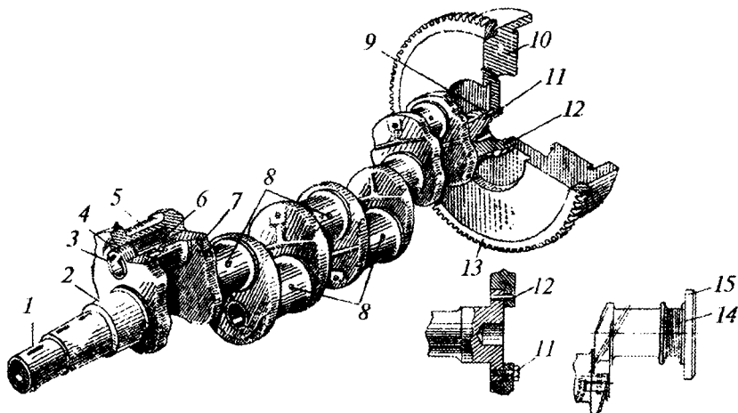
3.7-rasm. Tirsakli val va maxovik:
