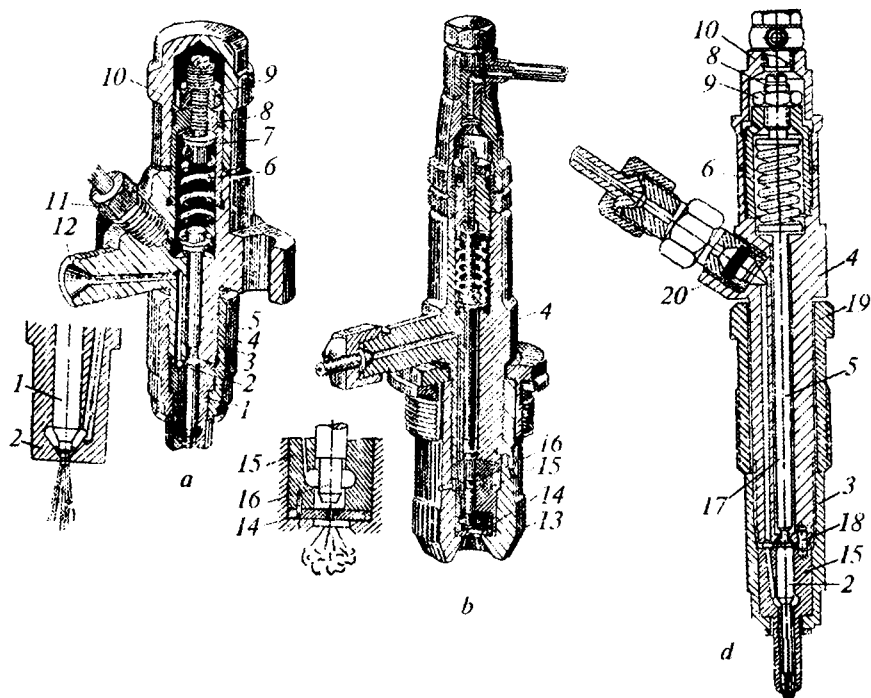
7.13-rasm. Forsunkalar:
