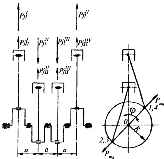
14.10-rasm. To'rt taktli, bir qatorli to'rt silindrlı motorni muvozanatlash
