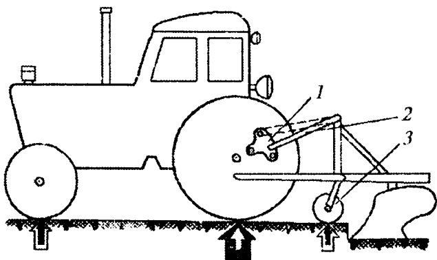
21.12-rasm. Traktor yetakchi g'ildiraklari mexanik vazminlashtirgichining sxemasi:
