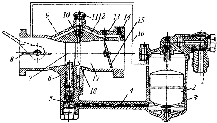
6.9-rasm. Aralashma oqimi gorizontol yo'naltirilgan karburator (K-16A) ning sxemasi:
