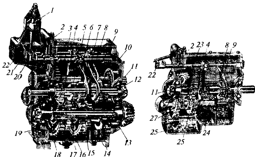
11.7-rasm. Bir juft shesternasi ilashadigan uzatmalar qutisining (DT-75) tuzilishi:
