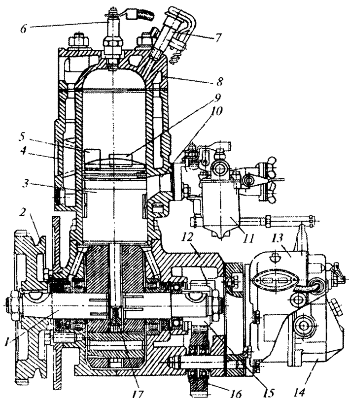
12.2-rasm. ПД-10M yurgizib yuborish motori (maxovik va startyor g'ilo'i olingan holda):
