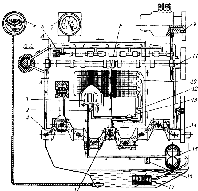
9.9-rasm. Kombinatsiyalangan moylash tizimining (Д-144) sxemasi:
