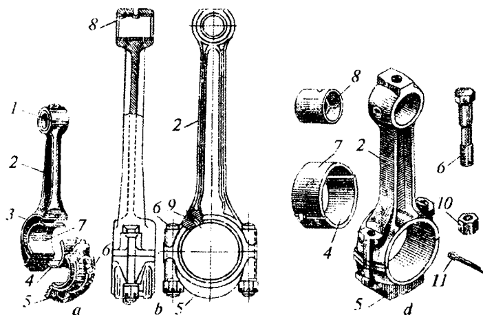
3.6-rasm. Shatunlar: 1 — yuqorigi kallak; 2 — sterjen; 3 — pastki kallak; 4 va 7 — po'lat vkladishlar; 5 — pastki kallak qopqog'i; 6 — shatun bolti; 8 — vtulka; 9 — pastki kallak teshigi; 10 — gayka; 11 — shplint
