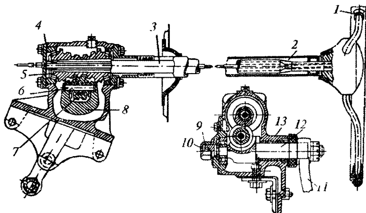
20.7-rasm. Avtomobilning rul mexanizmi:
