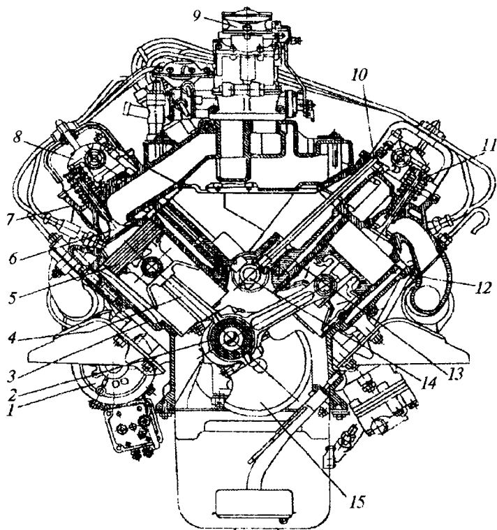
2.15-rasm. Silindrlari «V» tarzda joylashtirilgan benzinli motorning ko'ndalang qirqimi:
