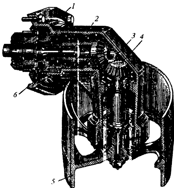
21.3-rasm. Traktorning harakatlantirish shkivi: 1 — choʻyan korpus; 2 — quvvat olish vali; 3 va 4 — konus shesterna; 5 — shkiv; 6 — qistirma
