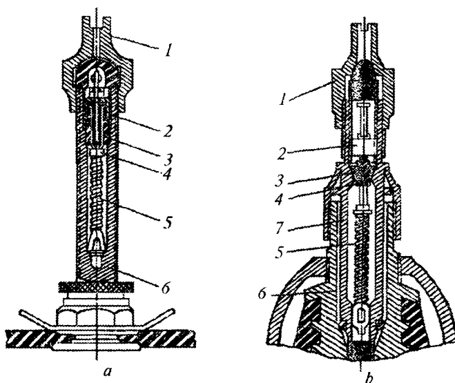
19.11-rasm. Avtomobil (a) va traktor (b) shinalarining ventili:
