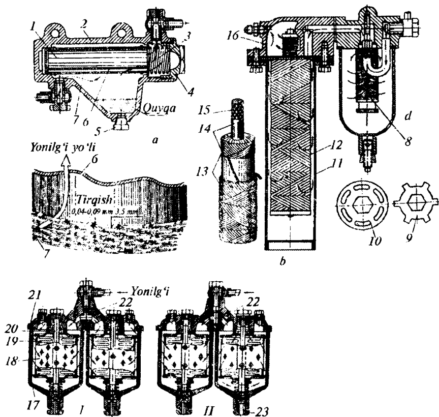
7.4-rasm. Yonilg'i filtrlari: a — metall tasmani, b — mayin, d — metall plastinali, e — buklama qog'oz elementli filtrlar; 1 — metall tasmani filtrlovchi element; 2 va 11 — korpus; 3 — prujina; 4 — qisuvchi tiqin; 5 — konus tiqin; 6 — stakan; 7 — jez tasma; 8 — metall plastinali filtrlovchi element; 9 — yulduzcha; 10 — disk; 12 — ipli filtrlovchi element; 13 — ip; 14 — filtrlovchi qog'oz; 15 — sim to'r quvurcha; 16 — qopqoq; 17 — filtrlar korpusi; 18 — karten silindr; 19 — filtrlovchi element; 20 — sterjen; 21 — qopqoq; 22 — uch yo'lli jo'mrak; 23 — tiqin bolt
