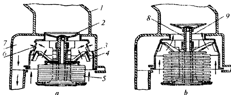
10.7-rasm. Termostat va uning ishlash sxemasi: a — suvning kichik doira bo'ylab, b — suvning katta doira bo'ylab harakat qilishi; 1 — qisqa quvur; 2 — asosiy klapan; 3 — korpus; 4 — yordamchi klapan; 5 — qovurg'ali jez silindr; 6 — teshik; 7 — kanal; 8 — shtok; 9 — korpus uyasi
