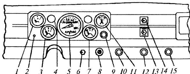
20.22-rasm. ГАЗ-51А avtomobili shchitiga joylashtirilgan asboblار
