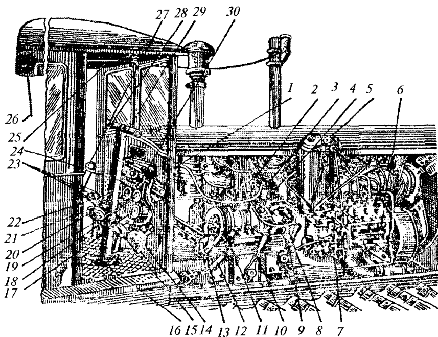
20.20-rasm. DT-75 traktorining boshqarish organlari va nazorat asboblari
