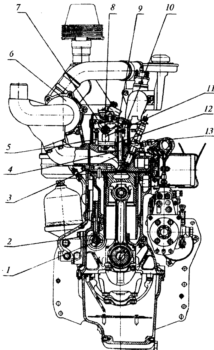
30.7-rasm. D-245 dizel motori (ko'ndalang kesim):
