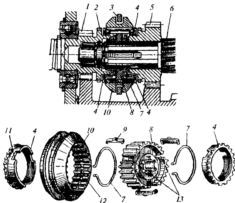
17.5-rasm. Uzatmalar qutisining sinxronizatori:
