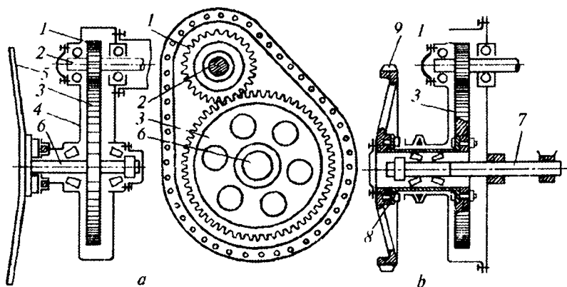
18.7-rasm. Traktorning oxirgi uzatmasi:
