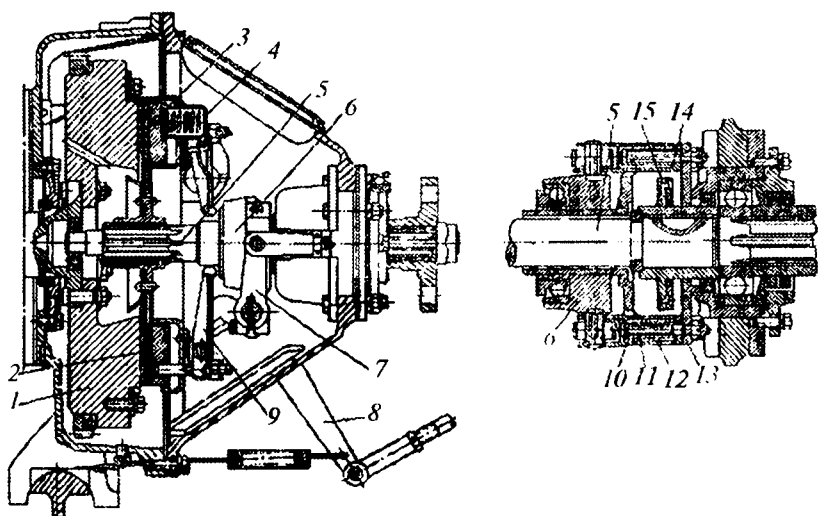
16.6-rasm. Bir diskli muftasil qo'shilgan ilashish muftasi (JT-75):
