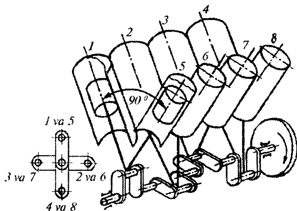
2.10-rasm. Silindrlari «V» tarzda joylashtirilgan sakkiz silindrlı motor tirsaklı valining sxemasi
