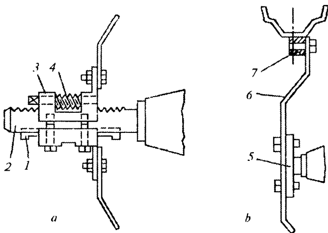
19.4-rasm. Yetakchi g'ildiraklar oralig'ini o'zgartirish usullari:
