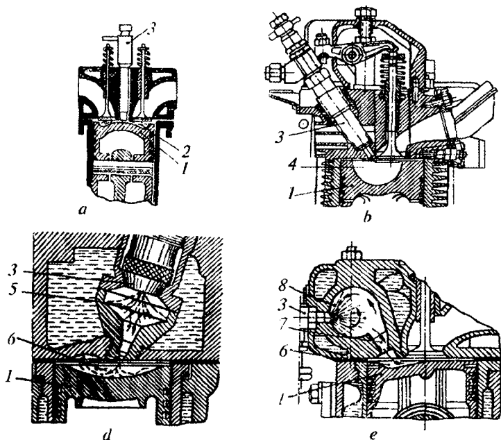
7.2-rasm. Dizel motorlari yonish kamerasining shakllari:
