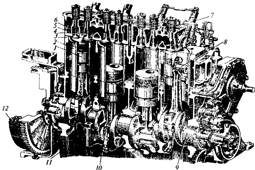
2. 12-rasm. To'rt silindrli, to'rt taktli dizel motorining bo'ylama qirgimi:
