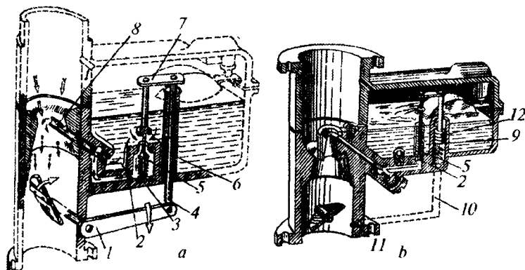
6.7-rasm. Ekonomayzerlar sxemasi:
