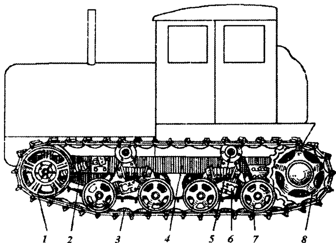
19.12-rasm. Oʻrmalovchi zanjirli traktorning yurish qismi:
