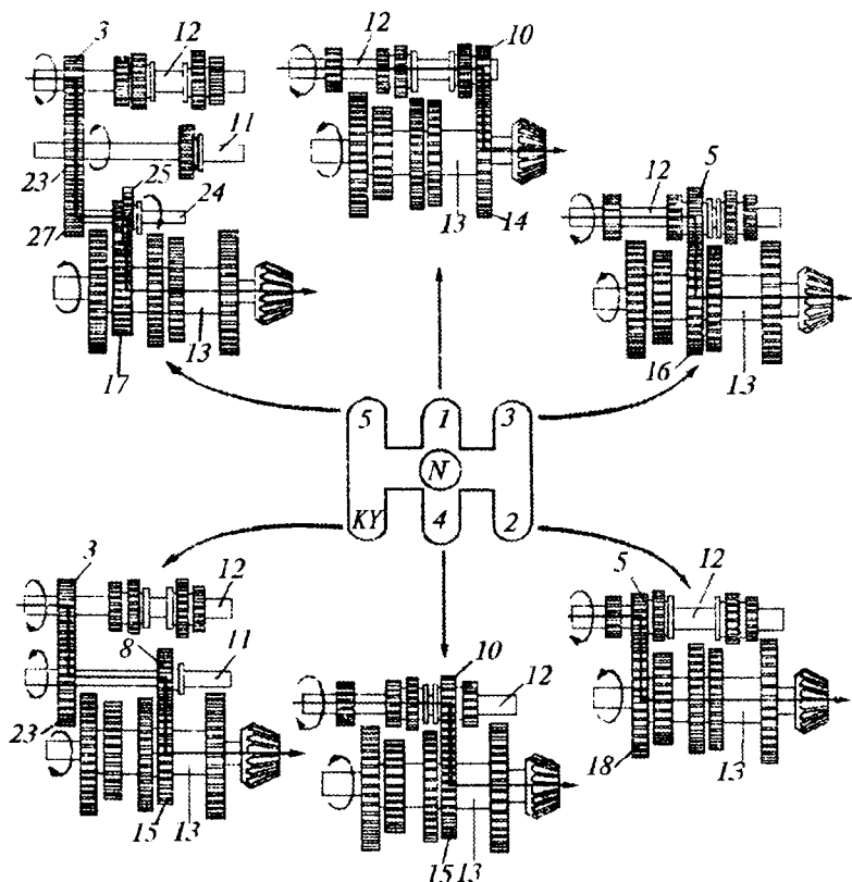
17.8-rasm. Bir juft shesternasi ilashadigan uzatmalar qutisining (JT-75) turli uzatmalarda ishlash sxemasi (raqamlar 17.7-rasmdagilarga mos keladi)
