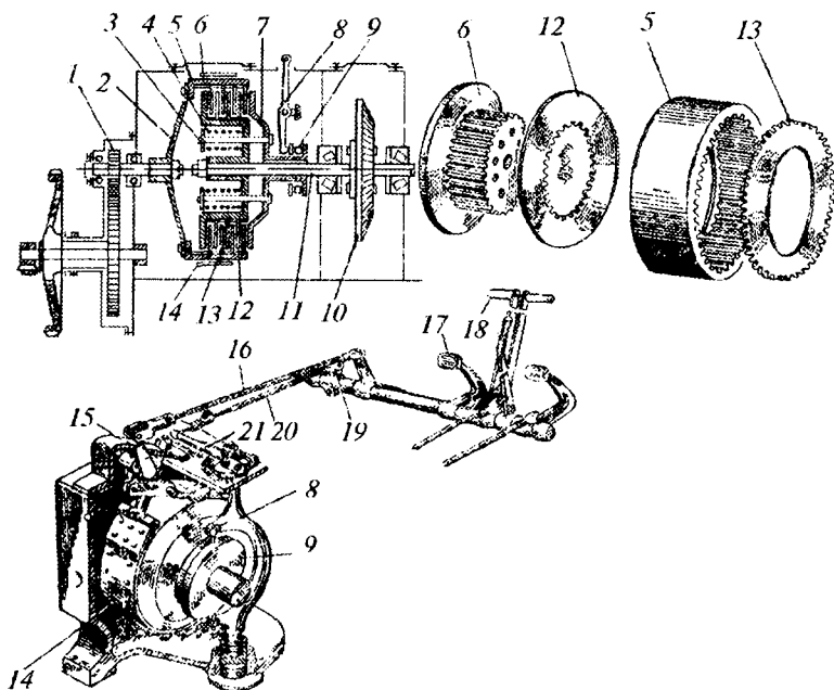
18.5-rasm. Frikcion boshqarish muftasining sxemasi:
