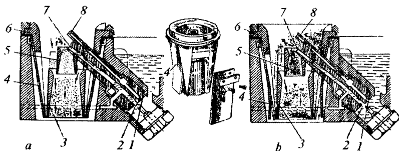
6.6-rasm. Diffuzordagi siyraklanishni o'zgartiruvchi asosiy dozalovchi tizim:
