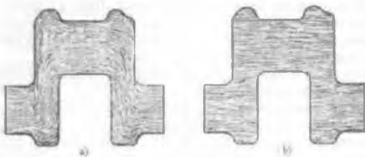
10.10-rasm. Tirsakli val mikrostrukturasi sxemasi: a – shtamplangan; b – zagotovkadun kesib olingan.
