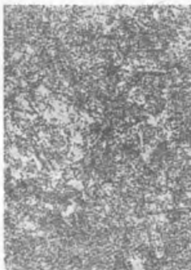
5.4-rasm. Y8 markali toblungan po'latda martensitning ninasimon strukturasi.
