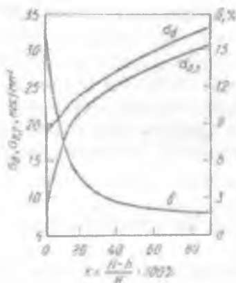
3.2-rasm. Sovuq holda prokalashda D1 markali duralyuminiyni mexanik xossasini siqilish darajasiga bog'liqligi (A. V. Tretyakov, K.M. Radchenko).
