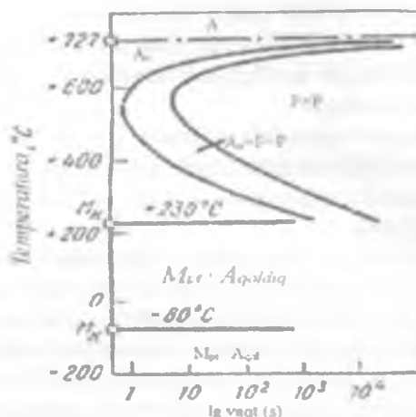
5.2 - rasm. 0,8 % C ga ega bo'lgan po'latlar uchun martensitli nuqtalari bilan S – diagramma: A – turg'un austenit; A_p – o'ta sovutilgan austenit; A_{qoldiq} – qoldiq austenit; M_p – martensit; F – ferrit; K – karbid.
