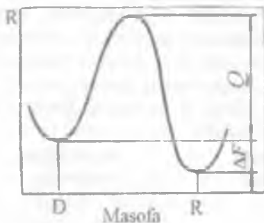
3.4 - rasm. Deformatsiyulashgan va qayta kristallangan donalar chegarasi orqali atomlarni o'tishida erkin energiyaning o'zgarish sxemasi.
