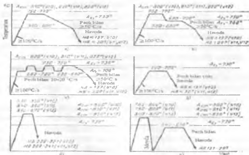
10.3-rasm. Y10, Y11 va Y12 markali po'latlarga tafsifiy etiladigan dastlabki termik ishlov berish rejimlari.
