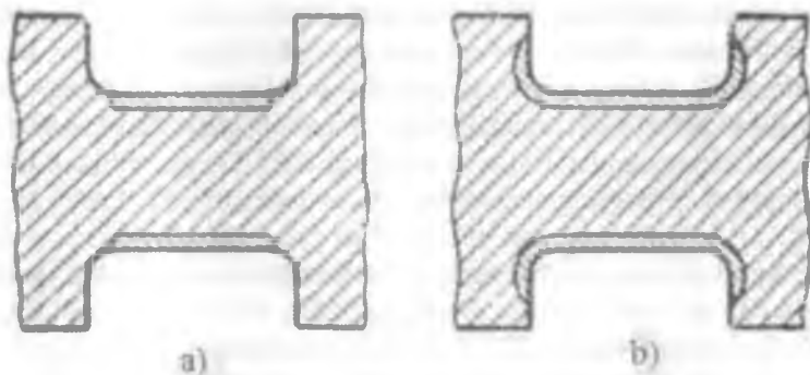
10.11-rasm. Val she'kasini toblangan qatlamning joylashishi.
