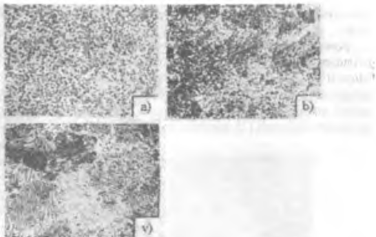
10.14-rasm. SHX15 markali po'latning mikrostrukturasi: a – normal yumshatishdagi normal holatdagi; b – yumshatishda oxirigacha qizdirilmagan holatdagi; v – yumshatishda o'ta qizish holatdagi x 500.
