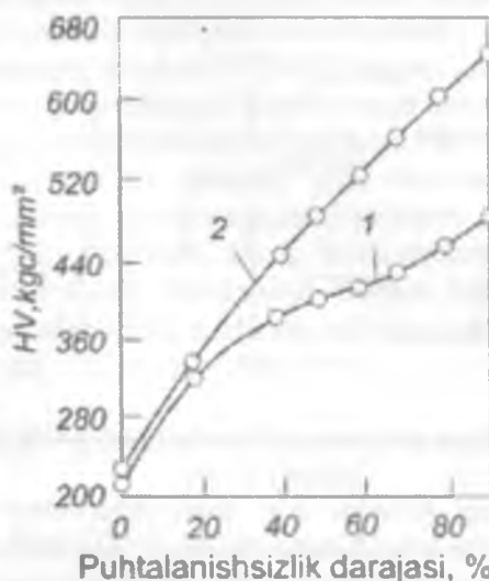
7.2-rasm. Nimonik – 90 qotishmasida 1000° C temperaturada sovuq holda cho‘zilgan va eskitirilgan qattiqligicha toblangan 4 mm diametrli simni kiryalashda siqilish darajasini ta’siri. (U. Betteridja ma’lumotiga asosan): 1 – sovuq holda cho‘zilgan; 2 – deformatsiya + 450° C temperaturada 16 soat mobaynida eskirtish.
