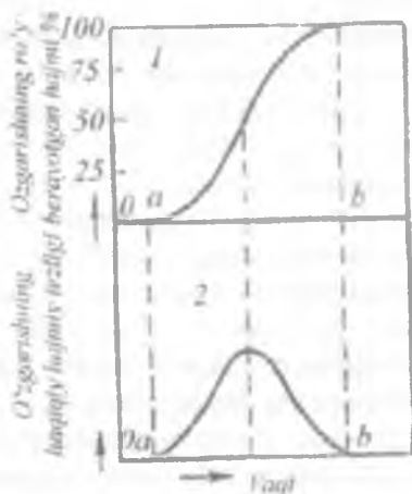
4.3-rasm. Doimiy temperaturada fazalar o'zgarishi kinetikasi: 1-kinetik egri chiziq; 2-haqiqiy hajmiy o'zgarish tezligining izotermik ushtab turish vaqtiga bog'liqligi; oa – inkubatsion davr; ab – to'liq o'zgarish vaqti.
