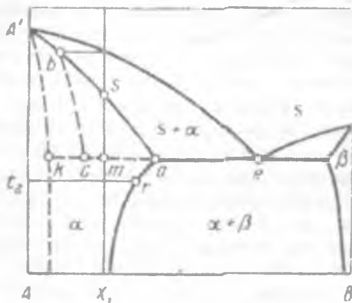
2.2-rasm. Evtetik turdagi sistemada muvozanat bo'lmagan solidus A' da va X_1 qotishmada dendritli kimyoviy notekislikda bc qattiq eritmaning o'rtacha tarkibini o'zgarish egri chizig'i.
