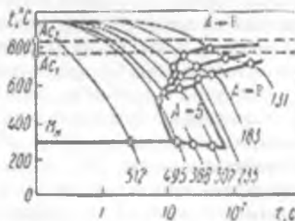
5.11-rasm. 0,34 % S, 1 % Mn, 0,76 % C ga ega bo'lgan 35FC markali po'latni termokinetik diagrammasi (K. F. Starodubov, YU. Z. Borkovskiy, V. V. Purusov).
