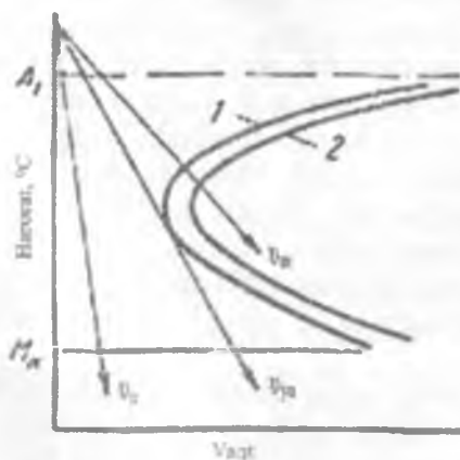
5.10-rasm. C – diagramma bo'yicha toblashning kritik tezligini aniqlash:
