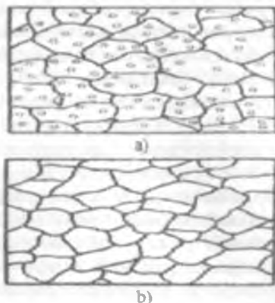
10.6-rasm. 4 % misga ega bo'lgan alyuminili qotishmani tuzilishi o'zgarishining sxemasi (toblashdan keyin). a – dastlabki holat; b – toblashdan so'ng.
