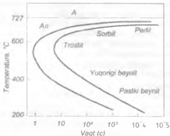
4.5-rasm. Evtektoidli po'latlar uchun austenitning izotermik o'zgarishi diagrammasini qurish:
