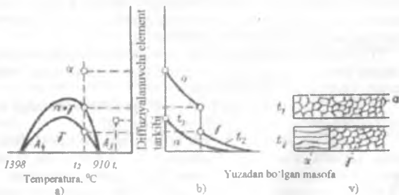
9.2-rasm. Temir – diffuziylanuvchi element holat diagrammasi sxemasi (a), qatlam qalinligi bo'yicha diffuziylanuvchi element miqdorini o'zgarishi (b) va t_1 va t_2 temperaturadagi diffuziylanuvchi qatlamning mikrostrukturasini sxemasi (v).
