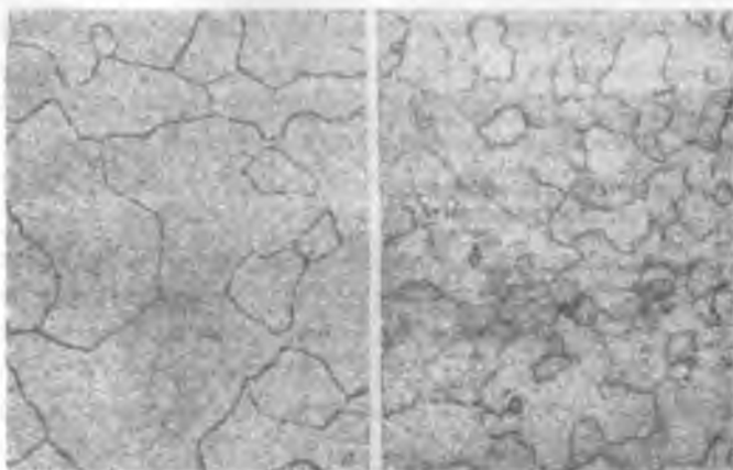
7.3-rasm. Titaning \beta qotishmasini (BT15) odatdagi toblash (a) va YUTTMIBdan keyingi (b) mikrostrukturasi. X300 (S. G. Glazunov, I. S. Pol'kin).
