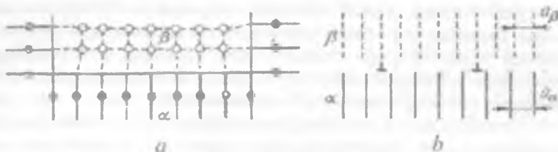
4.2-rasm. \alpha va \beta fazalr kristallar orasidagi kogerentli (a) va yarimkogerentli (b) chegaralarini tuzilishi sxemasi.
