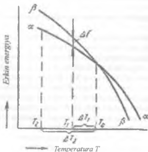
4.1-rasm. Ikki fazaning erkin energiyasini temperaturaga bog'liqligi.
