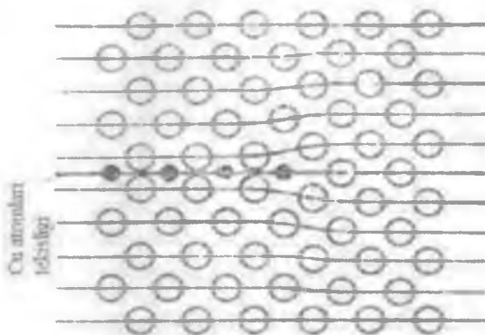
10.7-rasm. Gin'e – Preston zonasi sxemasi (Gerol'd bo'yicha): oq aylana – alyuminiy atomlari; qora aylana – mis atomlari.
