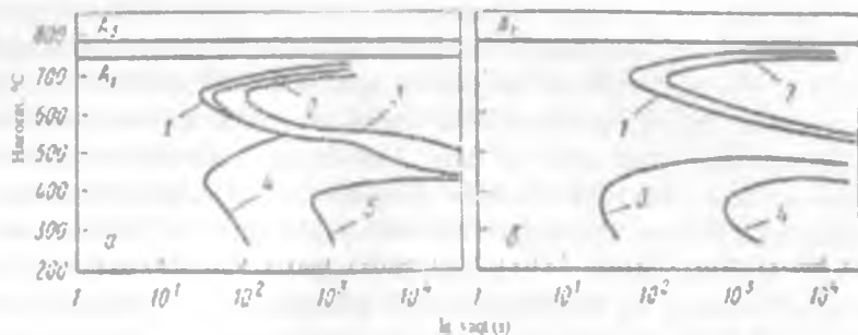
5.9-rasm. Perlitli va beynitli o'zgarishlardagi C – egri chiziq bilan ajralib turadigan legirlangan po'latlarda austenitning izotermik parchalanish diqshrammasi (Roze va Peter)
