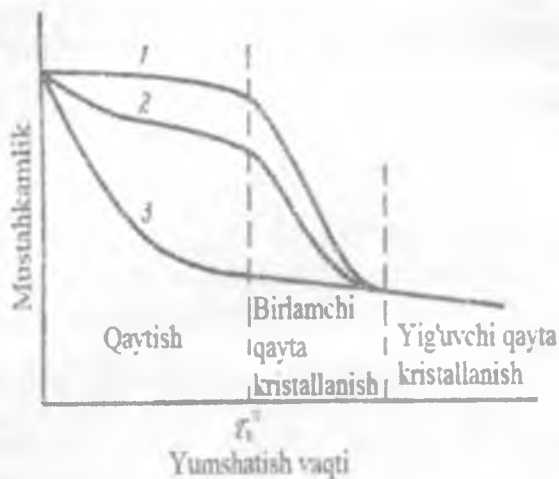
3.5 – rasm. Doimiy temperaturada puxtalangan metallni mustahkamlik xossalarini yumshatishni kechish vaqti davomiyligini oshishi bilan.
