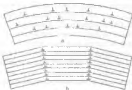
3.3 - rasm. Poligonizatsiyalash sxemasi:
