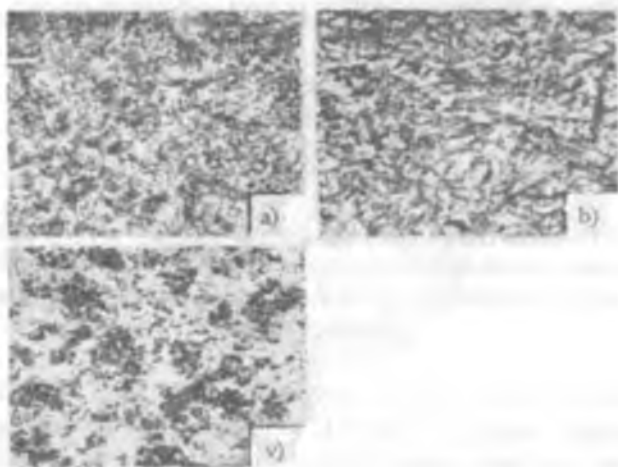
10.15-rasm. SHX15 markali podshipnikli po'latning mikrostrukturasi: a – normal holatdagi toblashdan so'ng – bu yerda martensit kristallari va karbidlar berkingan holatida; b – toblushdan so'ng o'ta qizdirishdan keyin – kata o'lchamli martensit va karbidlar; v – toblashdan so'ng oxirigacha qizdirilmagan holatda (martensit, troostit va karbid; x500.
