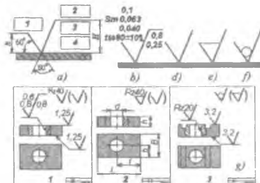
2.29-rasm. Sirt g'adir-budirligining belgilash strukturasi.
