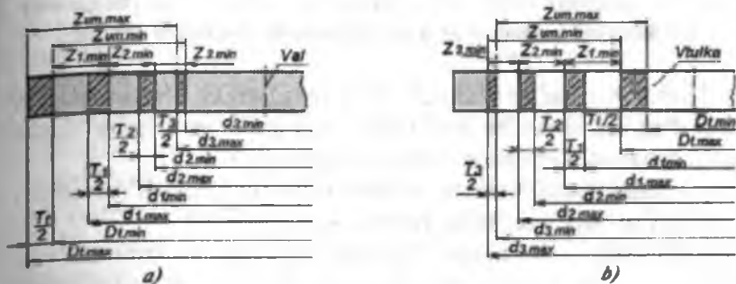
7.5 -rasm. Sozlangan dastgohlarda ishlashda texnologik o'tuvlar bo'yicha a—val va b—vtulka tanavori oraliq qattalari maydonlarining va chegaraviy o'lchamlarining sxemasi.
