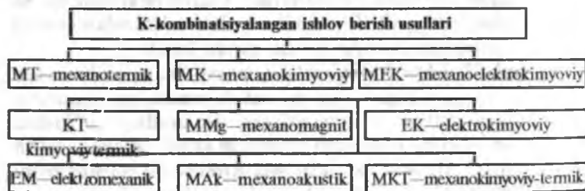
4.2-rasm. Kombinatsiyalashgan ishlov berish usullarining tasnifi.
