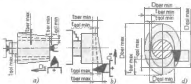
2.16-rasm. Elastik deformatsiyalanishdan xatoliklarni hisoblash sxemasi: a—ko'nussimon; b—notekis yon sirt; d—ovalsimon ko'ndalang kesim.
