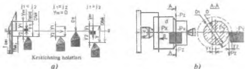
2.14-rasm. Texnologik tizimning elastik deformatsiyalarini aniqlash sxemasi:
