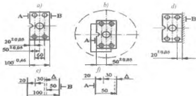
3.16-rasm. Yo'nish va parrmalashda bazalar doimiyluk tamoyilini qo'llash.
