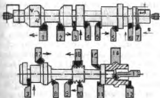
5.8-rasm. Turli keskichlari bilan tashqi va ichki silindr sirtlarga ishlov berish sxemalari: 1, 2, 7—o'tuvchi o'ng va chap keskichlar; 3—kesuvchi (ariqcha o'yuvchi) keskich; 4, 5—to'g'ri o'ng va chap keskich; 6, 14—fasonli keskich; 8, 9, 11, 12—radiusli gatel, faska yo'nuvchi o'ng va chap keskichlar; 10, 16—rezba yo'nuvchi keskichlar; 15, 17—egilgan to'g'ri va o'tuvchi chap keskichlar.
