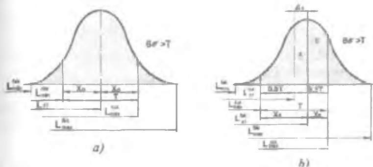
2.10-rasm. Taqsimot maydoni qo'yim maydoniga nisbatan (a) simmetrik va (b) nosimmetrik joylashishida ishga yaroqsizlik bo'lishi ehtimolliigi soni.
