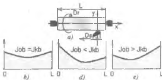
2.17-rasm Tanavorlarni yo'aish sxemasi: (a) va to'g'rilik dastgohi elementlarining bikrliklarining turli nisbatlaridagi elastik defomatsiyalanish grafiklari (b, d, e)
