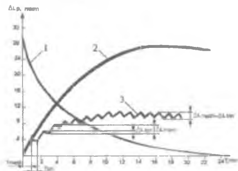
2.22-rasm. Keskich tanaffus bilan ishlashini uning issiqlik deformatsiyasiga ta'siri:
