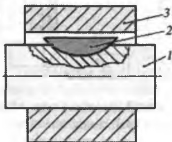
12.9-rasm. Valga segmentli shponka oʻtqazish amali.
