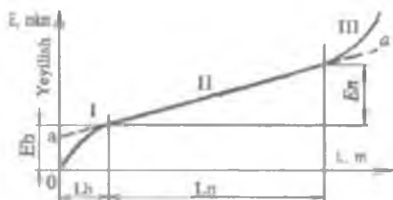
2.13-rasm. Yeyilishning kesish yo'liga bog'liqlik grafiqi.
