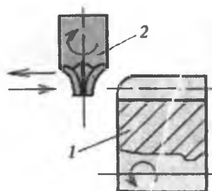
5.19-rasm. Tishlarni yumaloqlash sxemasi:
