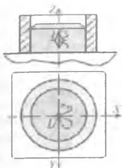
3.11-rasm. Qo'shaloq yo'naltiruvchi baza sxemasi.
