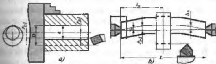
7.3-rasm. Ishlanuvchi sirtlar fazoviy og'ishlarini qatlamlarga ta'sirini ko'rsatuvchi sxema:
