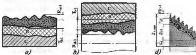
7.2-rasm. Tanavorning sirtqi va ichki qatlamlar sxemalari:
