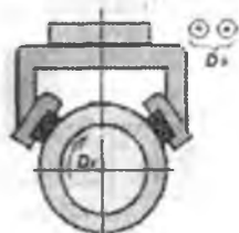
5.13-rasm. Supperfinshlash sxemasi.
