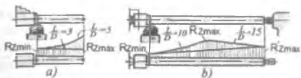
2.31-rasm. Texnologik tizim bikirligining sirt g'adir-budirlikiga ta'siri.
