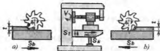
5.4-rasm. Gorizont-al-frezalash dastgohida silindrik frezalar bilan ishlov berish sxemalari: a—surishga qarshi frezalash; b—surish yo'nalishi bo'yicha frezalash.
