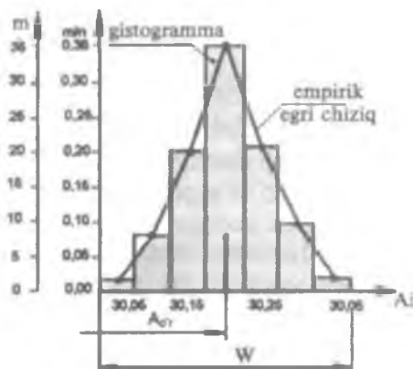
2.4- rasm. O'lchangan detallar o'lchamlarining taqsimoti.
