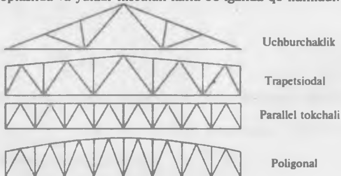
8.1-rasm. Fermalar.
