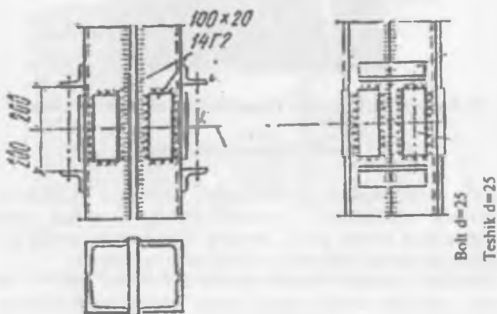
17.10- rasm. Ustunlarni bir-biriga biriktirilishi.
