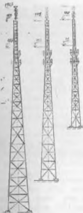
19.1-rasm. To'rtqirrali teleminoraning tipli sxemasi.
