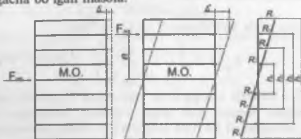
12.6-rasm. Fazoviy bikirli koeffitsiyentni aniqlash uchun chizma.
