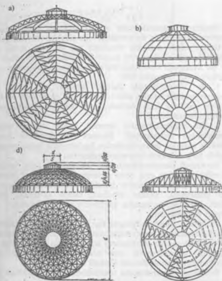
15.1-rasm. Gumbazlar:
