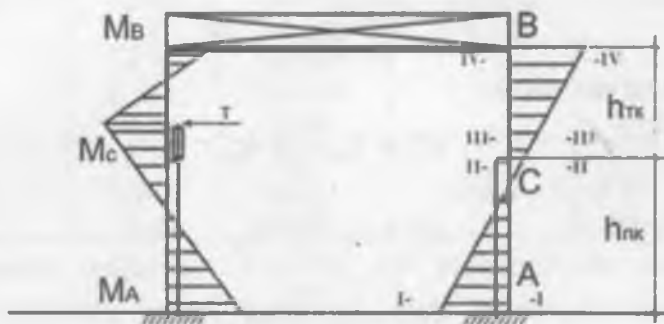
12.7-rasm. Gorizontaal yukdan hosil bo'ladigan eguvchi moment epyurasi.
