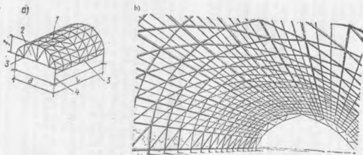
15.5-rasm. Bir to'rtli qobiqlar. 1) silindrik qobiq; 2) yon tomondagi diafragma; 3) bog'lovchi element; 4) ustun.
