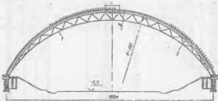
14.9-rasm. Pastki belbog'i zo'riqtirilgan arkalar:
