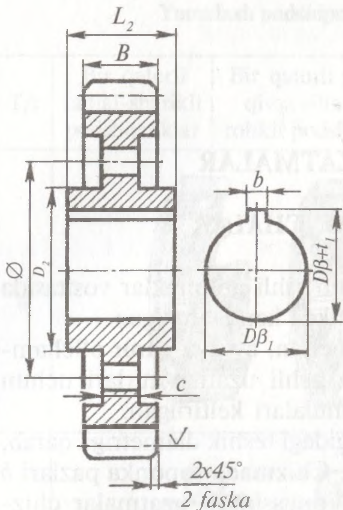
166-shakl. Silindrik tishli g'ildirakning konstruktiv o'lchamlari.
