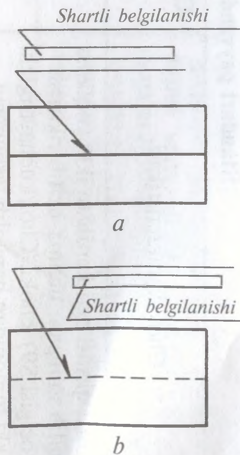
145-shakl. Chok shartli belgilarining qo'yilishi.
