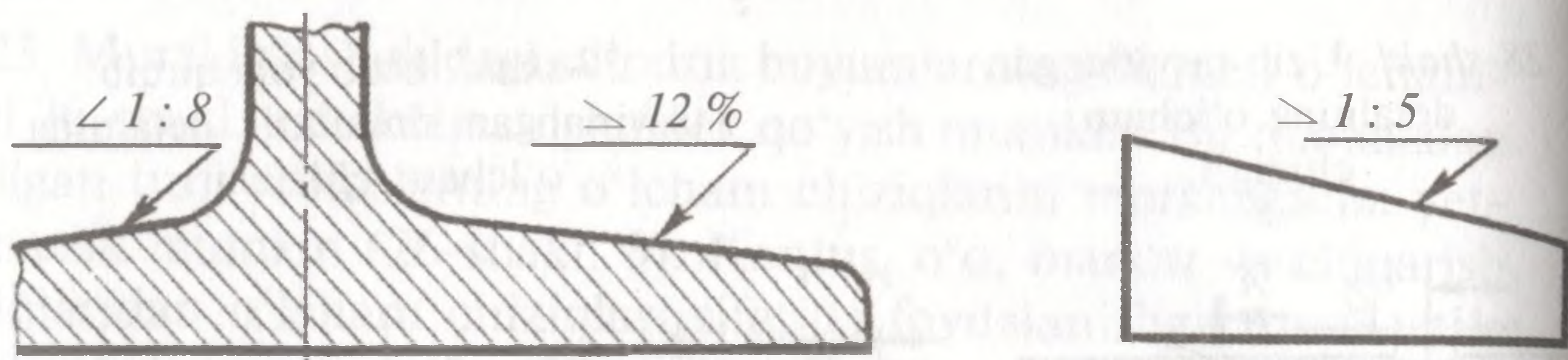
33-shakl. Qiyalikning belgilanishi.
