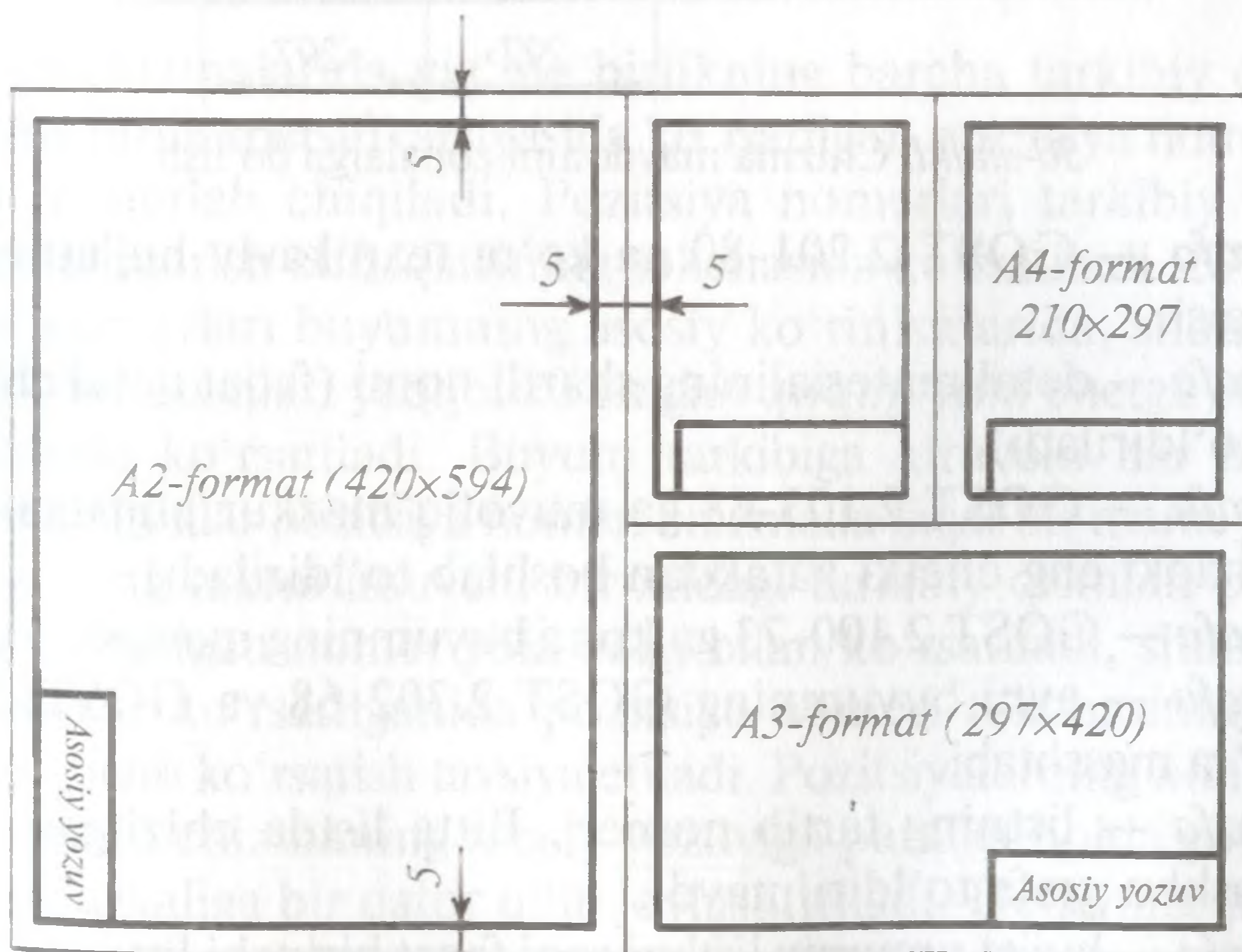
54-shakl. Albom qilib tikiladigan formatlar va asosiy yozuvlarning joylashtirilishi.
