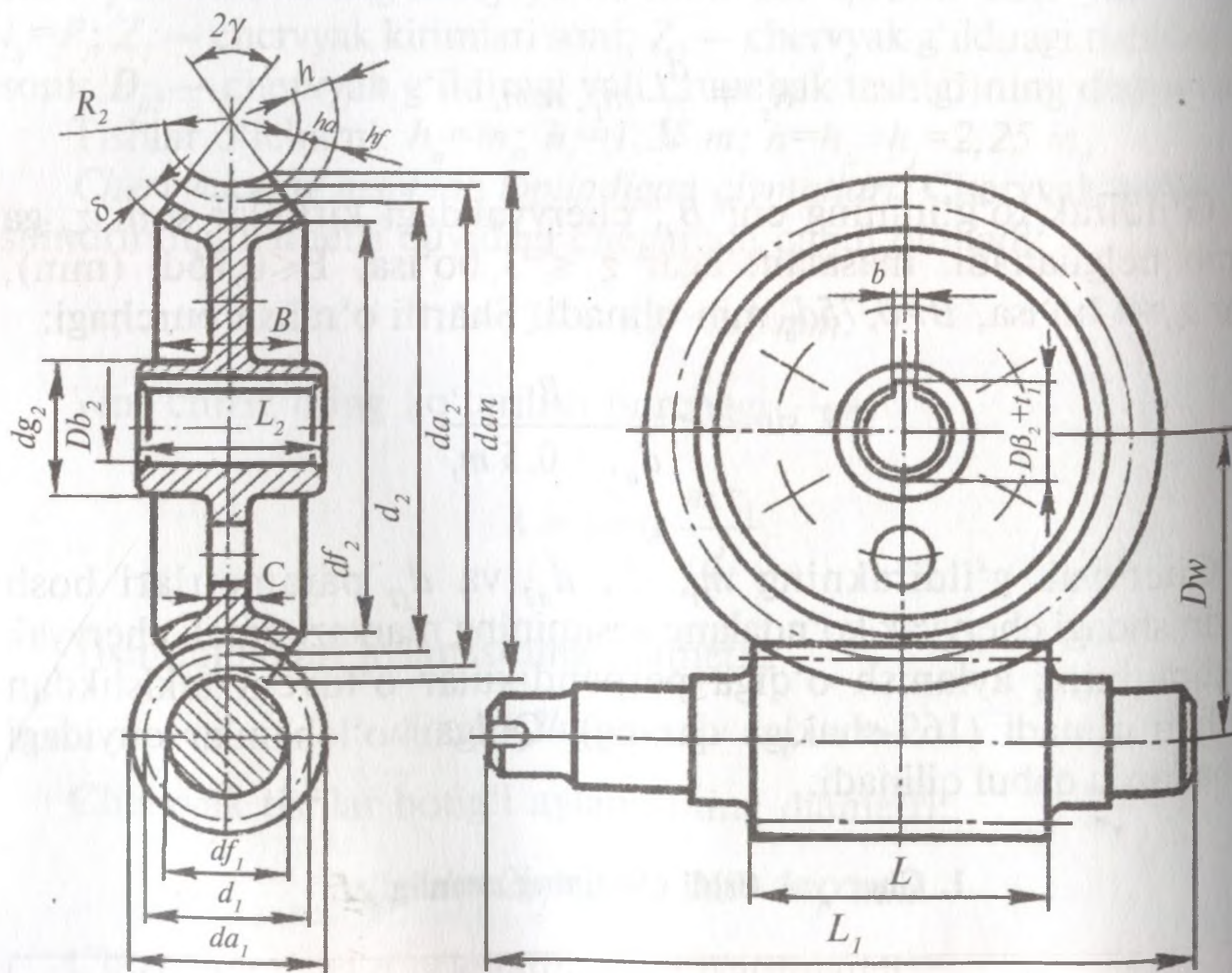
169-shakl. Chervyakli uzatmalar.
