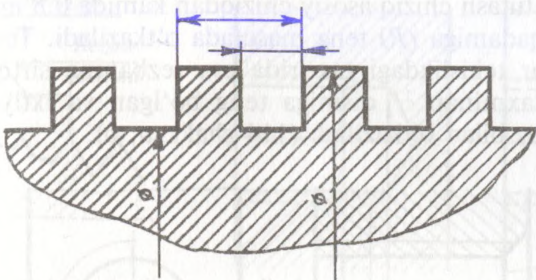
112-shakl. To'g'ri burchakli rezbaning profili.
