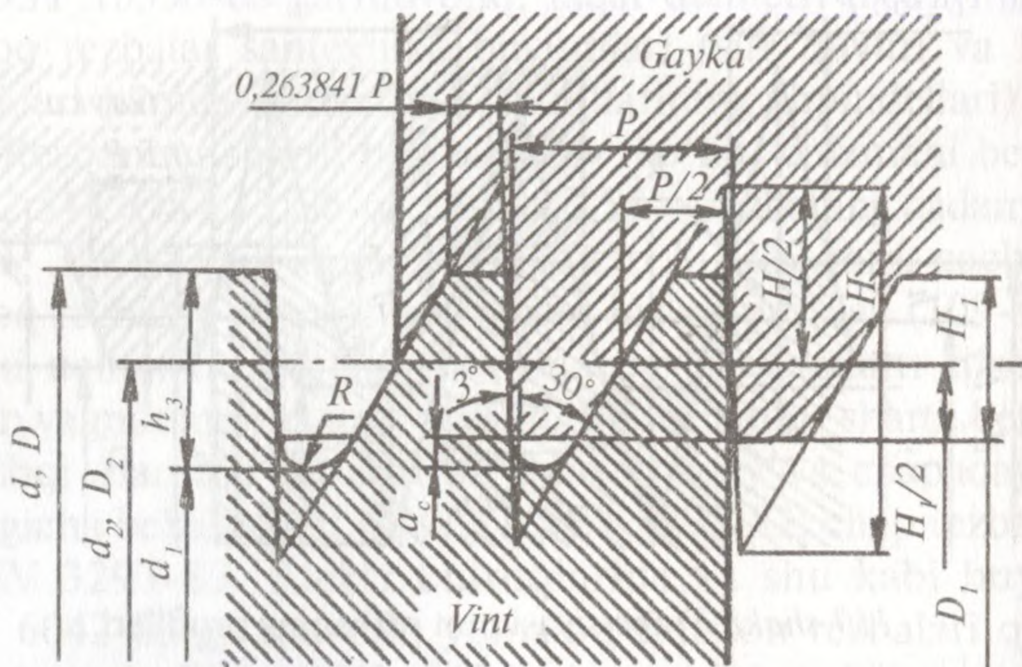
111-shakl. Tirak rezbaning profillari.
