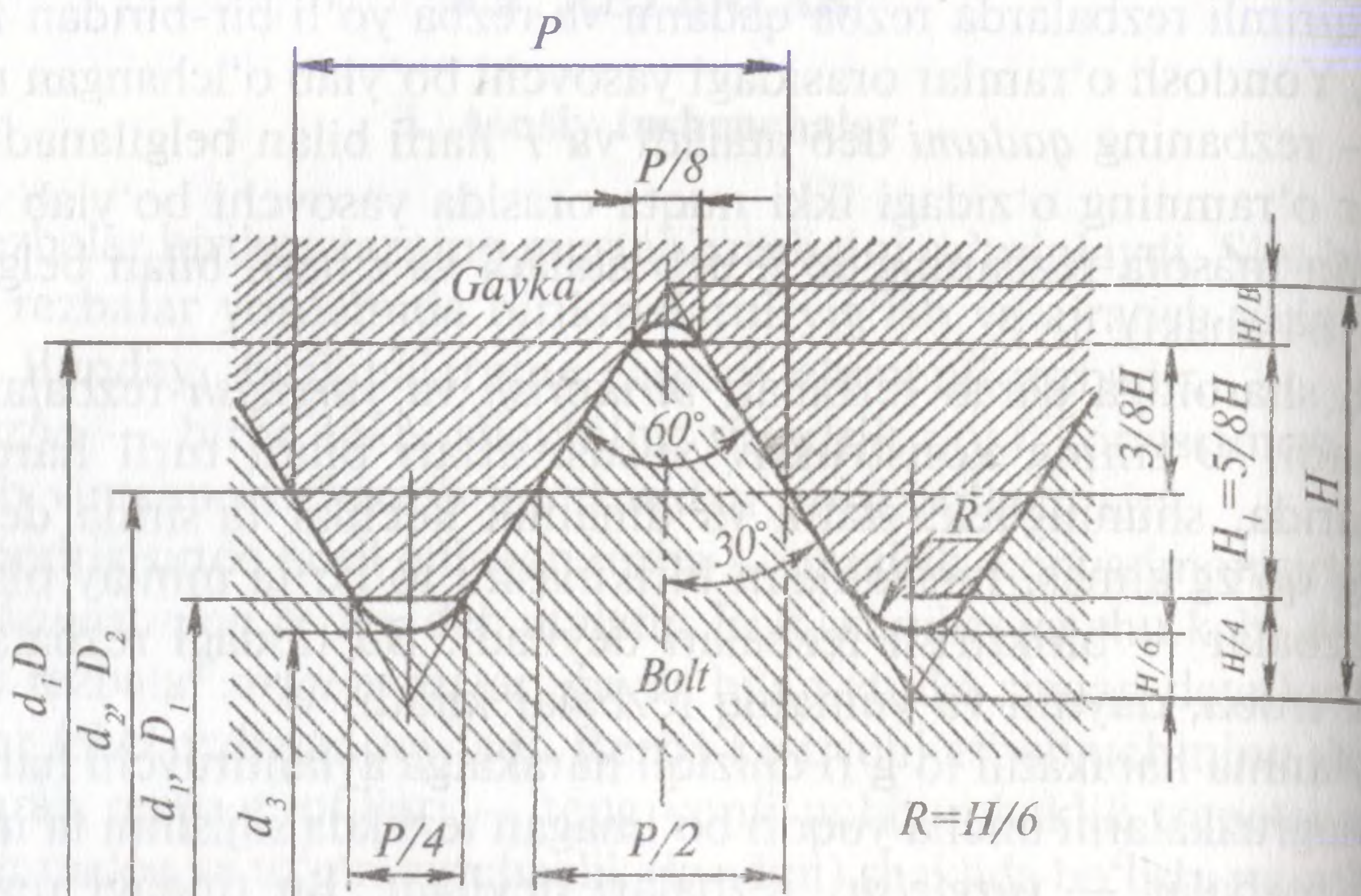
105-shakl. Metrik rezbaning profillari.
