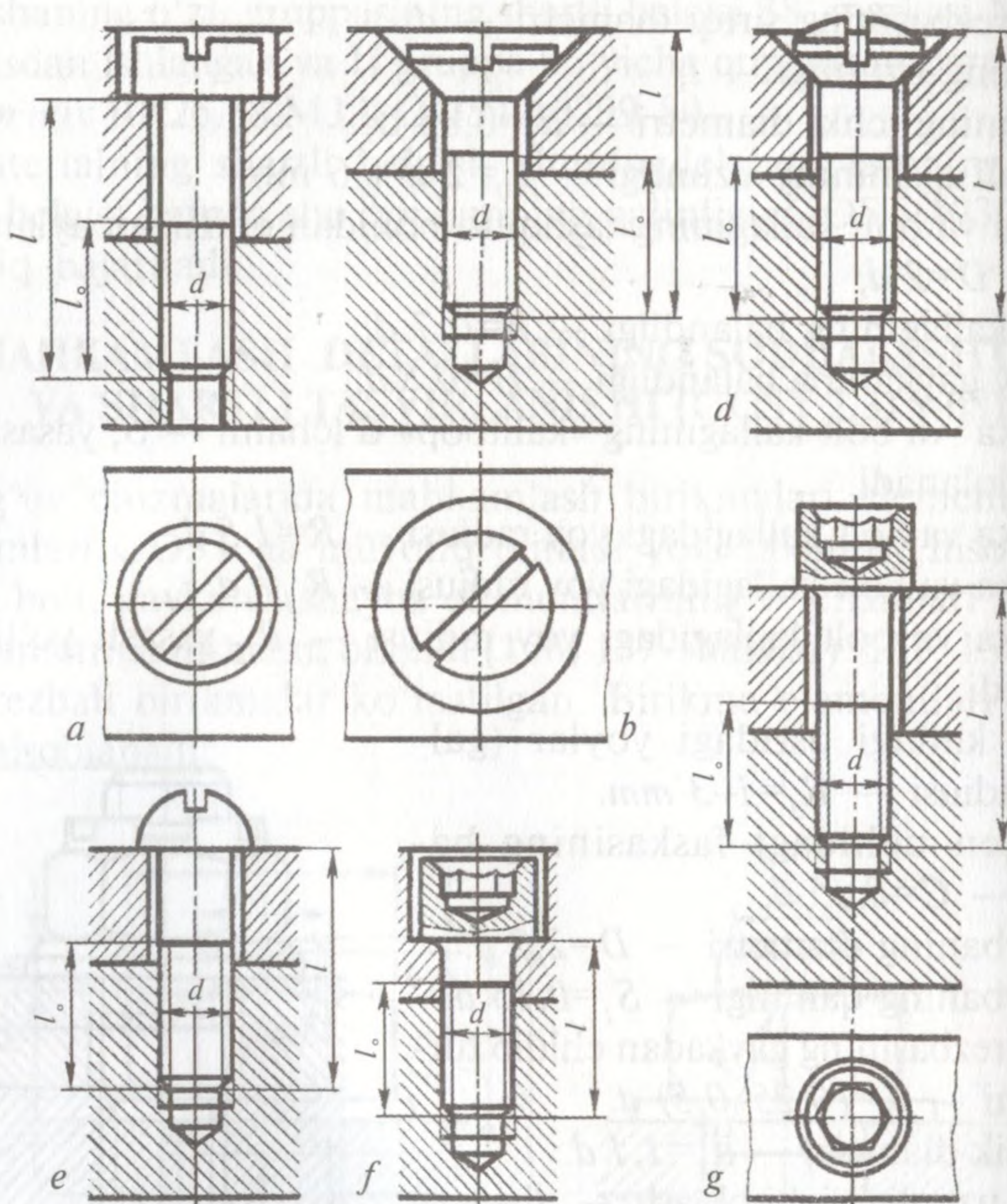
158-shakl. Vintli birikmalar:
