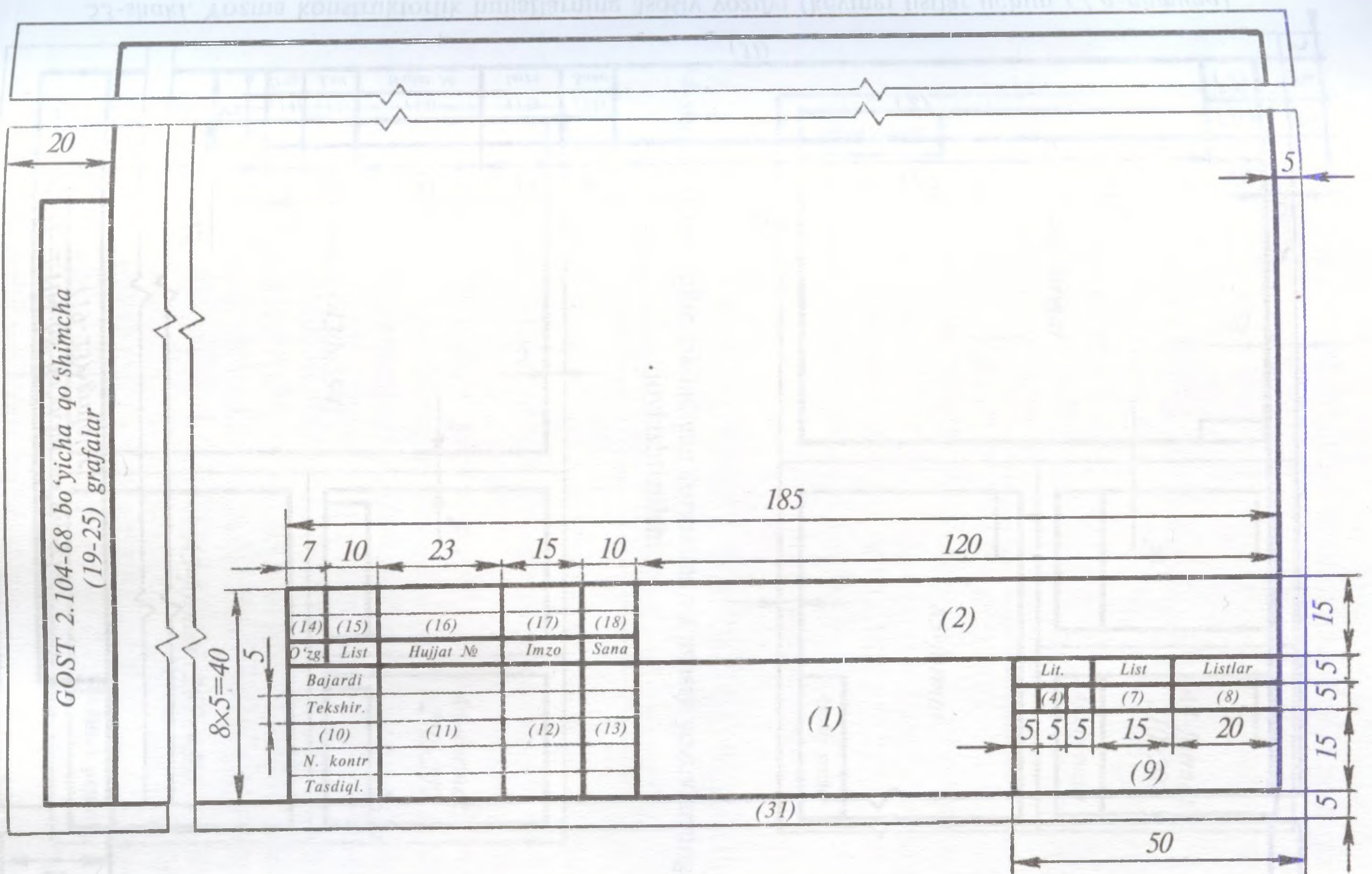
52-shakl. Yozma konstruktorlik hujjatlarning asosiy yozuvi (2-namuna).
