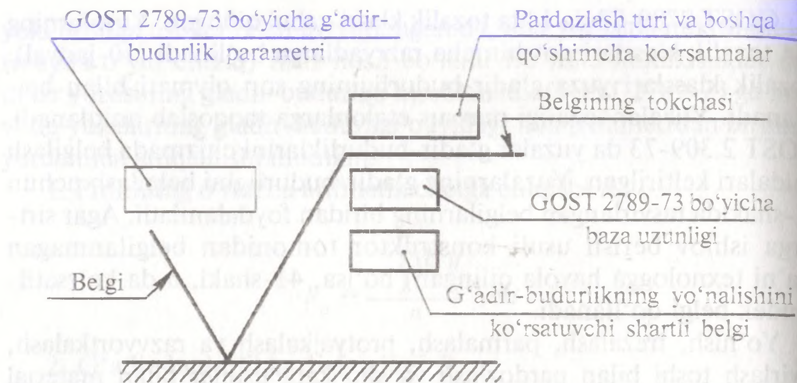
42-shakl. Yuzalar g'adir-budurligini ko'rsatuvchi tokchali belgi.
