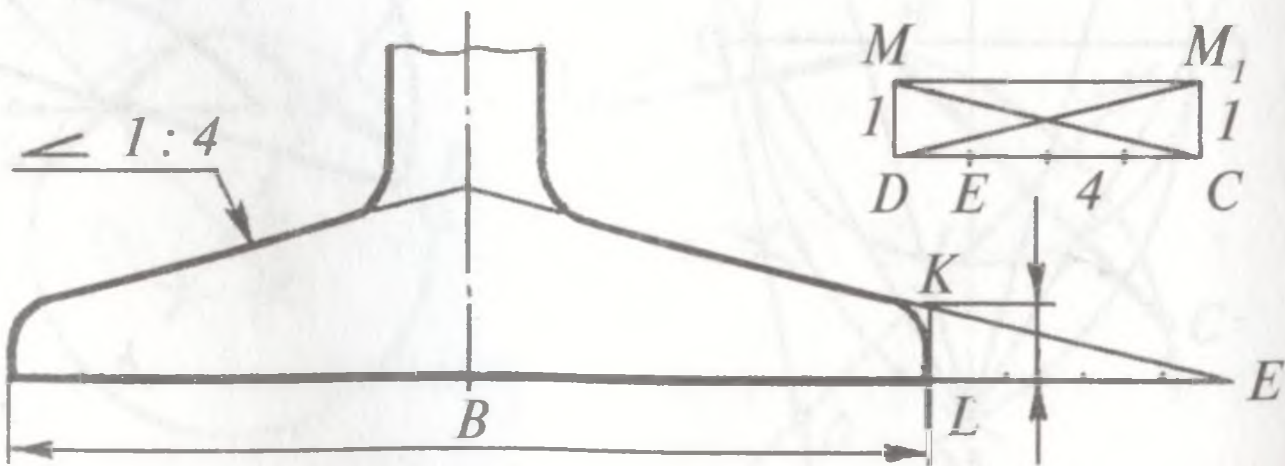
74-shakl. Qiyalik yasash.
