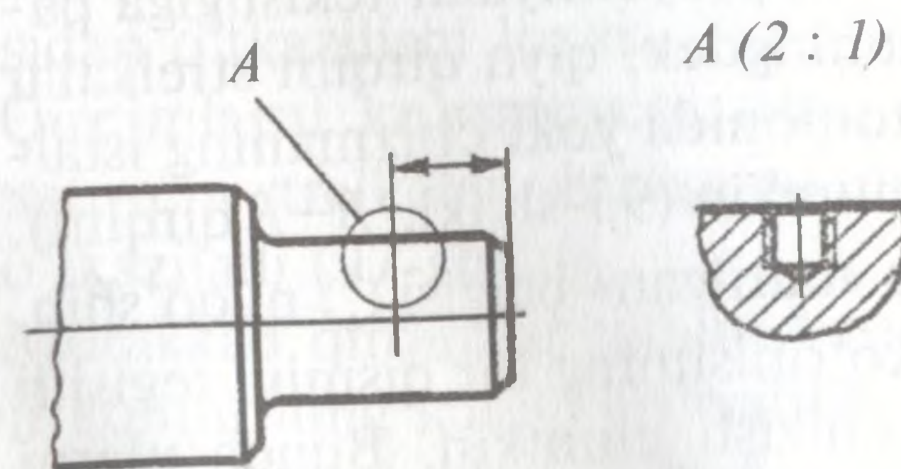
100-shakl. Chetga chiqarish elementining tasvirlanishi.
