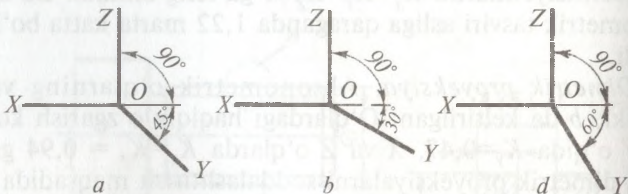
119-shakl. Qiyshiq burchakli frontal izometrik o'qlar vaziyati.
