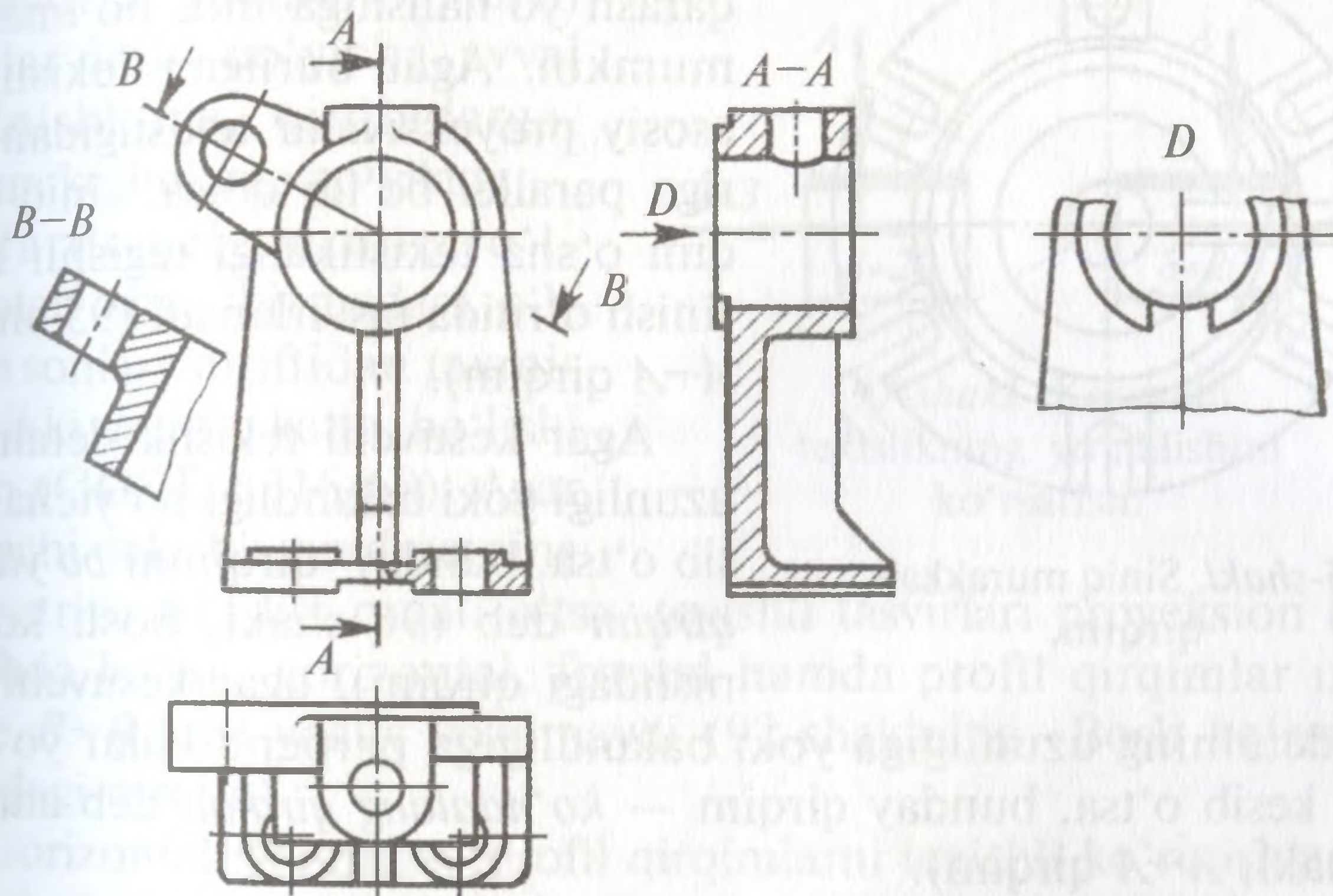
93-shakl. Qiya qirqim va mahalliy ko'rinish.
