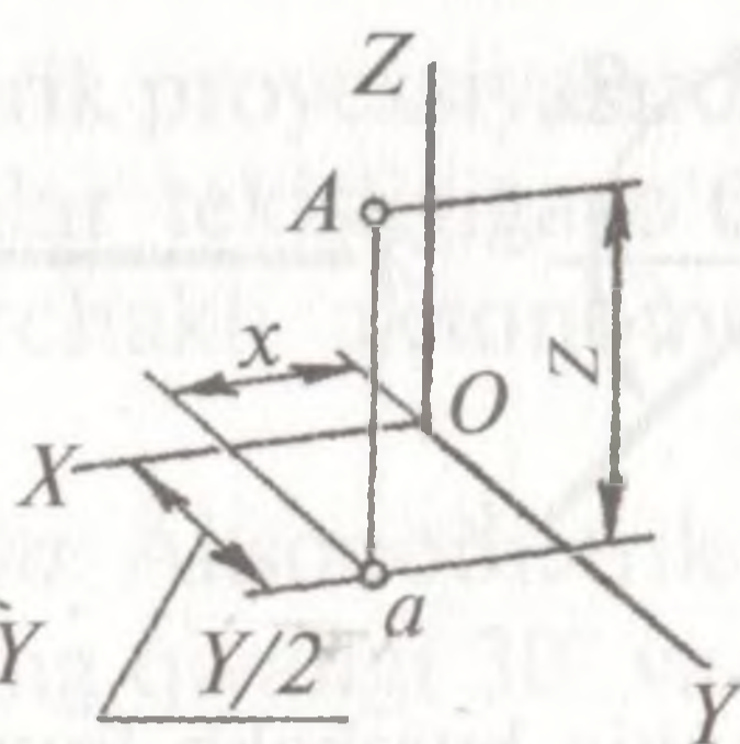
To'g'ri burchakli diametriya
