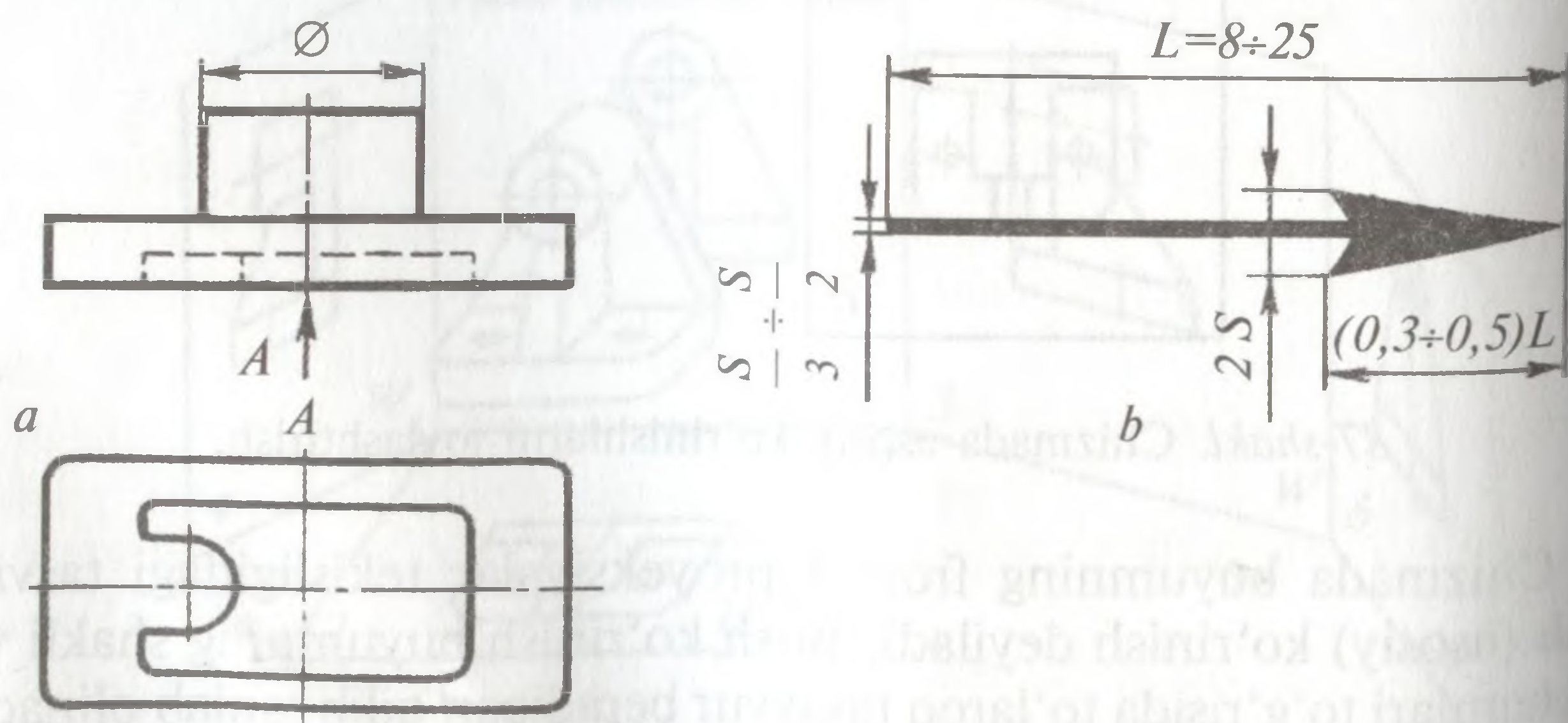
90-shakl. Strelka va strelka bo'yicha ko'rinishning joylashtirilishi.
