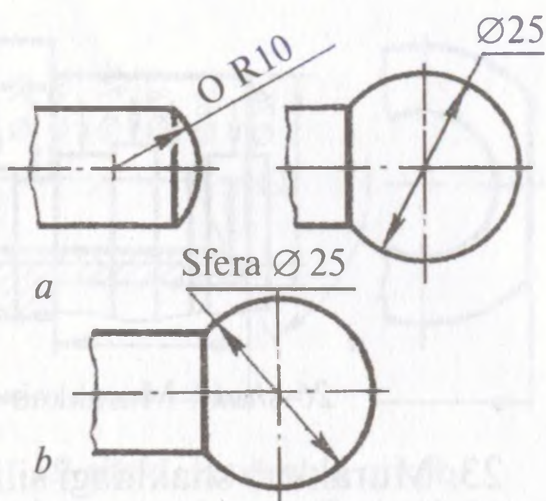
24-shakl. Sferaning o'lchamlarini ko'rsatish.
