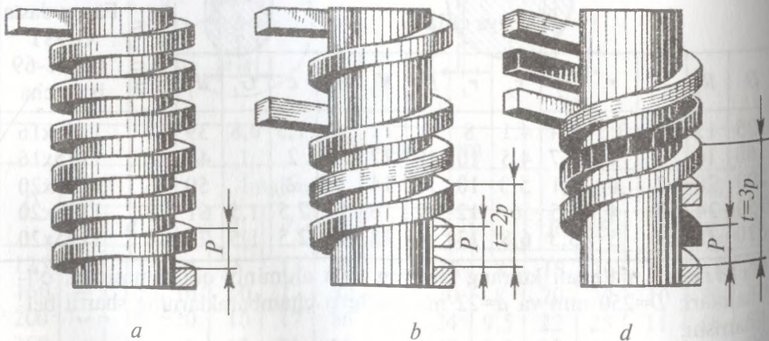
104-shakl. Bir va ko'p kirimli rezbalar.
