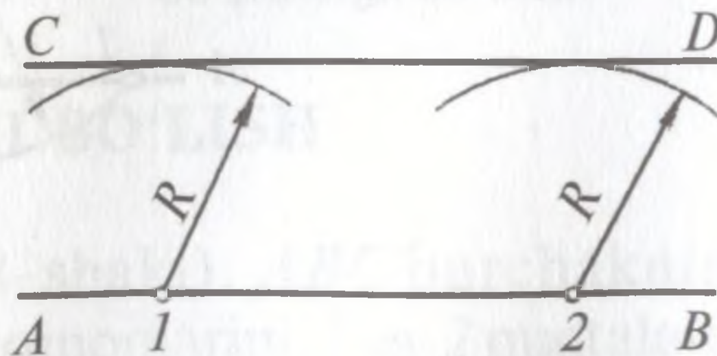
64-shakl. Parallel to'g'ri chiziqlar o'tkazish.
