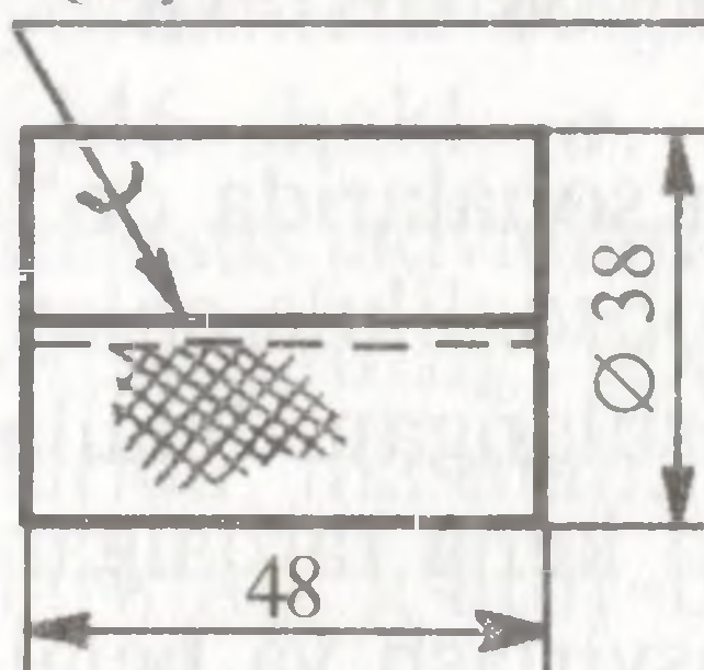
153-shakl. Qalaylangan chokni belgilash.
