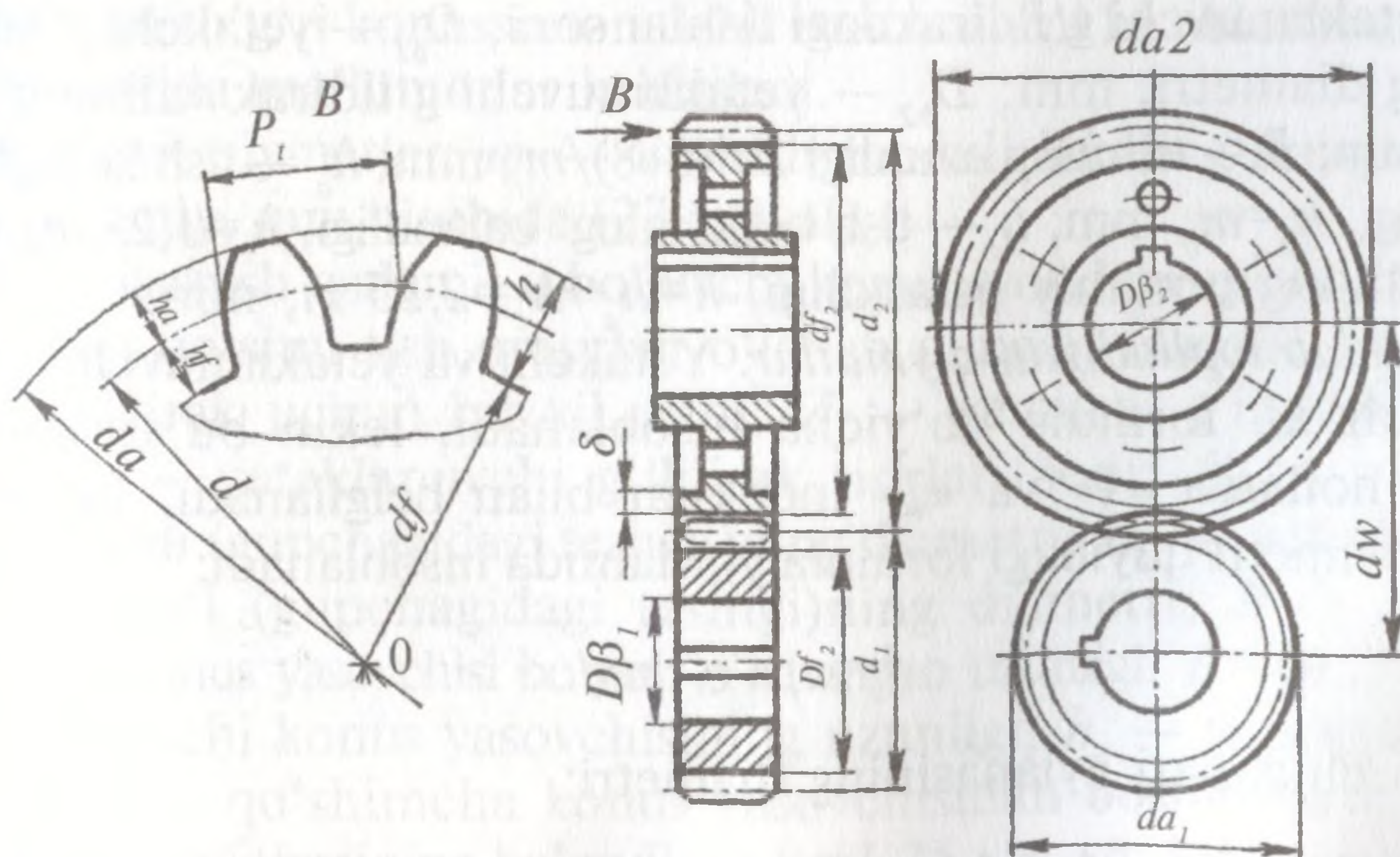
165-shakl. Silindrik tishli uzatmalar.
