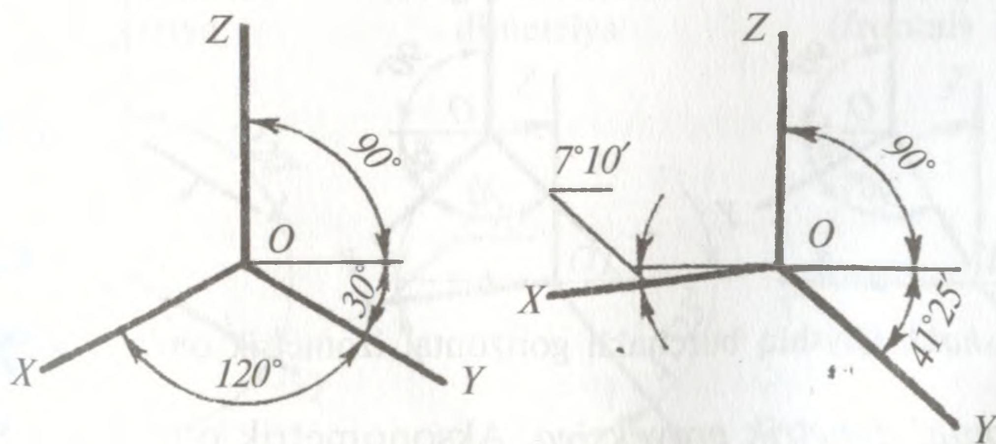
118-shakl. To'g'ri burchakli aksonometrik o'qlar vaziyati.
