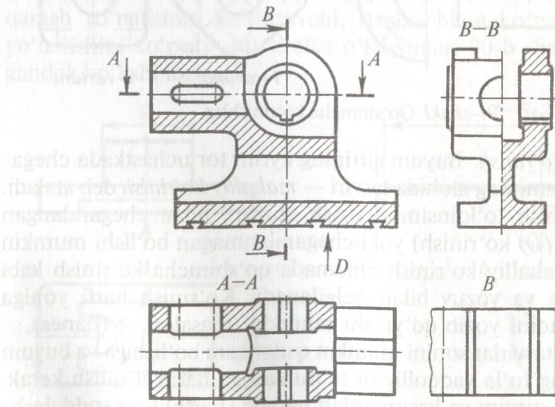
92-shakl. Qirqim va mahalliy ko'rinishlarni tasvirlash.
