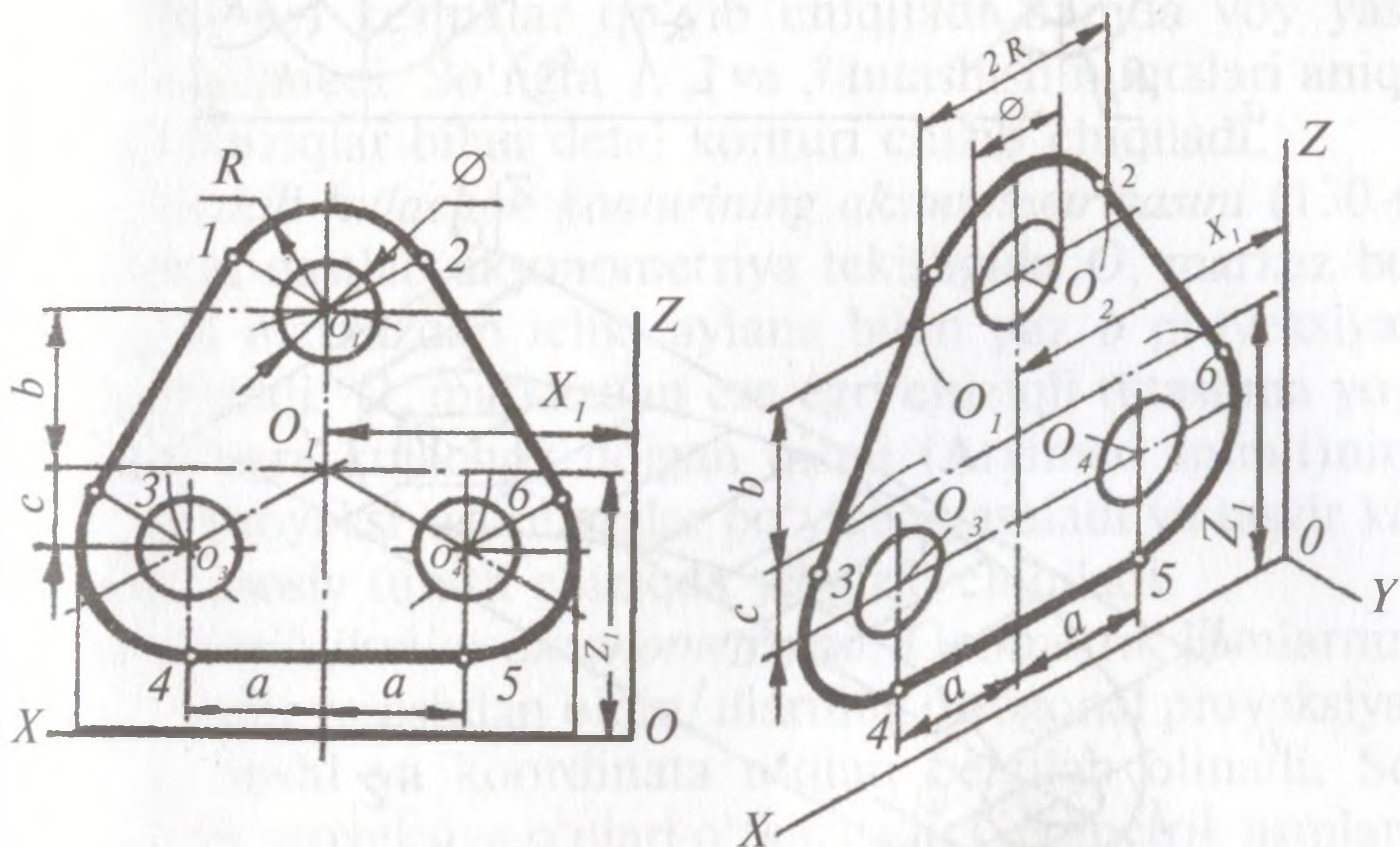
To'g'ri burchakli dimetriya
