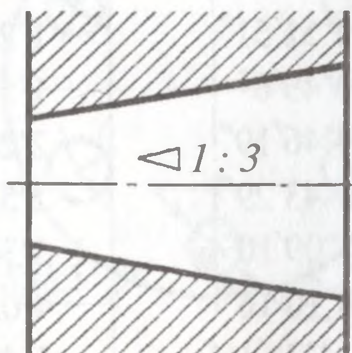
32-shakl. Konuslikning belgilanishi.
