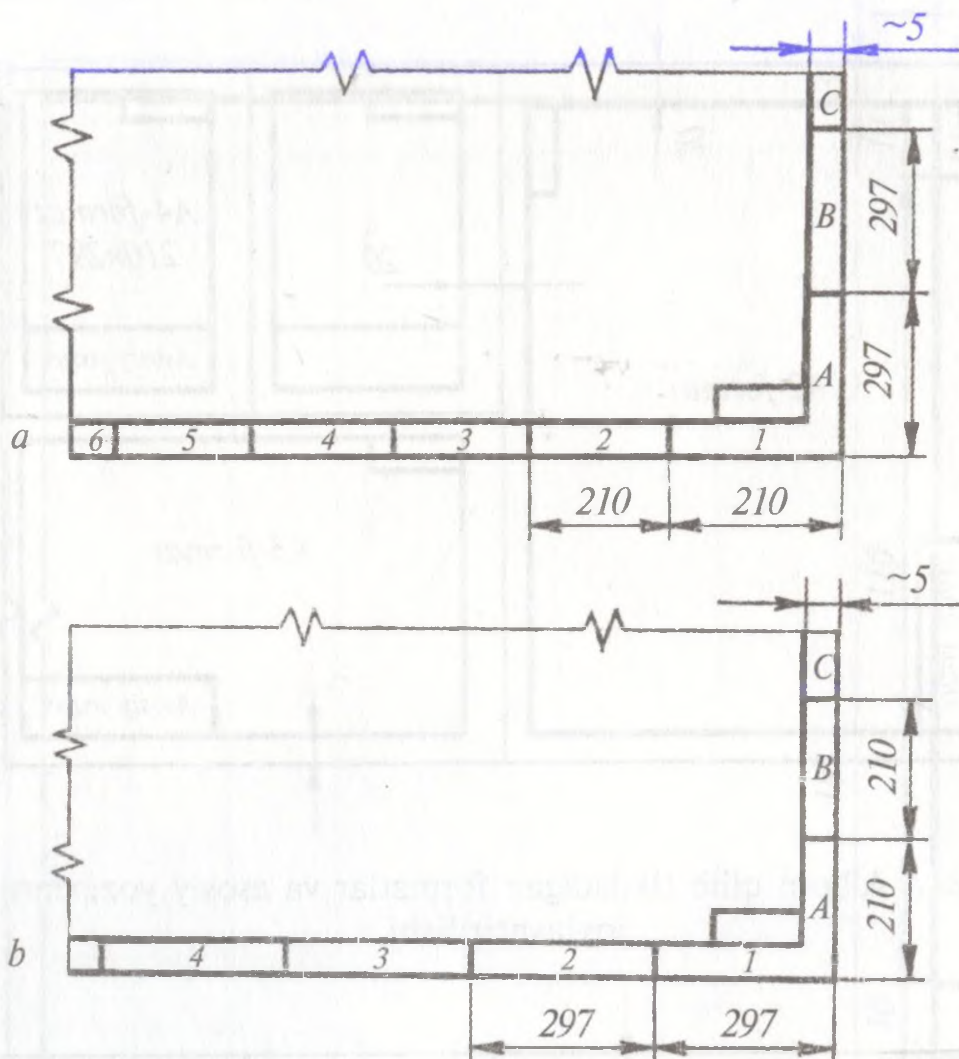
56-shakl. Chizma maydonini zonalarga bo'lish.
