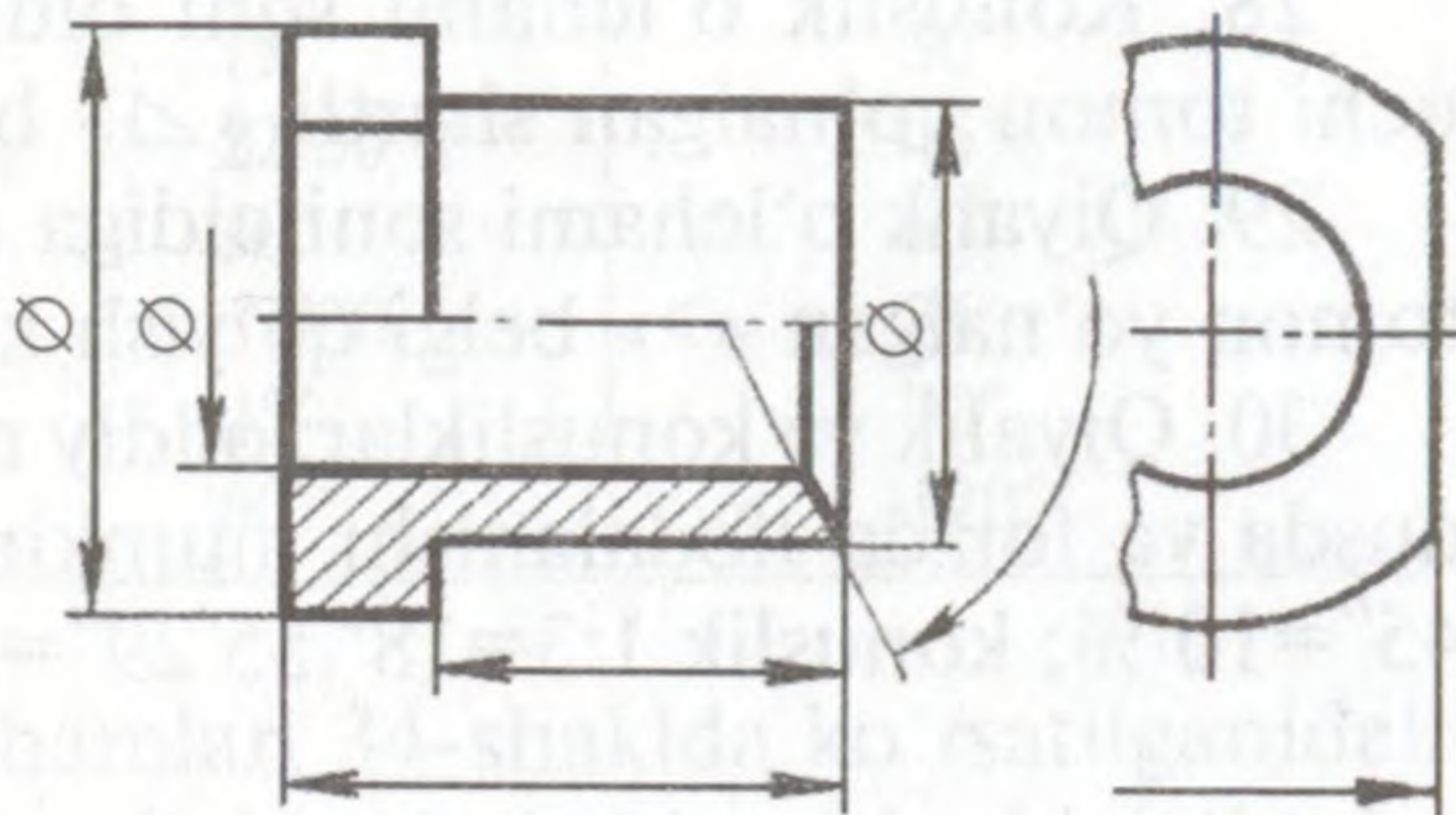
29-shakl. Uzib yoki qirqib tasvirlangan simmetrik detalning o'lcham chiziqlari.
