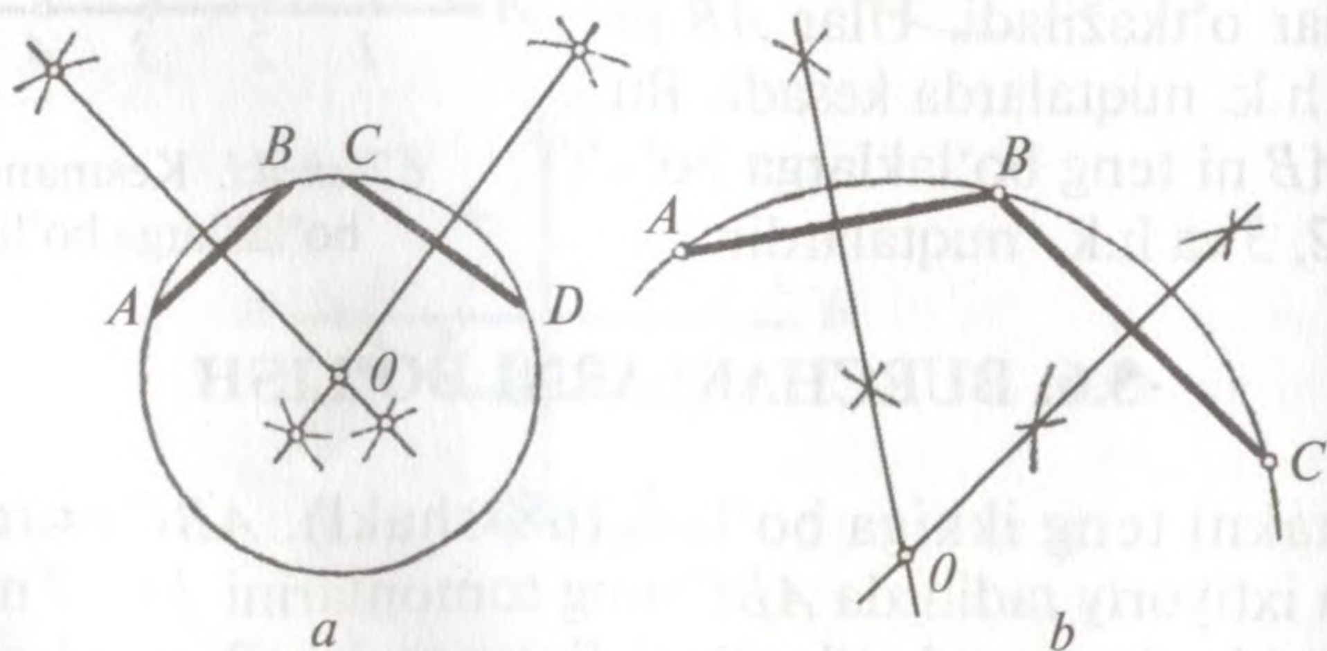
70-shakl. Aylana yoki aylana yoyi markazini aniqlash.
