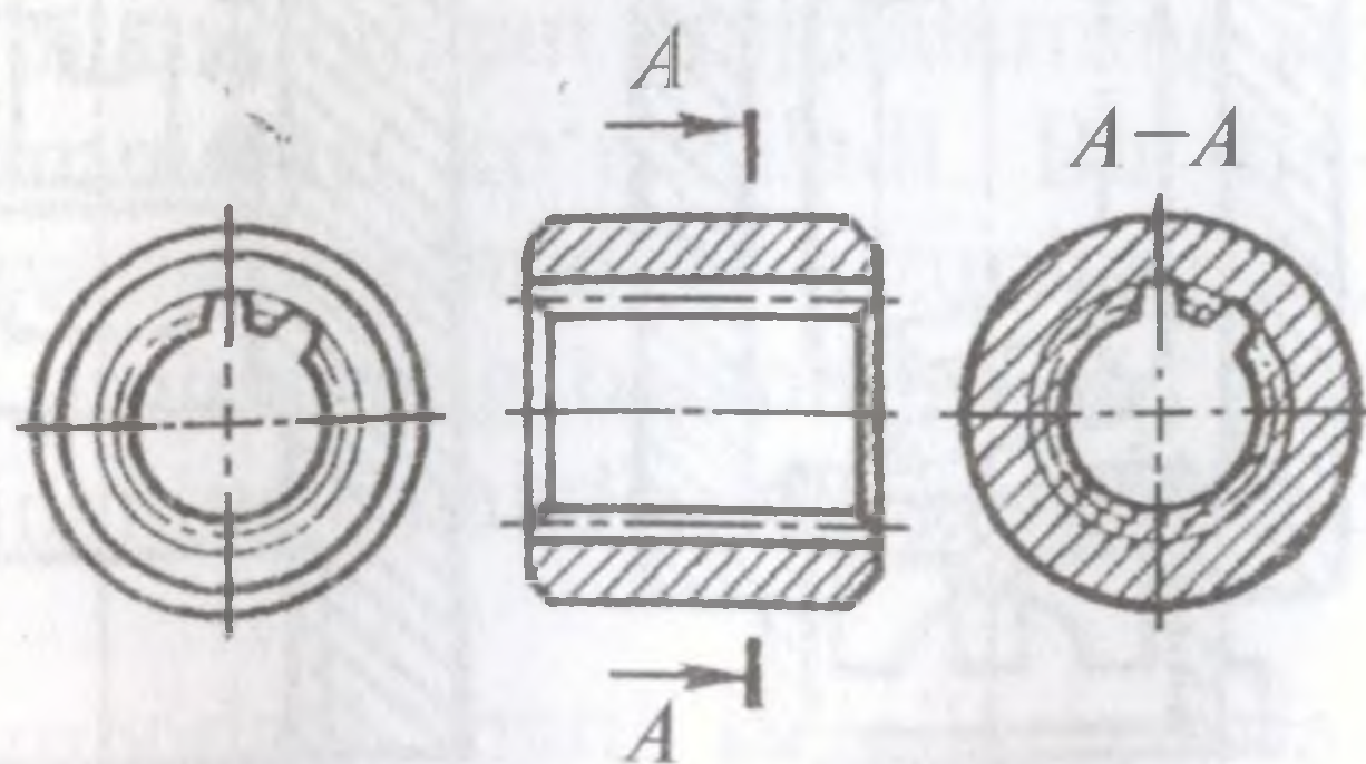
160-shakl. Vtulka qirqimida shlitsalarni tasvirlash.
