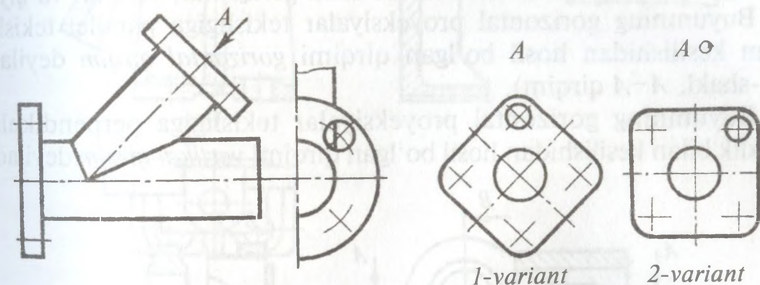
91-shakl. Qo'shimcha ko'rinishlar.
