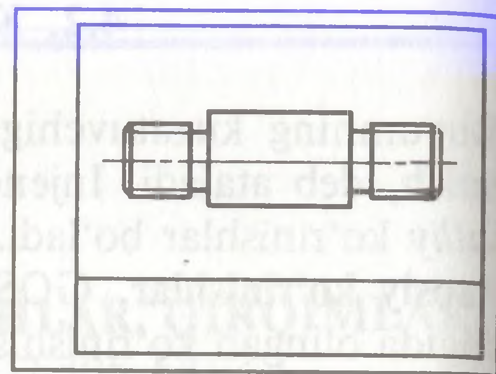
89-shakl. Aylanish sirtlarini chizmada tasvirlash.
