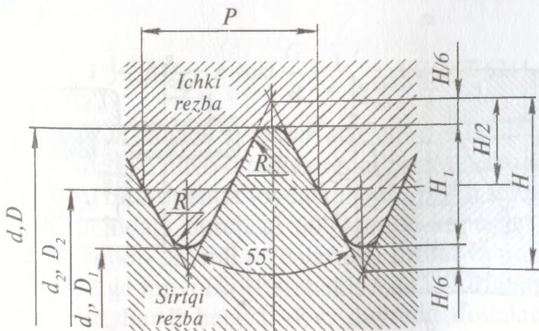
107-shakl. Silindrik truba rezbaning profillari.
