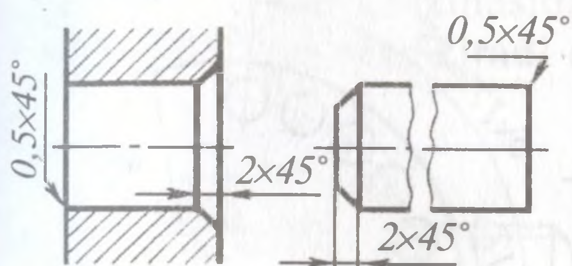
34-shakl. 45° burchakli faskaning belgilanishi.
