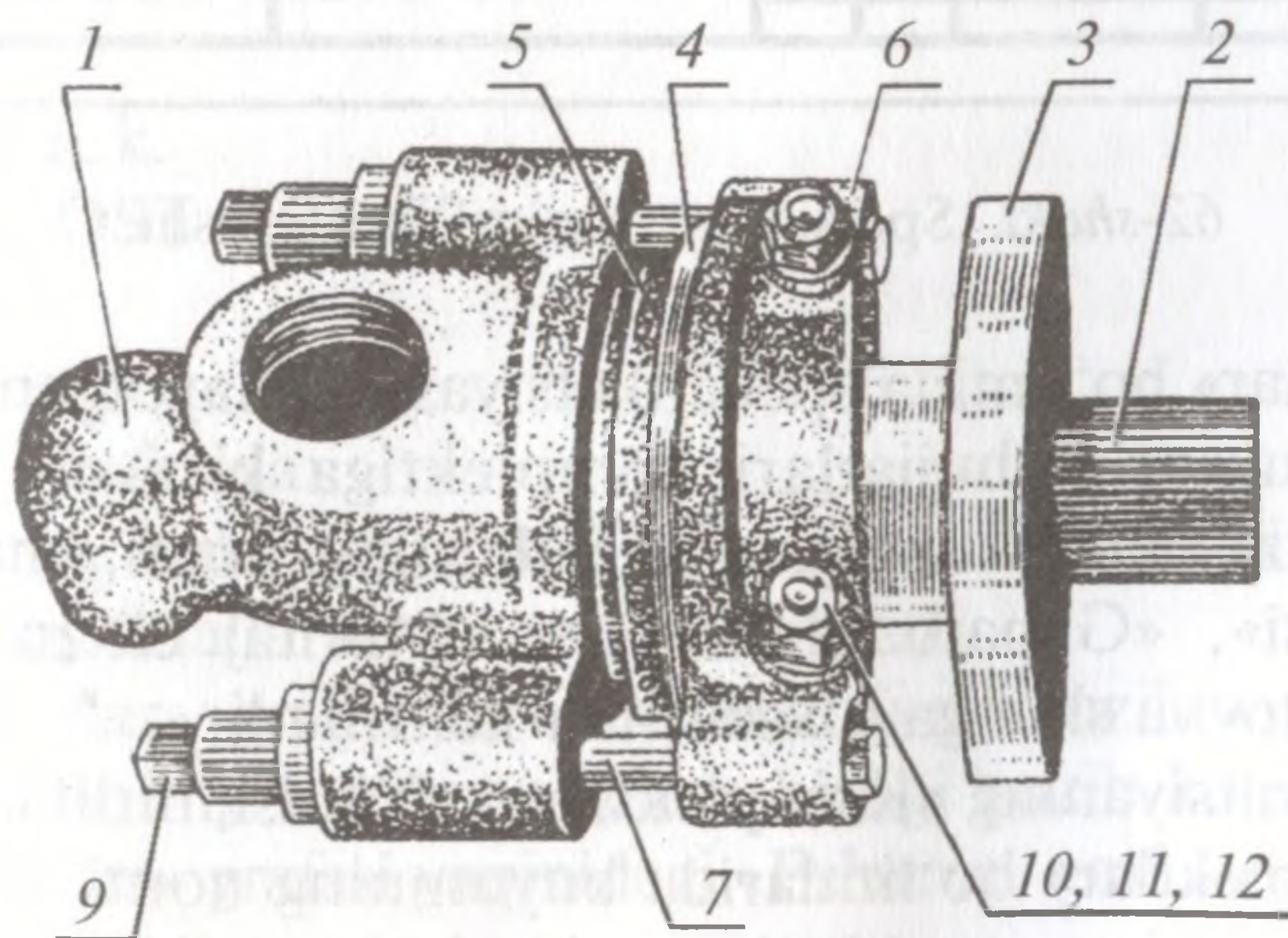
61-shakl. Mufta.
