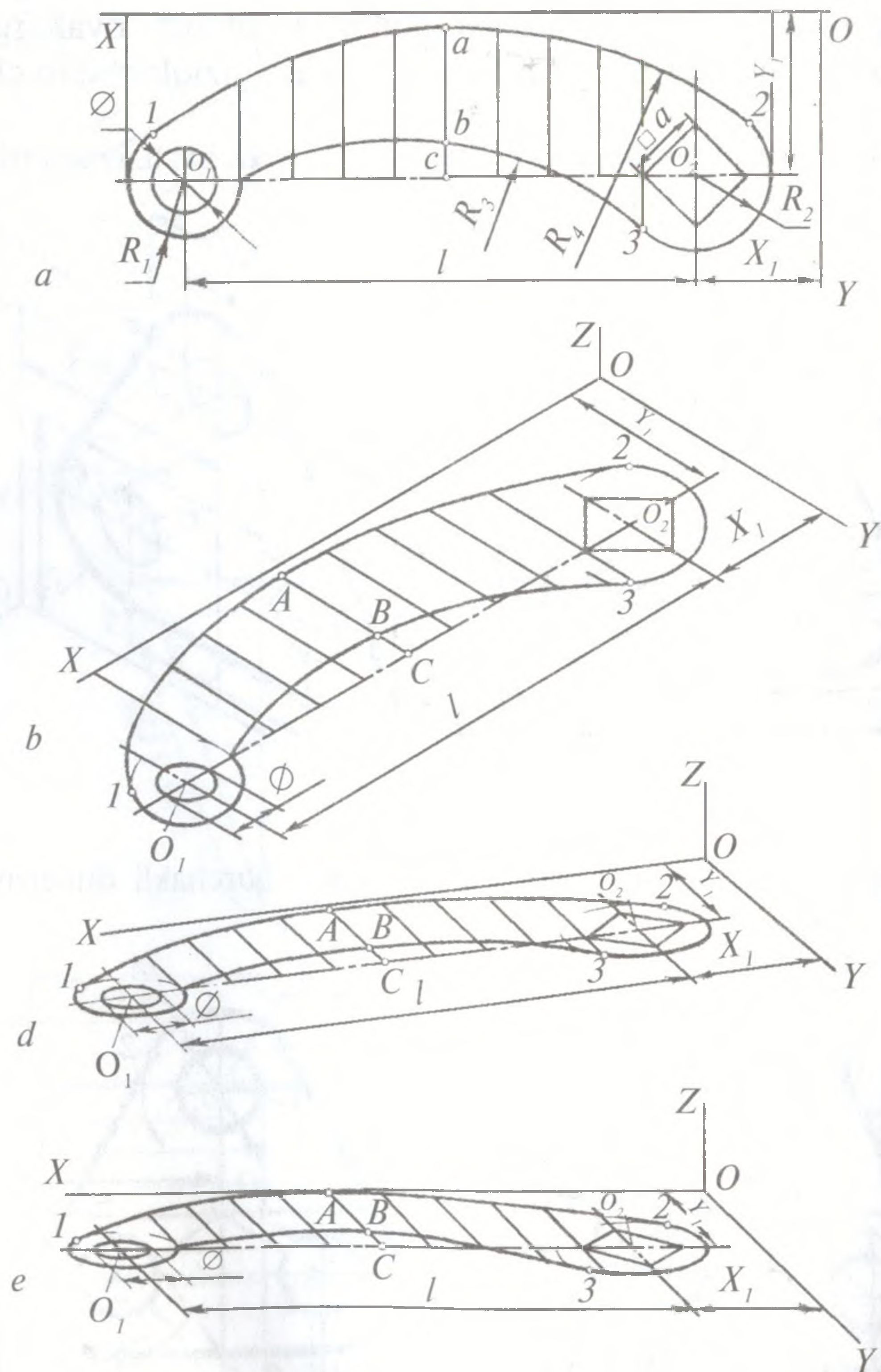
129-shakl. Dasta konturi aksonometriyasini yasash:
