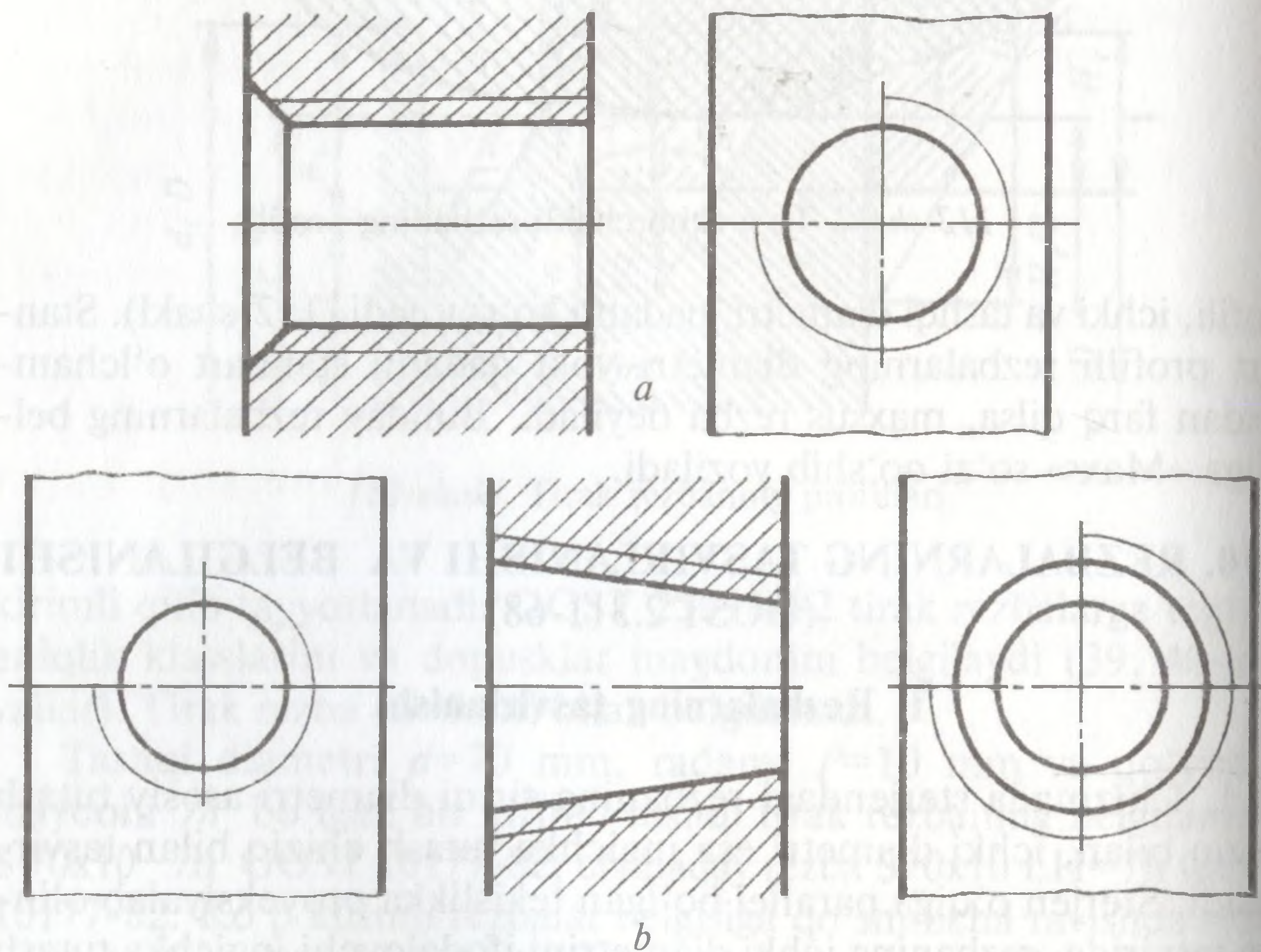
114-shakl. Teshikda rezbaning tasvirlanishi.
