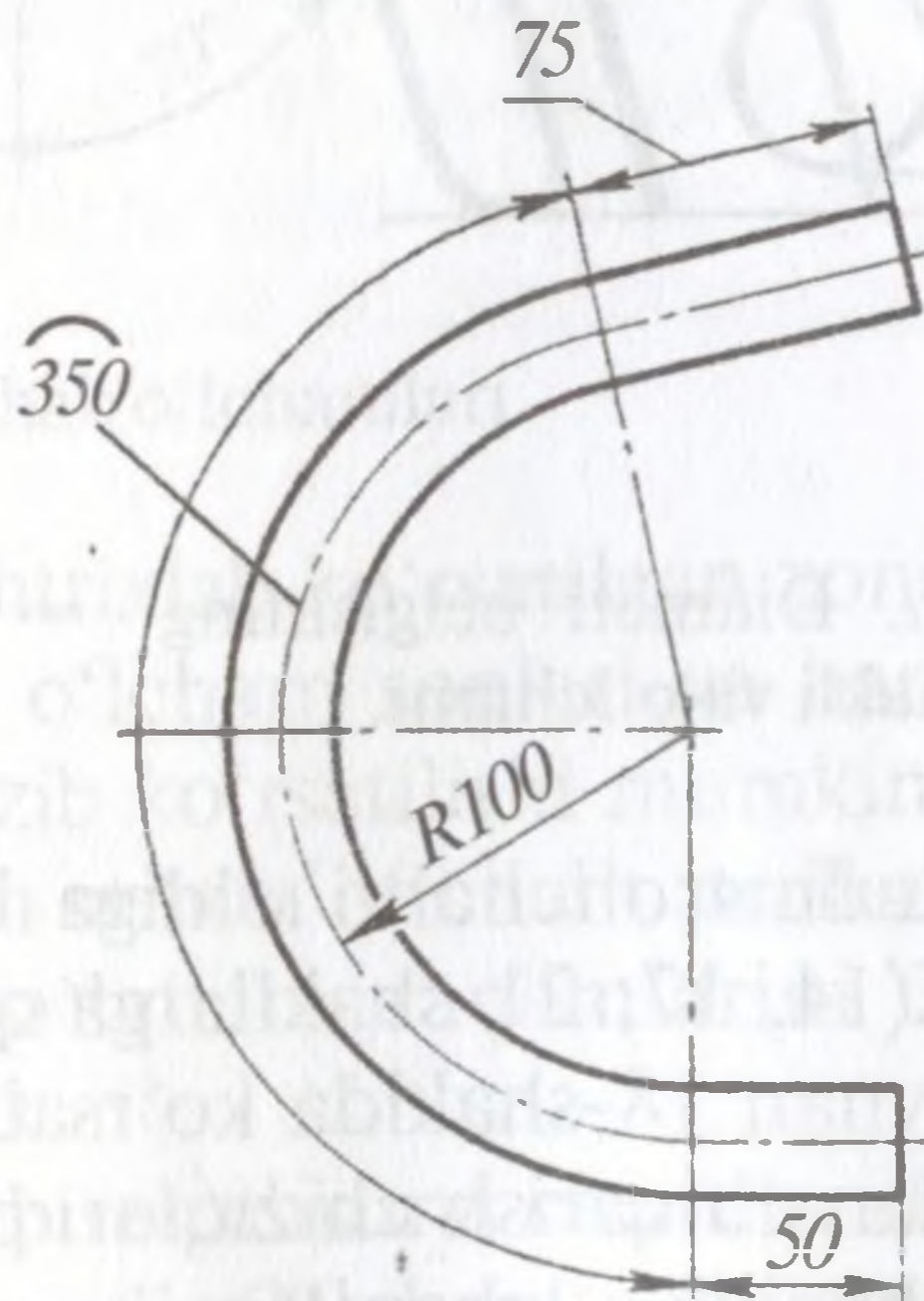
14-shakl. Aylana yoyining o'lchamini qo'yish.
