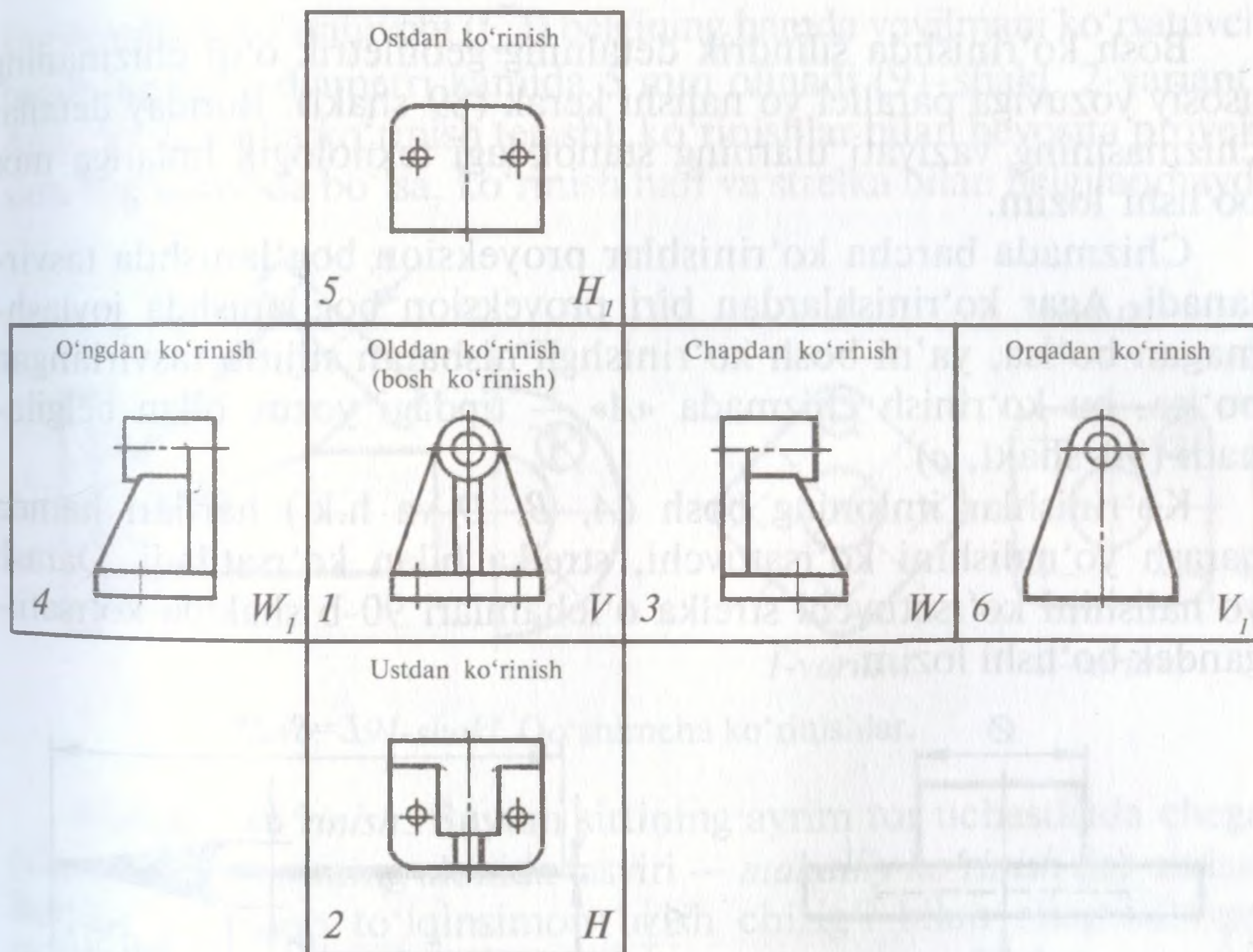
87-shakl. Chizmada asosiy ko'rinishlarni joylashtirish.
