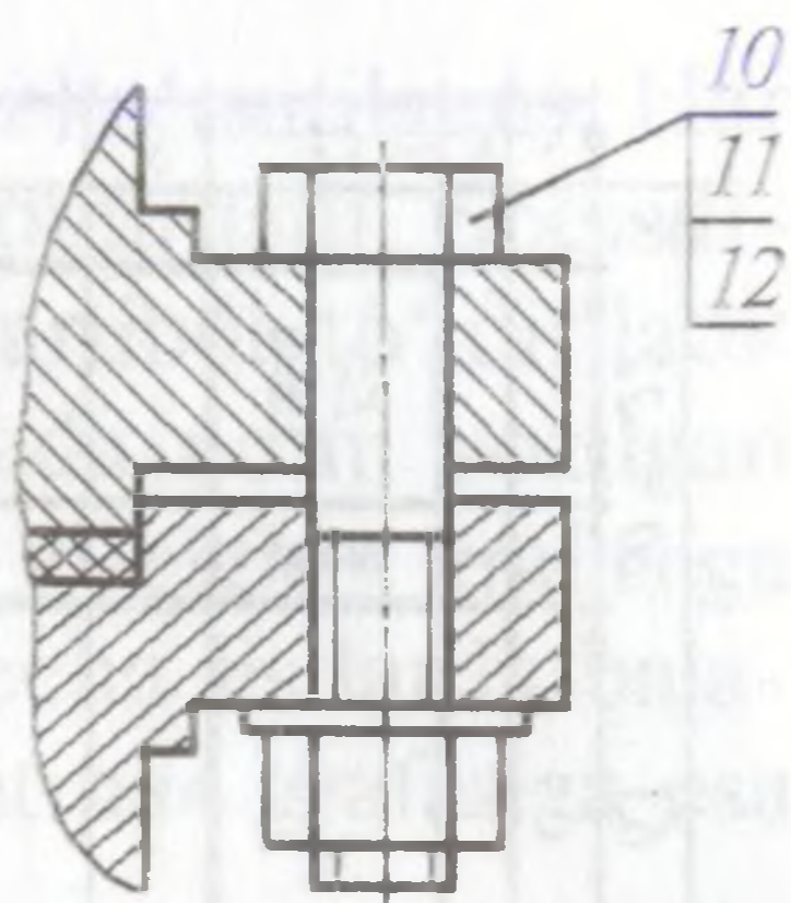
58-shakl. Mahkamlash gruppasiga pozitsiya nomerlarini qo'yish.
