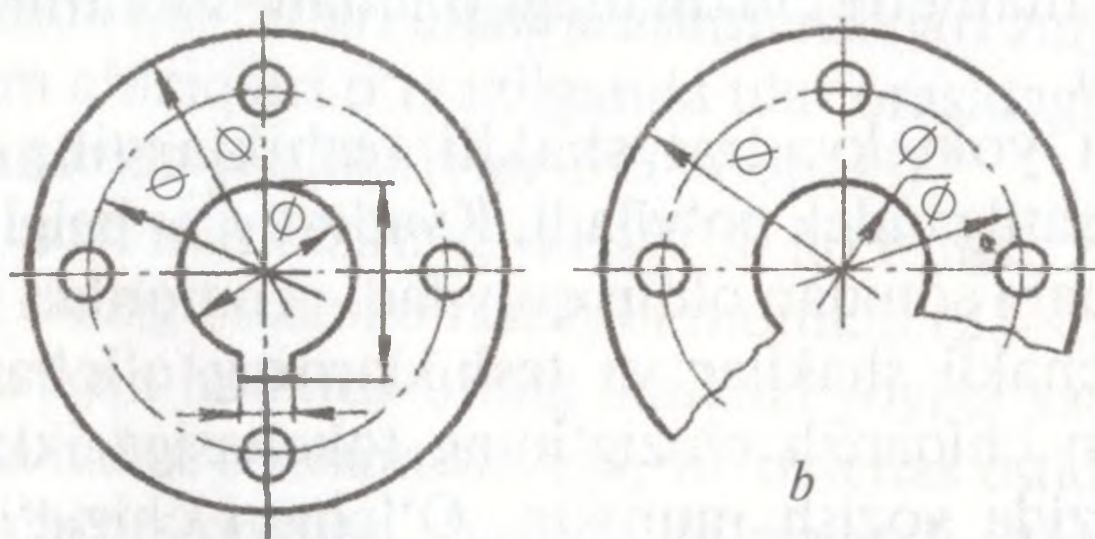
27-shakl. Diametr o'lcham chiziqlarini uzib tasvirlash.
