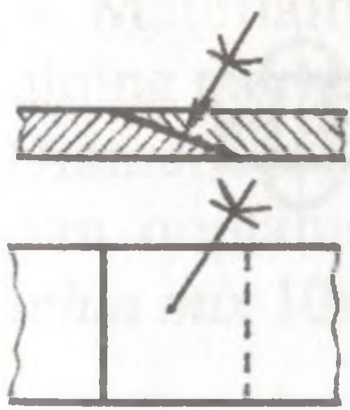
149-shakl. Yelimlangan choklarni belgilash.
