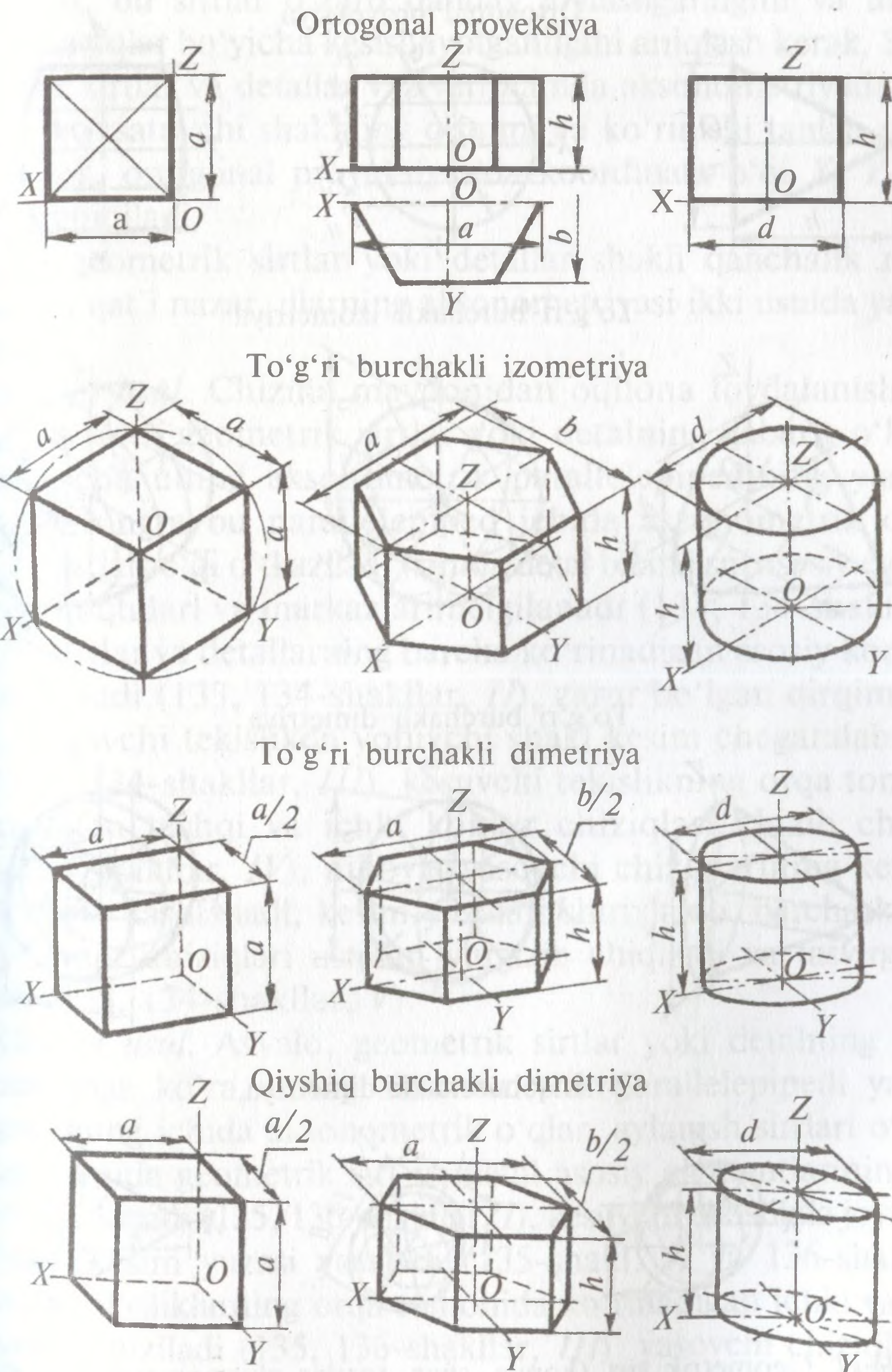
131-shakl. Geometrik sirt (qutb, oltioyoqli prizma, silindr)lar aksonometriyasini yasash.
