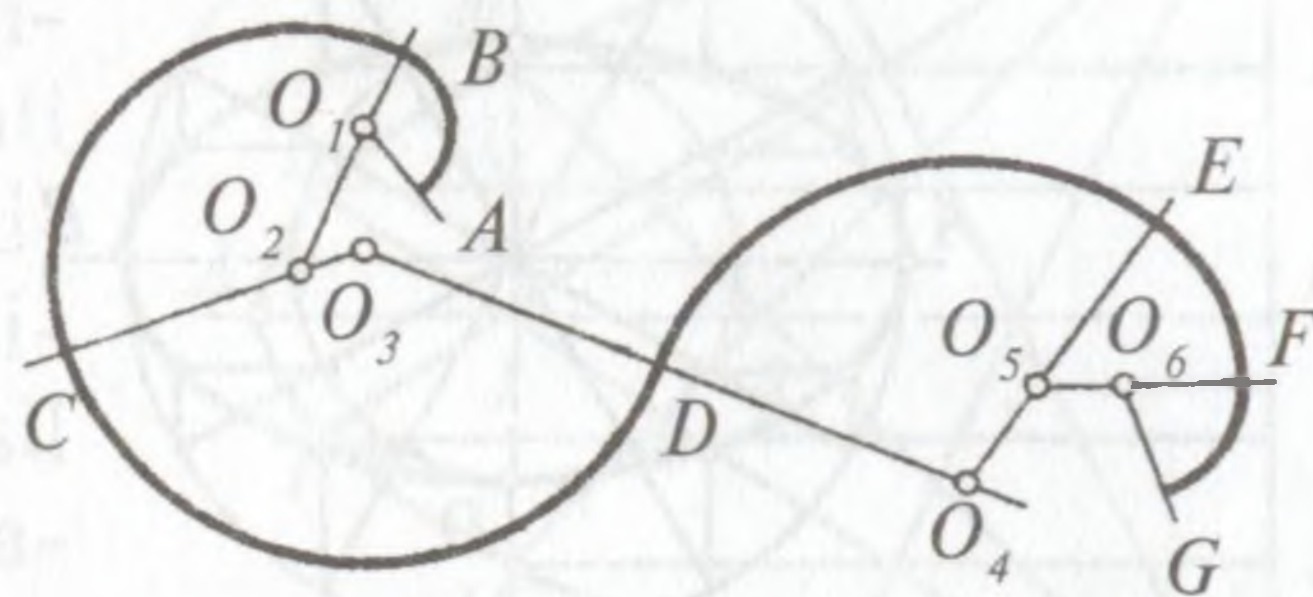
76-shakl. Lekalo yoylarini sirkulda chizish.
