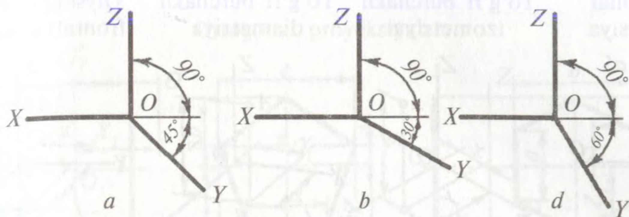
121-shakl. Qiyshiq burchakli frontal diametrik o'qlar vaziyati.
