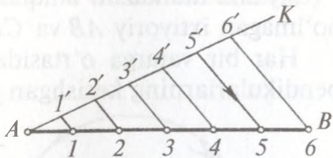
67-shakl. Kesmani teng bo'laklarga bo'lish.
