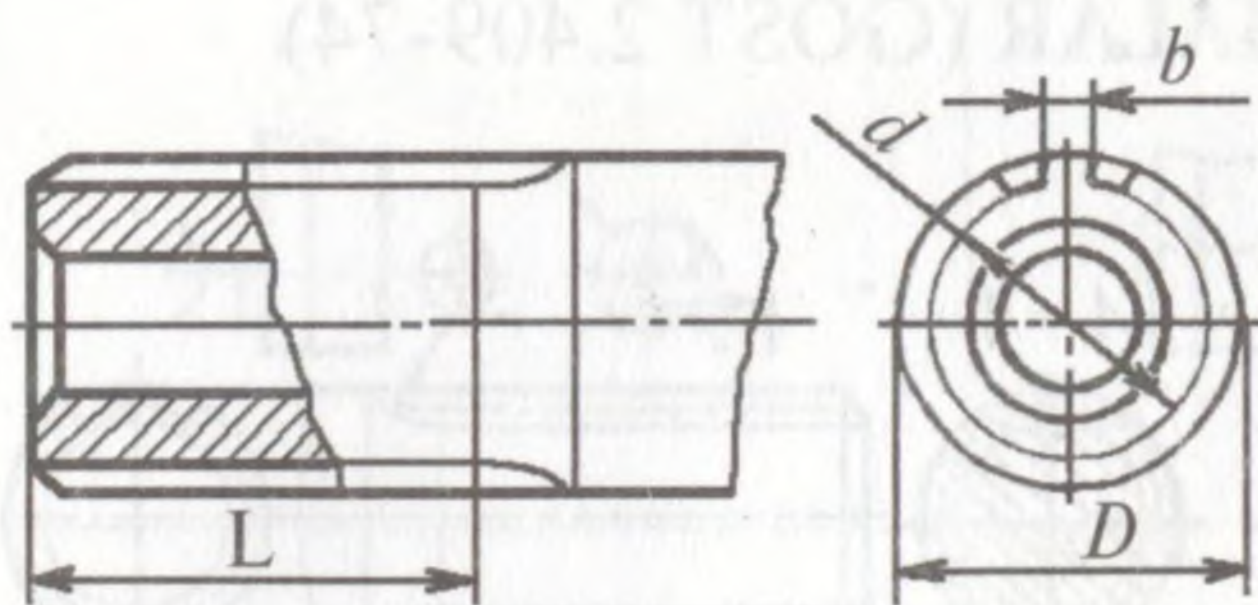
161-shakl. Shlitsali valga o'lcham qo'yish.
