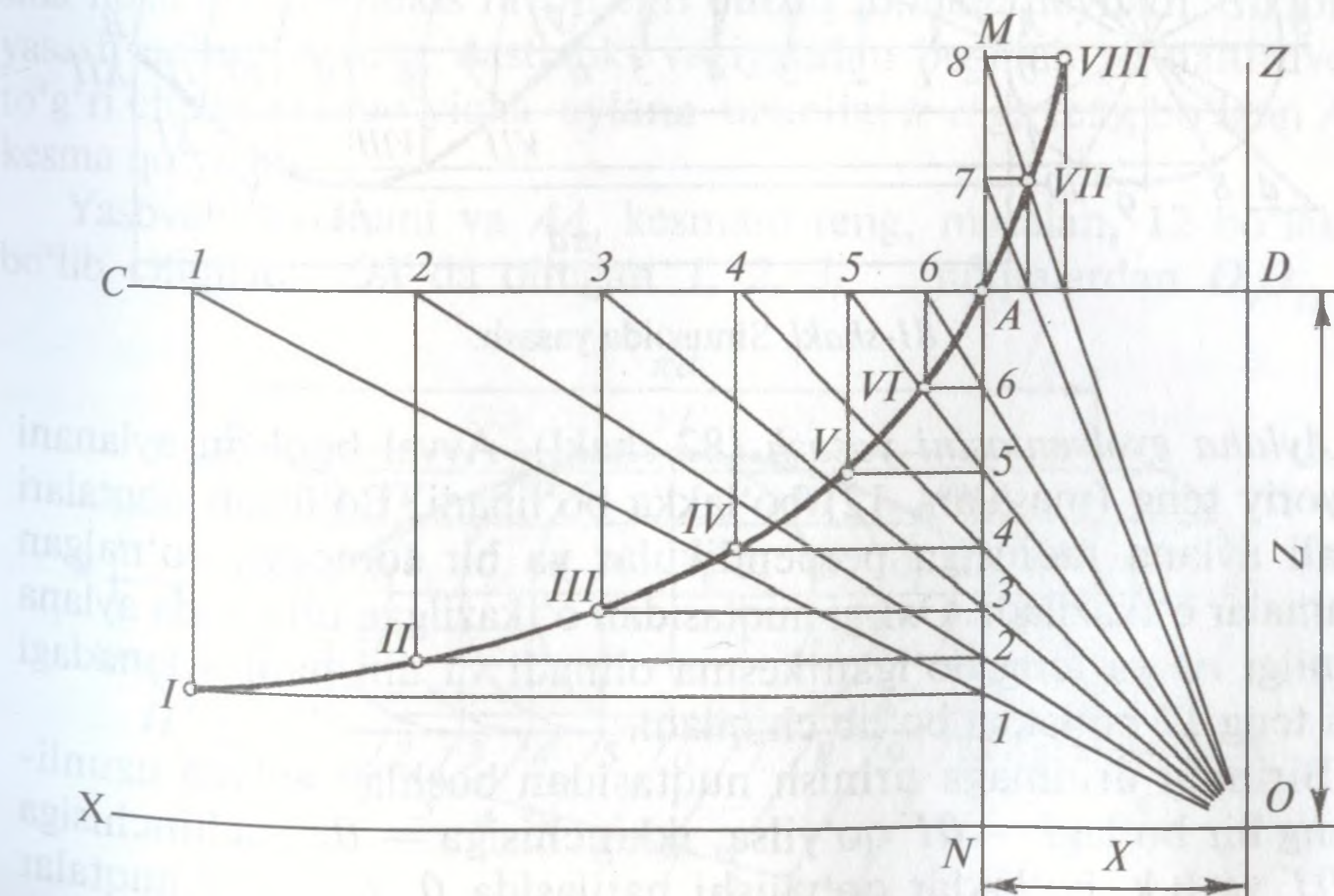
80-shakl. Giperbola yasash.
