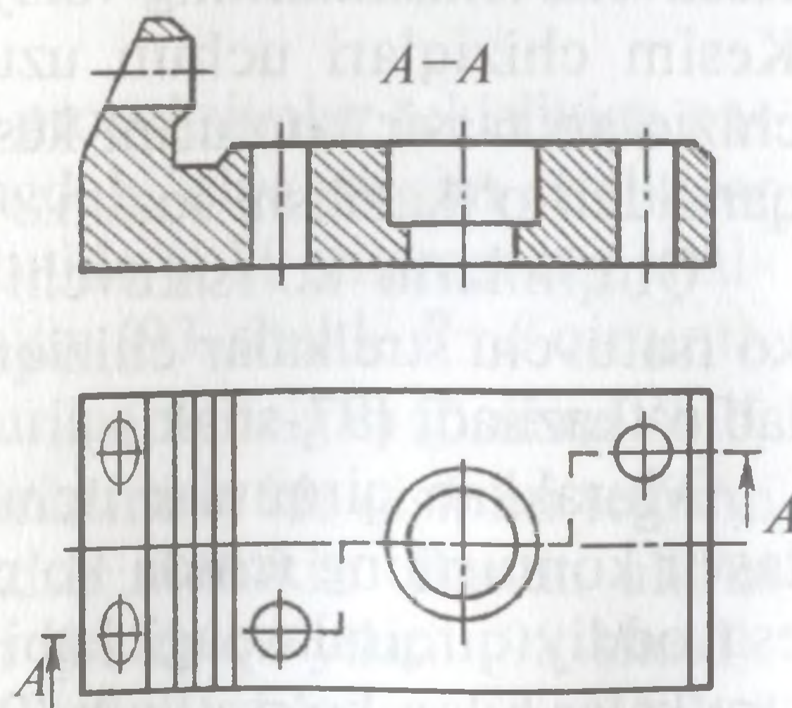
94-shakl. Pog'onali murakkab frontal qirqim.
