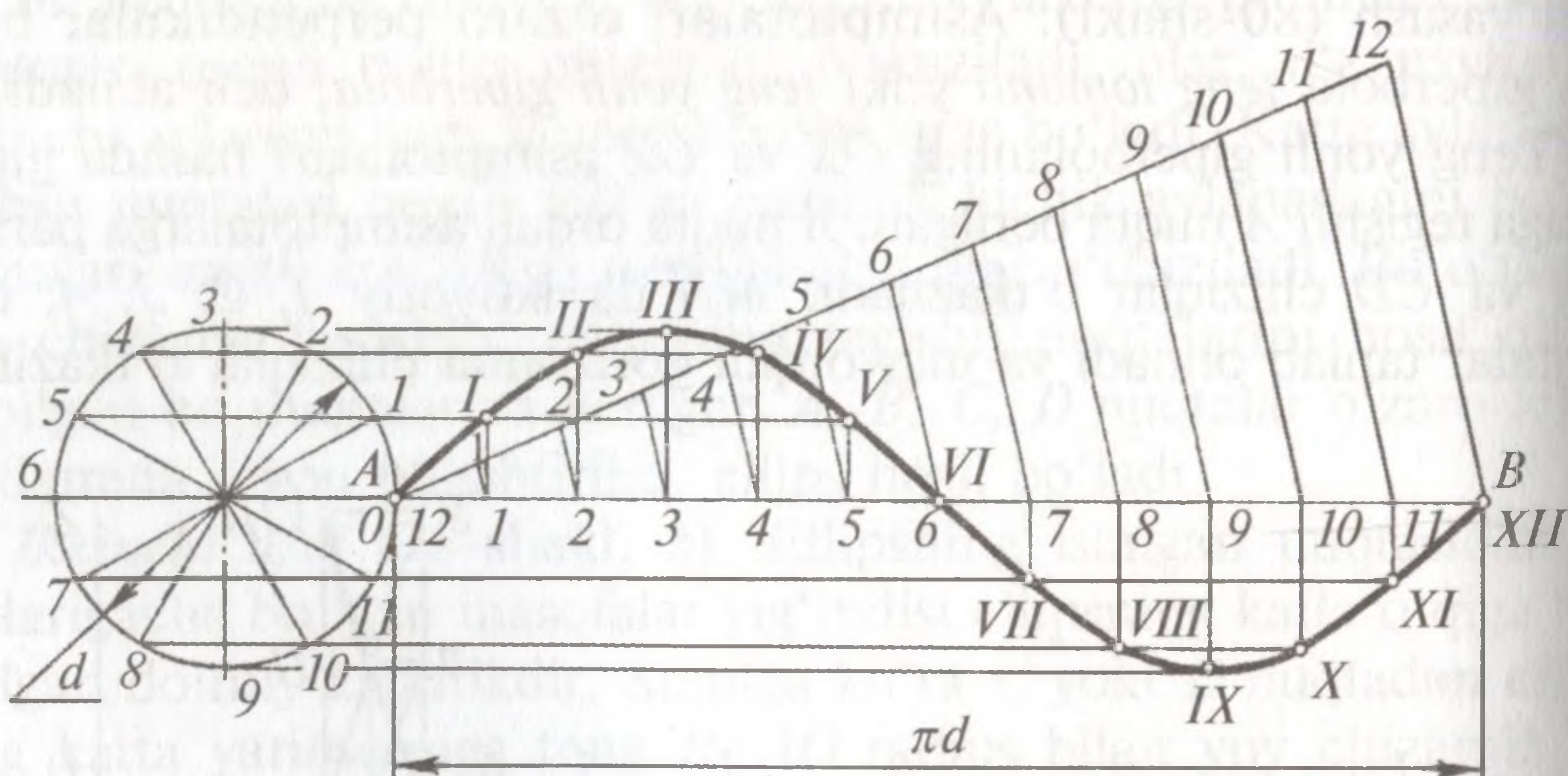
81-shakl. Sinusoida yasash.
