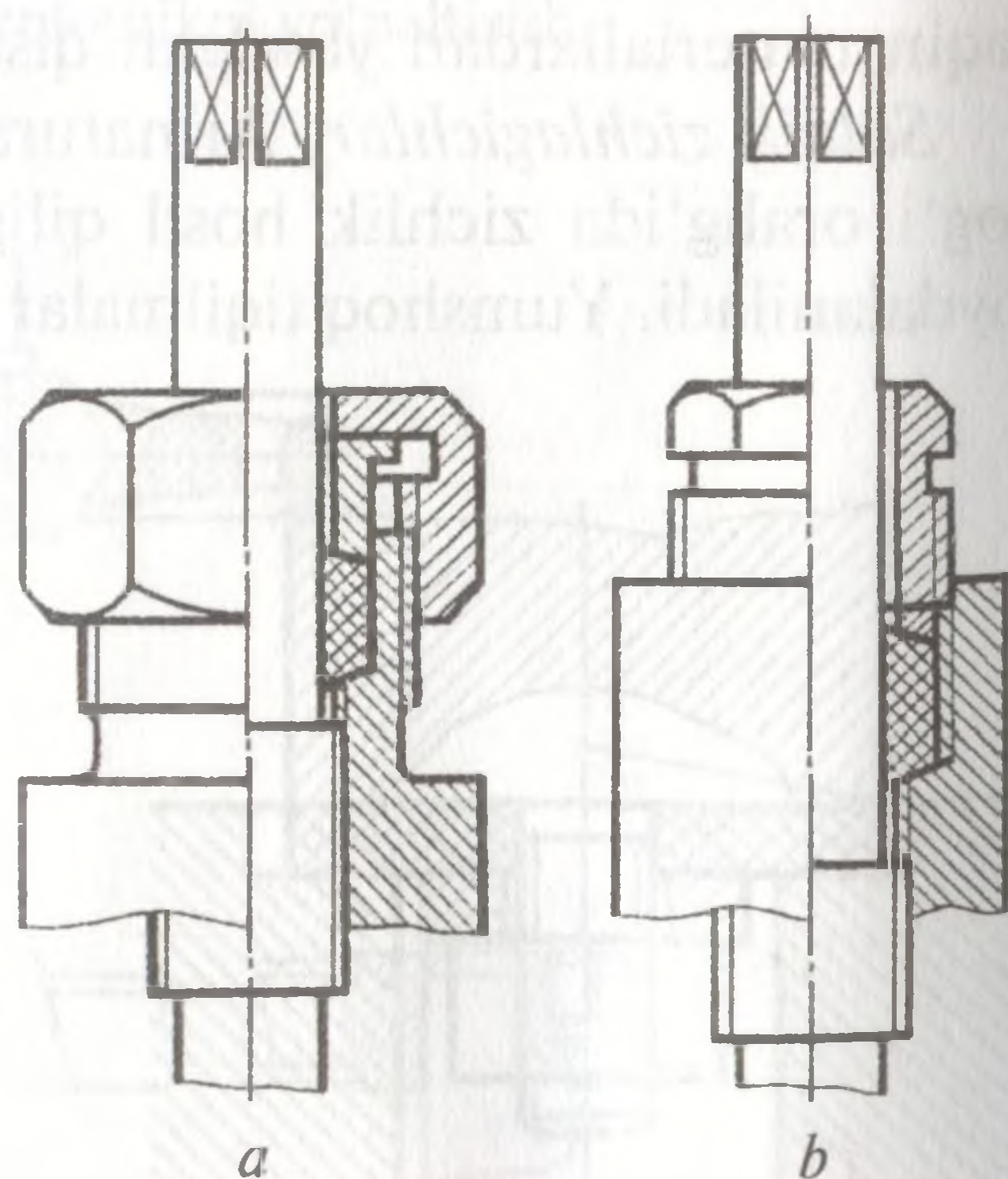
176-shakl. Ustama gaykalar yordamida tiqilmalarni qisish.
