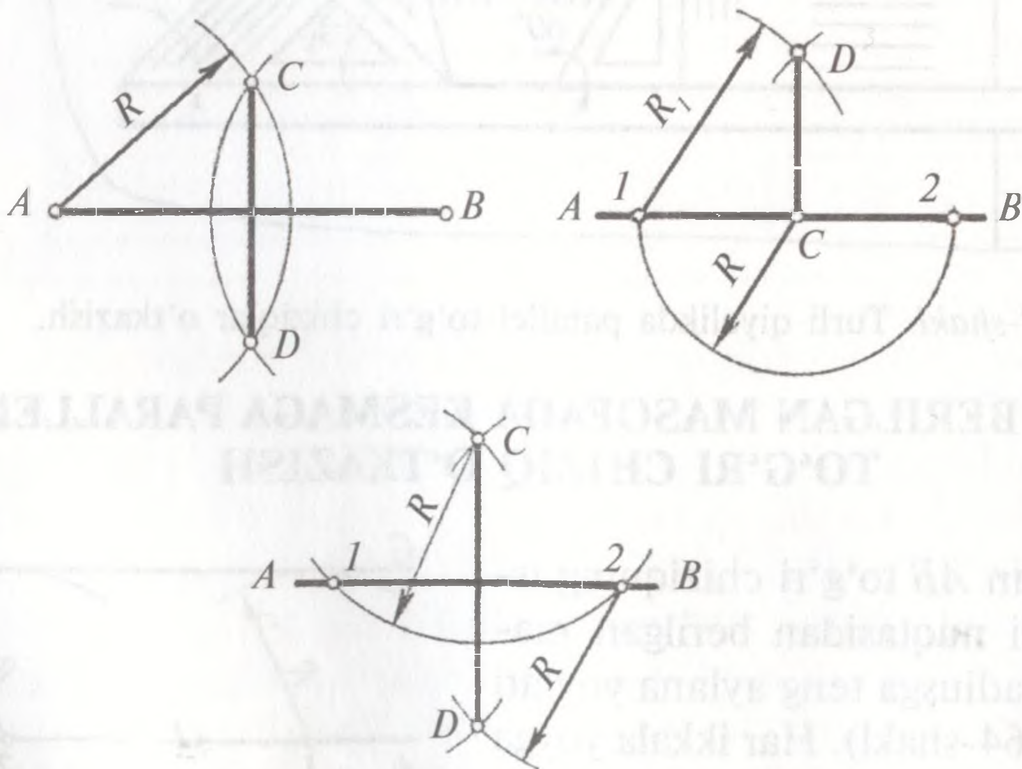
65-shakl. Berilgan to'g'ri chiziqqa perpendikular o'tkazish.
