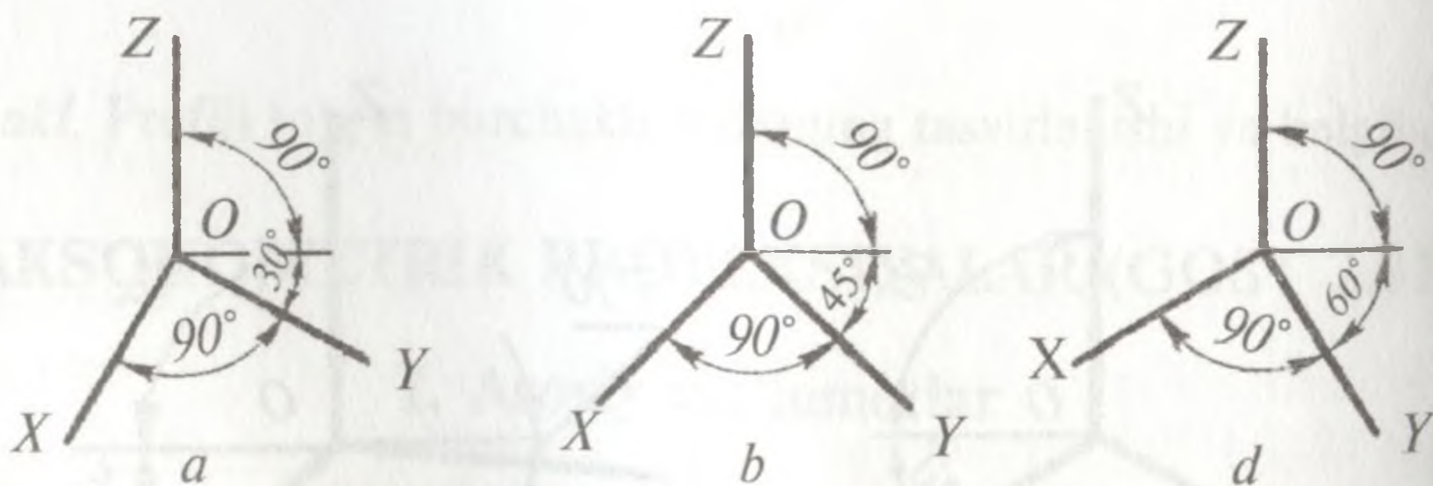
120-shakl. Qiyshiq burchakli gorizontal izometrik o'qlar vaziyati.
