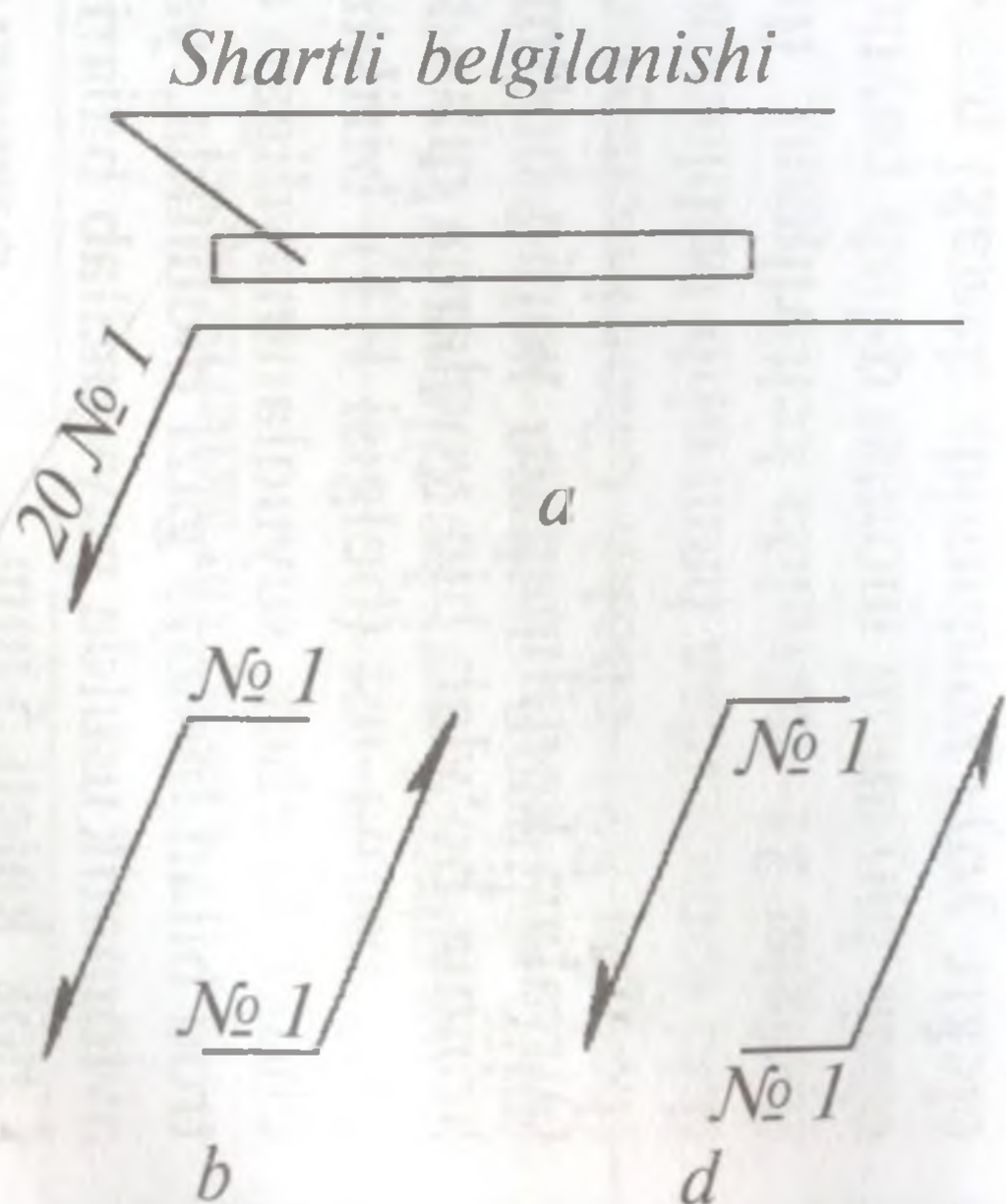
147-shakl. Bir xil choklarni belgilash.
