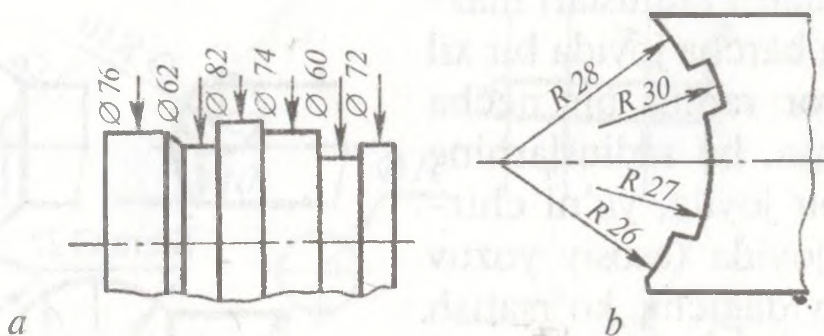
26-shakl. Murakkab shakllarga o'lchamlar qo'yish.
