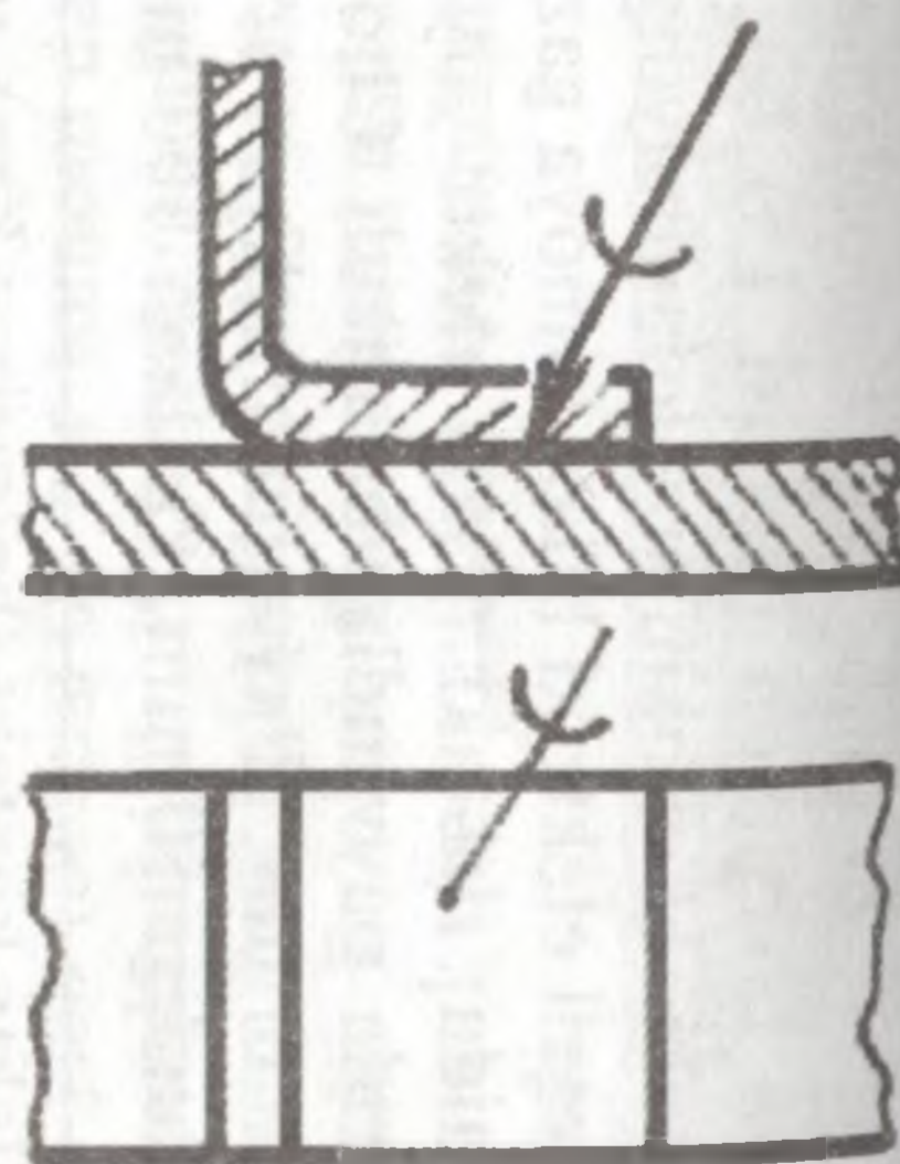
148-shakl. Qalaylangan choklarni belgilash.
