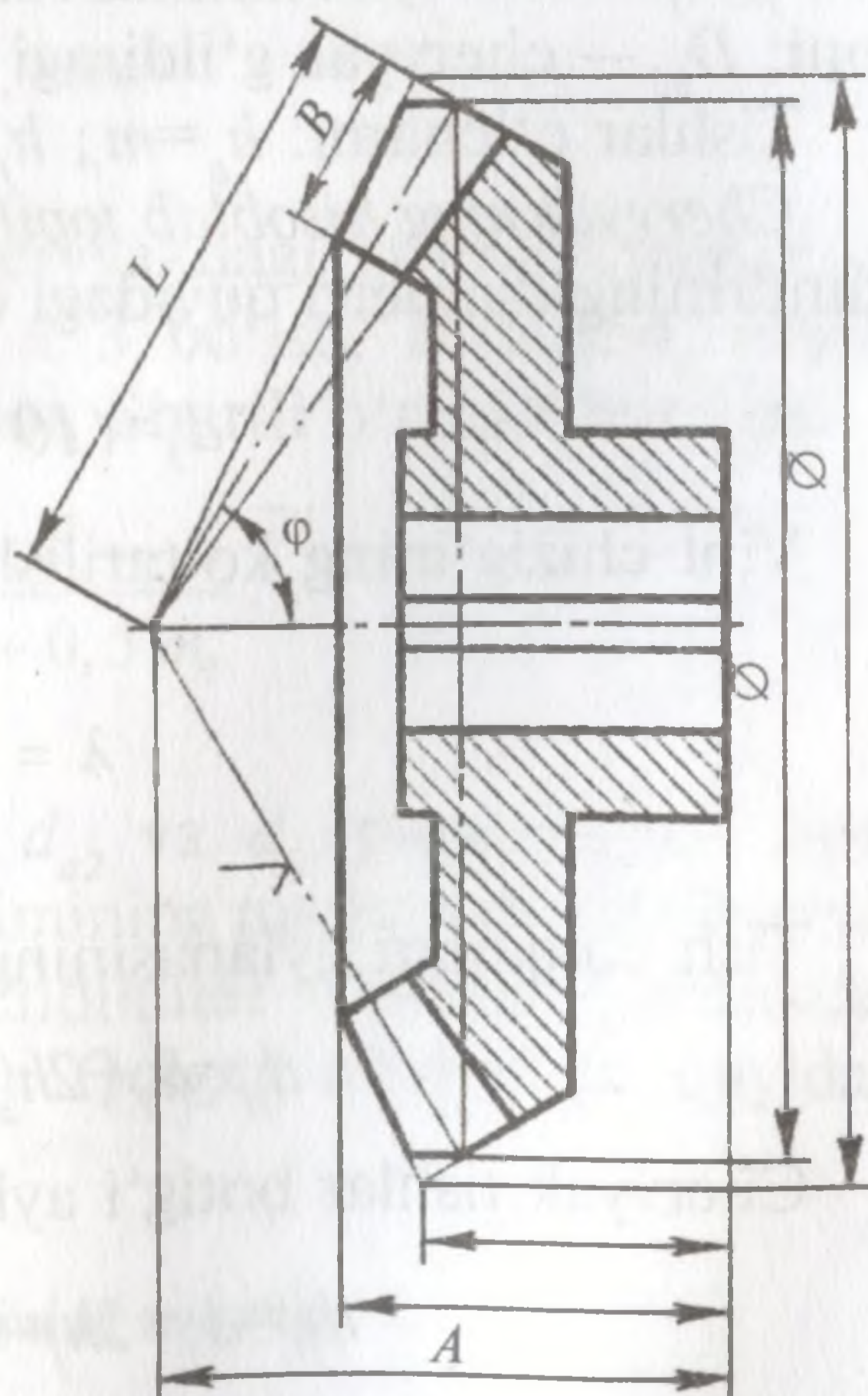
168-shakl. Konussimon tishli g'ildirakning konstruktiv o'lchamlari.
