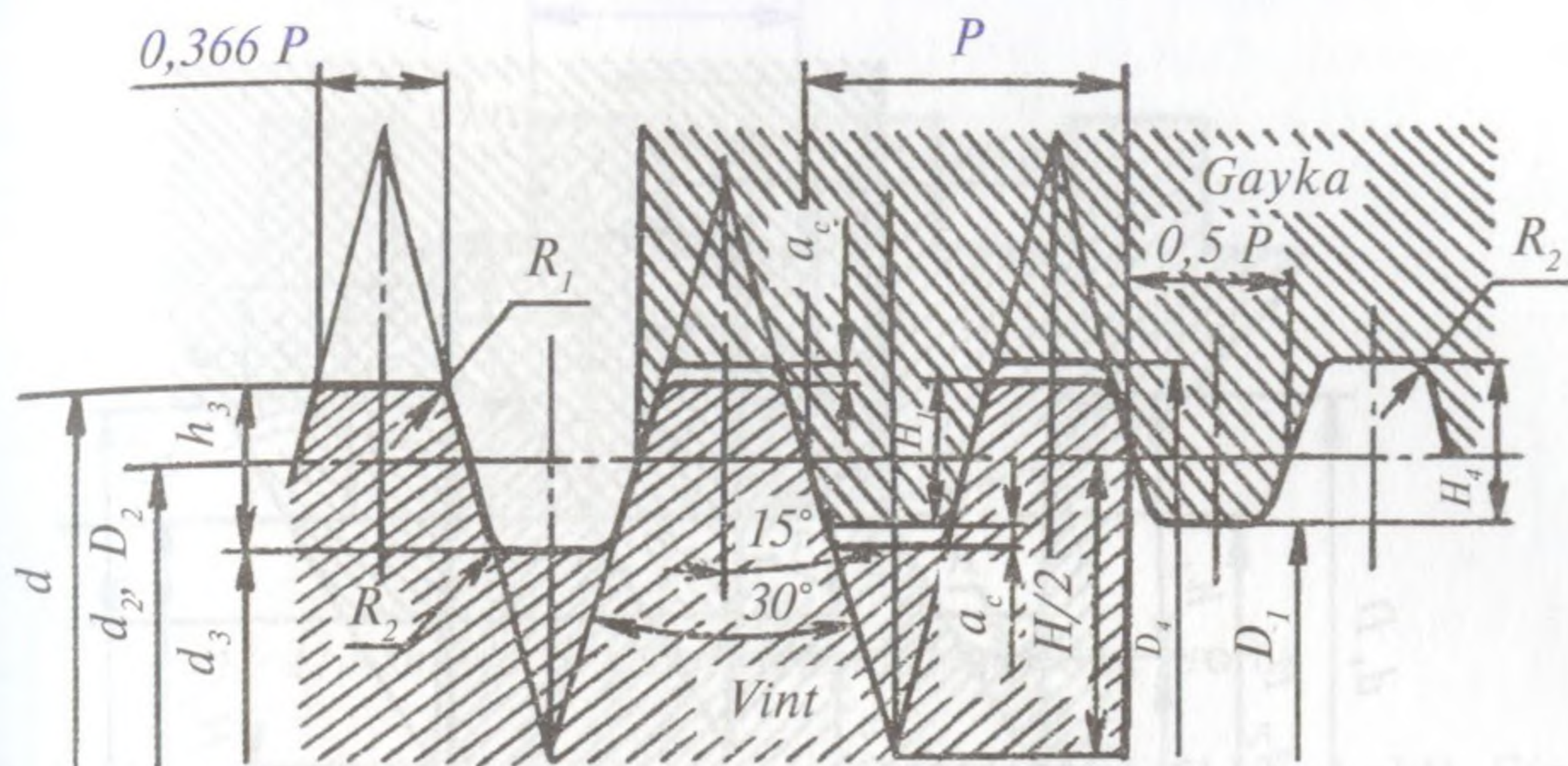
110-shakl. Trapetsiyasimon rezbaning profillari.
