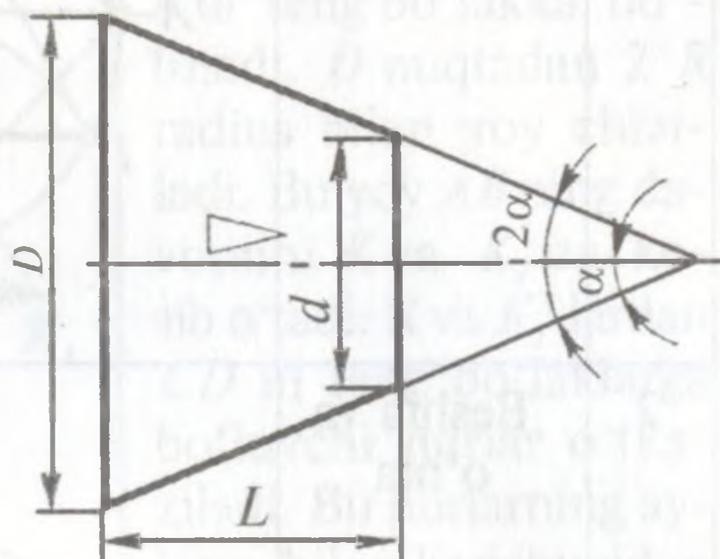
75-shakl. Konuslik.
