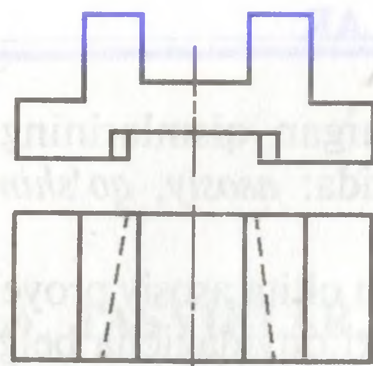
88-shakl. Chizmada ko'rinmas kontur chizig'idan foydalanish.
