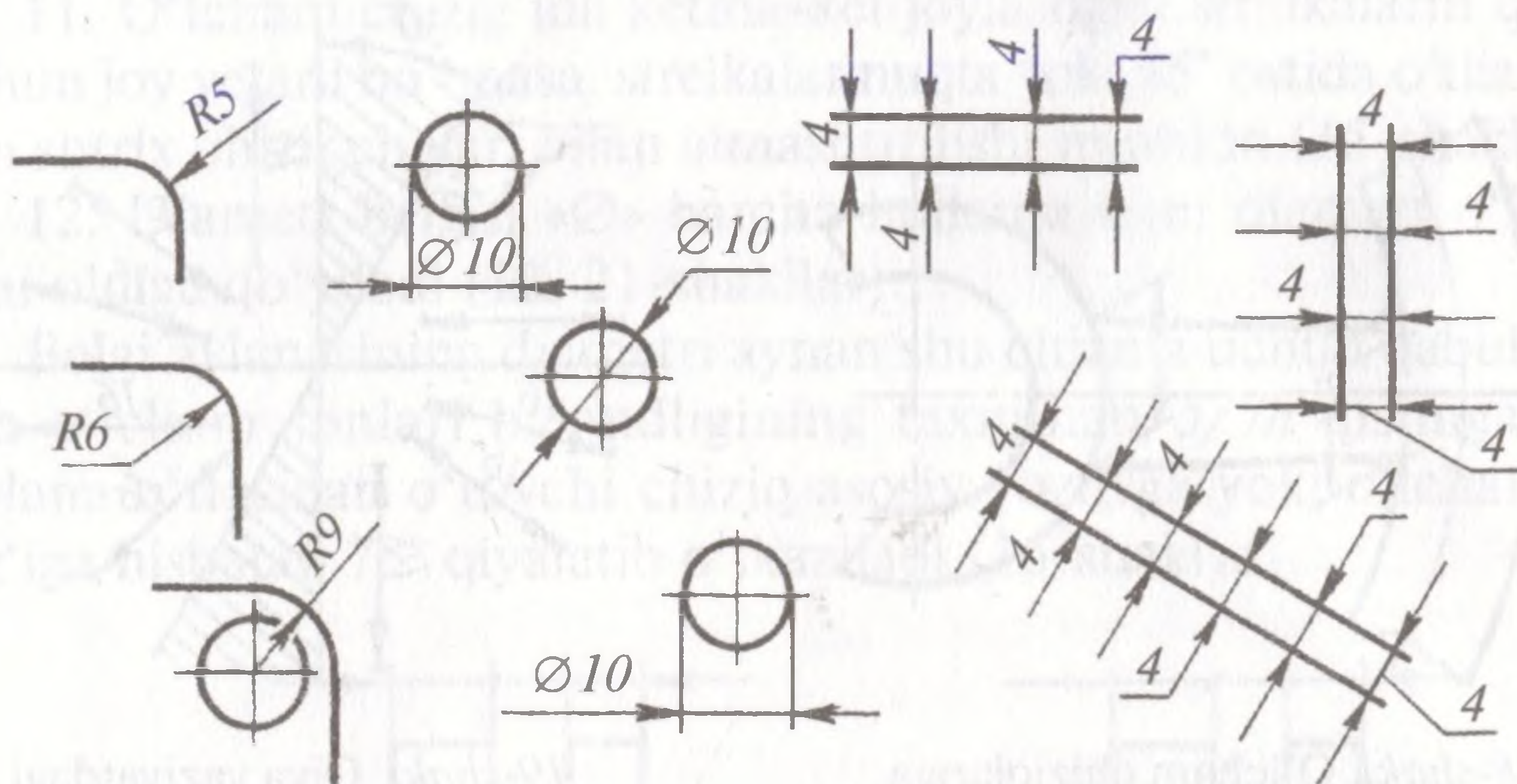
21-shakl. Tor joylarga o'lcham sonlarining yozilishi.
