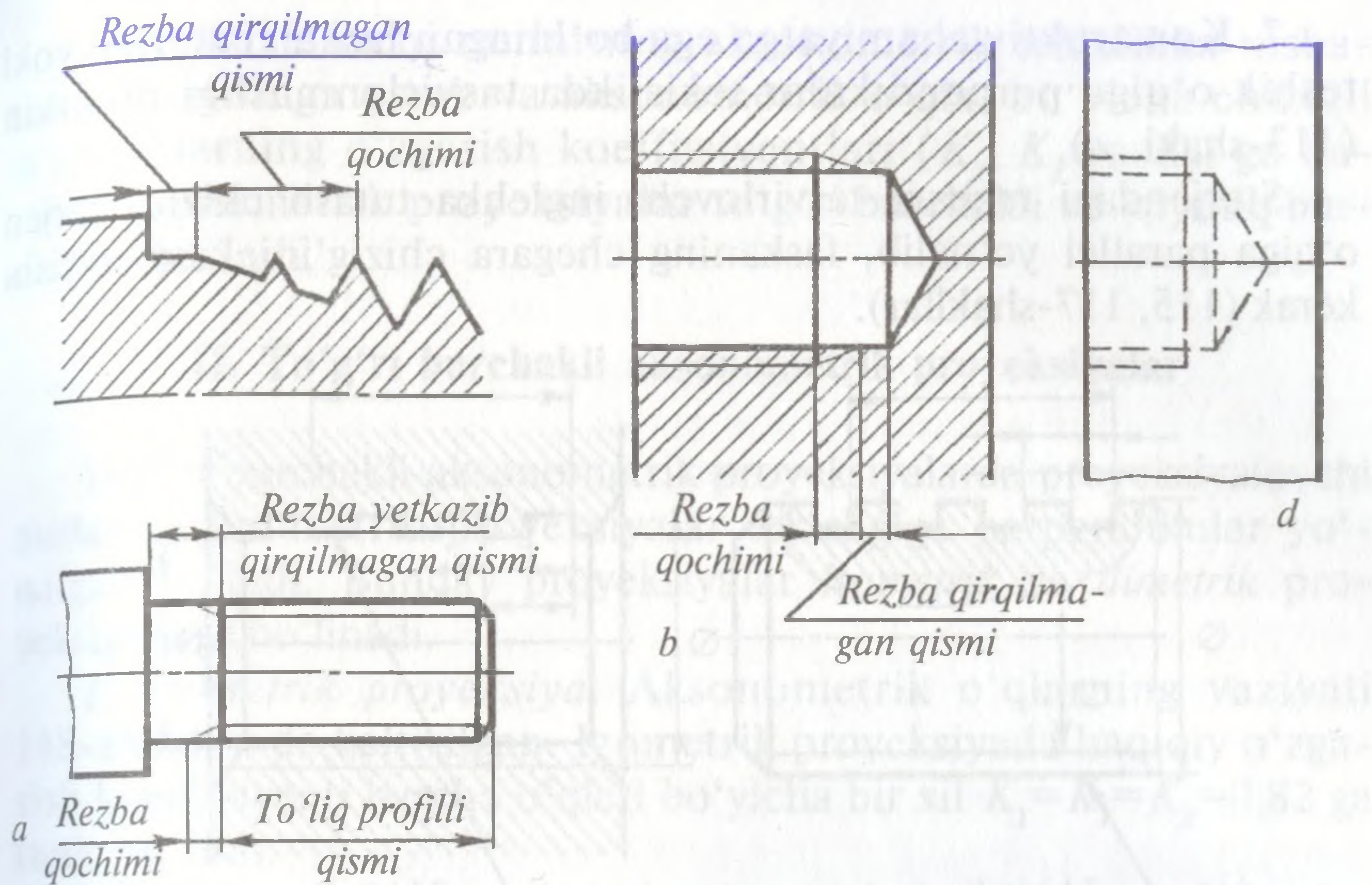
115-shakl. Rezba chegarasini belgilash.
