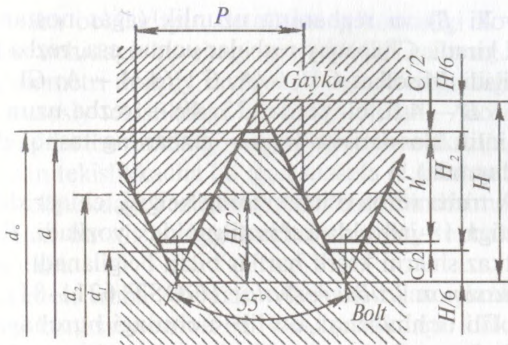
106-shakl. Duymoviy rezbalarning profillari.
