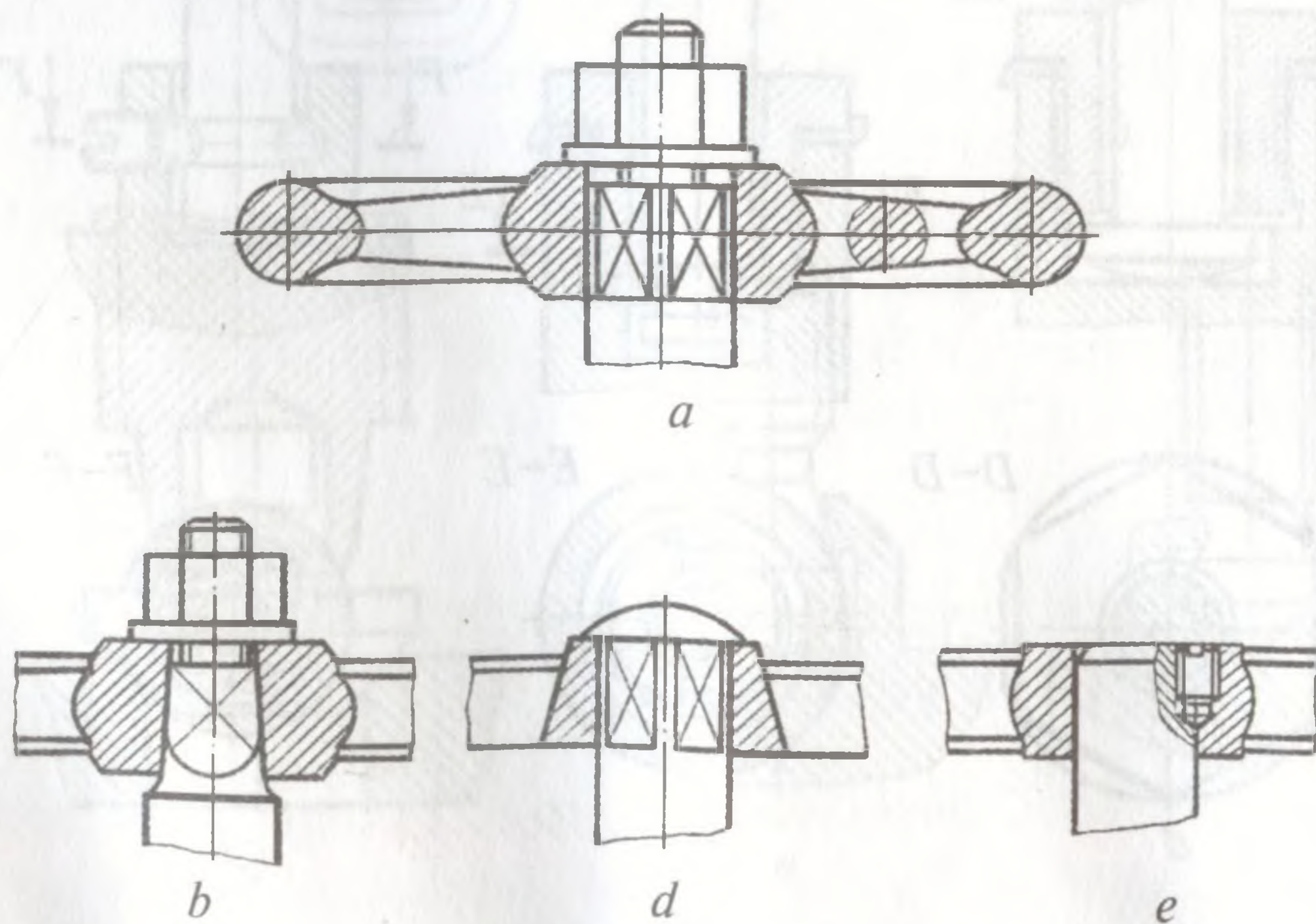
173-shakl. Shpindelga chambaraklarni biriktirish.
