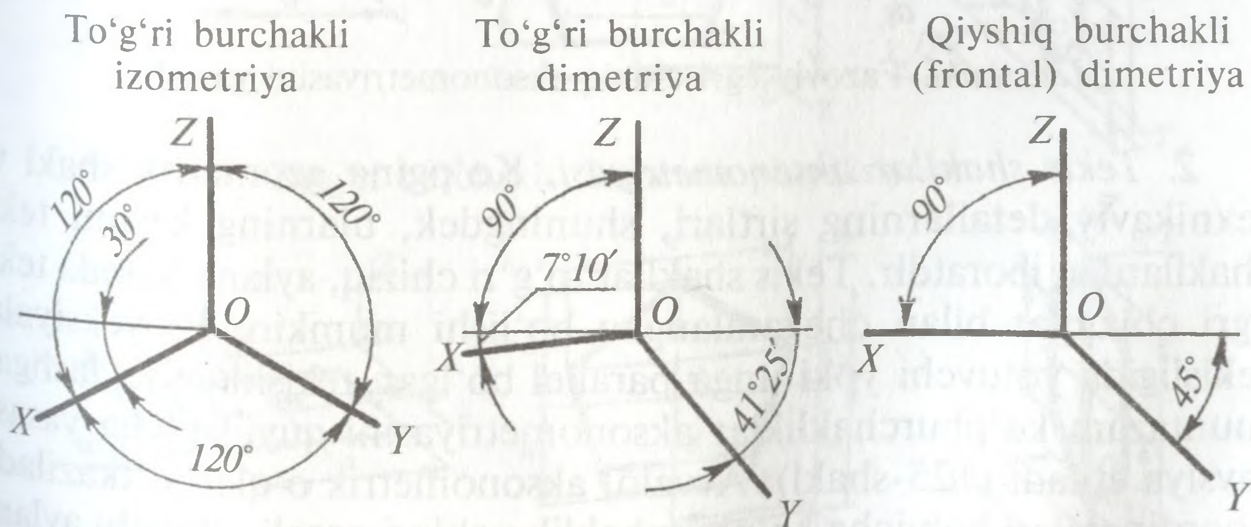
122-shakl. Aksonometrik o'qlar vaziyati.
