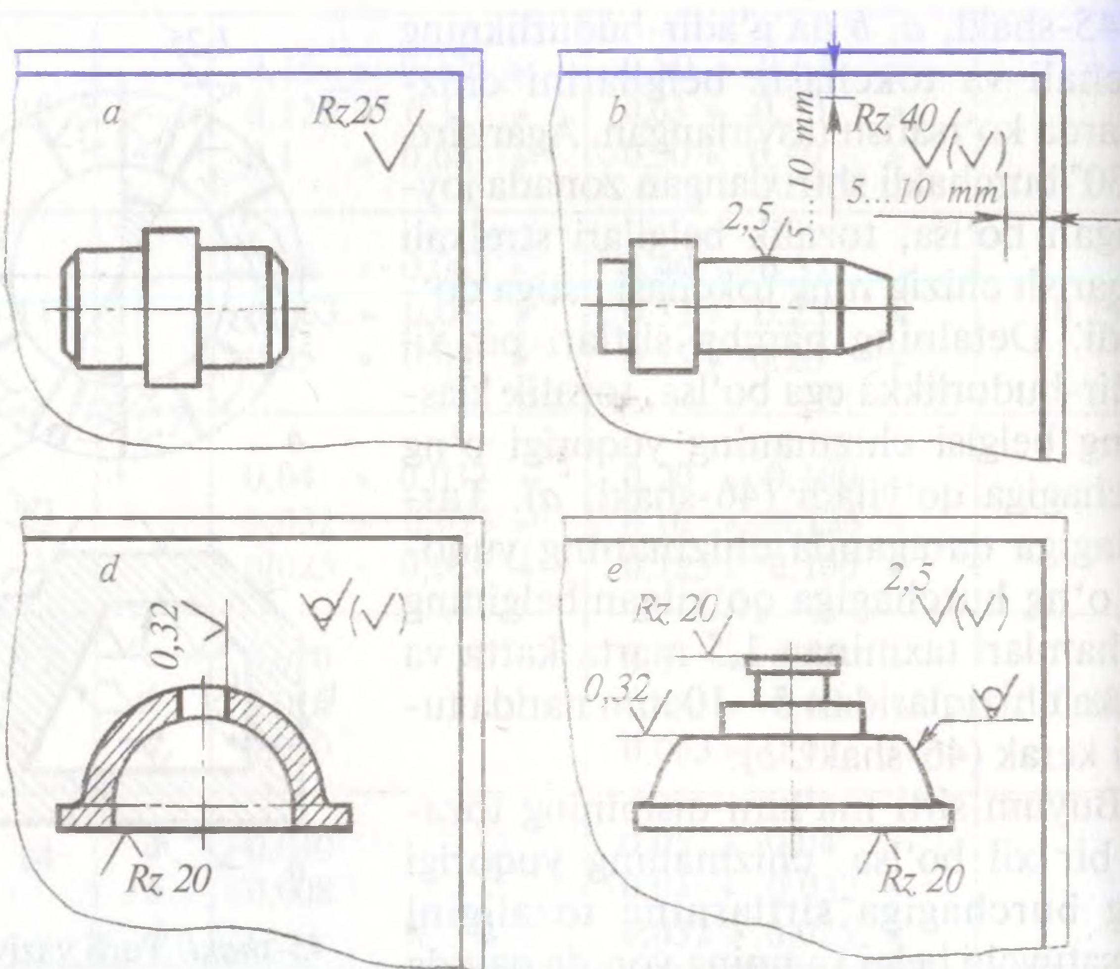
46-shakl. Chizmalarda g'adir-budurlik belgilarining qo'yilishi.
