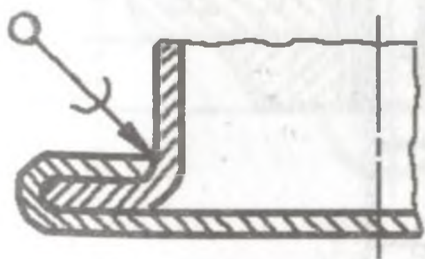
151-shakl. Yopiq kontur bo'yicha qalaylangan chokni belgilash.
