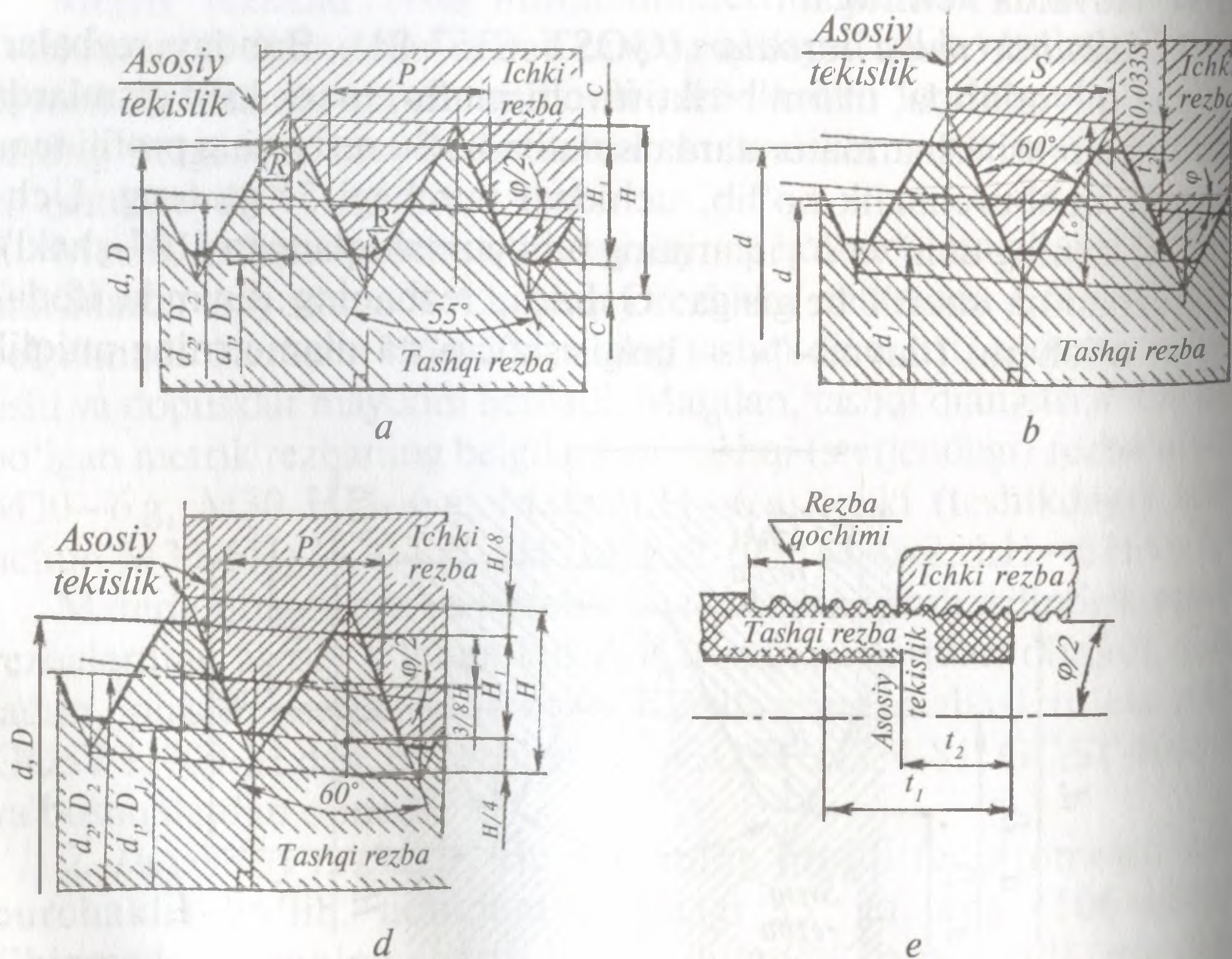
108-shakl. Konussimon rezbalarning profillari.
