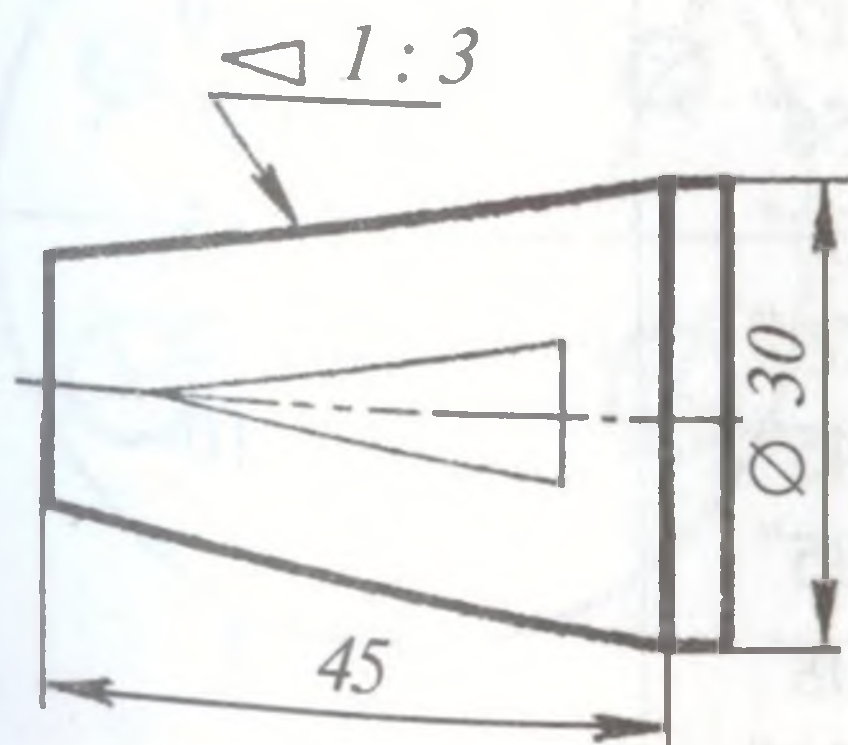
32-shakl. Konuslikning belgilanishi.
