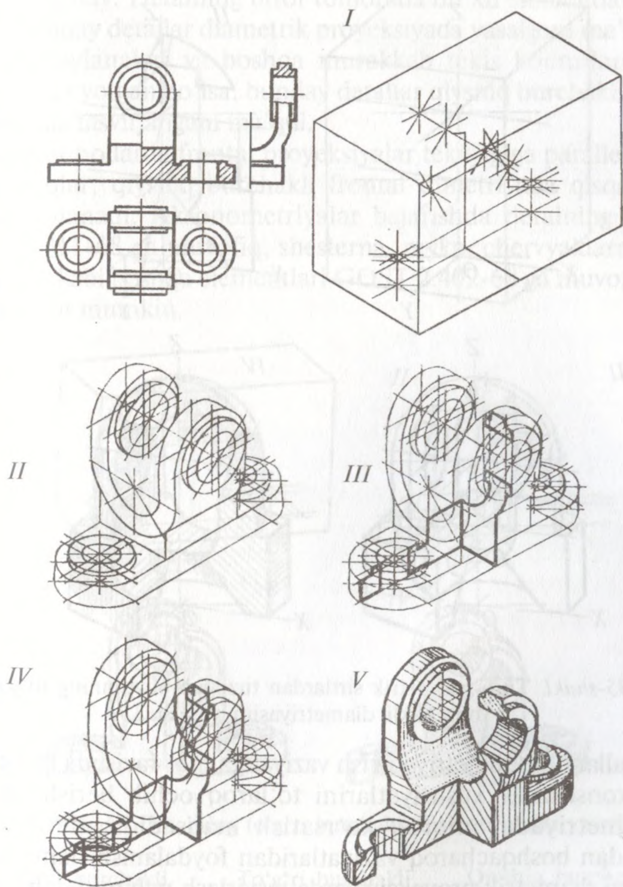
134-shakl. Detalning to'g'ri burchakli izometriyasini yasash.
