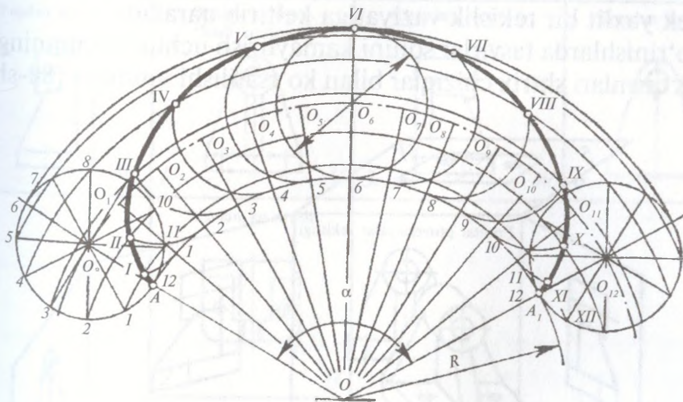
85-shakl. Giposikloida yasash.
