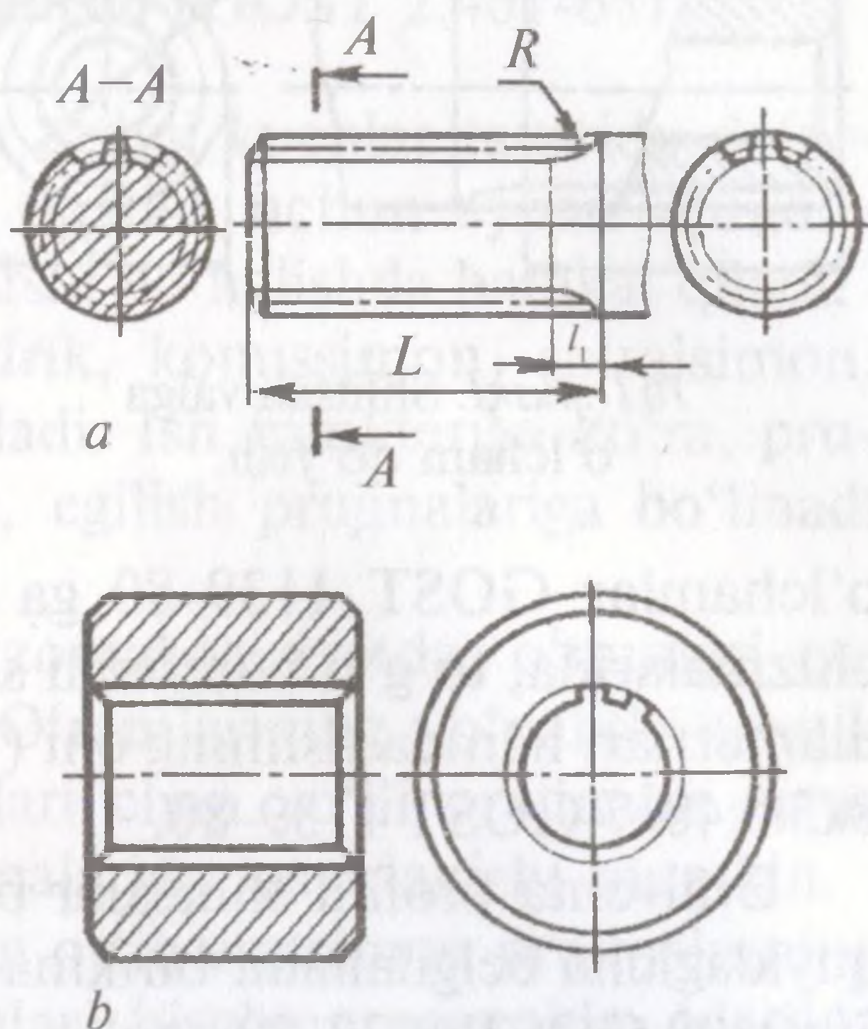
159-shakl. Shlitsa tishlari chiziqlarining tasvirlanishi.
