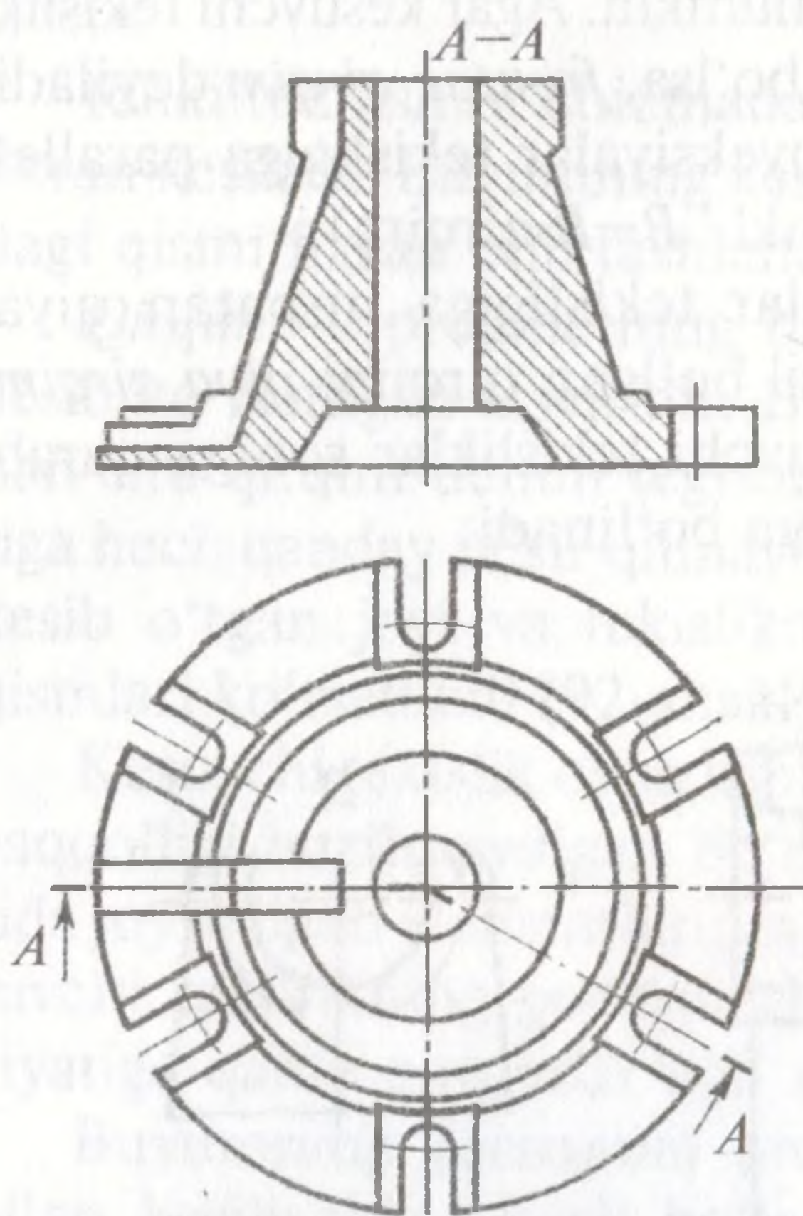
95-shakl. Siniq murakkab qirqim.
