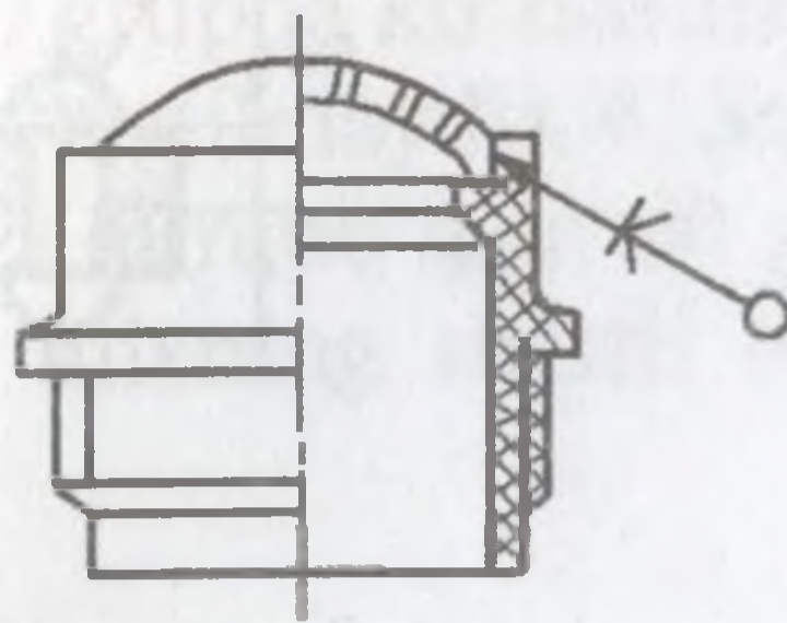
150-shakl. Yopiq kontur bo'yicha yelimlangan chokni belgilash.
