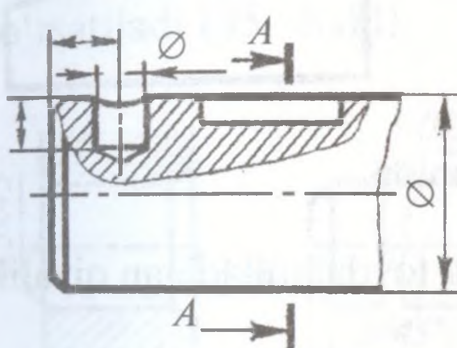
28-shakl. Uzib tasvirlangan detalning o'lcham chizig'i.
