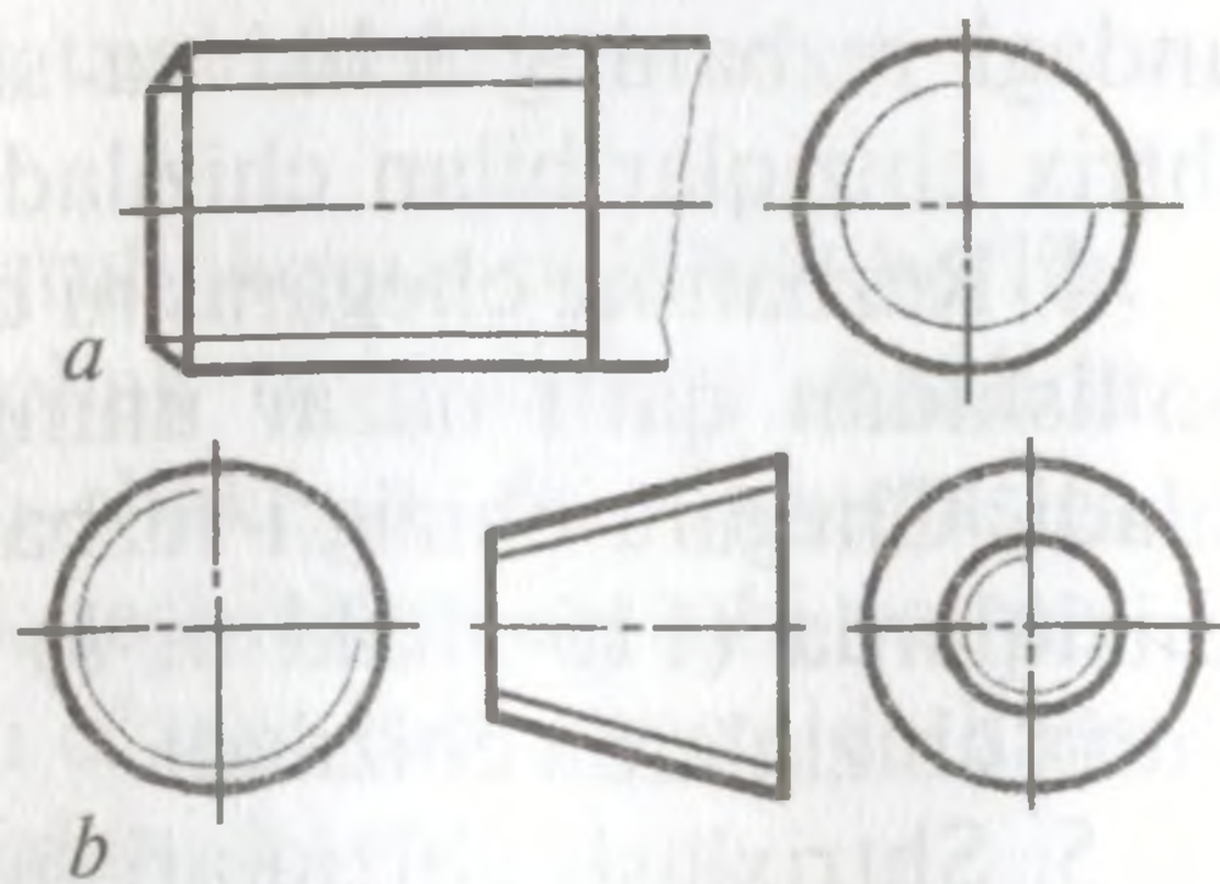
113-shakl. Sterjendagi rezbaning tasvirlanishi.
