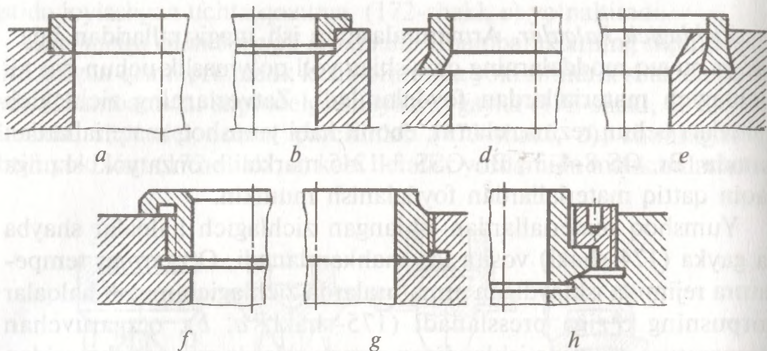
175-shakl. Metall zichlagich halqalarni mahkamlash.
