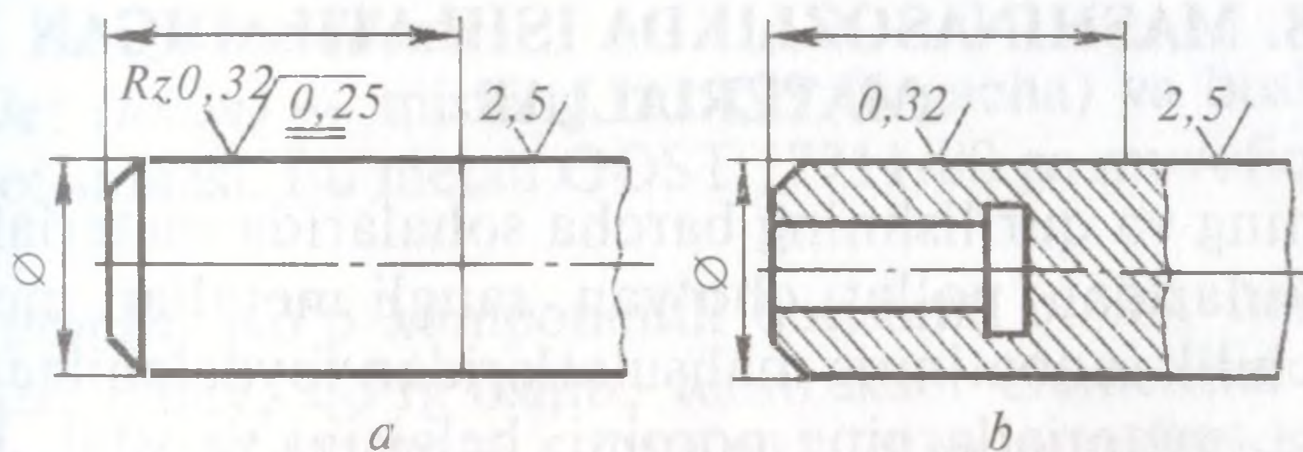
48-shakl. Bitta yuzaning turli uchastkalaridagi g'adir-budurligining belgilanishi.
