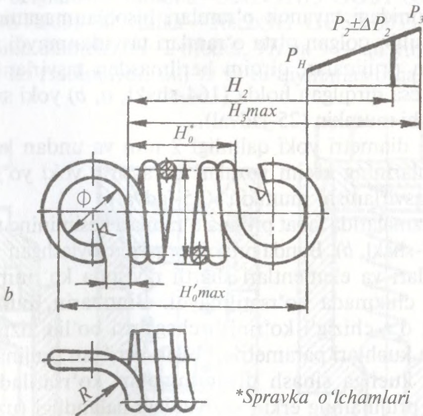
164-shakl. Prujinalarning ish chizmalari.
