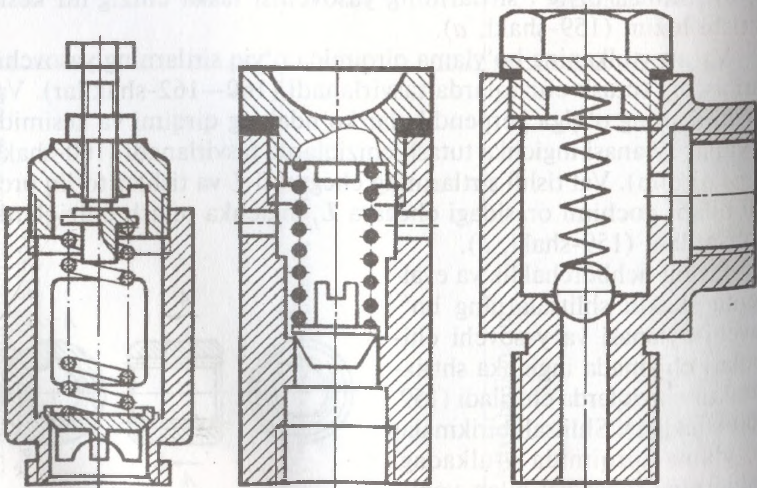
163-shakl. Yig'uv chizmalarida prujinalarni tasvirlash.
