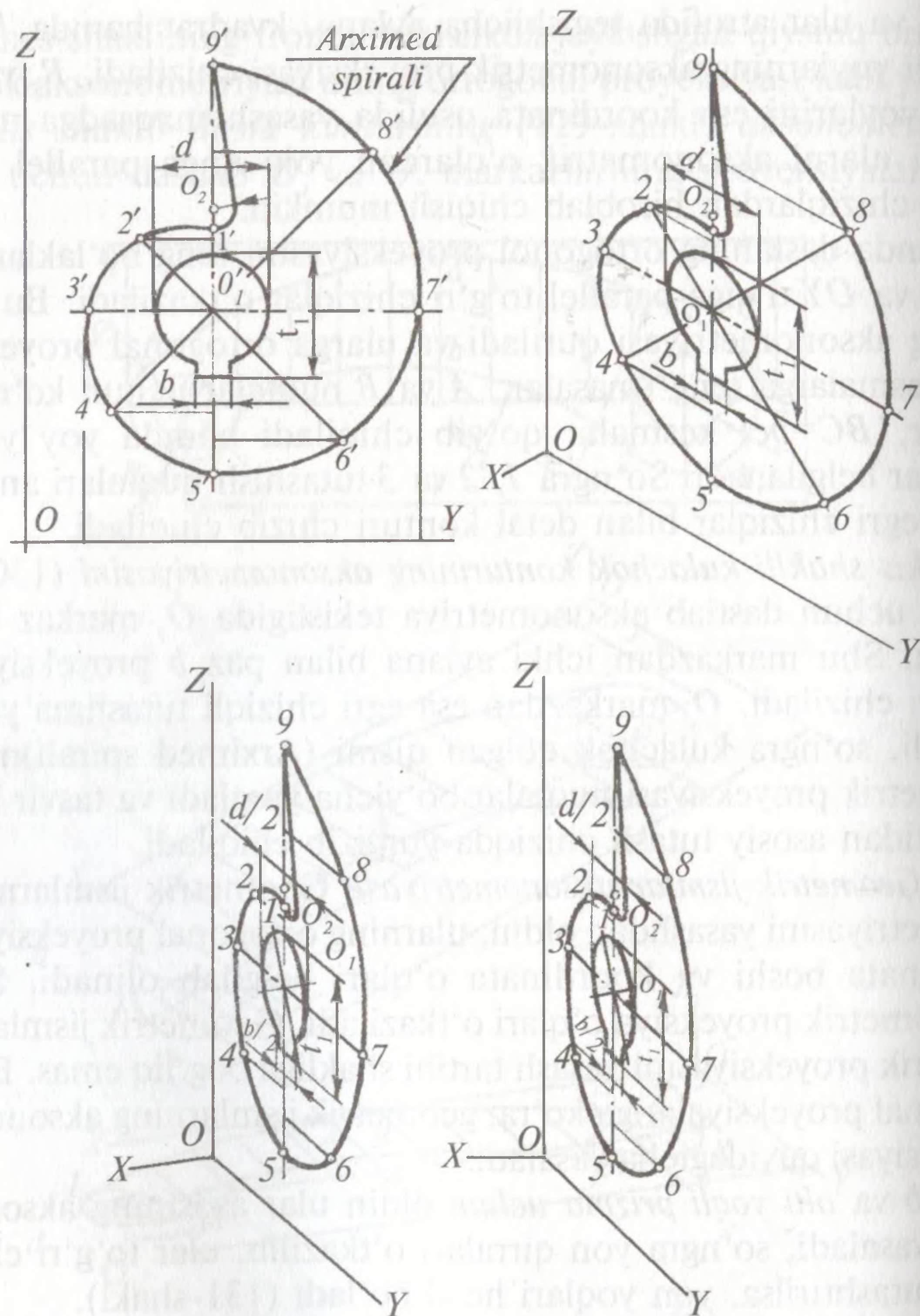
130-shakl. Kulachok konturi aksonometriyasini yasash.
