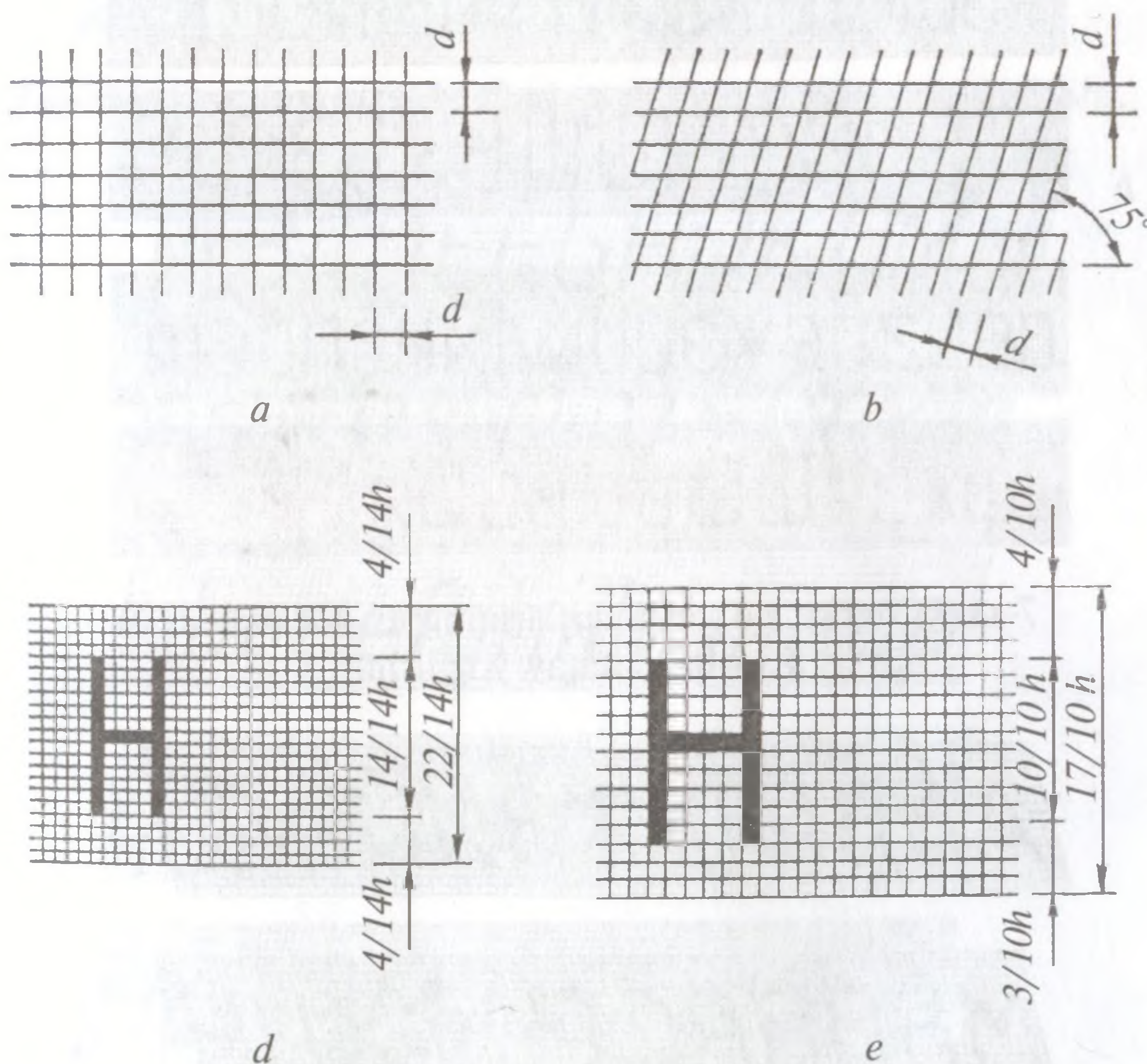
6-shakl. Yordamchi to'rlardan foydalanib shriftlarning yozilishi:
