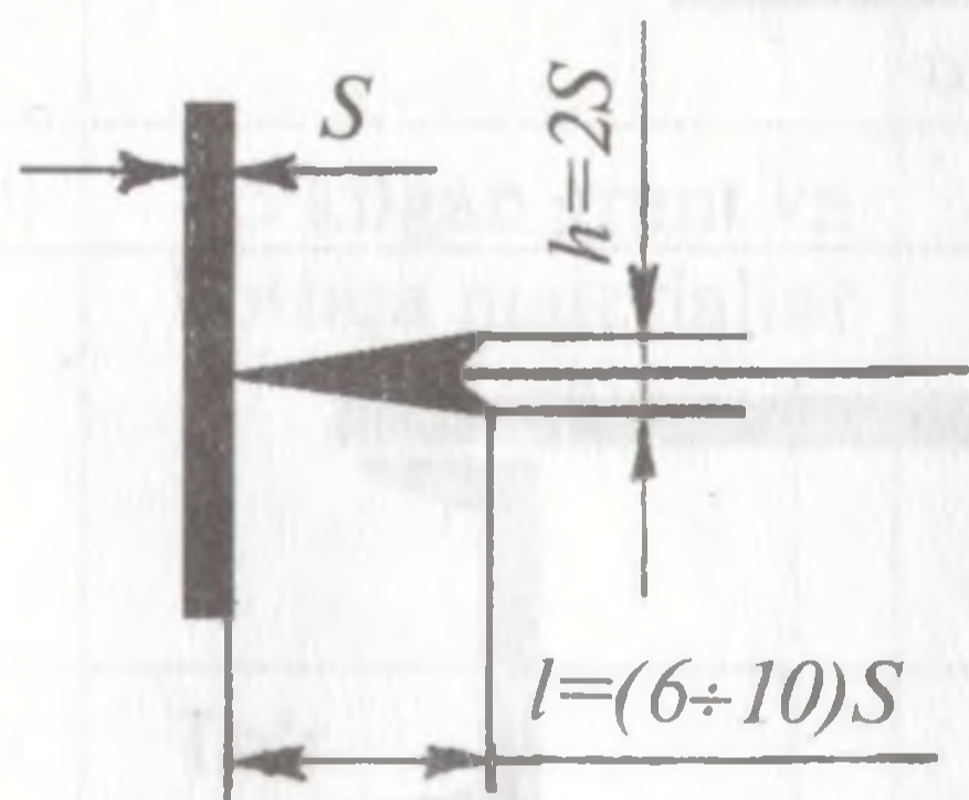
10-shakl. Strelkaning o'lchami.
