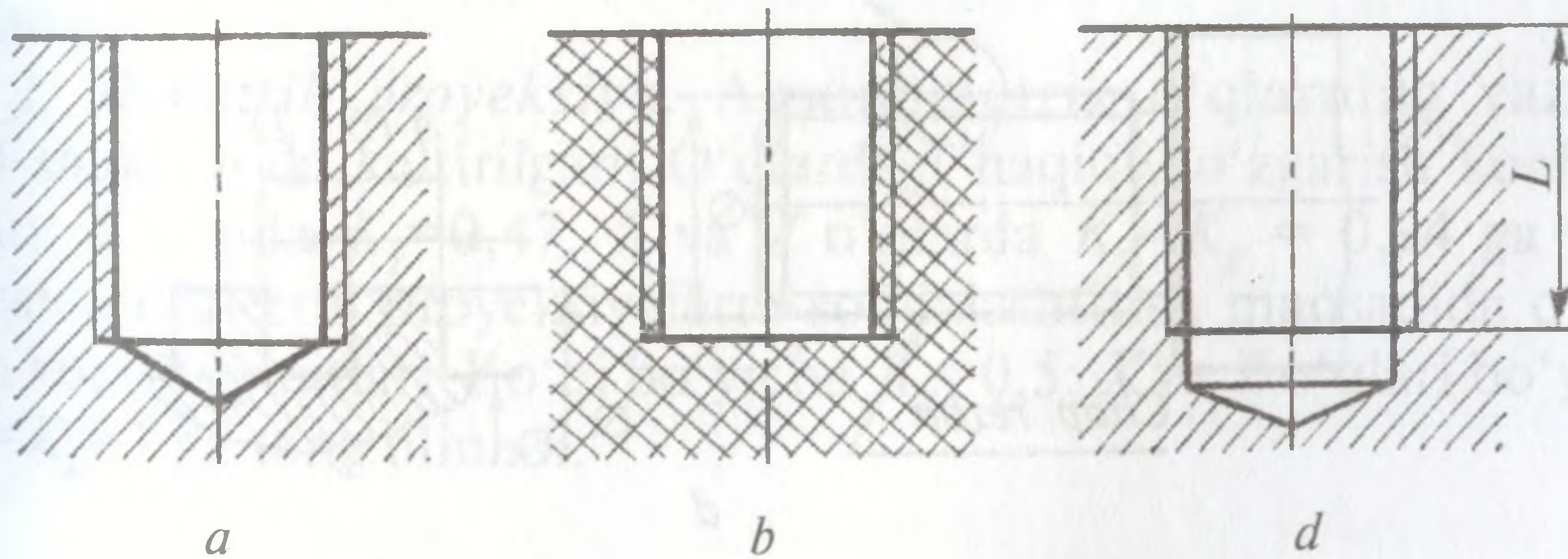
116-shakl. Uyachada rezbaning tasvirlanishi.
