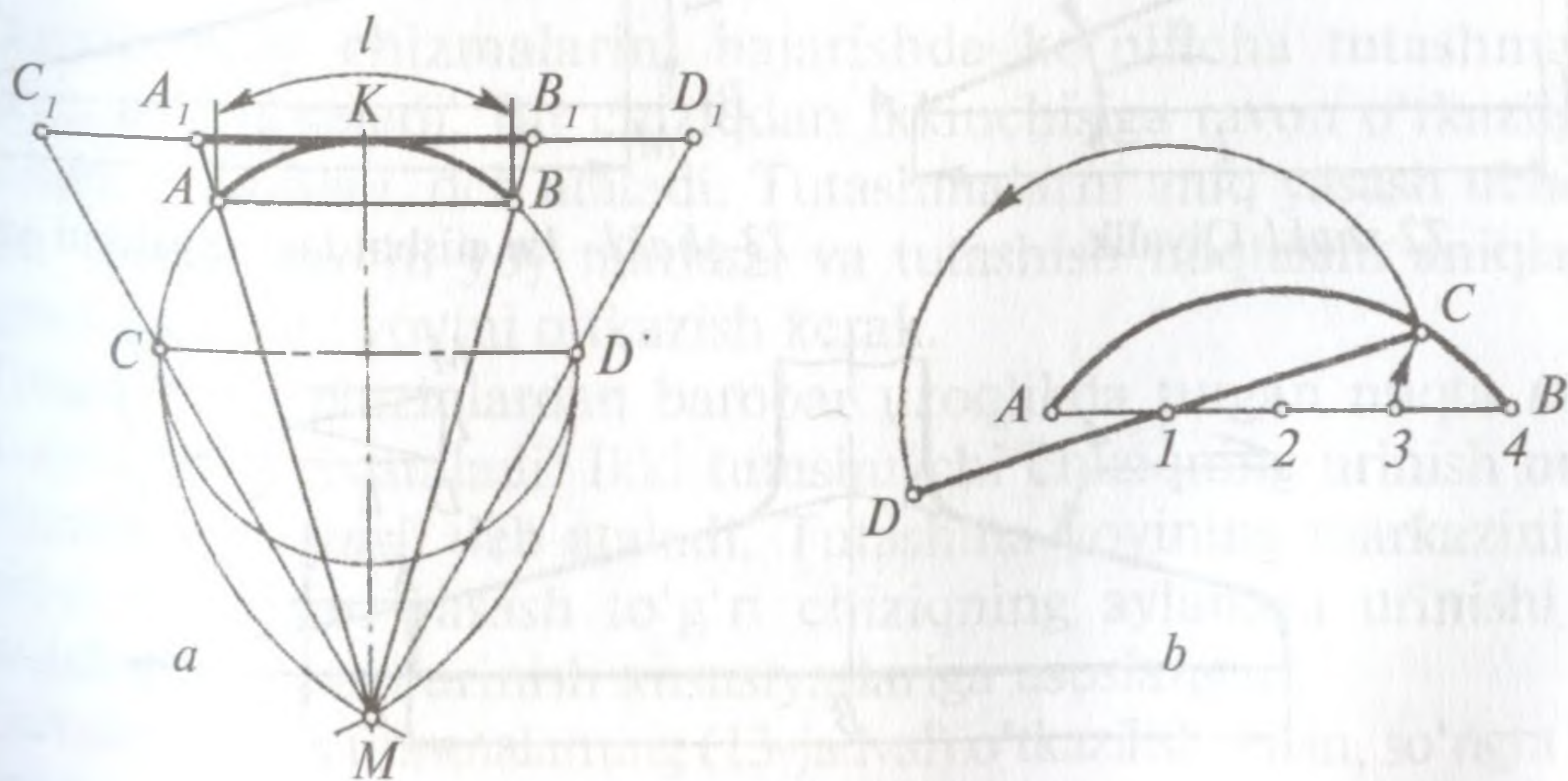
71-shakl. Aylana yoyini to'g'rilash.
