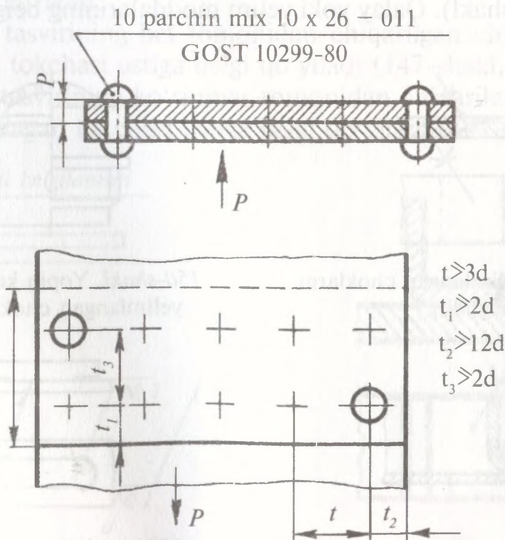
154-shakl. Ustma-ust parchin mixli birikmalar.
