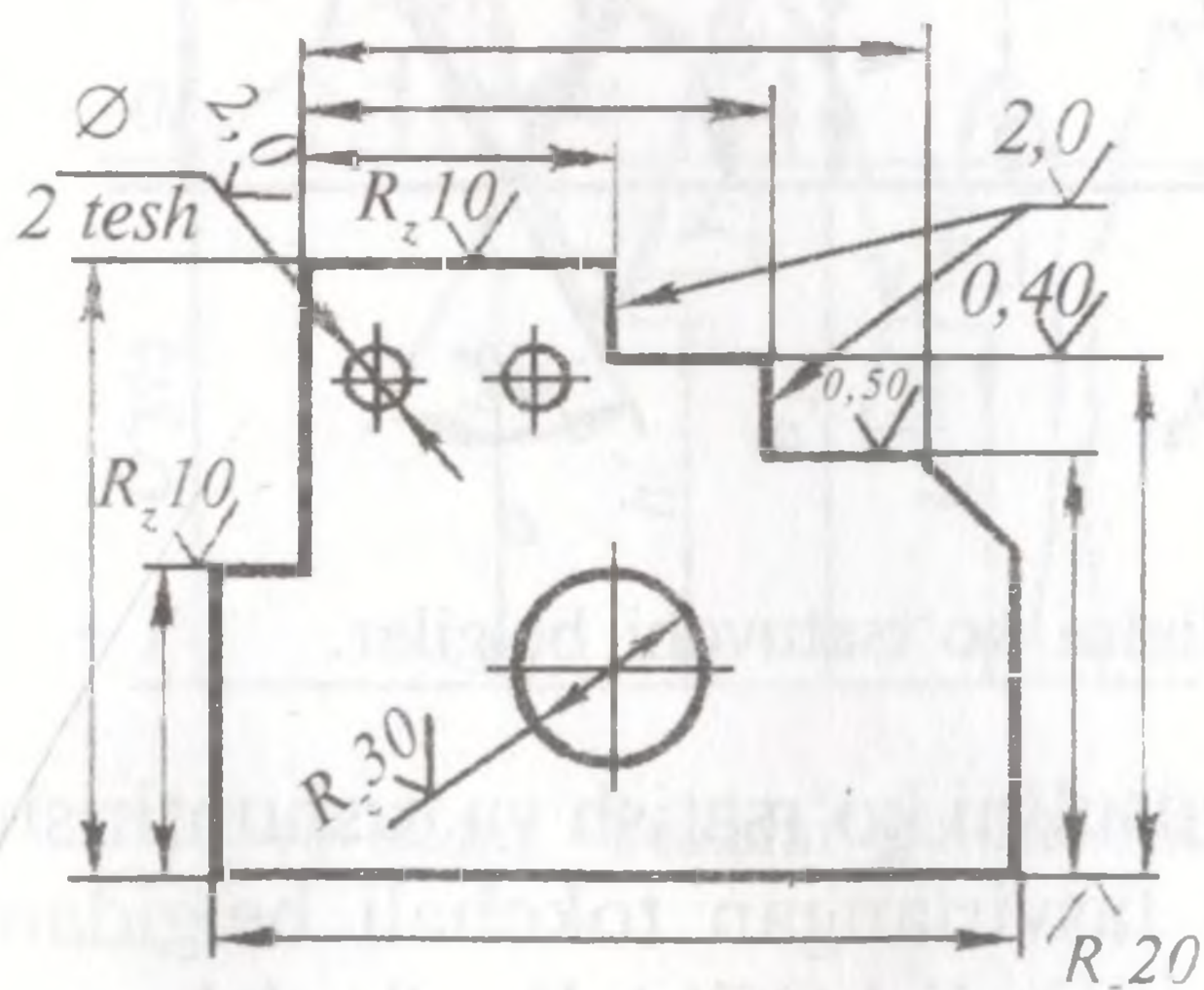
43-shakl. G'adir-budurlik parametrlarini va belgilarini chizmada tasvirlash.
