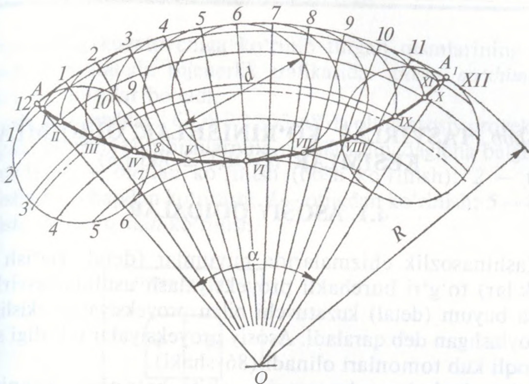
84-shakl. Episikloida yasash.
