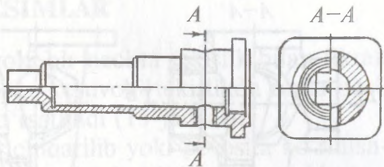
96-shakl. Bo'ylama va ko'ndalang qirqim.
