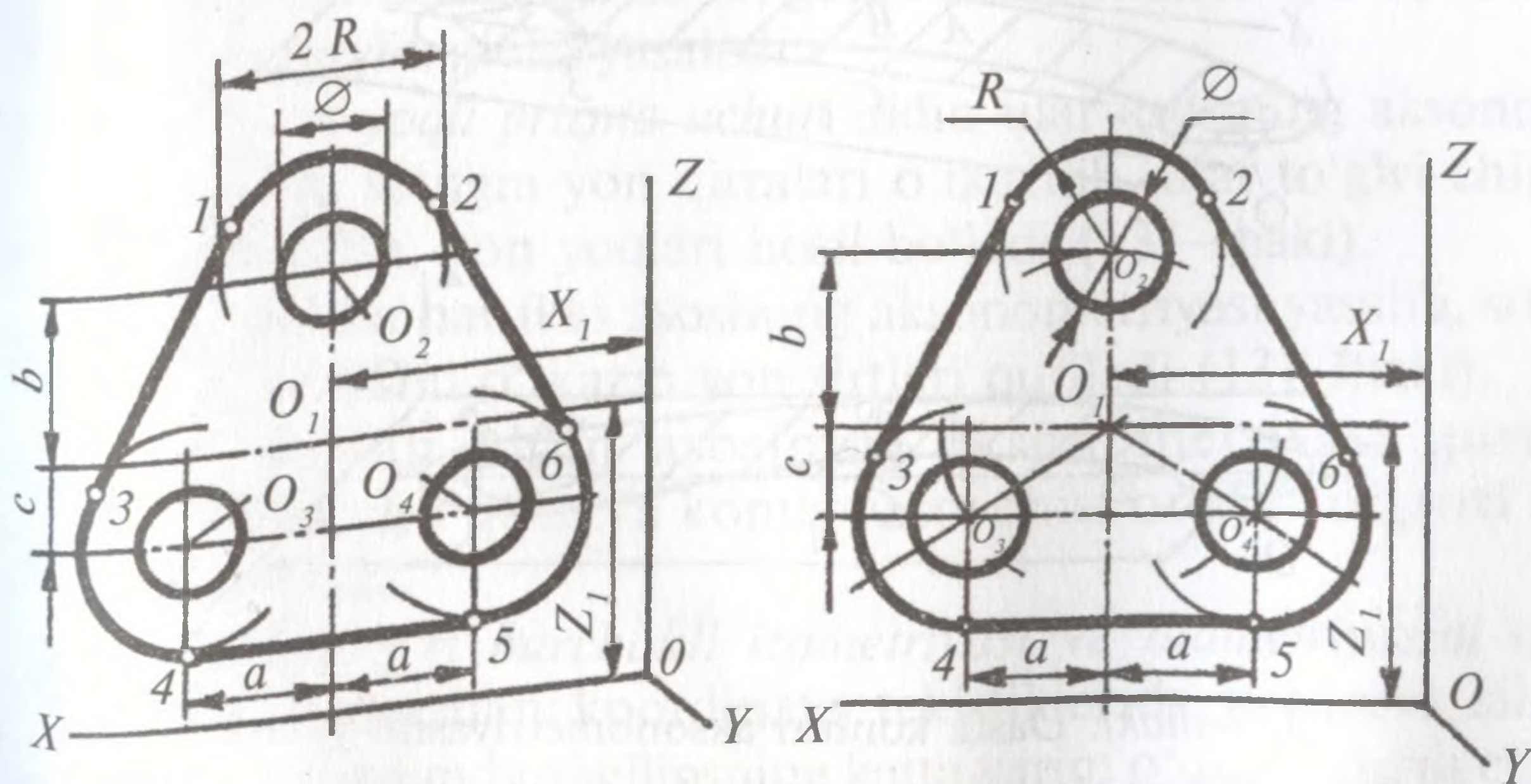
128-shakl. Flanes konturi aksonometriyasini yasash.
