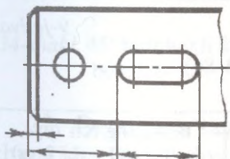
30-shakl. O'lchamlarni gruppalab tasvirlash.
