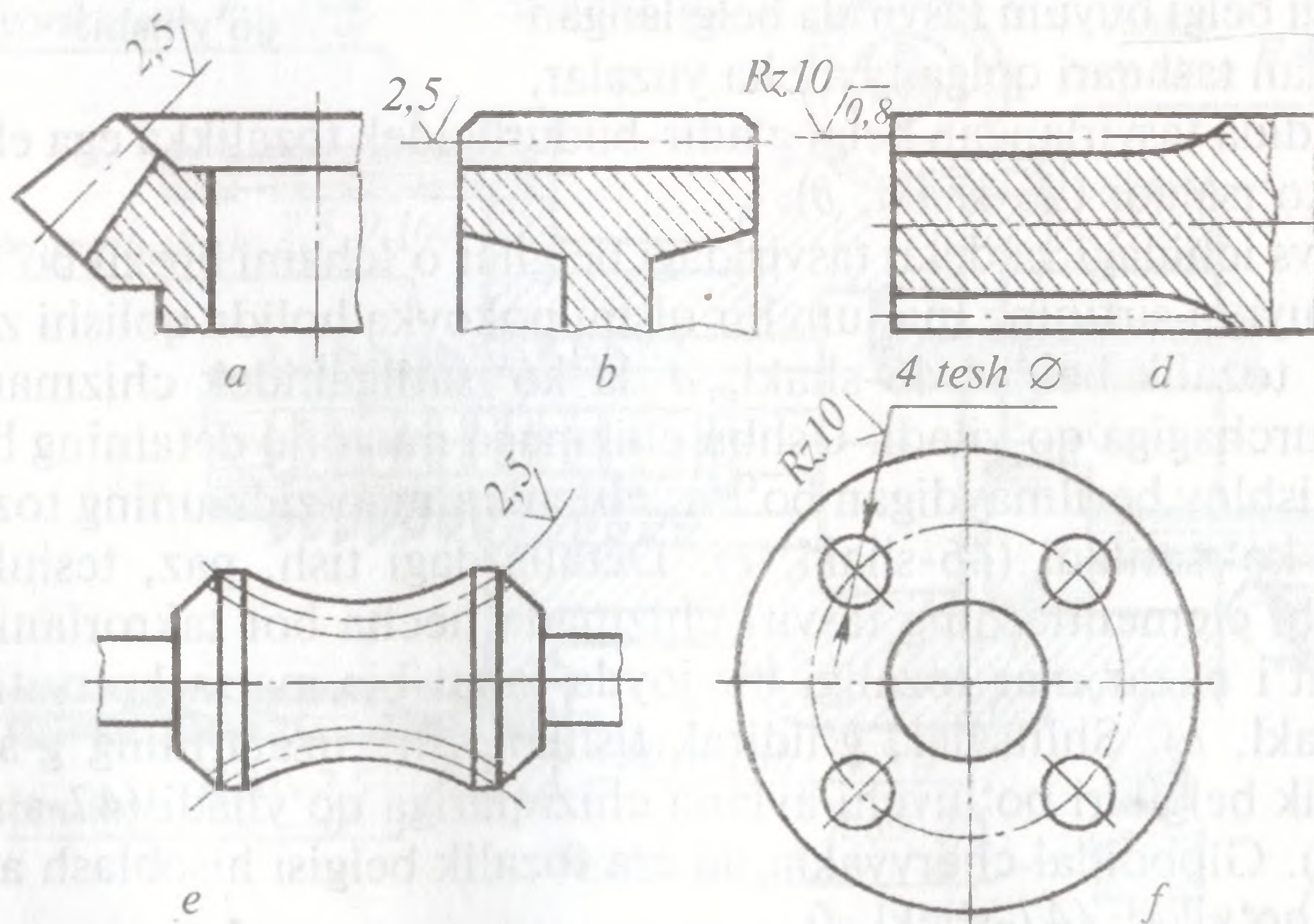
47-shakl. Takrorlanuvchi elementlar yuzalarining g'adir-budurligining belgilanishi.
