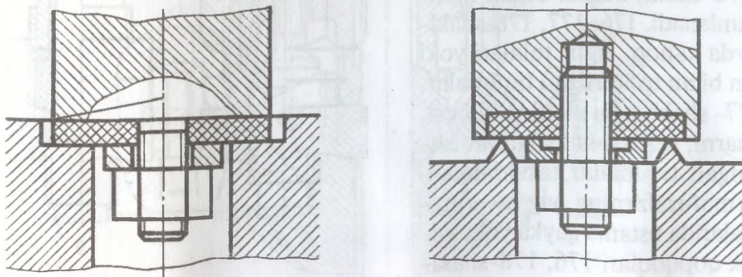
174-shakl. Yumshoq zichlagich halqalarni mahkamlash.
