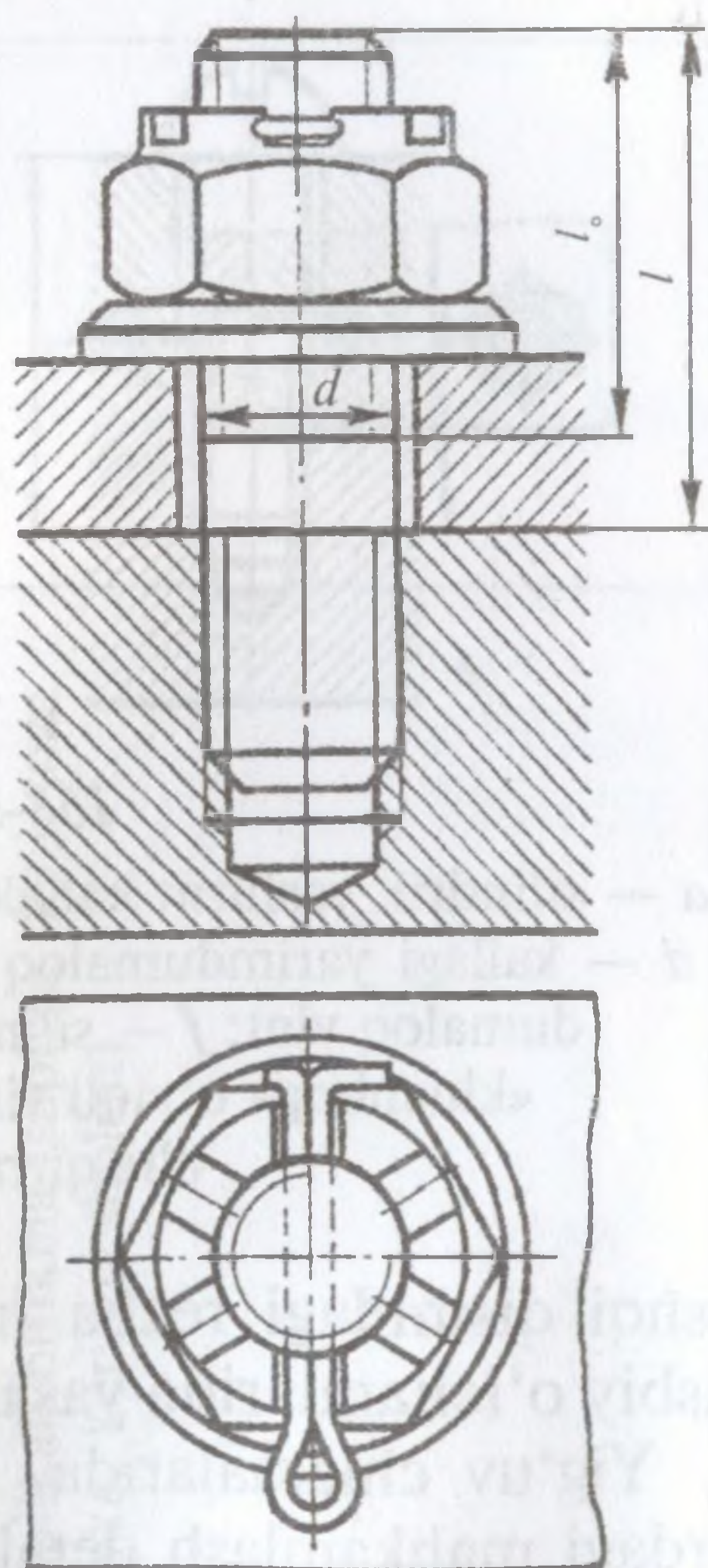
157-shakl. Shpilkali birikmalar.
