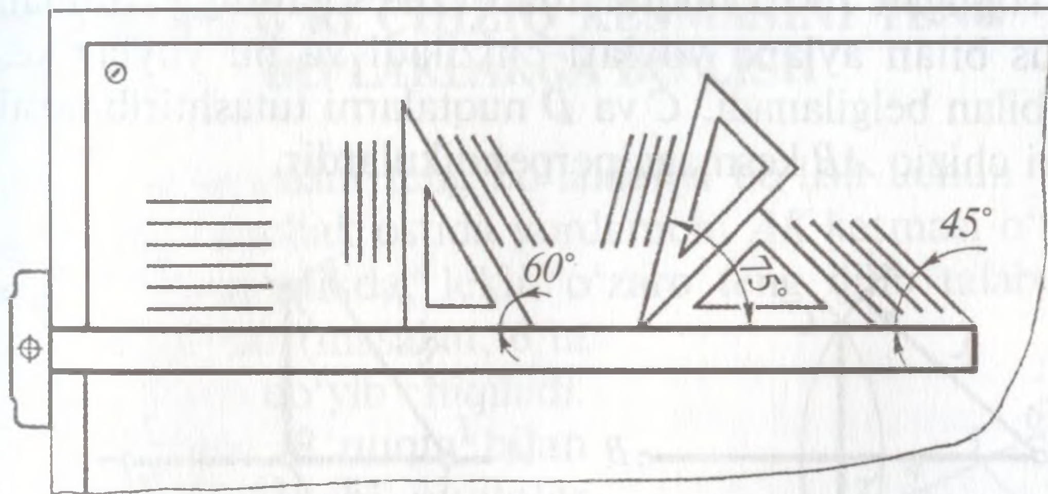
63-shakl. Turli qiyalikda parallel to'g'ri chiziqlar o'tkazish.
