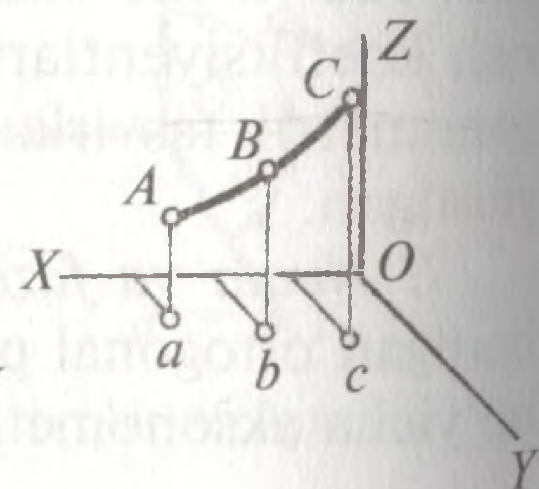
124-shakl. Fazoviy egri chiziq aksonometriyasini yasash.
