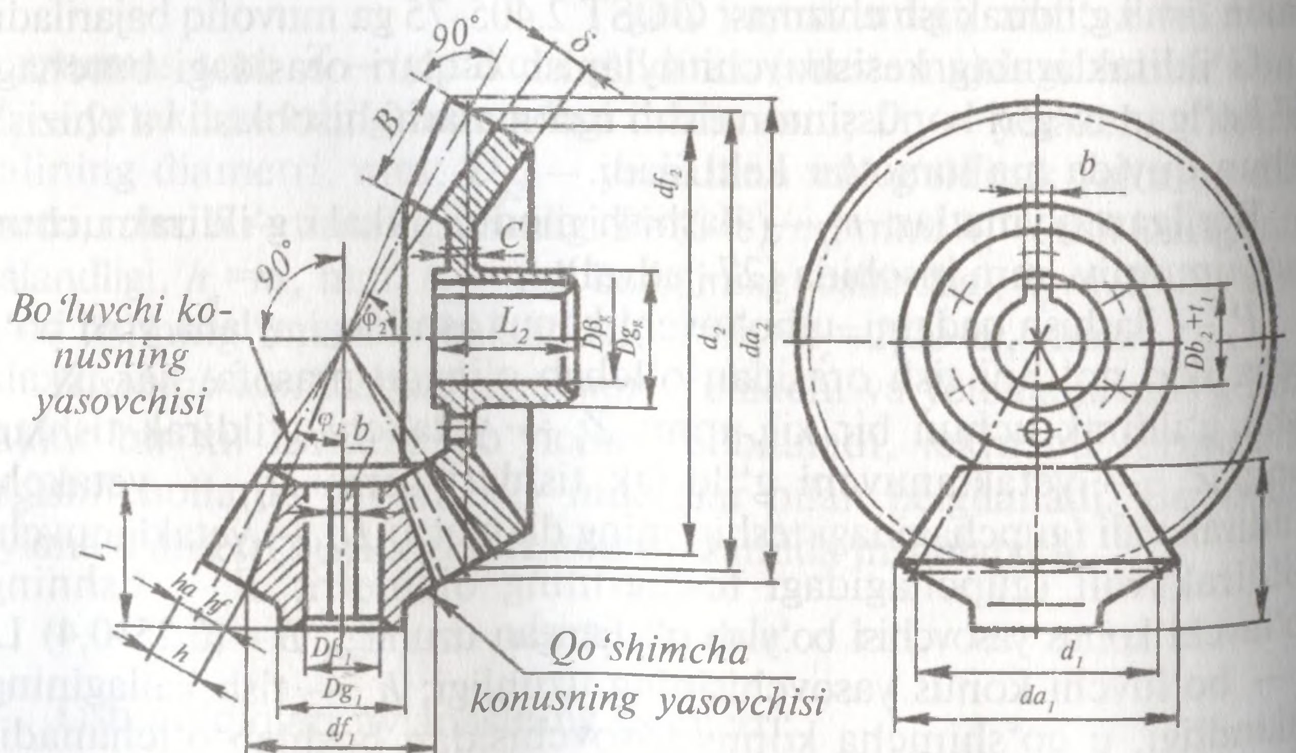
167-shakl. Konussimon tishli uzatmalar.
