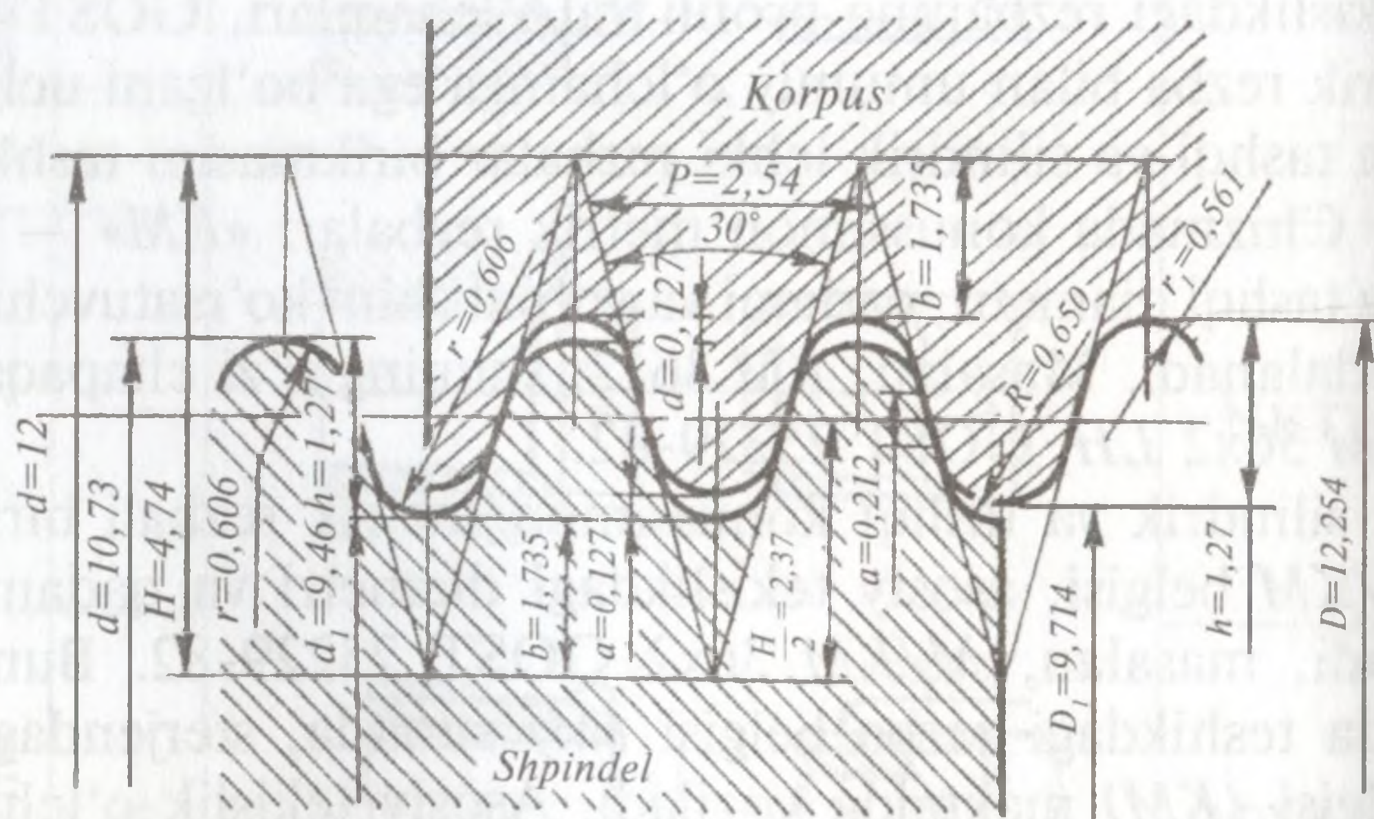
109-shakl. Yumaloq profilli rezbalar.
