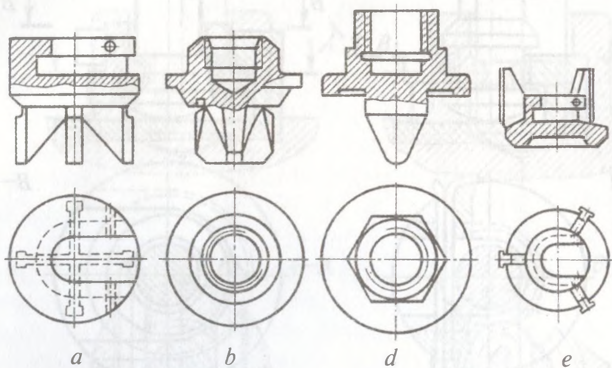
172-shakl. Korpus ichida zolotnikni yoʻnaltirish.
