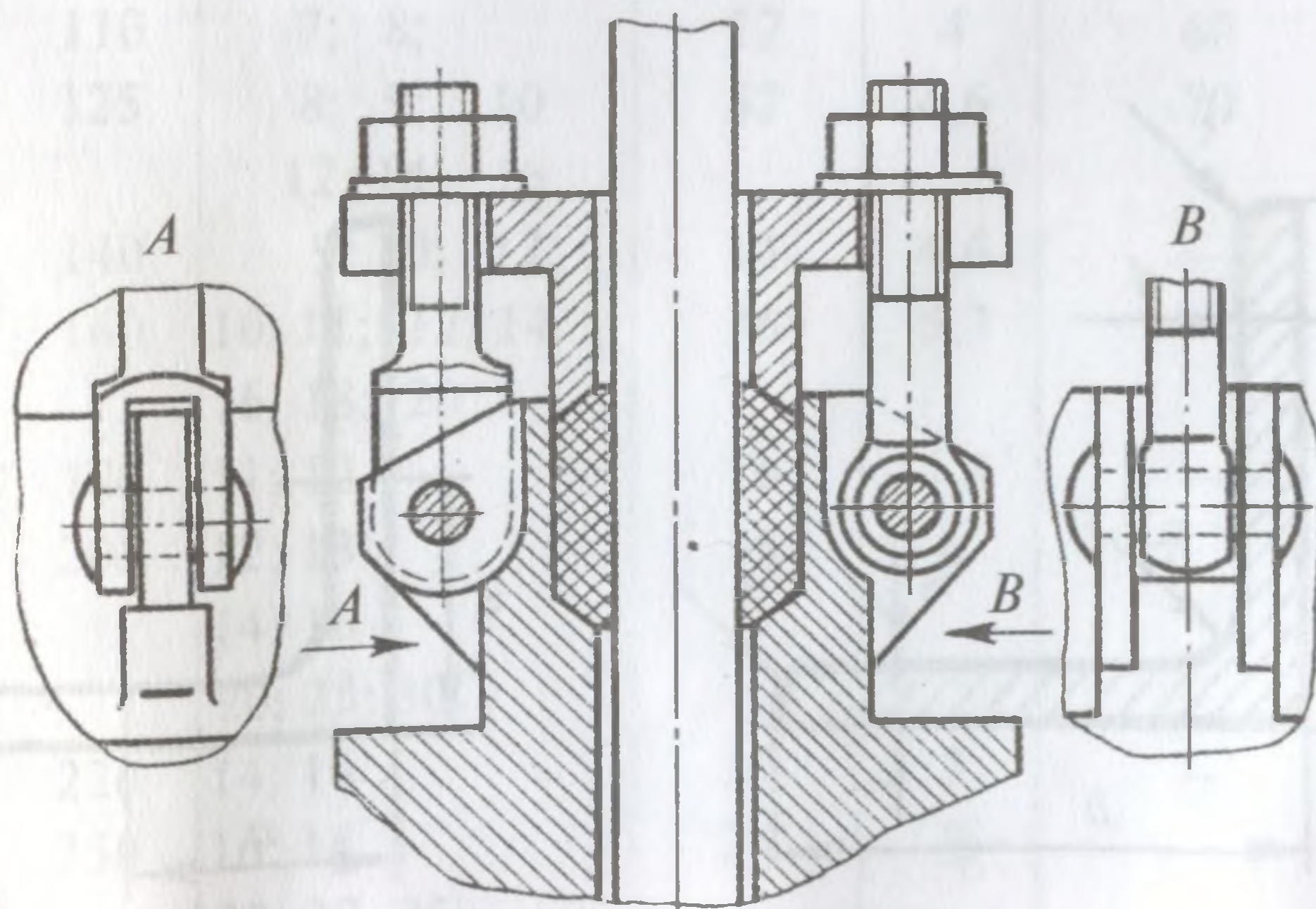
178-shakl. Salnik qopqog'ini tashlama boltlar vositasida mahkamlash.
