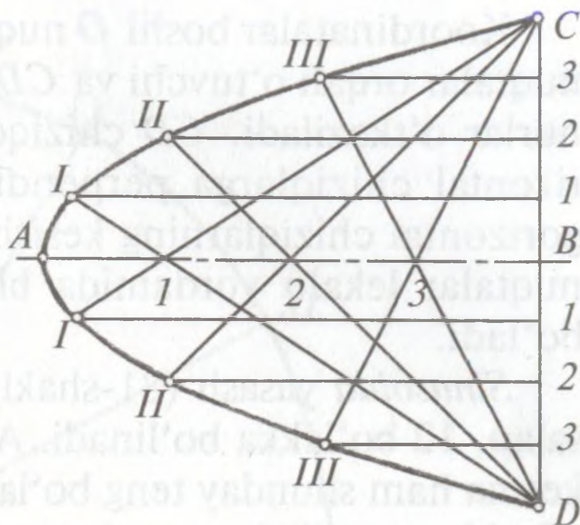
79-shakl. Parabola yasash.
