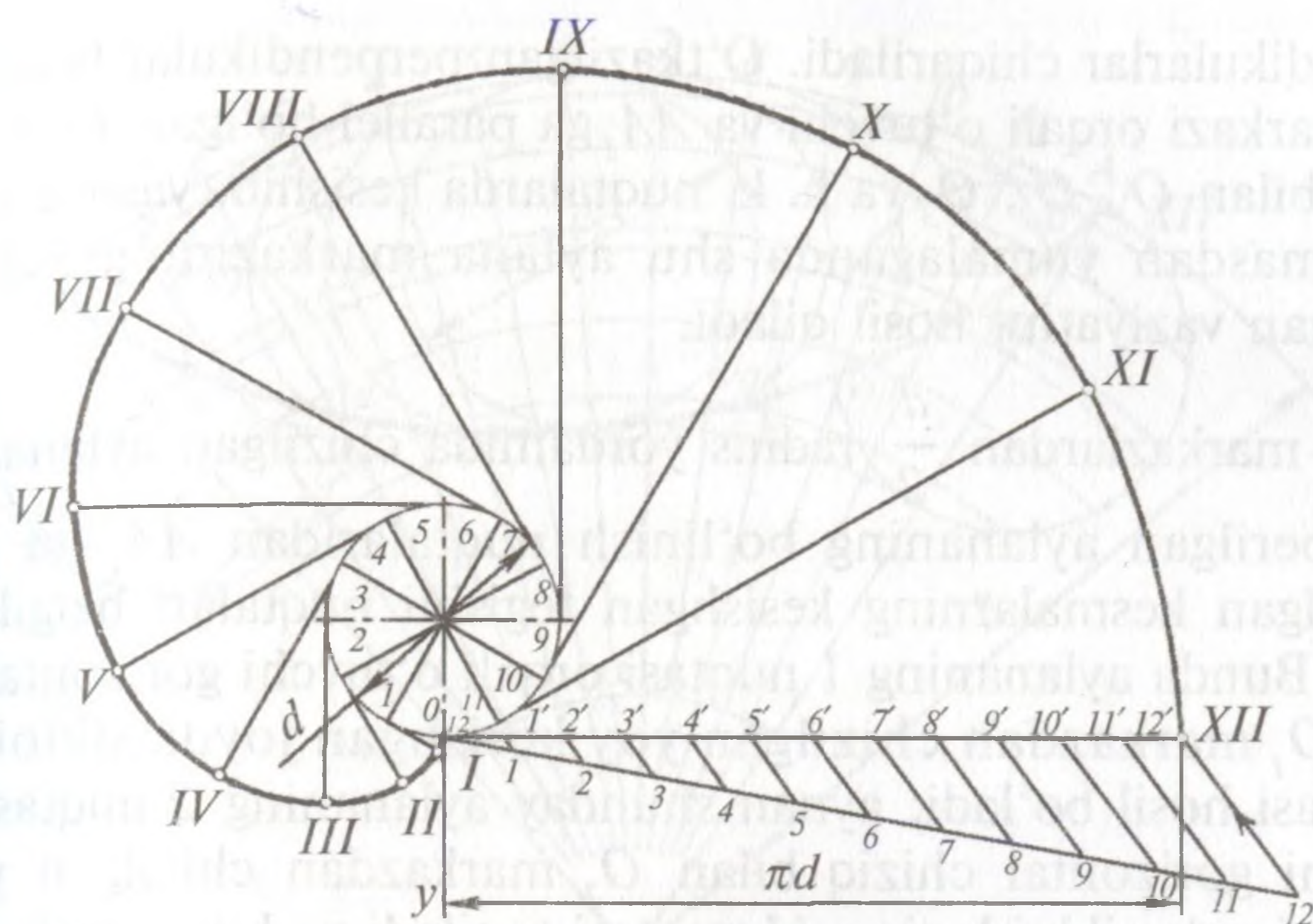
82-shakl. Aylana evolventasini yasash.
