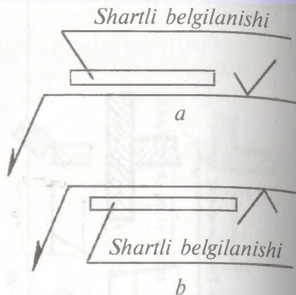
146-shakl. Payvand birikma choklariga tozalik belgilarini qo'yish.
