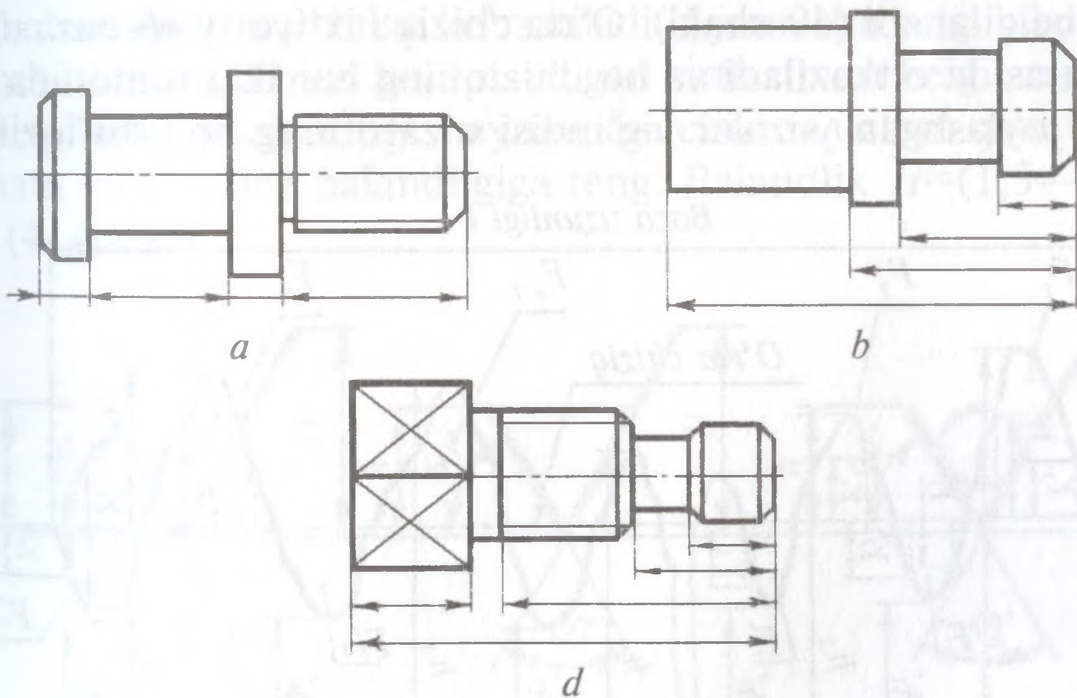
39-shakl. O'lcham qo'yish usullari.
