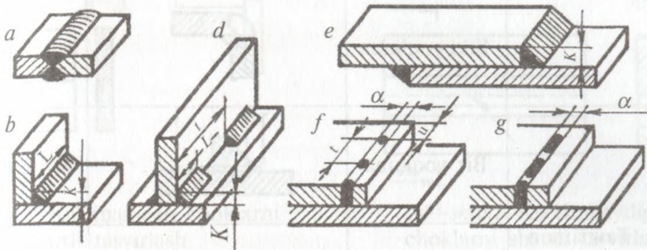
138-shakl. Payvand birikmalarning turlari.
