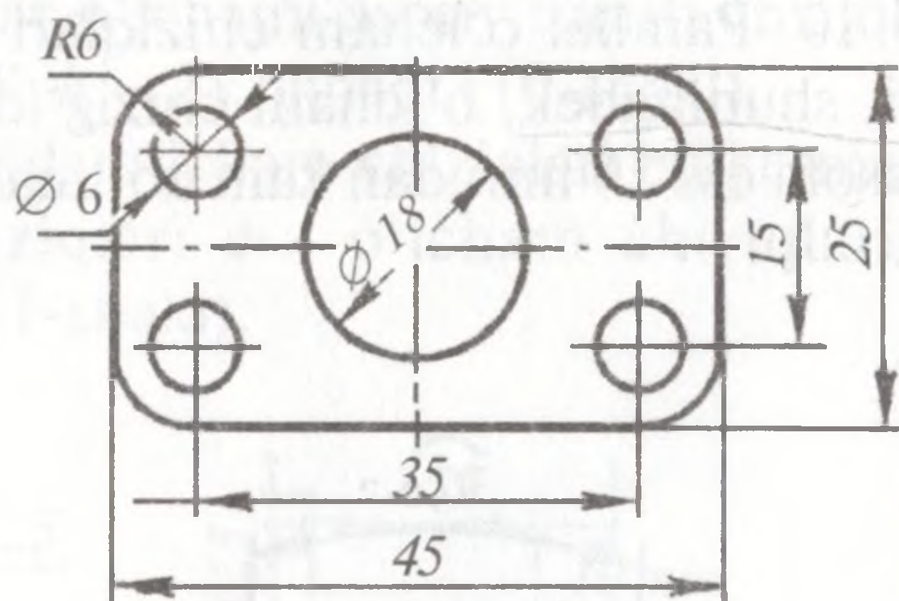
17-shakl. O'lchamlar qo'yish.
