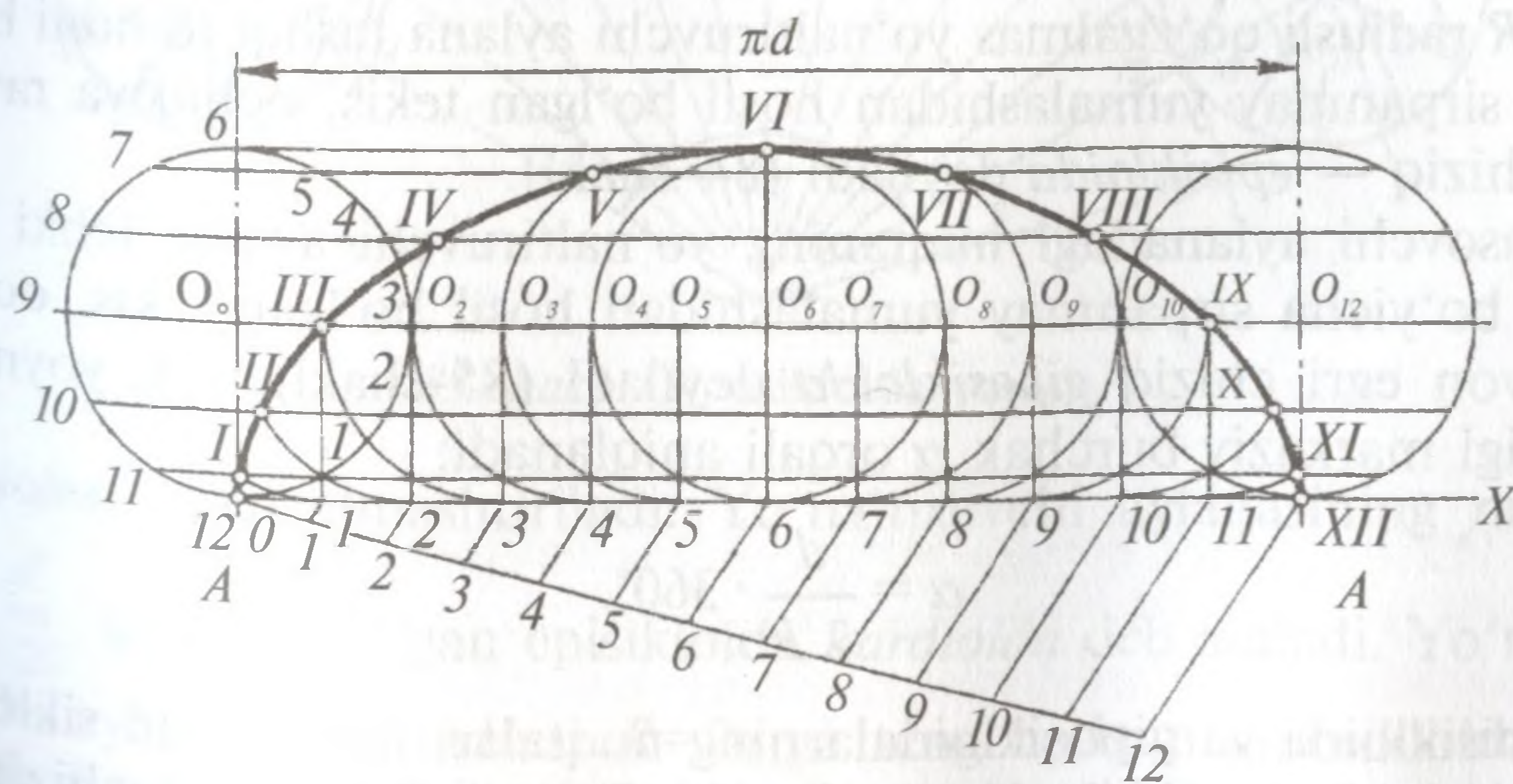
83-shakl. Sikloida yasash.
