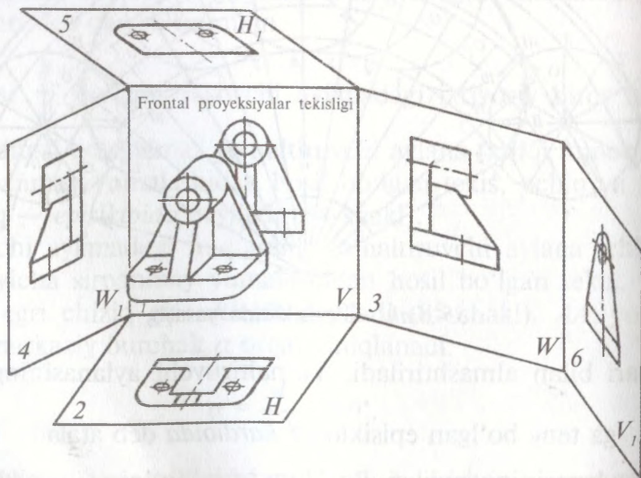
86-shakl. Buyumning asosiy proyeksiya tekisliklariga nisbatan joylashuvi.
