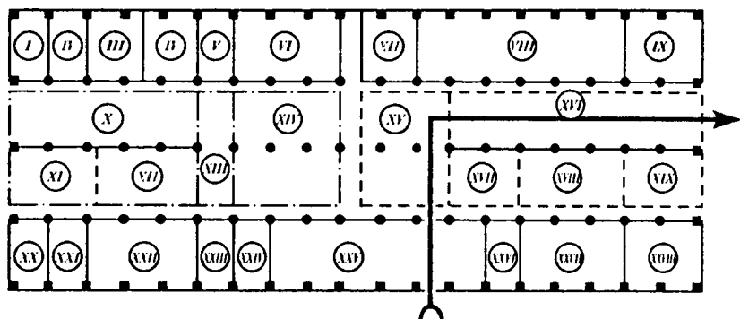
7.18-rasm. Traktorlarni ta'mirlash korxonasida ta'mirlash texnologik jarayonini Γ simon sxemali qilib joylashtirish:
