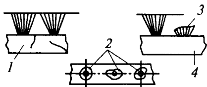
4.21 - rasm. Paxta terish apparatining cho'tkalarida sodir bo'ladigan nuqsonlar:
