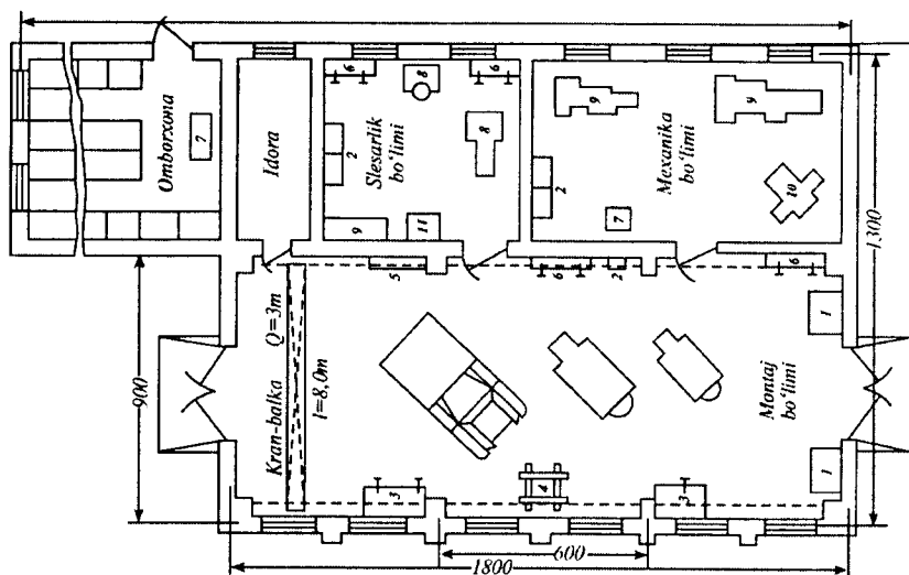
7.6 - rasm. Toshkent viloyati O'rtacha Chirchiq tumanidagi «Kim Pen Xva» shirkati xo'jaligi ustaxonasining rejas (30 ta traktorga mo'ljallangan).
