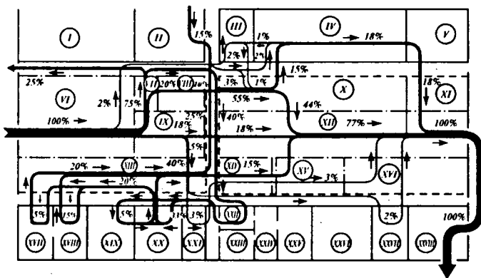
7.17-rasm. Traktorlarni ta'mirlash korxonasida texnologik jarayon to'g'ri chiziqli yuk oqimli va to'g'ri sxemali qilib joylashtirish:
