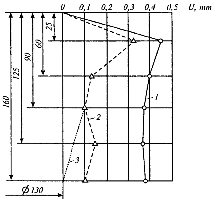
6. 7- r a s m. A—01M rusumli dvigatel silindr gilzalarining balandligi bo'yicha yeyilish grafiqi:
