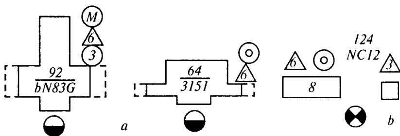
7.10-rasm. Jihozlarni raqamlash namunalari, ishchi joylarining va turli tarmoqlarning belgilanishi
