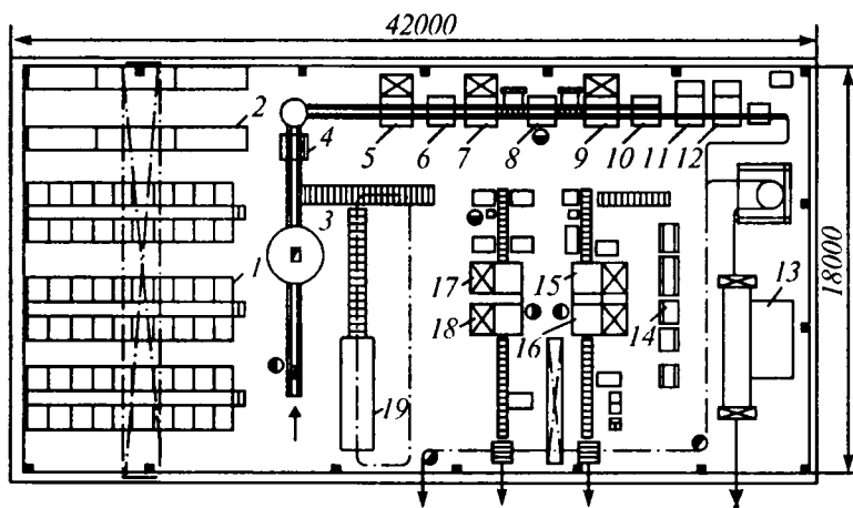
7.12-rasm. Traktor dvigatellarini ta'mirlash maxsus korxonasining yuvish, qismlarga ajratish bo'limining rejasi varianti:
