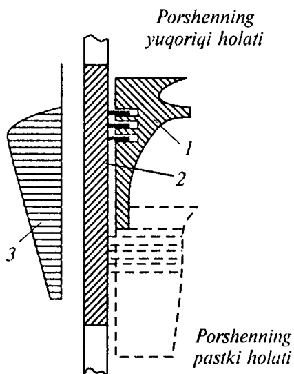
6.6- r a s m. Silindr gilzalarining yeyilish grafigi:
