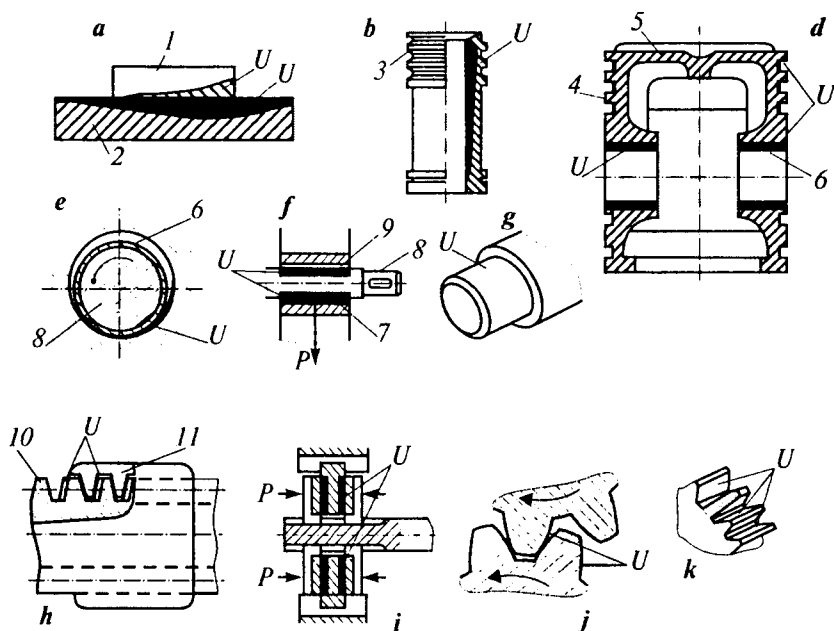
1.12- ras m. Mashina detallarining mexanik yeyilish namunalari:
