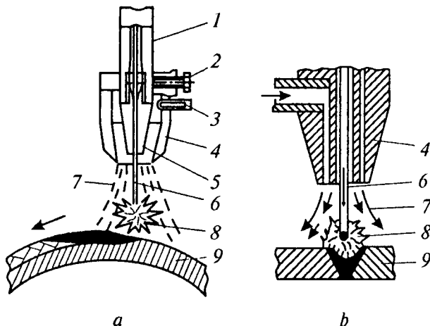
5.9- r a s m . Silindrik buyumlarni karbonat angidrid gazı muhitida mexanizatsiyalashtirilgan usulda suyltirib qoplash va tekis buyumni payvandlash sxemasi:
