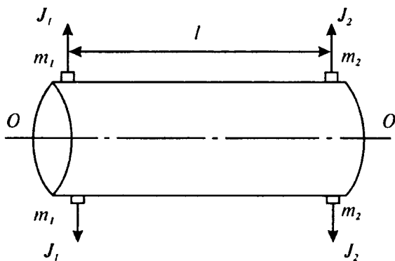
4.31-rasm. Detallarni dinamik muvozanatlash sxemasi.
