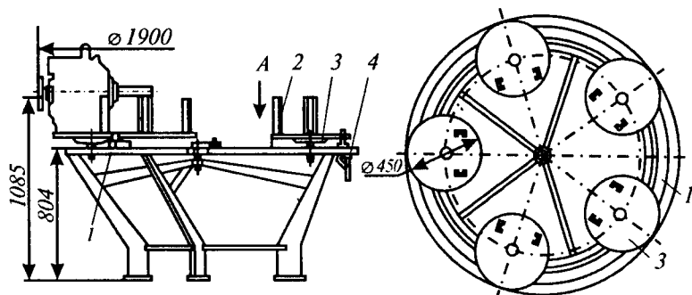
4.12 - rasm. Uzatmalar qutisini qismlarga ajratish stendi: 1 — burilma stol; 2 — uzatmalar qutisini oʻrnatish uchun kronshteyn; 3 — disk ustunlar bilan birga aylanadigan disklar; 4 — mahkamlash qurilmasi.
