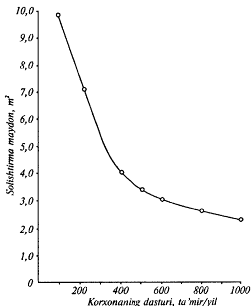
7.1-r a s m . Ta'mirlash ustaxonasi maydonining korxona dasturiga bog'liqligi.
