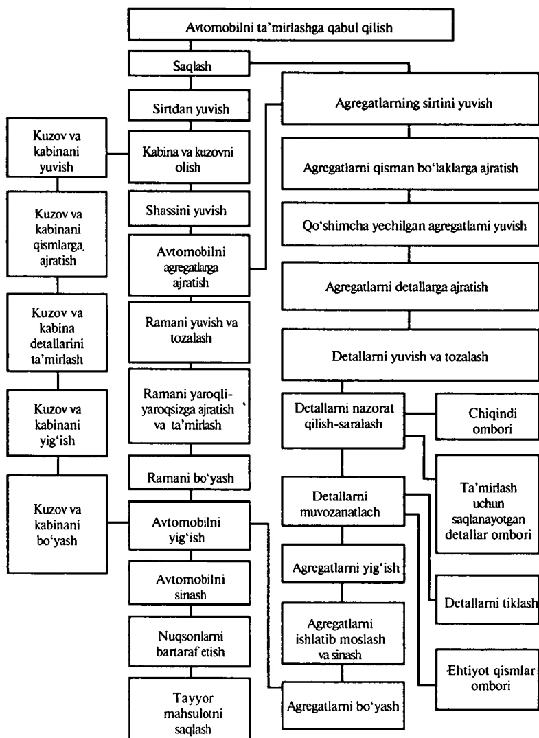
4.2 - r a s m . Yuk avtomobillarini ta'mirlash texnologik jarayonining sxemasi.
