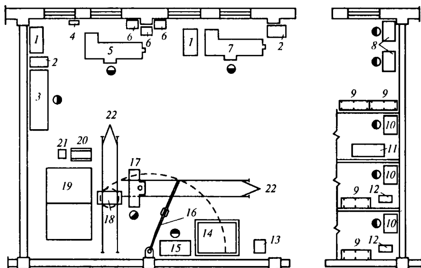
7.9-rasm. Payvandlash va qoplash bo'limining rejası namunası:
