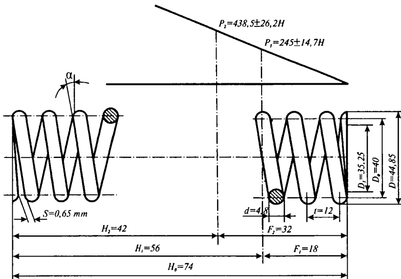
6.24-rasm. A-01M , A-41 , YMZ , SMD rusumli ichki yonuv dvigatellarining gaz taqsimlash mexanizmi klapan prujinasining texnik koʻrsatkichlari:
