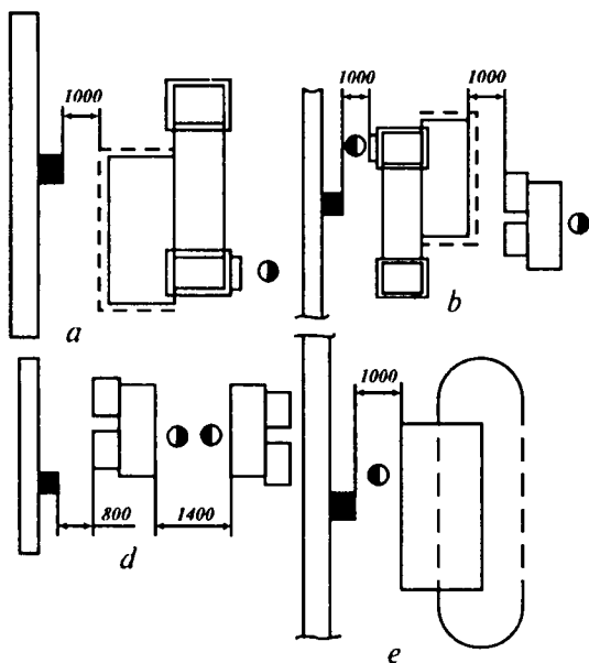
7.15 - r a s m . Yuvish jihozlarini joylashtirish sxemasi:
