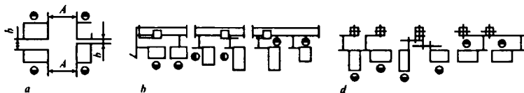
7.11-rasm. Dastgohlarning bino elementlariga nisbatan joylashish sxemalari va oraliq masofalari:
