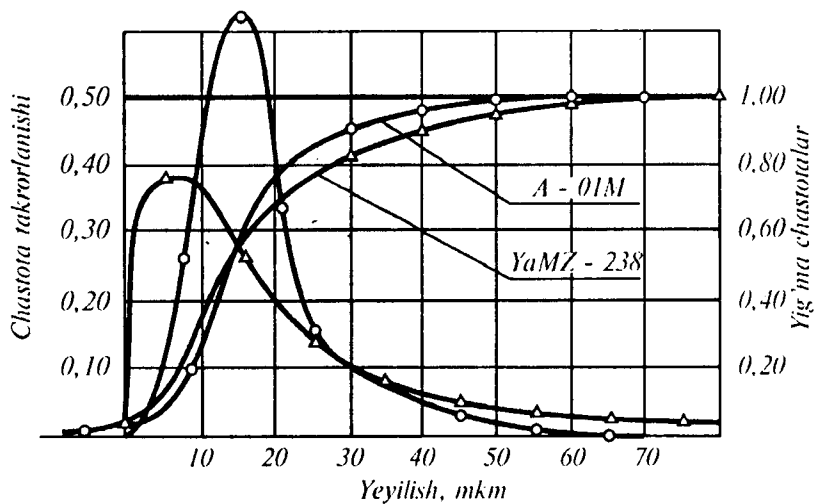
6.18-r a s m . Butkul ta'mirlashga kelgan A- 01M va YM3-238 dvigatellari' porshen barmoqlari o'qchamlarining tarqalish grafigi.
