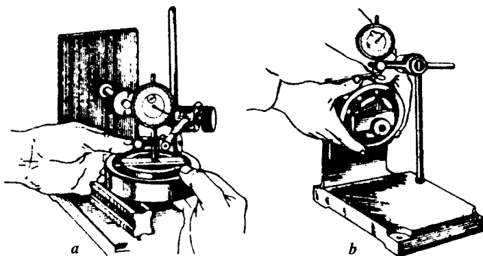
4.28 - rasm. Dumalanish podshipniklaridagi tirqishlarni indikator bilan o'lchash: a — o'q yo'nalishidagi tirqishni o'lchash; b — radial tirqishni o'lchash.
