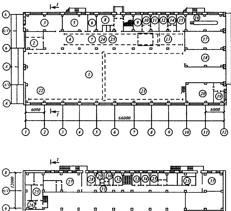
7.20 - rasm. Xo'jalikning markaziy ta'mirlash ustaxonasi bo'limlarini joylashtirish rejası:
