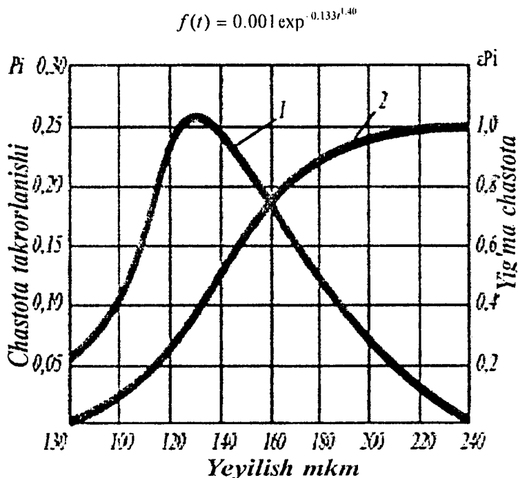
6.9-rasm. A—01M va YMZ—236 rusumli dvigatellar silindr gilzalari ichki yuzasi yeyilish qiymatlarining taqsimlanish egri chizig'i: ko'rsatkichlar tarqalishining differensial (1) va integral (2) egri chizig'i.
