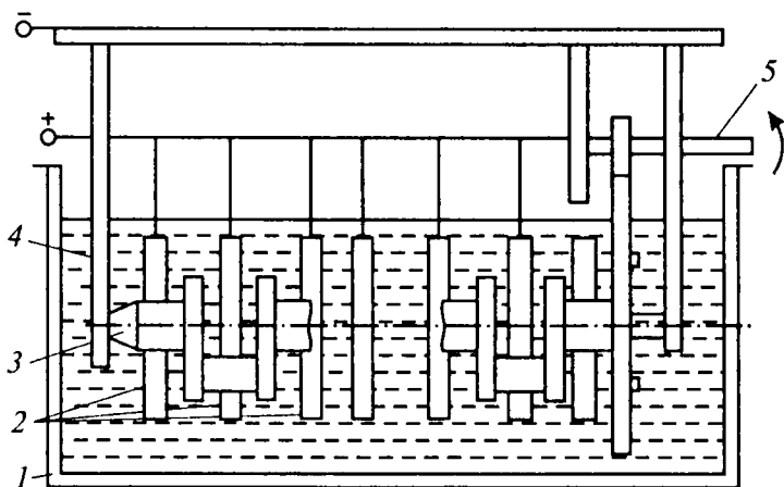
6.30-rasm. Tirsakli vallarni ta'mirlash (po'latlash) uchun qurilma sxemasi:
