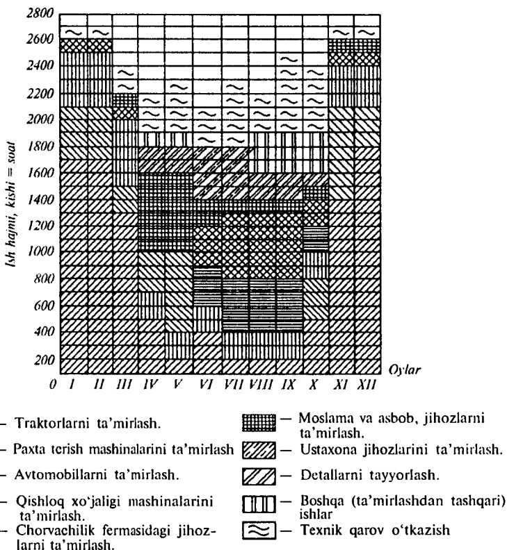
7.3 - r a s m. Ustaxonani ish bilan ta'minlash grafigi
