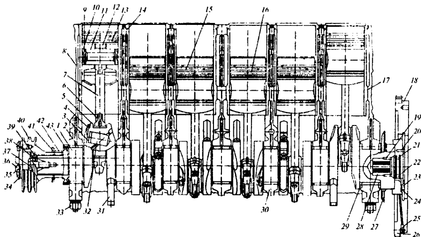
6.13 - ras m. A-01M dvigateli krivoship-shatun mexanizmi:
