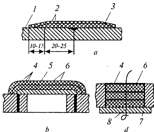
5.19-rasm. Detallarning yorilgan joyini ustqo'yma o'rnatib berkitish:
