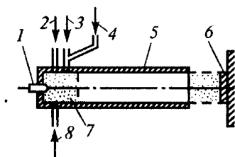
5.15- rasm. Detonatsion purkash sxemasi:
