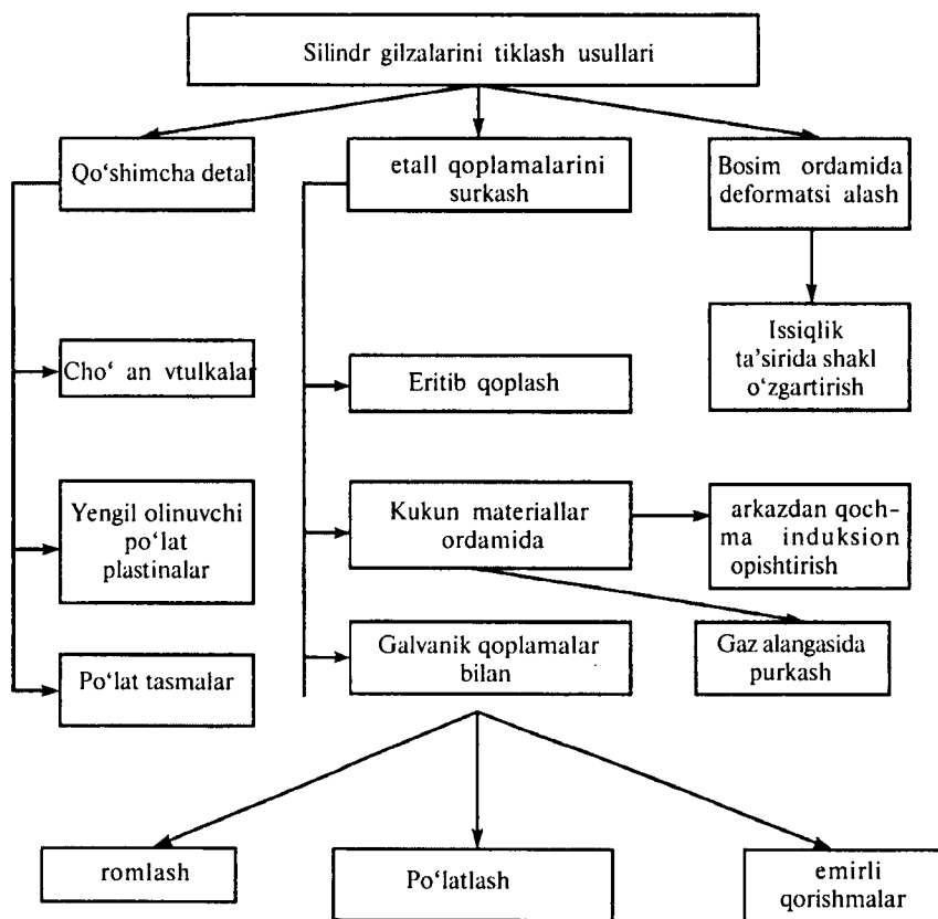
6.8 - rasm. Dvigatellar silindrlari gilzalarini tiklash usullarining tasnifi.
