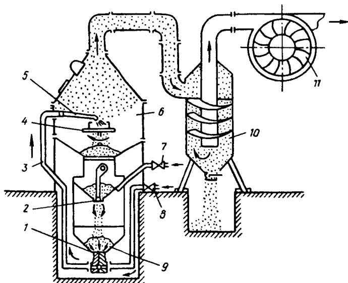
4.10 - r a s m. Detallarni danak kukunlari bilan tozalash uskunasi:
