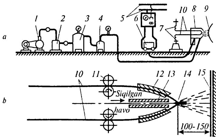
5.16-rasm. Elektryoyli metallash uskunasi va elektrmetallizatorning sxemasi:
