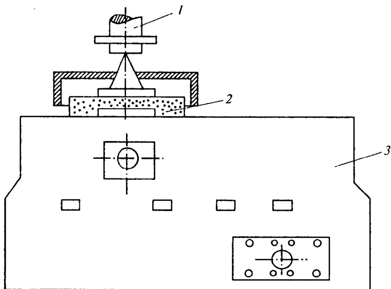
6.4- ras m. Silindrlar blokni silliqlovchi moslama:
