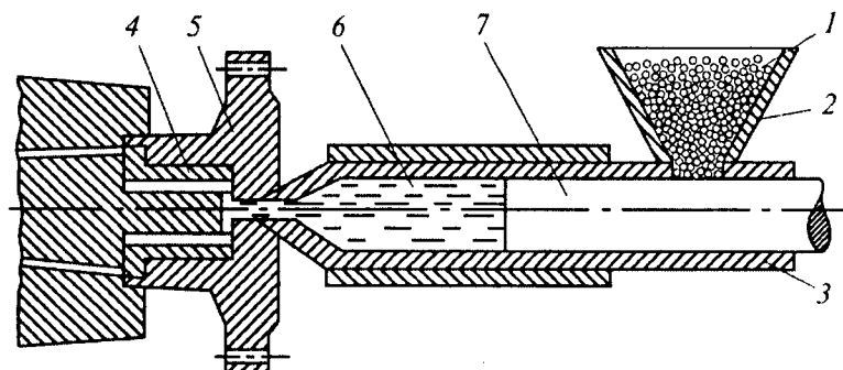
5.21-r a s m . Detallarni bosim ostida quyish usulida tiklash sxemasi:
