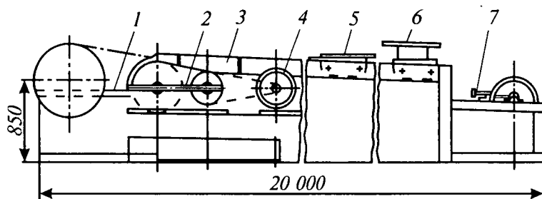
4.11-rasm. Agregatlarni qismlarga ajratish uchun konveyer:
