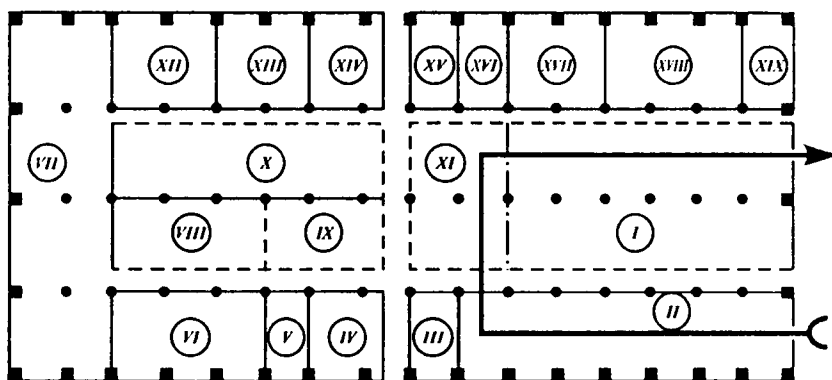
7.19-rasm. Dvigatellarni ta'mirlash bo'limining texnologik jarayonini joylashtirish ko'rinishi (Π simon yuk oqimi):
