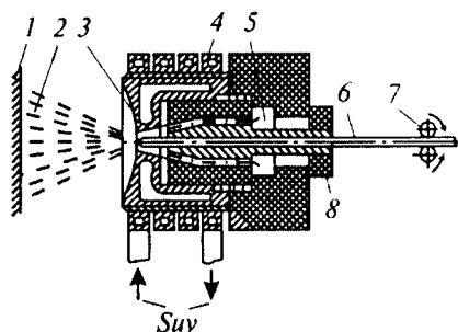
5.14-r a s m. Yuqori chastotali purkash apparatining tuzilishi (purkash) kallagi:
