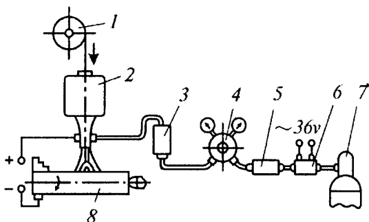
5.5-rasm. Karbonat angidrid gazi muhitida elektr yoy bilan suyultirib qoplash uskunasining sxemasi:
