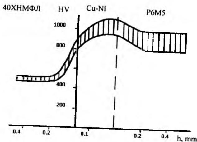
12.17-rasm. Tezkesar po‘lat P6M5-po‘lat 40XHMΦ kompozitsiyasining ko‘ndalang kesiml bo‘yicha mikroqattiqligi taqsimlanishi
