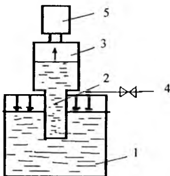
7.41-rasm. Past bosim bilan quyish sxemasi: 1. Eritish pechi, 2. Metall quvvur, 3. Shakl, 4. Siqilgan havo oqimi, 5. Ventilyasiya tuynugi. Past bosimda quyish texnologiyasida siqilgan havoning bosimini o'zgartirish bilan formalarni to'ldirish tezligini o'zgartirish mumkin.
