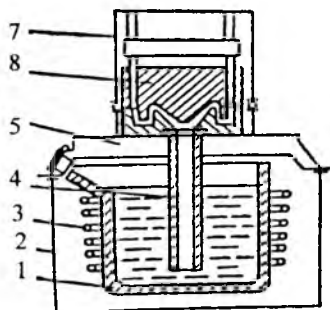
7.42-rasm. Bosim qarshiligi usulida quyish sxemasi: 1-tigel; 2-pechning germetik qoplamasi; 3-qizdirgichlar; 4-metalo'tkazgich; 5-qopqog; 6-press shakl; 7 - press shaklning germetik qobig'i. Bu usulda quymalarning sirtlarini tozaligi oshadi, mexanik xossalari yaxshilanadi, g'ovaklari bartaraf etiladi.
