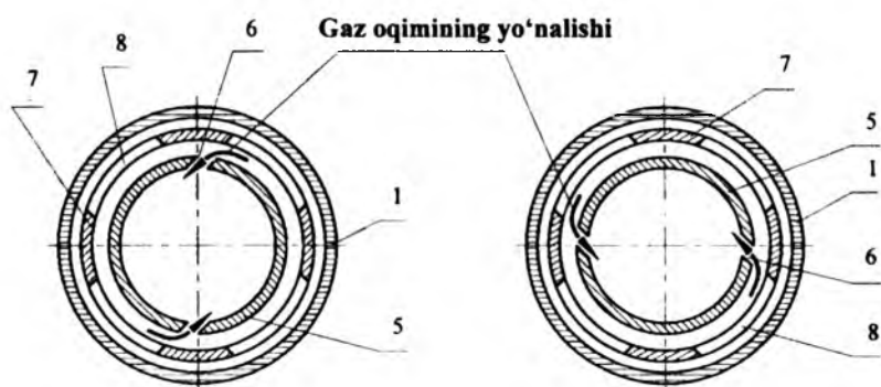
12.2-rasm. Yangi tipdagi plazmakimyoviy reaktor: 1-korpus; 2-plazmagenerator; 3-koaksial tirqishlar; 4-soplo; 5,7-silindrlar; 6-teshik; 8-kesik; 9-elektrokalfifer; 10-chiqish teshiklari.
