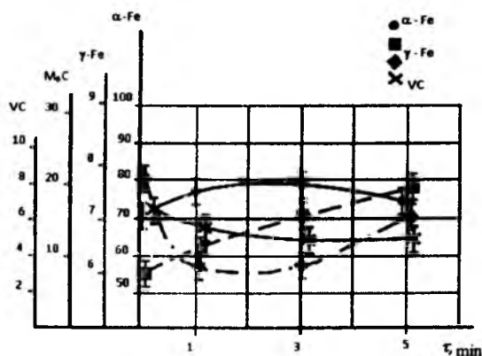
12.14-rasm. Tezkesar po'lat P6M5 faza tarkibining o'zgarish grafigi, izotermik tutib turish temperaturasi 350^\circ\text{C}
