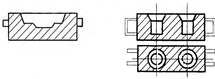
7.2-rasm. Gorizontaal ajralish chizig‘i va kombinatsiyalangan ajralish chizig‘iga ega kokillar sxemasi.
