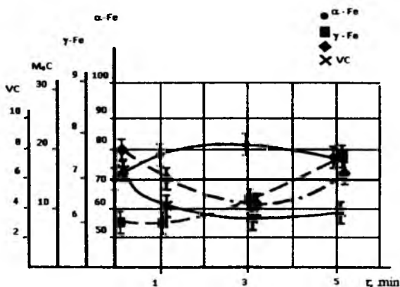
12.13-rasm. Tezkesar po'lat P6M5 faza tarkibining o'zgarish grafiği, izotermik tutish temperaturasi 280°C.
