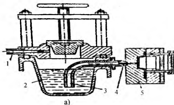
7.14-rasm. Kuchstz bosim ostida quyma quyish sxemasi.
