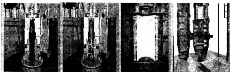
12.1-rasm. ПУБ-300 plazmakimyoviy qurilmasi va uning ishlash prinsipi:
