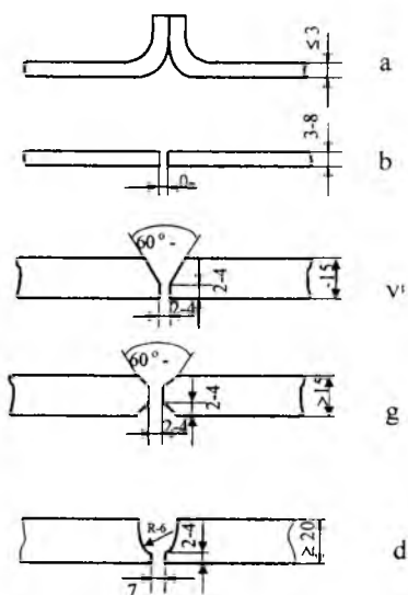
9.6-rasm. Metallarni elektr yordamida payvandlashda qalinligiga ko‘ra chetlarini
