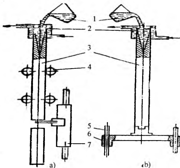
7.48-rasm. Uzlüksiz quyish va yarim uzluksiz quyish sxemasi: 1-cho'mich (kovsh), 2-suv sovutiluvchi kristalizator, 3-profil tayyorlamasi, 4-tortuvchi roliklar, 5-yo'naltiruvchilar, 6-travers, 7-tayyorlamalar kesuvchi arra.
