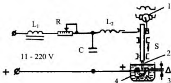
12.30-rasm. Elektr uchkunli usulda ishlash sxemasi: 1-elektir dvigatel; 2-asbob; 3-zagotovka; 4-vanna.
