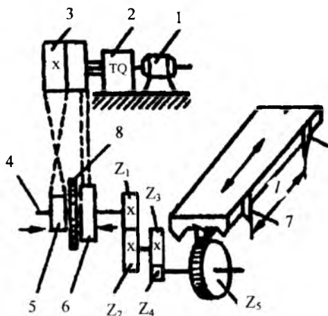
10.8-rasm. Bo'ylama randalash dastgohi harakatlanadi, shkvivlar ichiga elektromagnitlar joylashtirilgan.
