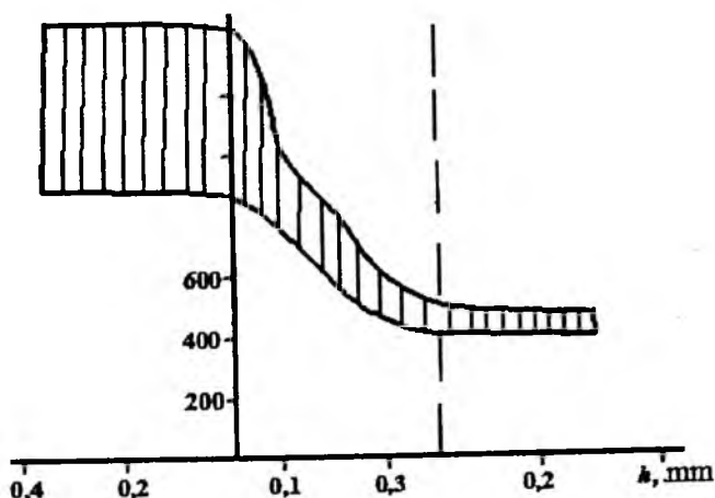
12.27-rasm. Molibden asosidagi MoTiC-po'lat40X kompozitsiyasi termik ishlangan keyingi ko'ndalang kesimi bo'yicha mikroqattqligining taqsimlanishi.
