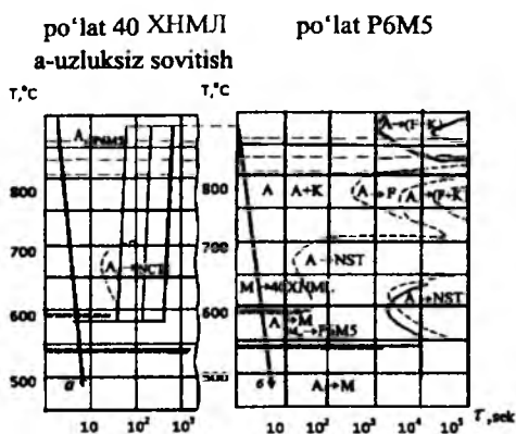
12.12-rasm. Tezkesar po'lat P6M5-po'lat 40XHMΦ kompozitsiyasini termik ishlash rejimlari:
