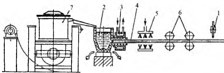
7.50-rasm. Bronzaning uzluksiz quyish gorizontall mashinasi.
