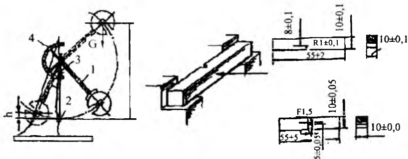
1.6-rasm. Mayatnikli kopyor va namuna.
