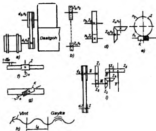
10.4-rasm. Pog'onali uzatmalar: a – tasmali; b – zanjirli; v – tishli; g – shnekli; d – reyka va reyka tishili g'ildirak; e – reyka va reykali shnek; yo – vintli; j – kinematik zanjir.
