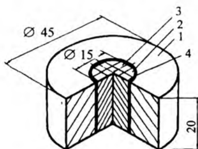
12.29-rasm. Kompozitsiyada qoldiq ichki kuchlanishlarni aniqlash va tengodatchiklarni yopishtirish chizmasi: 1- quyma tana; 2-quyilma; 3-tengodatchik ПДВ - 10/100, 4-o'tish qatlami.
