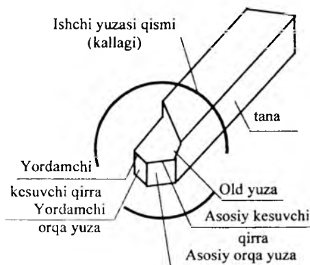
10.2.-rasm. Keskichning asosiy qismlari.
