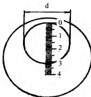
1.2-rasm.Brinnell lupasi.
