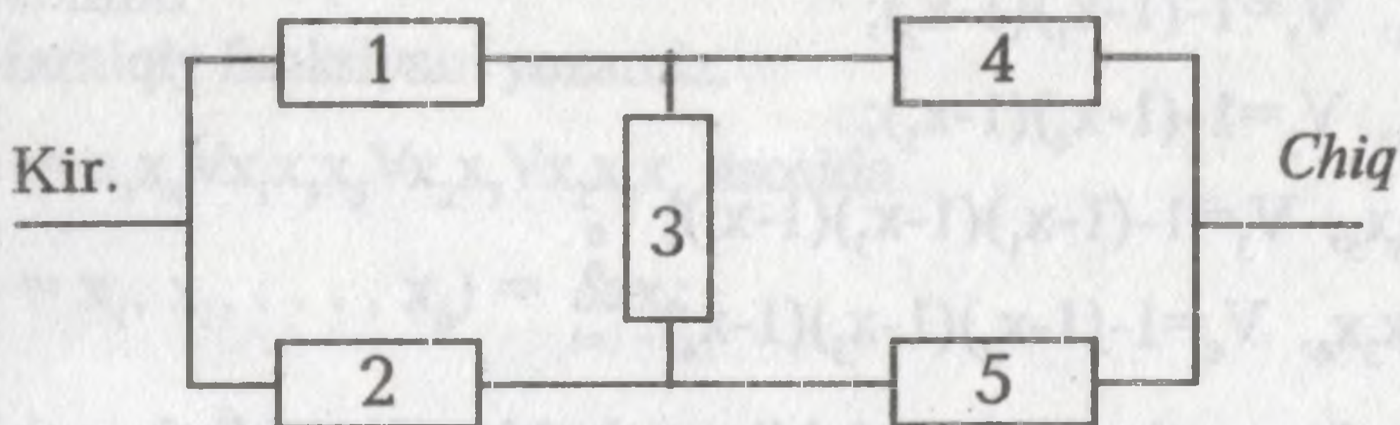
4.1-rasm. Most (ko'prik) sxemasi
