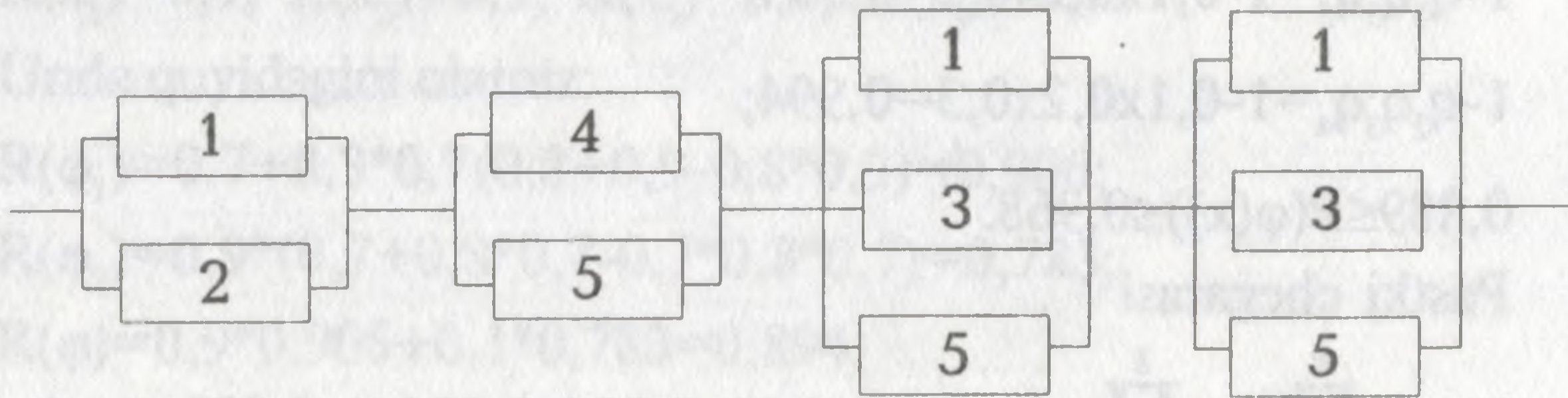
4.2-rasm. Minimal kesishishlar yig'indisi.
