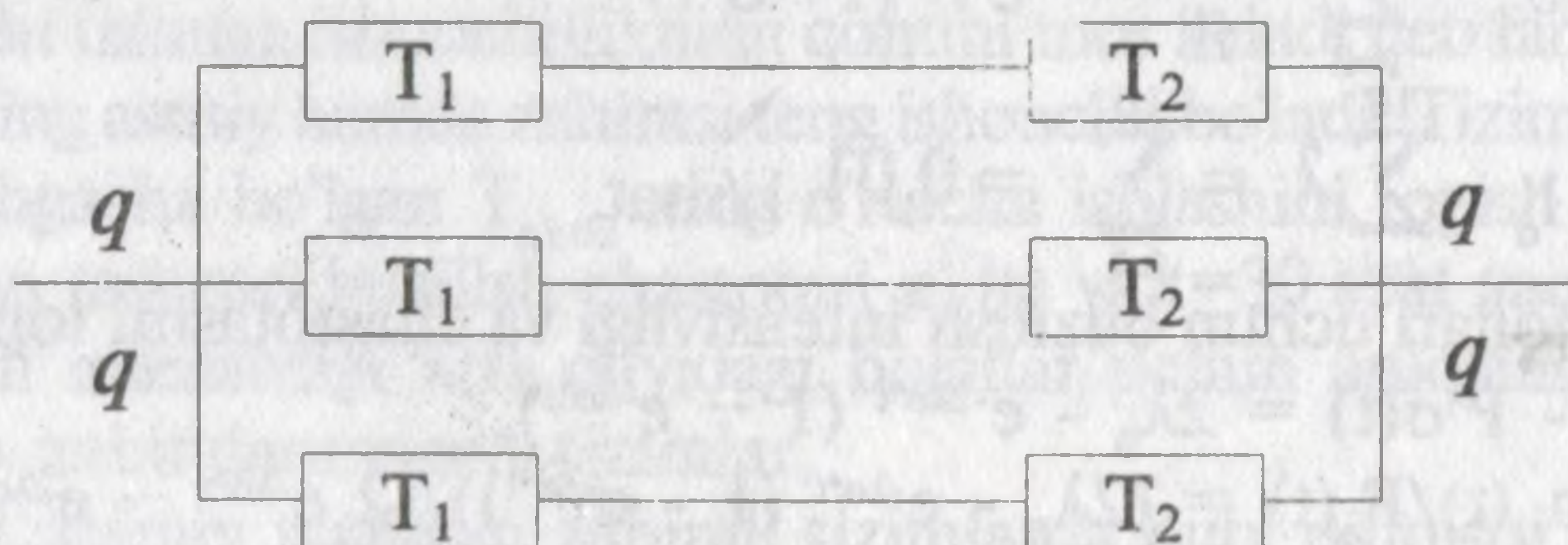
3.1-rasm. Ishonchlilik sxemasini hisoblash.
