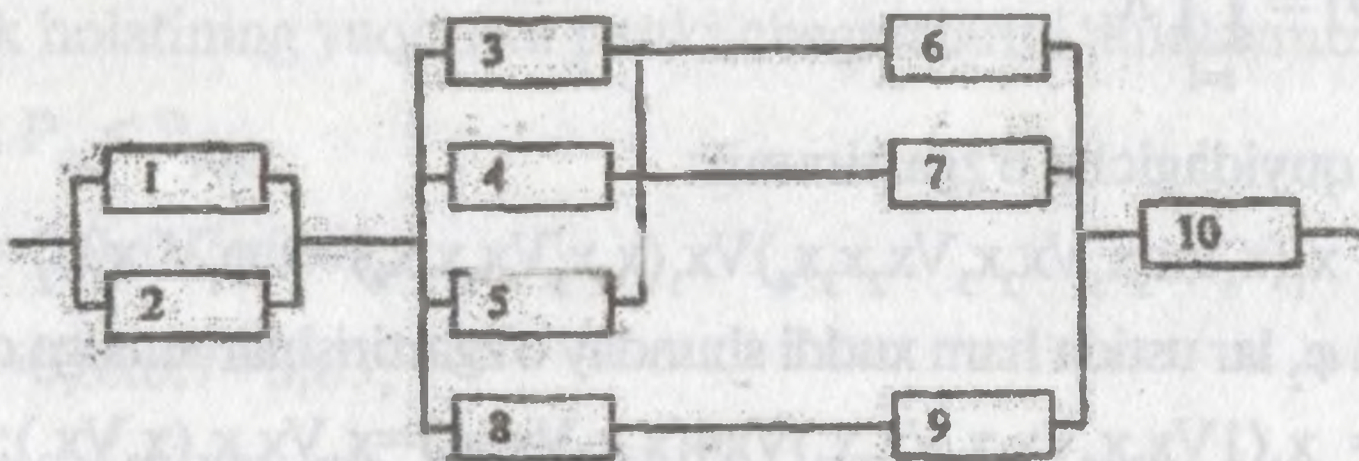
5.1-rasm. Ketma-ket — parallel tizimning strukturasi.
