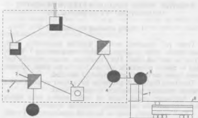
7.1-rasm. Elektrlashgan temir yo'llarda elektr ta'minotining prinsipial chizmasi: 1-issiqlik elektr stantsiyasi; 2- gidroelektrstantsiya; 3- atom elektr stantsiyasi; 4-nohiiaviy transformator nimstantsiyasi; 5- yuqori kuchlanishli tuman liniyasi; 6-tortuvchi nimstansiya; 7- ta'minot liniyasi; 8-kontakt tarmog'i; 9-energiya tizimlarini bog'lovchi liniya.
