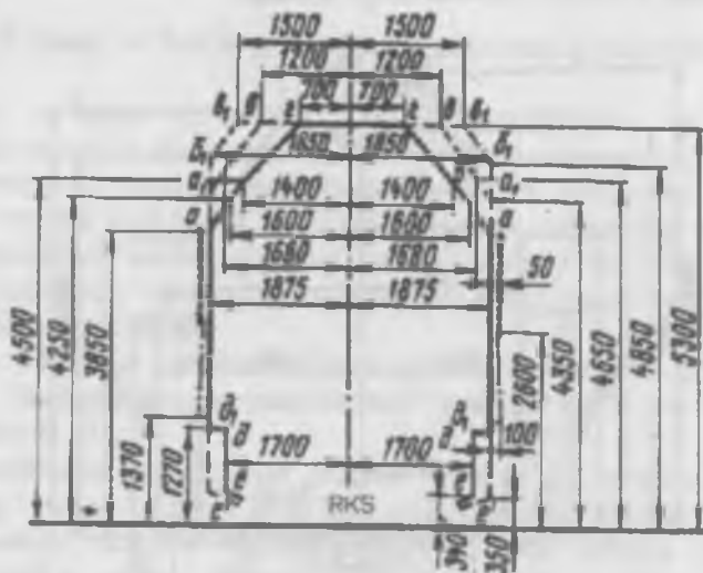
3.9-rasm. Temir yo'llarda harakat tarkibi gavariti «T».
