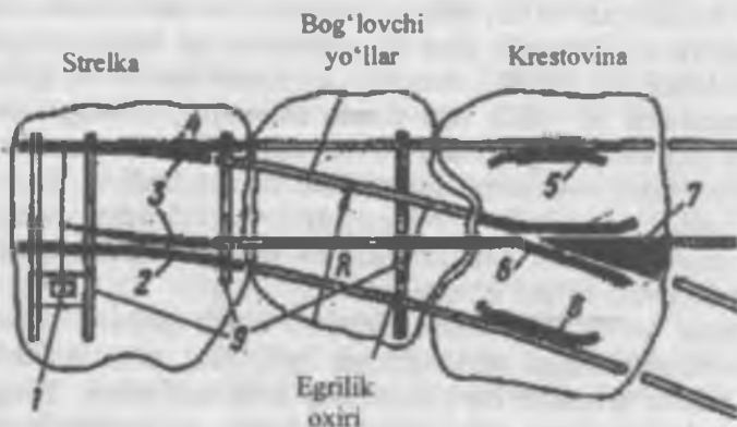
5.38-rasm. Oddiy strelkali o'tkazgich chizmasi: 1-o'tkazuvchi mexanizm; 2, 4-rama relslari; 3-ayri yo'naltirgich (отрпак); 5,8-kontrrelslar; 6-usovik; 7-krestovina; 9-o'tkazgich bruslari (shpallar).
