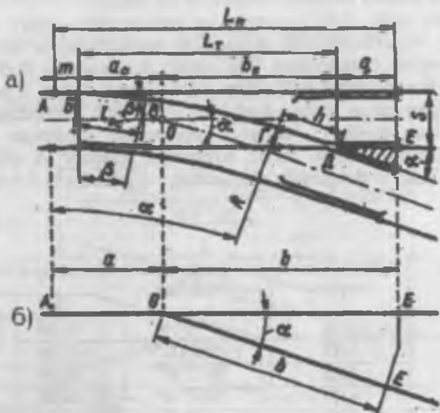
5.43-rasm. Stelkali o'tkazgichning geometrik elementlari (unsurlari).
