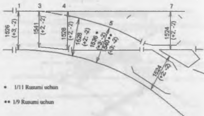
T2,b-rasm. 1524 mm li yo'l uchun o'lchov joylari: 1 – ramali rels ulanmasi; 2 – ramali rels burilish egrisining boshlanish joyi; 3 – strelka ayrilarining uchi; 4 – ayrilar o'zagi; 5 – o'tkazgich egrisining o'rtasi; 6 – o'tkazgich egrisining oxiri; 7 - krestovina.
