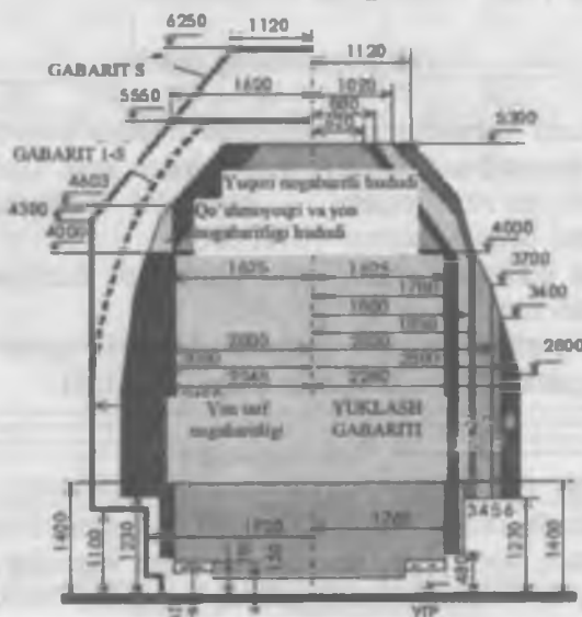
T12-rasm. Harakat tarkibi gʻabariti.
