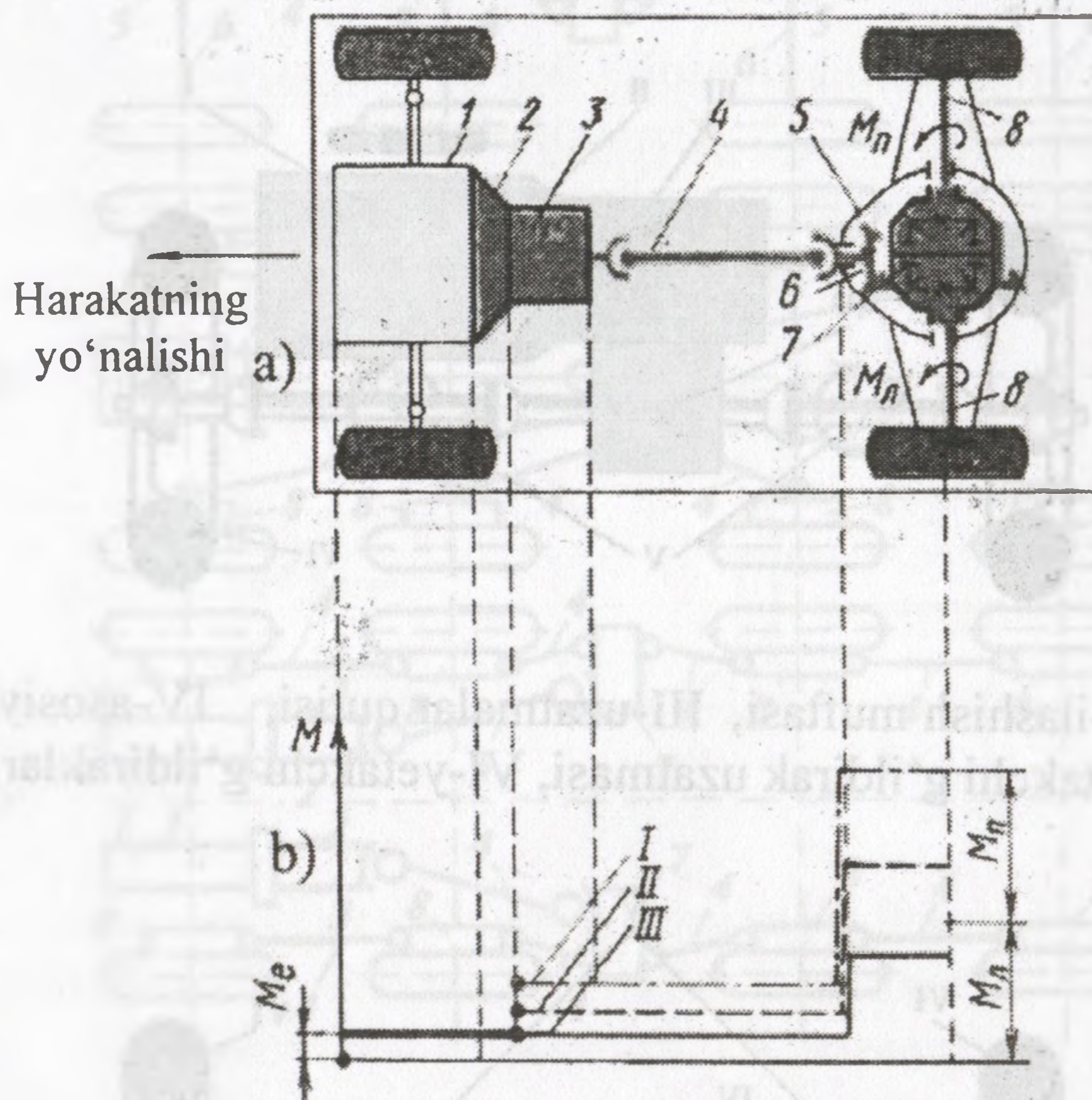
4.1-rasm. Mexanik transmissiyada burovchi momentning uzatilishi: 1-dvigatel; 2-ilashish muftasi; 3-uzatmalar qutisi; 4-kardan uzatmasi; 5-orqa ko'prik; 6-asosiy uzatma; 7-differensial; 8-yarim o'qlar.
