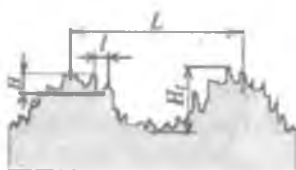
2.27-rasm. Sirt g'adir-budirlik va to'liqsimonligi.
