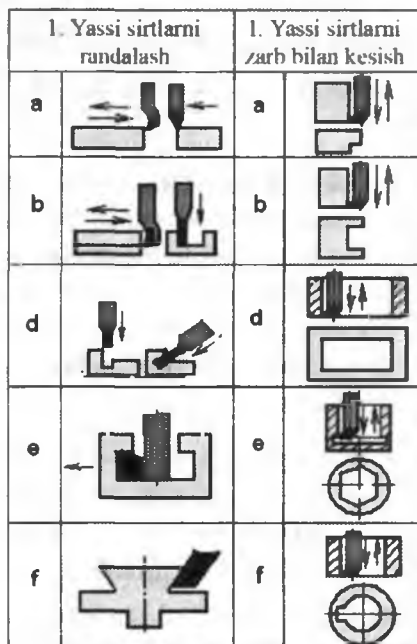
5.2-rasm. Yassi sirtlarni randalash va zarb bilan kesish-o'yish sxemalari: 1—randalash:
