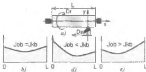
2.17-rasm. Tanavorlarni yo'aish sxemasi: (a) va to'g'ri karlik dastgohi elementlarining birliklarining turli nisbatlaridagi elastik defomatsiyalanish grafiklari (b, d, e)
