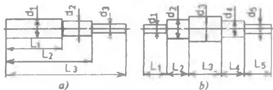
2.18-rasm. Pog'onali vallarning ko'rinishlari.
