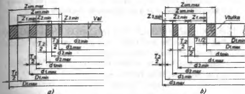
7.5 -rasm. Sozlangan dastgohlarda ishlashda texnologik o'tuvlar bo'yicha a—val va b—vtulka tanavori oraliq qattalalari maydonlarining va chegaraviy o'lchamlarining sxemasi.
