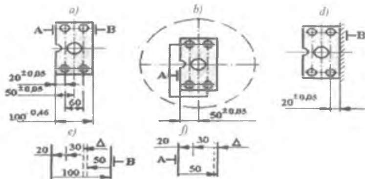
3.16-rasm. Yo'nish va parrmalashda bazalar doimiylik tamoyilini qo'llash.
