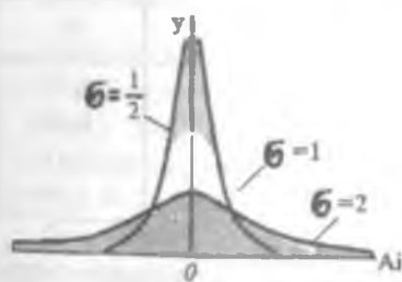
2.6-rasm. O'rtacha kvadrat og'ishining tabiiy taqsimot egri chiziq'i shakliga ta'siri.
