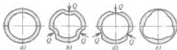
2.26-rasm. Silindri ichki yoʻnishda qoʻyilgan siquvchi Q kuchlardan sodir boʻlavchi mahkamlash xatoligining taʼsirini aniqlash sxemalari: a —tanavor; b — Q kuchlar bilan siqilgan holati; d —siqilgan holda ichi yoʻnilgan holat; e —siqishdan boʻshatilgan holat.
