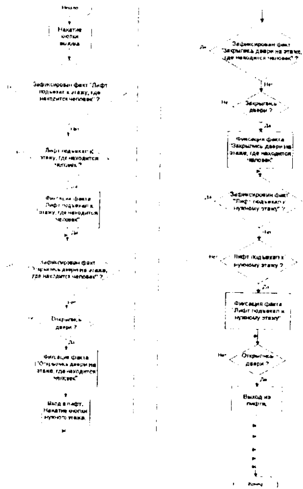
Рис. 16. Алгоритм реализации в конкретной среде выполнения с учетом ее особенностей.
