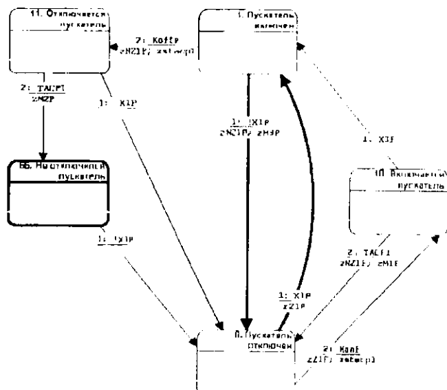
Рис. 6. Граф переходов автомата управления переверсивным приводом.
