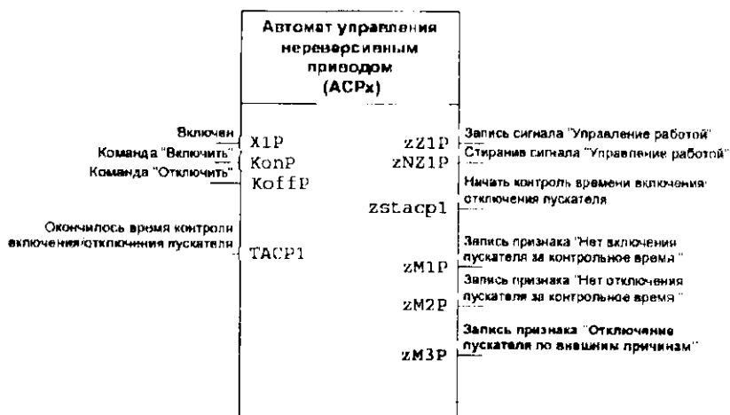
Рис. 5. Схема связей автомата управления переверсивным приводом.
