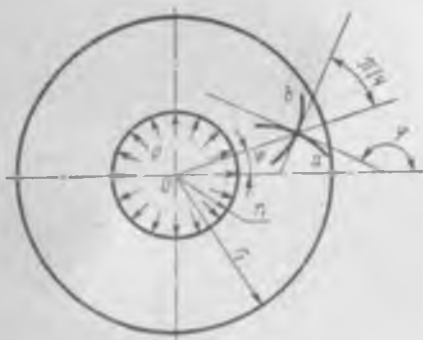
Рис. 9.20. Направление линий скольжения в толстостенной трубе, нагруженной внутренним давлением
