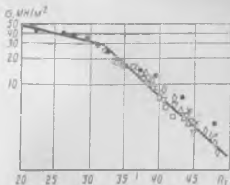
Рис. 11.22. График зависимости предела длительной прочности от температурно-временного параметра Ларсона—Миллера [30]: ● — кратковременные испытания; ○ — 649° C; □ — 740° C; △ — 760° C; ▽ — 815° C; ◇ — 871° C; × — 970° C
