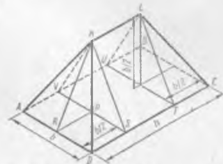
Рис. 10.19. Поверхность функции напряжений для прямоугольного сечения
