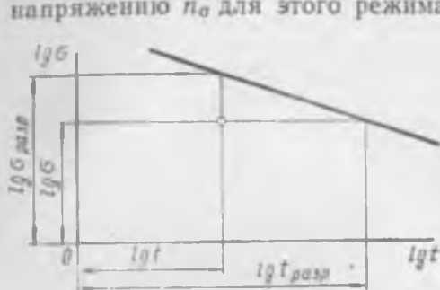
Рис. 11.30. К определению коэффициента запаса по времени и напряжениям при напряжении, постоянном во времени
