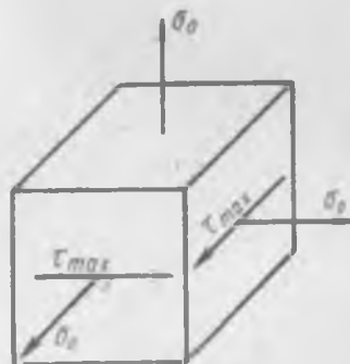
Рис. 9.3. Напряженное состояние в условиях плоской деформации
