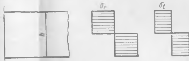
Рис. 10.25. Эпюры окружных и радиальных напряжений по высоте для пластины, находящейся в предельном состоянии
