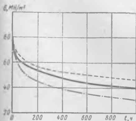
Рис. 12.10. Сопоставление экспериментальной (сплошная линия) и теоретических кривых релаксации для меди при температуре 165^{\circ}\text{C} и начальном напряжении \sigma(0) = 94,9 \text{ MN/m}^2 . Штриховая линия по теории старения в формулировке (12.15), штрихпунктирная линия по теории течения Л. М. Качанова [26]
