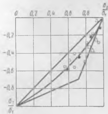
Рис. 3.7. Результаты испытаний труб из меди (○), алюминия (●), мягкой стали (□) и обезуглероженной мягкой стали (△), проведенных Тейлором и Квинни [26]
