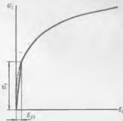
Рис. 5.10. Схематизированная диаграмма деформирования со степенным упрочнением
