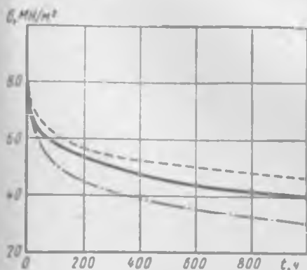
Рис. 12.10. Сопоставление экспериментальной (сплошная линия) и теоретических кривых релаксации для меди при температуре 165^{\circ}\text{C} и начальном напряжении \sigma(0) = 94,9 \text{ MN/m}^2 . Штриховая линия по теории старения в формулировке (12.15), штрихпунктирная линия по теории течения Л. М. Качанова [26]
