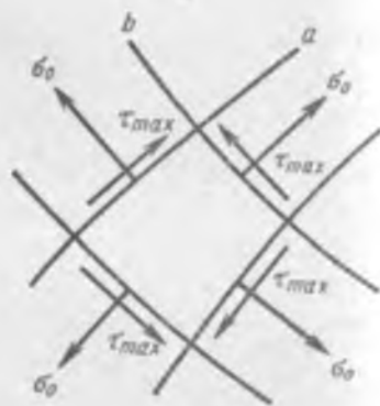
Рис. 9.5. Напряженное состояние элемента, выделенного линиями скольжения
