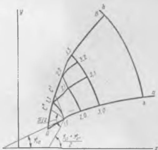
Рис. 9.28. К решению смешанной задачи
