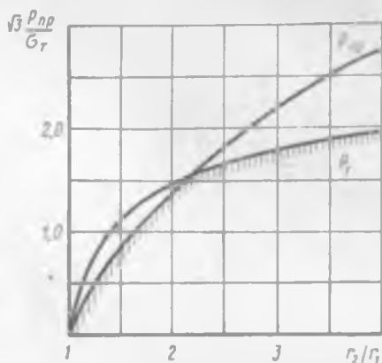
Рис. 10.35. Графики зависимости удвоенного давления, при котором возникают пластические деформации при первом нагружении, и предельного давления от отношения наружного радиуса трубы к внутреннему
