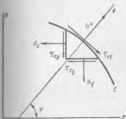
Рис. 9.8. Напряженное состояние элемента у поверхности тела
