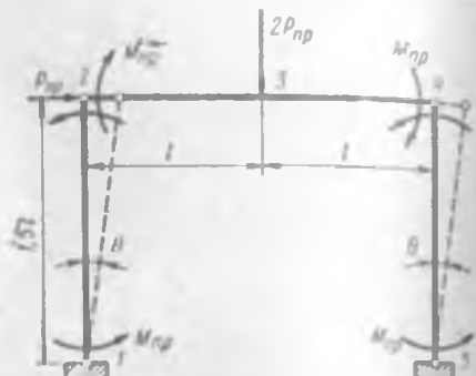
Рис. 10.7. Механизм бокового смещения
