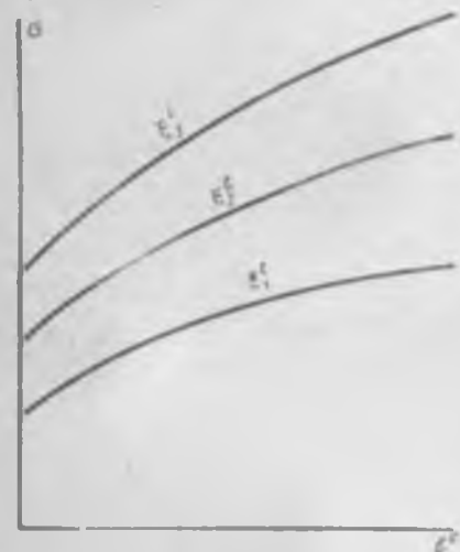
Рис. 12.8. Графики зависимости напряжения от деформации ползучести при постоянной скорости ее ( \epsilon_3^c > \epsilon_2^c > \epsilon_1^c )
