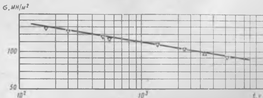
Рис. 15.1. Сопоставление графика зависимости (15.5) с результатами опытов [7]
