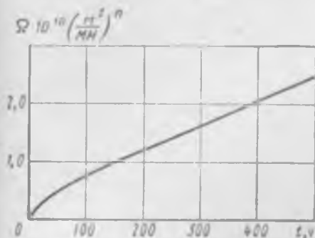
Рис. 13.21. Ориентировочный график функции \Omega для стали 45X14H14B2M при температуре 600^\circ\text{C}
