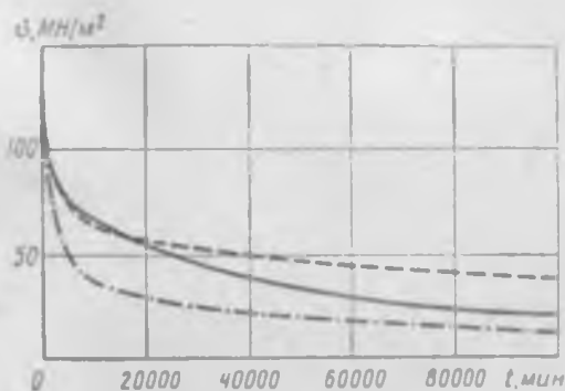
Рис. 12.11. Сопоставление экспериментальной (сплошная линия) и теоретических кривых релаксации для хромолибденовой стали при температуре 525^{\circ}\text{C} и начальном напряжении \sigma(0) = 146 \text{ MN/m}^2 . Штриховая линия — по теории старения в варианте (12.15), штрихпунктирная линия по теории течения Л. М. Качанова [26]
