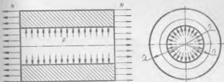
Рис. 6.1. Схема нагружения толстостенной трубы
