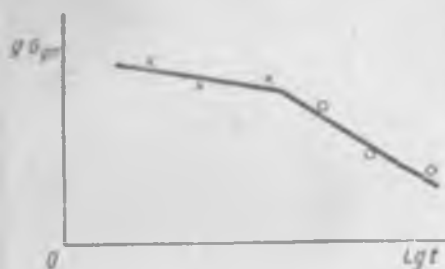
Рис. 11.20. График зависимости предела длительной прочности от времени испытания до разрушения
