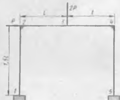
Рис. 10.6. Прямоугольная порталная рама
