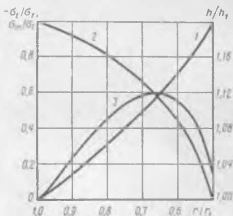
Рис. 8.9. Эюры меридиональных (кривая 1) и окружных (кривая 2) напряжений, а также эюра толщины стенки (кривая 3) для случая волочения трубы без противонапряжения ( \alpha = 14^\circ , f = 0,1 )
