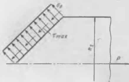
Рис. 9.38. Равновесие жесткой области на выходе из матрицы
