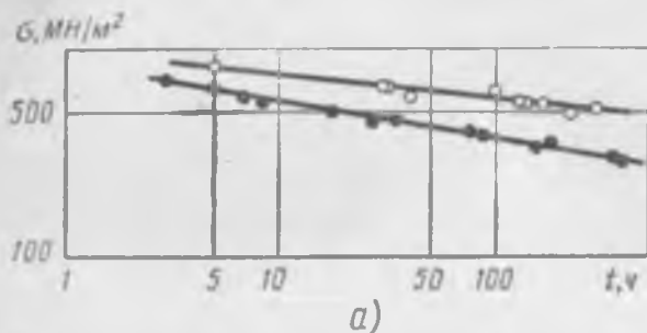
Рис. 11.25. Графики зависимости предела длительной прочности от времени испытания до разрушения:
