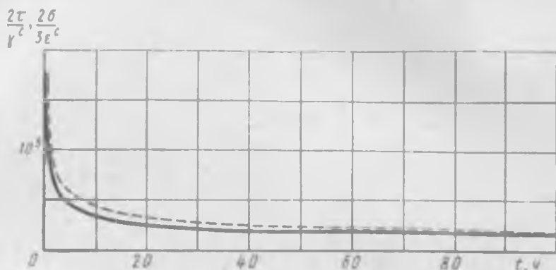
Рис. 12.17. Графики зависимости от времени величин \frac{2\tau}{\gamma^2} (сплошная линия) и \frac{2\sigma}{3\epsilon^2} (штриховая линия) [17]
