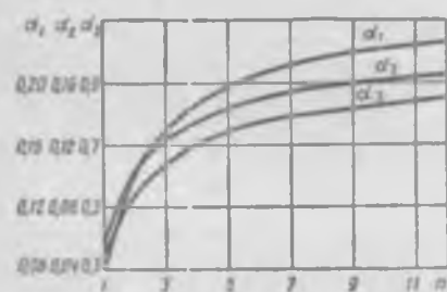
Рис. 13.2. Графики зависимостей коэффициентов \alpha_1 , \alpha_2 и \alpha_3 от показателя степени n
