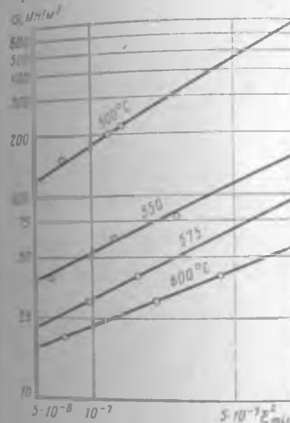
Рис. 11.7. Графики зависимостей напряжения от минимальной скорости деформации ползучести для хромомолибденовой стали марки 60Х16М2А [21]
