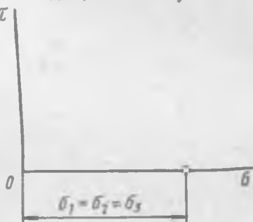
Рис. 1.11. Круговая диаграмма напряжений для трехосного равного растяжения
