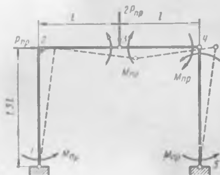
Рис. 10.9. Комбинированный механизм
