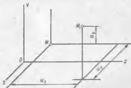
Рис. 2.1. Перемещение точки тела в результате деформации
