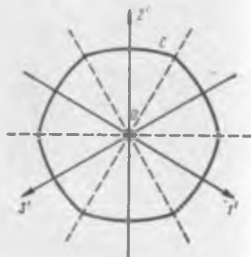
Рис. 3.2. След пересечения поверхности начала пластичности в системе координат \sigma_1 , \sigma_2 , \sigma_3 с девнаторной плоскостью
