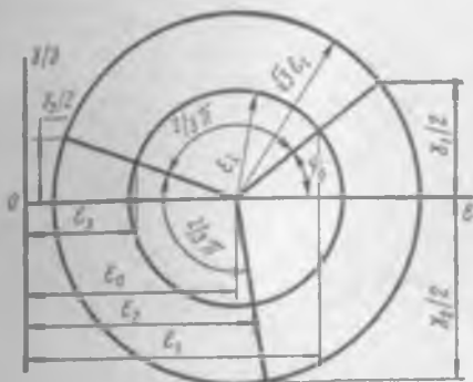
Рис. 2.3. Звезда Пелчинского для деформаций
