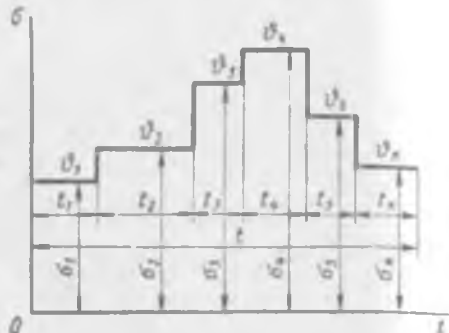
Рис. 11.31. Нестационарный режим напряженности и нагрева
