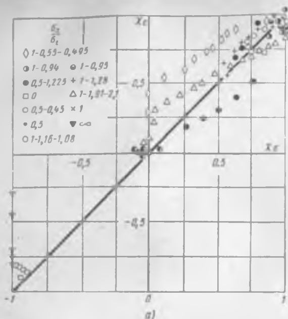
Рис. 4.17. Результаты опытов А. М. Жукова. Испытания образцов стали 30ХНЗА [13]:
