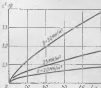
Рис. 11.12. Кривые ползучести стали 45X14H14B2M при 800^\circ\text{C} [10]
