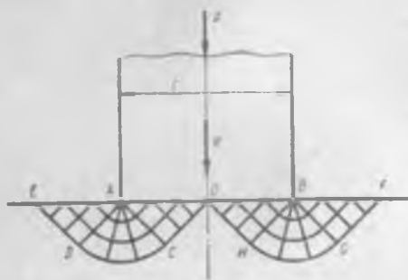
Рис. 9.24. Линии скольжения в жестко-пластическом теле, ограниченном плоскостью при вдавливании в него абсолютно жесткого штампа с плоским основанием (решение Хилла)
