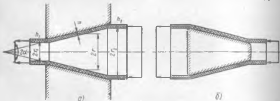
Рис. 8.8. Схемы волочения, обжатия, протяжки и раздачи
