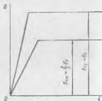
Рис. 10.33. Диаграммы растяжения материалов стержней
