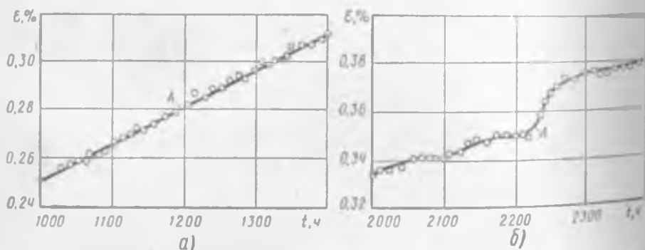
Рис. 11.2. Участки кривых ползучести, полученные при испытании образцов стали ЭН1454 при температуре 550° С и напряжении 90 МН/м² [22]:
