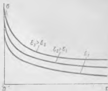
Рис. 12.2. Сечения поверхности в координатах \epsilon, \sigma, t плоскостями, перпендикулярными оси \epsilon , — кривые релаксации
