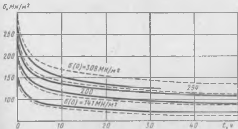
Рис. 12.12. Сопоставление экспериментальных кривых релаксации для хромомолибденовой стали 30ХМ при температуре 500^{\circ}\text{C} и различных начальных напряжениях (сплошные линии) с теоретическими, построенными по теории упрочнения в варианте (12.28), (12.29) (штриховые линии) [3]
