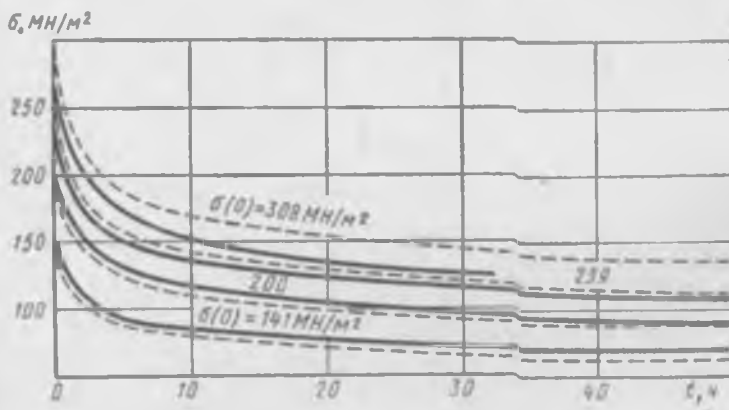
Рис. 12.12. Сопоставление экспериментальных кривых релаксации для хромомolibденовой стали 30ХМ при температуре 500^\circ\text{C} и различных начальных напряжениях (сплошные линии) с теоретическими, построенными по теории упрочнения в варианте (12.28), (12.29) (штриховые линии) [3]
