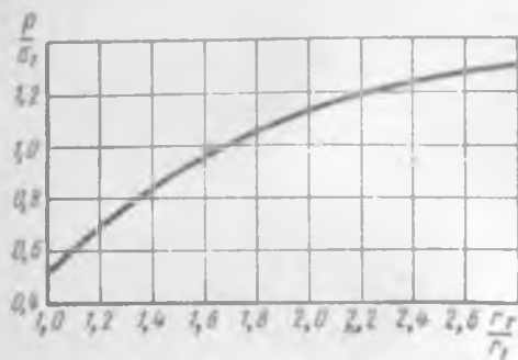
Рис. 6.4. К примеру расчета автоскрепления трубы. График зависимости давления автоскрепления от радиуса границы, разделяющей упругую и пластическую области
