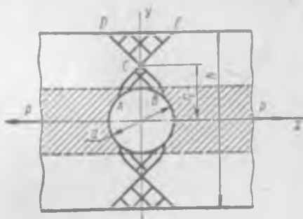
Рис. 10.14. Плита с отверстием, растянутая силой P , МН/м
