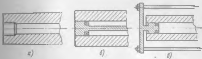
Рис. 6.3. Схемы двух способов автоскрепления:
