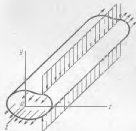
Рис. 9.1. Нагружение тела в условиях плоской деформации
