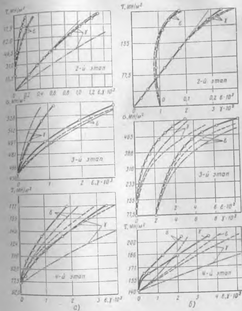
Рис. 4.21. Графики зависимости касательного и нормального напряжений от угловой и линейной деформаций для стальных труб в опытах Моррисона и Шепферда [28]. Сплошные линии — экспериментальные кривые, штриховые — по теории течения, штрих-пунктирные — по теории малых упруго-пластических деформаций; а — первый образец; б — второй образец
