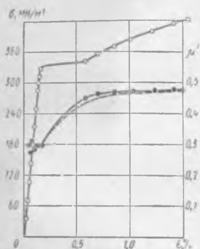
Рис. 4.16. Диаграмма растяжения и график зависимости коэффициента поперечной деформации от величины деформации для стали 30 [8]
