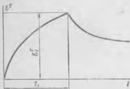
Рис. 12.9. К построению кривой обратной ползучести по теории ползучести с анизотропным упрочнением
