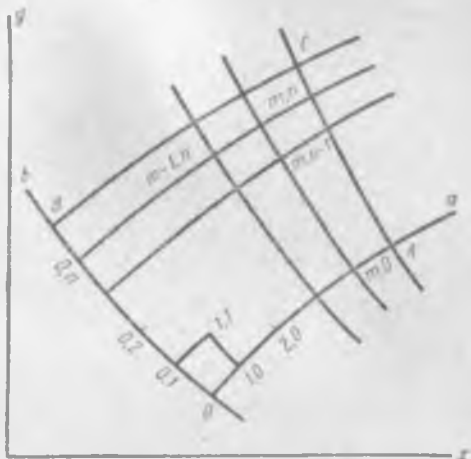
Рис. 9.25. К решению начальной характеристической задачи (задачи Римана)
