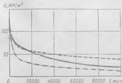
Рис. 12.11. Сопоставление экспериментальной (сплошная линия) и теоретических кривых релаксации для хромомолибденовой стали при температуре 525^{\circ}\text{C} и начальном напряжении \sigma(0) = 146 \text{ MN/m}^2 . Штриховая линия — по теории старения в варианте (12.15), штрихпунктирная линия по теории течения Л. М. Качанова [26]
