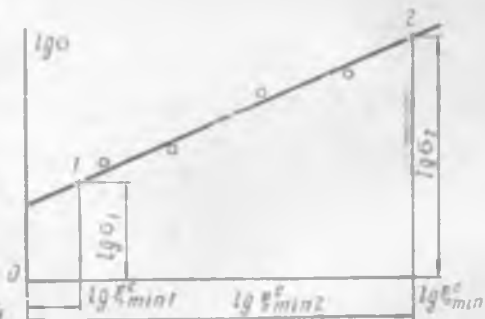
Рис. 11.8. К определению показателя степени n и коэффициента k
