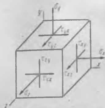
Рис. 1.3. Модель напряженного состояния
