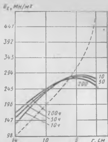
Рис. 14.1. Эпюры окружных напряжений для различных значений времени (сплошные линии) и в пределах упругости (штриховая линия) в равномерно нагретом до температуры 575°С диске постоянной толщины с отверстием из стали РЗ [14]
