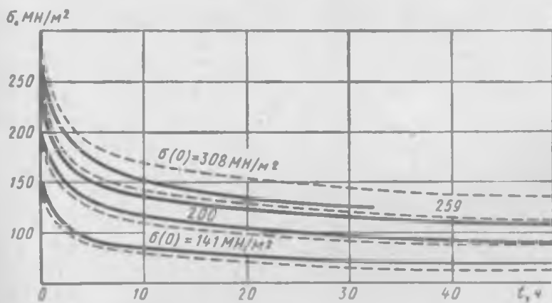
Рис. 12.12. Сопоставление экспериментальных кривых релаксации для хромолибденовой стали 30ХМ при температуре 500^{\circ}\text{C} и различных начальных напряжениях (сплошные линии) с теоретическими, построенными по теории упрочнения в варианте (12.28), (12.29) (штриховые линии) [3]
