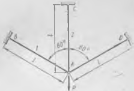
Рис. 12.24. Статически-неопределимая стержневая система
