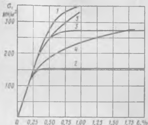
Рис. 12.23. Диаграмма мгновенного растяжения (кривая 1) титанового сплава BT5-1 при температуре 600° С [25] и диаграммы растяжения при постоянных скоростях деформации: \dot{\varepsilon} = 1,67 \cdot 10^{-4} 1/с (кривая 2); \dot{\varepsilon} = 16,7 \cdot 10^{-4} 1/с (кривая 3) и постоянных скоростях напряжения \dot{\sigma} = 7,5 МН/м 2 с (кривая 4) и \dot{\sigma} = 75 МН/м 2 с (кривая 5) [13]
