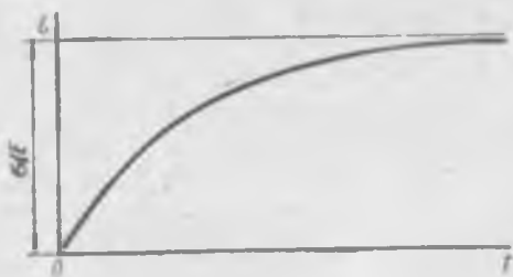
Рис. 16.6. Кривая последствия в теле Фойгта
