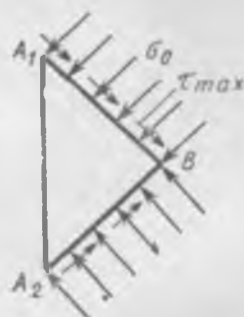
Рис. 9.31. Равновесие жесткой области, примыкающей к торцу
