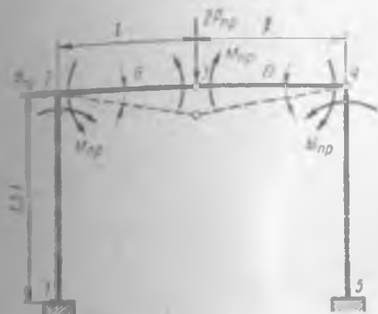
Рис. 10.8. Балочный механизм
