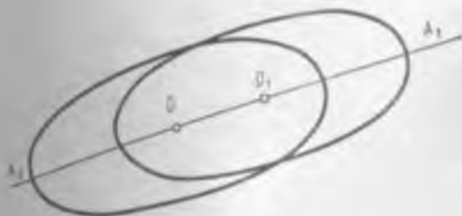
Рис. 4.24. Жесткое смещение поверхности пластичности в процессе нагружения
