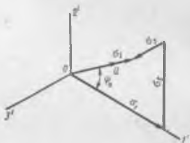
Рис. 1.7. Проекции осей \sigma_1, \sigma_2 и \sigma_3 на девиаторную плоскость и диаграмма Марциняка для напряжений
