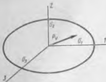
Рис. 1.8. Эллипсоид напряжений
