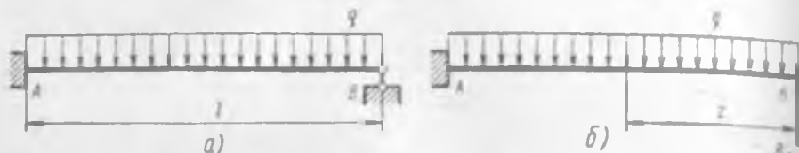
Рис. 10.3. Статически неопределимая балка (а); эквивалентная система (б)
