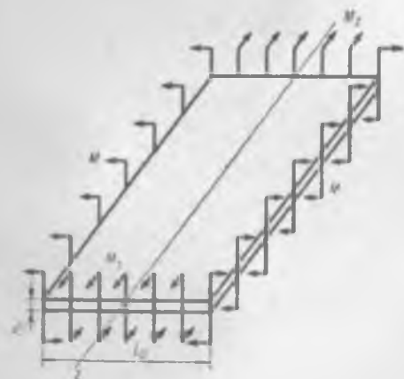
Рис. 8.5. Лист в условиях чистого изгиба
