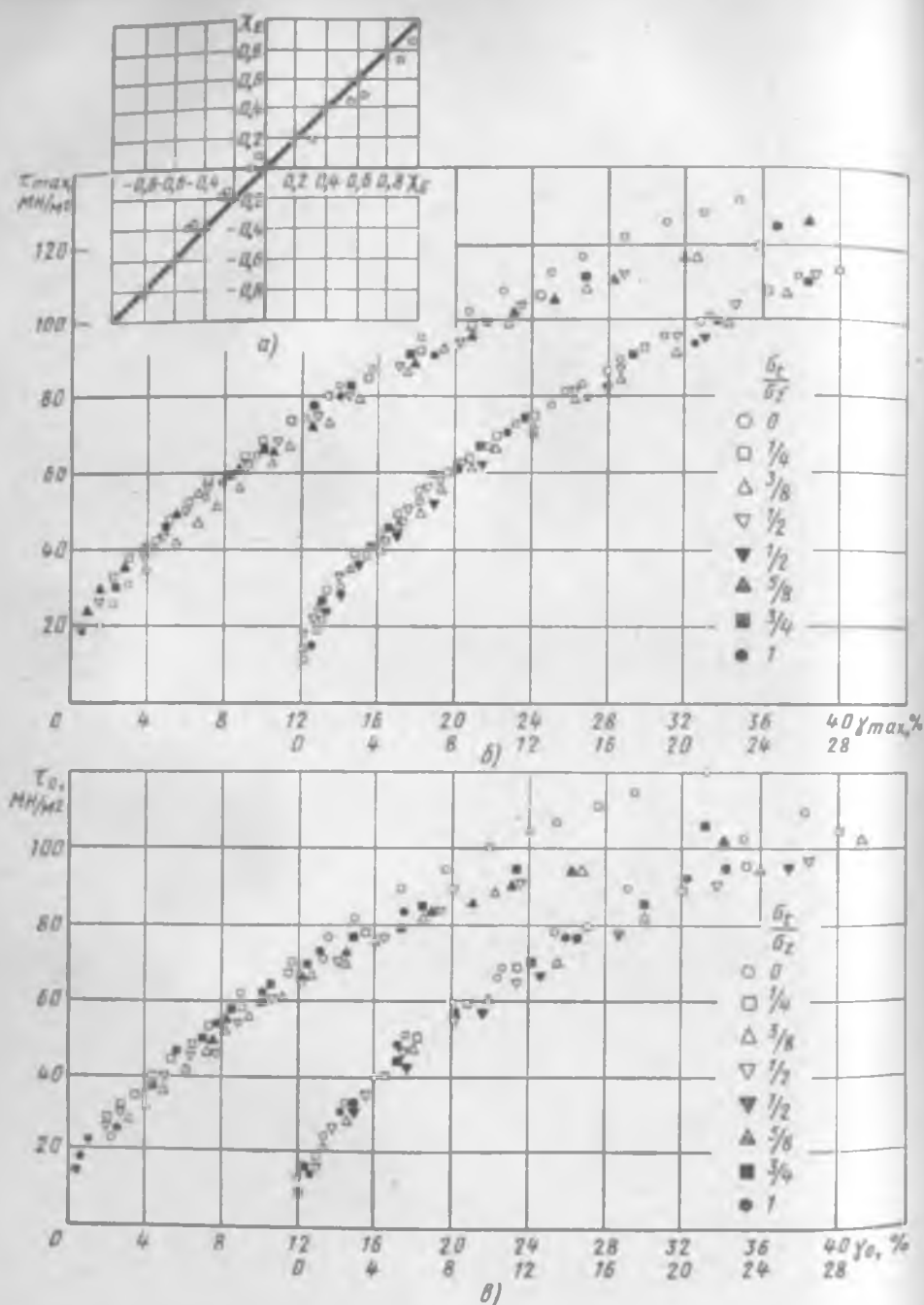
Рис. 4.13. Результаты опытов Дэвиса. Испытания медных образцов [6]:
