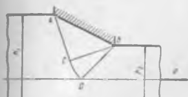
Рис. 9.37. К решению частного случая задачи волочения листа
