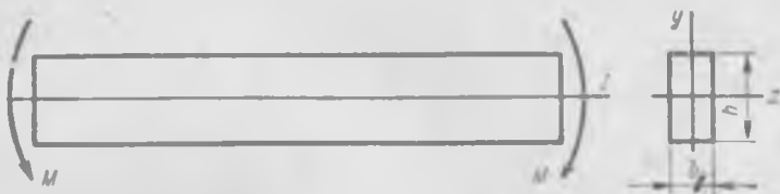
Рис. 14.2. Брус прямоугольного поперечного сечения в условиях чистого изгиба
