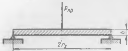
Рис. 10.28. Круглая пластина оперта по контуру и нагружена в центральной точке сосредоточенной силой
