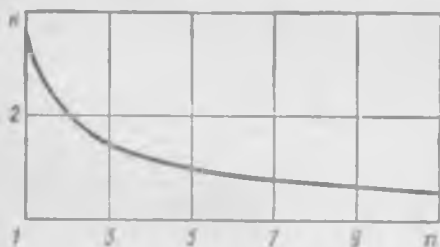
Рис. 13.24. График зависимости от показателя степени n коэффициента концентрации напряжений в бесконечной пластине с отверстием, растянутой силами, приложенными на бесконечности симметрично относительно центра отверстия, в условиях плоского напряженного состояния
