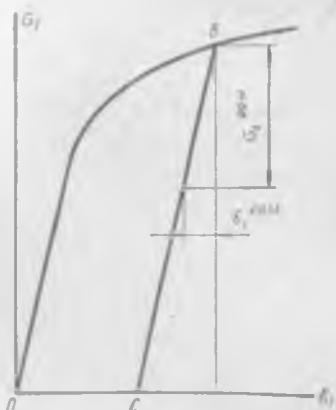
Рис. 4.23. Диаграмма деформирования при нагружении и разгрузке
