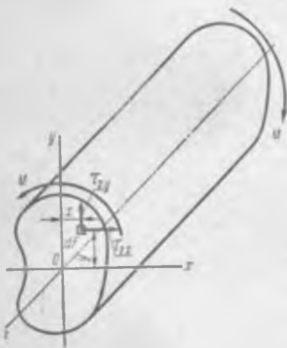
Рис. 10.16. Скрученный брус некруглого поперечного сечения
