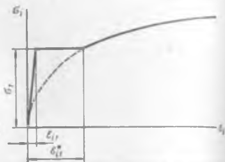
Рис. 5.8. Схематизированная диаграмма деформирования с площадкой текучести и степенным упрочнением
