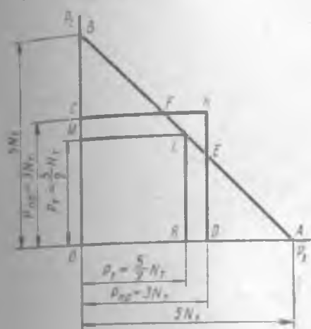
Рис. 10.34. Диаграмма приспособляемости для стержневой системы
