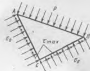
Рис. 9.34. Равновесие области равномерного напряженного состояния
