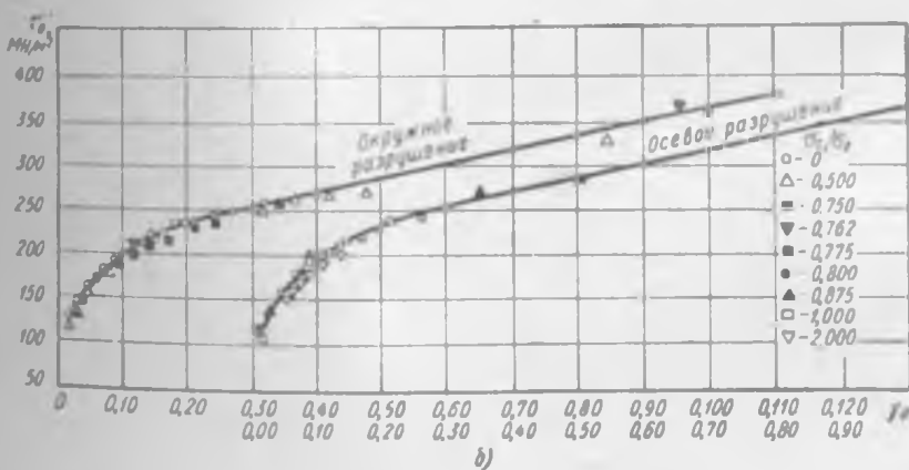
Рис. 4.14. Результаты опытов Дэвиса. Испытания стальных образцов [7]:
