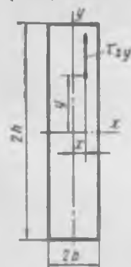
Рис. 13.12. Поперечное сечение скрученного бруса в форме вытянутого прямоугольника
