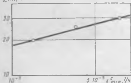
Рис. 11.13. График зависимости напряжения от минимальной скорости деформации ползучести для стали 45X14H14B2M при температуре 800°С
