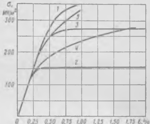
Рис. 12.23. Диаграмма мгновенного растяжения (кривая 1) титанового сплава ВТ5-1 при температуре 600° С [25] и диаграммы растяжения при постоянных скоростях деформации: \dot{\epsilon} = 1,67 \cdot 10^{-4} 1/с (кривая 2); \dot{\epsilon} = 16,7 \cdot 10^{-4} 1/с (кривая 3) и постоянных скоростях напряжения \dot{\sigma} = 7,5 МН/м 2 с (кривая 4) и \dot{\sigma} = 75 МН/м 2 с (кривая 5) [13]
