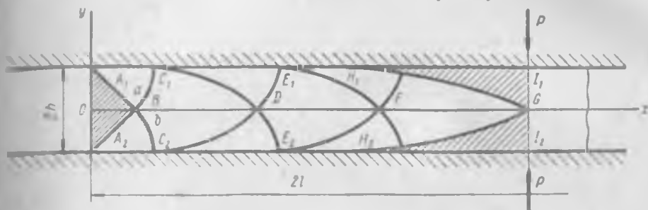
Рис. 9.30. К решению задачи сжатия слоя между жесткими шероховатыми плитами
