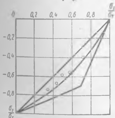
Рис. 3.6. Результаты испытаний стальных труб, проведенных Рошем и Эйрингом [14]
