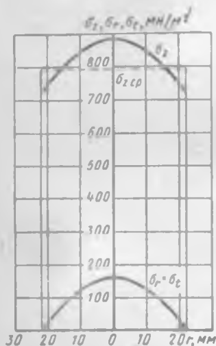
Рис. 5.4. Эпюры осевых, радиальных (окружных) напряжений в минимальном сечении шейки круглого образца из стали 30 для величины логарифмической деформации \bar{\epsilon} = 0,68 . Начальный диаметр образца d_0 = 6 мм, наименьший диаметр шейки d = 4,4 мм, радиус кривизны контура шейки в точке наименьшего сечения R = 4,8 мм
