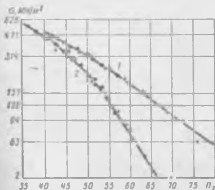
Рис. 11.23. График зависимости предела длительной прочности от температурно-временного параметра Мэнсона—Хаферда [27]:
