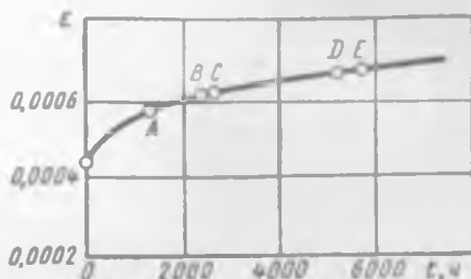
Рис. 11.3. Кривая ползучести, полученная при испытании образцов хромоникелемо-диборной стали при температуре 400^\circ\text{C} и напряжении 77,5\text{ МН/м}^2 с охлаждением без разгрузки [26]. Продолжительность охлаждения: в точке A — 118 ч; B — 53 ч; C — 54 ч; D — 93 ч; E — 120 ч.
