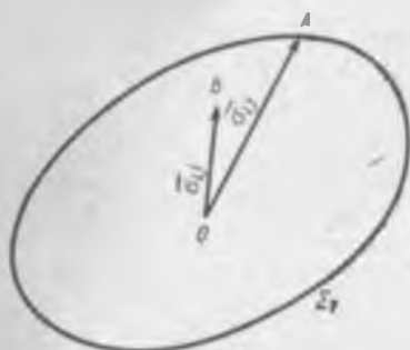
Рис. 3.1. Поверхность начала пластичности в шестимерном пространстве напряжений
