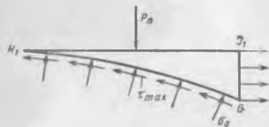
Рис. 9.32. Равновесие жесткой области, примыкающей к вертикальной плоскости симметрии
