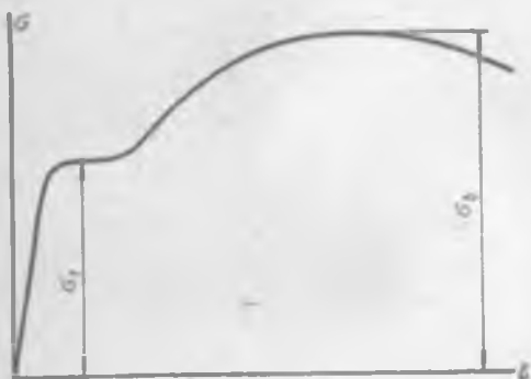
Рис. 5.1. Условная диаграмма растяжения
