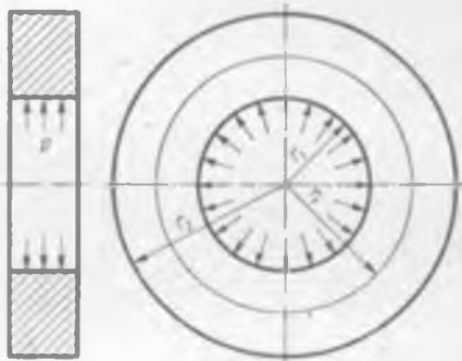
Рис. 6.6. Диск постоянной толщины, нагруженный внутренним давлением
