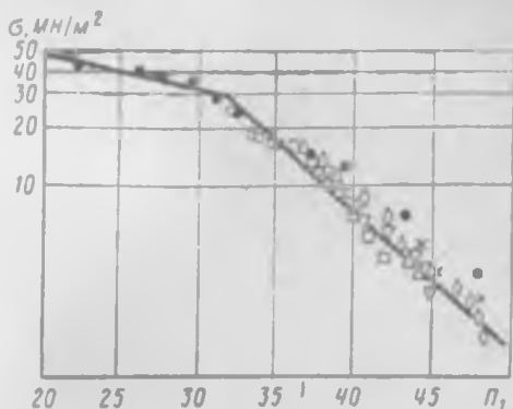
Рис. 11.22. График зависимости предела длительной прочности от температурно-временного параметра Ларсона—Миллера [30]: ● — кратковременные испытания; ○ — 649° С; □ — 740° С; △ — 760° С; ▽ — 815° С; ◇ — 871° С; × — 970° С
