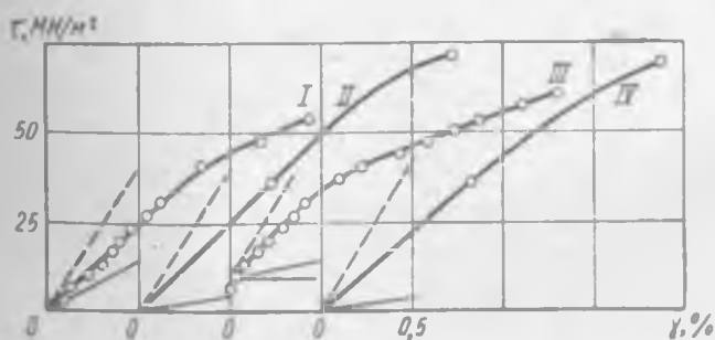
Рис. 4.19. Диаграммы догрузки в опытах А. М. Жукова и Ю. Н. Работнова [9]. Кривые с кружочками получены экспериментально, тонкие линии — по теории малых упруго-пластических деформаций, штриховые — по теории течения
