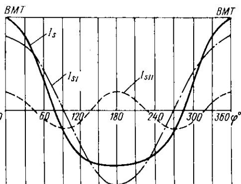
Рис. 5.4. Диаграммы сил инерции возвратно-поступательно движущихся частей:
