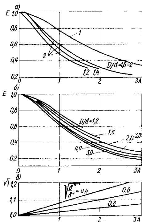
Рис. 9.7. Коэффициенты эффективности ребер E : а — для квадратных ребер; б — для круглых ребер; в — поправочный коэффициент
