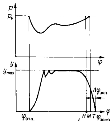
Рис. 7.10. Диаграмма потерь давления и перемещения пластины клапана
