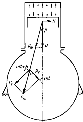
Рис. 5.9. Схема действия сил в компрессоре
