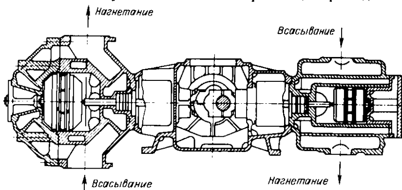
Рис. 12.6. Оппозитный компрессор
