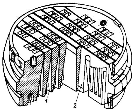
Рис. 7.9. Схема проточного клапана
