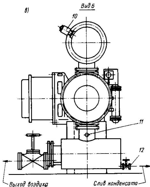
Рис. 12.5. Компрессорная установка 2BM2,5-12/9: а — вид сбоку; б — вид сверху; в — вид Б; 1 — холодильник промежуточный; 2 — компрессор; 3 — холодильник концевой; 4 — система смазки; 5 — фильтр-глушитель; 6 — клапан обратный; 7 — вентиль запорный; 8 — электродвигатель; 9 — вентиль байпасный; 10, 11 — клапаны предохранительные; 12 — вентиль продувки
