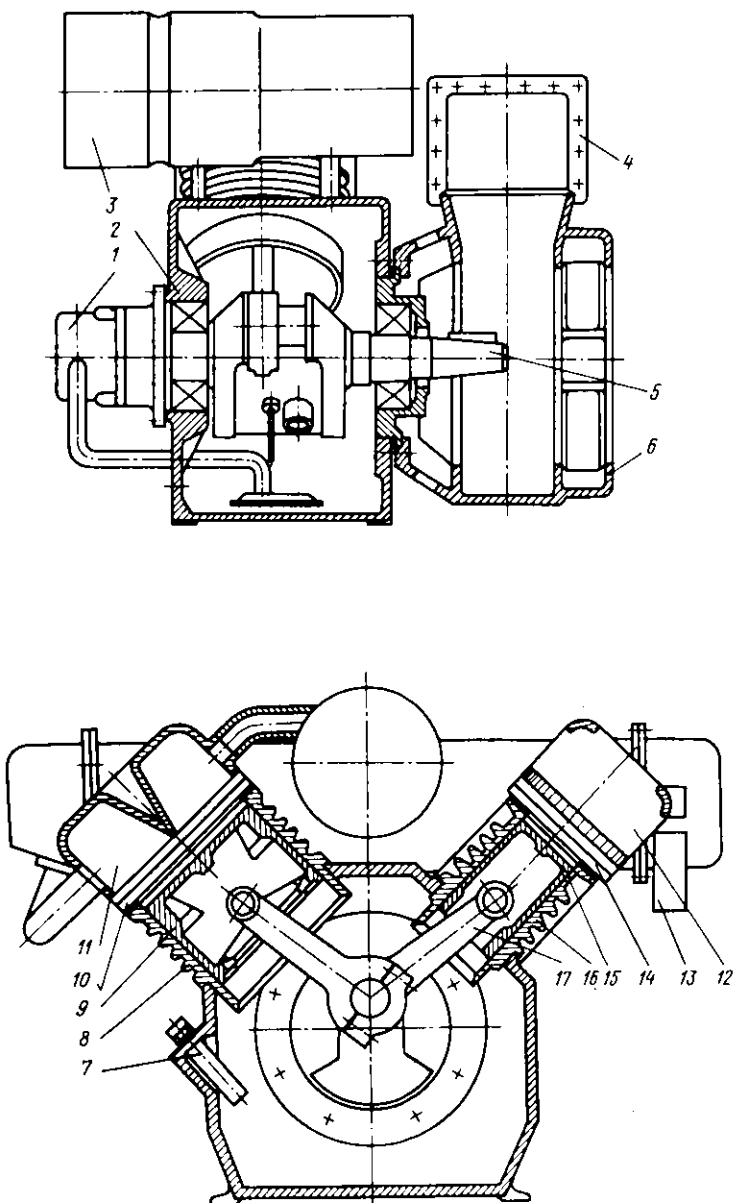
Рис. 12.2. Поперечный и продольный разрезы бескрейцкопфного компрессора 2BV1-2,5/13:
