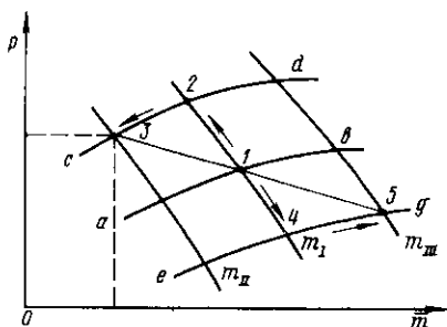
Рис. 11.4. Схема поворота характеристики компрессора регулятором
