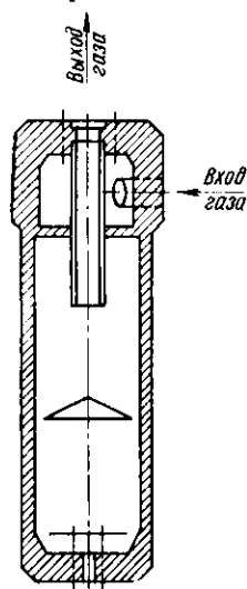
Рис. 9.11. Маслосепаратор типа «Циклон»
