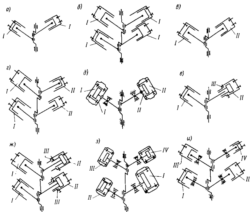
Рис. 6.4. Схемы исполнения компрессоров на унифицированной У-образной базе: а — двухрядная одноступенчатая; б — четырехрядная одноступенчатая; в — двухрядная двухступенчатая; г — четырехрядная двухступенчатая; д — двухрядная двухступенчатая крейцкопная; е — двухрядная трехступенчатая с дифференциальными поршнями; ж — четырехрядная двухступенчатая с дифференциальными поршнями; з, и — четырехрядная четырехступенчатая крейцкопная (I, II, III, IV — порядковые номера ступеней сжатия)
