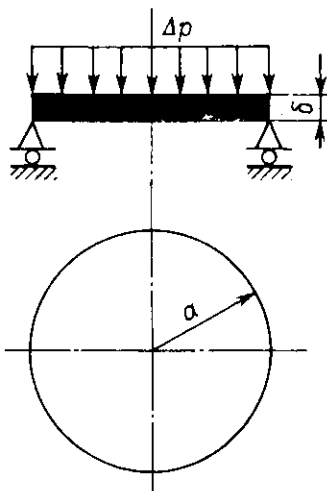
Рис. 7.21. К расчету тарелки тарельчатого клапана на прочность
