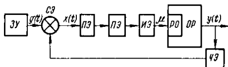
Рис. 11.2. Функциональная схема регулирования компрессора: ОР — объект регулирования; ЧЭ — чувствительный элемент; ЗУ — задающее устройство; СЭ — суммирующий элемент; ПЭ — промежуточный элемент; ИЭ — исполнительный элемент; РО — регулируемый орган; y — регулируемый параметр; g — задающее воздействие; x — ошибка; \mu — регулирующее воздействие
