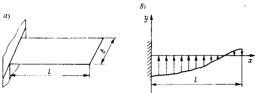
Рис. 7.14. К расчету прямого клапана: а — схема пластины; б — схема нагрузки на пластину
