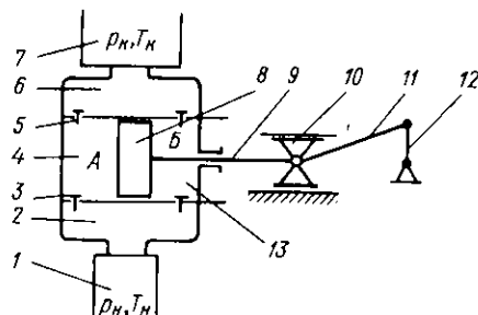
Рис. 2.1. Схема одноступенчатого компрессора с дисковым поршнем:
