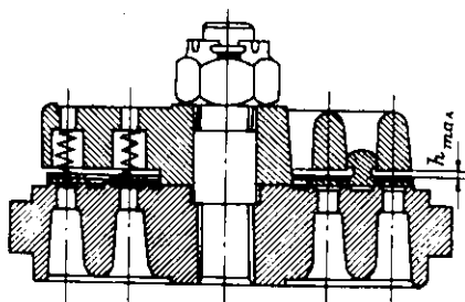
Рис. 7.4. Схема кольцевого клапана
