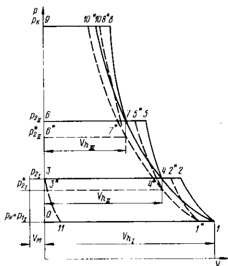
Рис. 11.5. График изменения совмещенной индикаторной диаграммы многоступенчатого компрессора при теоретическом процессе и дросселировании всасываемого газа:
