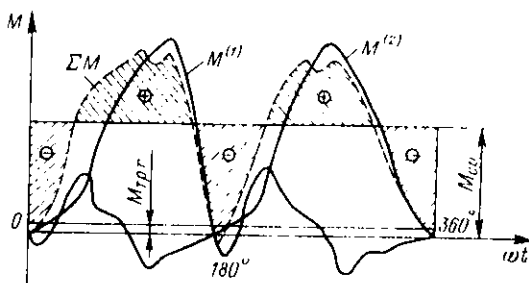
Рис. 5.14. График зависимости противодействующего момента от угла поворота вала
