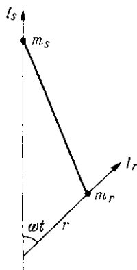
Рис. 5.3. К расчету сил инерции
