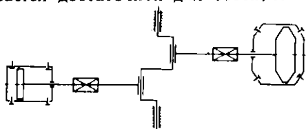
Рис. 4.3. Схема оппозитного компрессора с трапециевидным поршнем первой ступени
