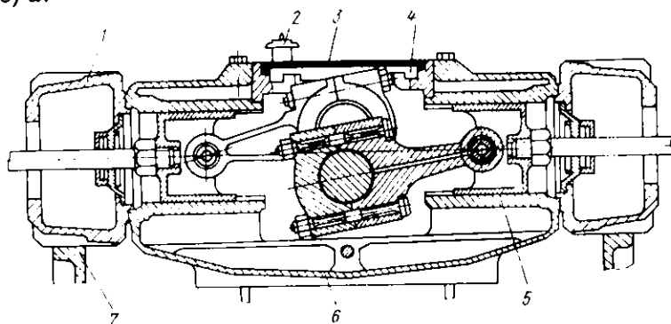
Рис. 6.10. Типичная конструкция двухрядной оппозитной базы:
