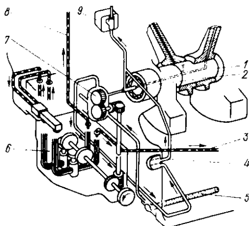
Рис. 10.4. Смазка механизма движения под давлением, а цилиндров — разбрызгиванием
