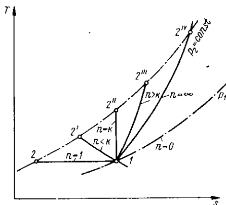
Рис. 1.3. Кривые процессов сжатия в координатах Ts
