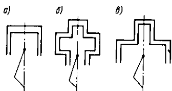
Рис. 4.1. Схемы компрессоров с поршнями: а — тройковым; б, в — дифференциальным
