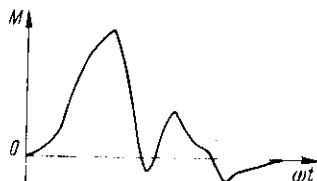
Рис. 5.13. Диаграмма противодействующего момента одного ряда
