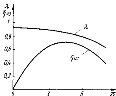
Рис. 2.11. Безразмерные характеристики ступени поршневого компрессора
