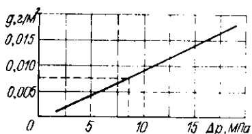
Рис. 10.2. Зависимость удельного расхода масла от давления
