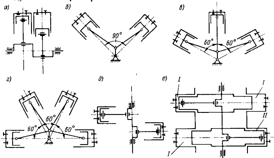
Рис. 6.3. Схемы исполнения компрессоров, унифицированных по цилиндрам: а — вертикальный с числом цилиндров 2; б — V-образный с числом цилиндров 2, 4, 6; в — Ш-образный с числом цилиндров 3 и 6; г — X-образный с числом цилиндров 4 и 8; д — оппозитный с числом цилиндров 2, 4, 6, 8; е — оппозитный двухрядный с числом цилиндров в первой ступени — 3; во второй ступени — 1 и обводным крейцкопфом при D_I = D_{II} (I, II — порядковые номера ступеней сжатия).
