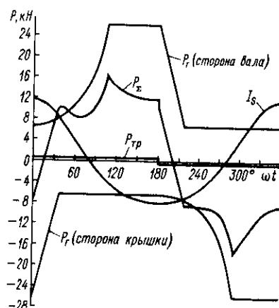
Рис. П.5. Силловые диаграммы для ряда со второй ступенью
