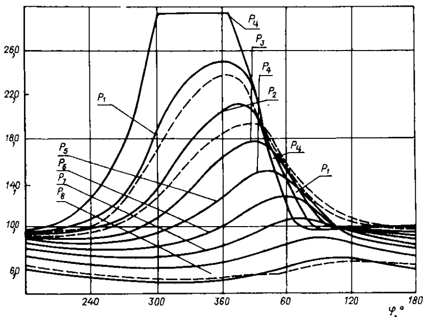
Рис. 8.1. Расчетные зависимости давлений в цилиндре и межкольцевых объемах уплотнения поршня от угла поворота вала \varphi при P_H = 10 МПа, \Pi = 3 ; a = 0,3 и числе колец в уплотнении z = 9 ;
