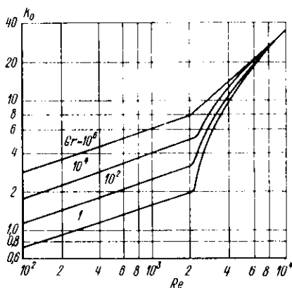
Рис. 9.9. Зависимость \alpha_0 при ламинарном и переходном режимах течения от числа Рейнольдса
