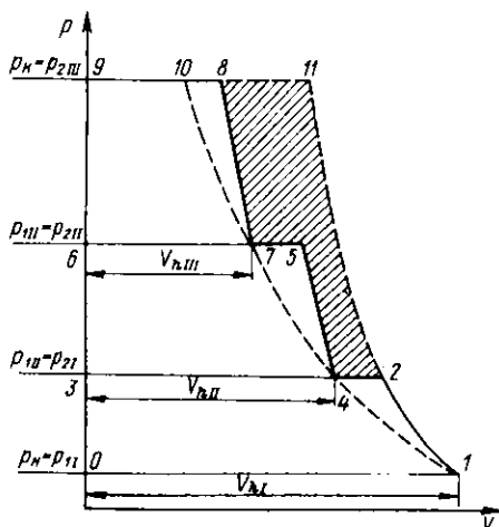
Рис. 3.2. Индикаторные диаграммы многоступенчатого и одноступенчатого сжатия при теоретическом процессе: F_{0-1-11-9-0} — площадь, отражающая индикаторную работу при сжатии и перемещении газа от p_{н1} до p_{н2} в одной ступени; F_{0-1-2-4-3-7-8-9-0} — площадь, отражающая индикаторную работу при сжатии и перемещении газа в трех ступенях; F_{2-4-5-7-8-11-2} — площадь, отражающая уменьшение индикаторной работы при сжатии газа в трех ступенях
