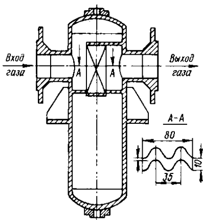
Рис. 9.10. Жалюзийный водомаслоотделитель
