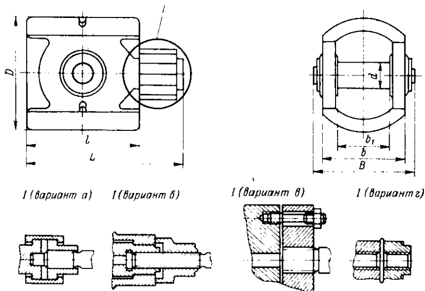
рис. 6.26. Основные конструктивные параметры крейцкопфов
