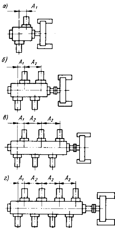
Рис. 6.8. Базы оппозитные: а — двухрядная; б — четырехрядная; в — шестирядная; г — восьмирядная
