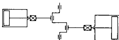
Рис. 4.2. Схема оппозитного компрессора
