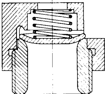
Рис. 7.6. Схема тарельчатого клапана
