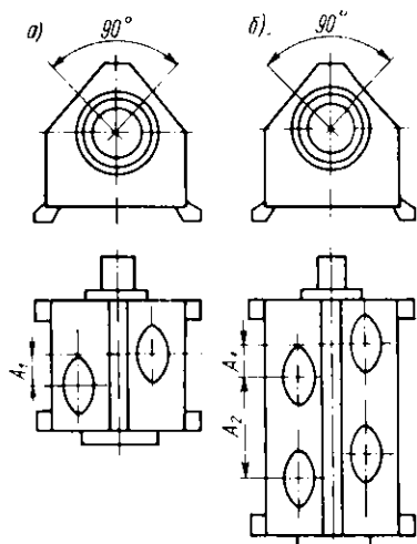
Рис. 6.6. Базы У-образные: а — двухрядная; б — четырехрядная
