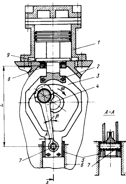
Рис. 12.3. Поперечный разрез по ряду компрессора с обводным крейцкопфом:
