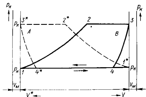
Рис. 2.7. Схематизированные индикаторные диаграммы рабочих полостей ступени с дисковым поршнем:
