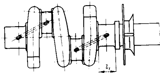
Рис. 6.14. Конструкция составного кривошипного вала
