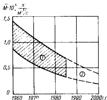
Рис. 6.1. Диаграмма снижения удельной металлоемкости компрессоров общего назначения с производительностью \bar{V} = 0,15 \pm 2,0 \text{ м}^3/\text{с} :
