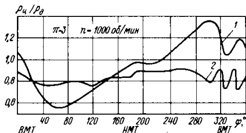
Рис. 11.7. Зависимость отношения плотности газа в цилиндре \rho_{\text{ц}} и дополнительном мертвом пространстве \rho_{\text{д}} от угла поворота коленчатого вала \varphi :
