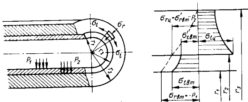
Рис. 6.34. Напряжение в толстостенном цилиндре с запрессованной втулкой
