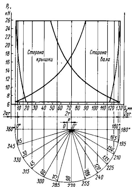
Рис. П.2. Индикаторные диаграммы полостей первой ступени
