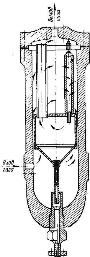
Рис. 9.12. Фильтрующий водомаслоотделитель
