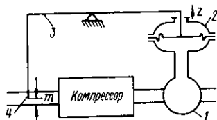
Рис. 11.3. Схема стабилизации давления газа в газосборнике:
