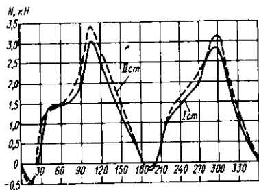
Рис. П.6. Диаграммы нормальных сил
