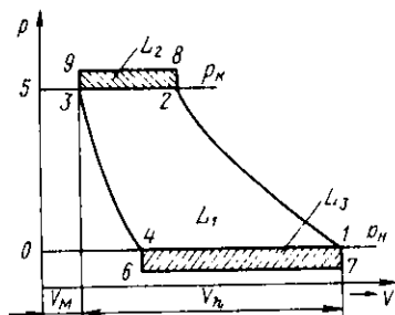
Рис. 2.9. Вторая схематизация индикаторной диаграммы: L_1 — номинальная адиабатная работа; L_2 — работа проталкивания через клапаны линии нагнетания; L_3 — работа проталкивания через клапаны линии всасывания; 4—1 — постоянное давление p_{\text{ж}} ; 2—3 — постоянное давление p_{\text{н}} ; 1—2 и 3—4 — адибаты
