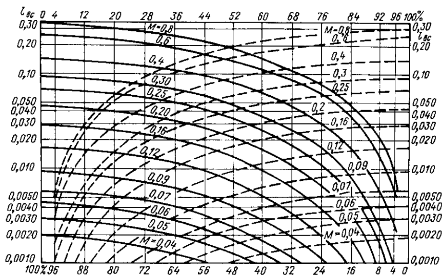
Рис. 7.17. Безразмерная диаграмма теоретической работы, теряемой во всасывающем клапане:
