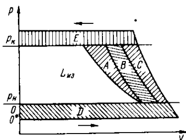
Рис. 2.10. Влияние различных факторов на индикаторную работу:
