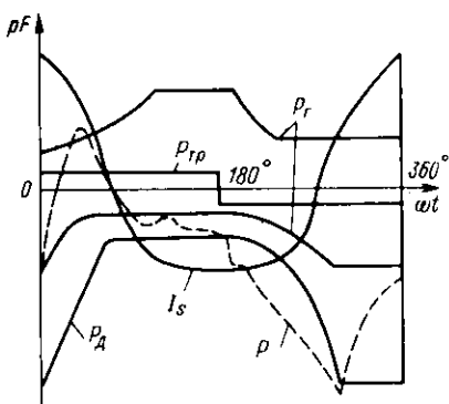
Рис. 5.12. Силовые диаграммы
