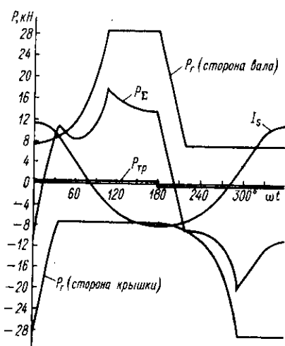
Рис. П.4. Силловые диаграммы для ряда с первой ступенью
