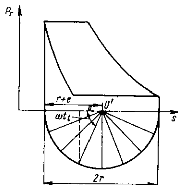
Рис. 5.11. Графический метод учета поправки на конечную длину шатуна
