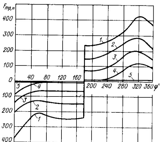
Рис. 8.8. График сил трения кольца в зависимости от угла поворота вала при переходе от контактного к лабиринтному режиму работы:
