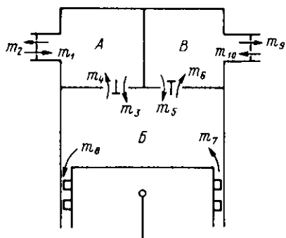
Рис. 2.3. Схема потоков газа в одноступенчатом компрессоре с тронковым поршнем: А — полость всасывающих клапанов; Б — полость цилиндра; В — полость нагнетательных клапанов
