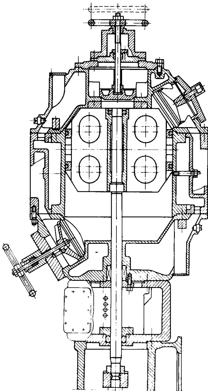
Рис. 6.32. Схема цилиндра оппозитного компрессора
