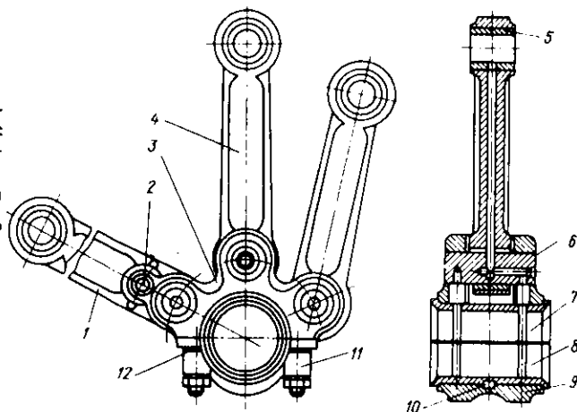
Рис. 6.22. Конструкция узла с прицепными шатунами:
