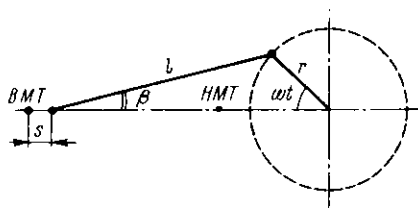
Рис. 5.1. Схема кривошипного механизма
