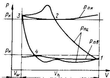
Рис. 2.4. Кривые изменения давления в зависимости от объема цилиндра: p_{пв} — в полости всасывания; p_{пн} — в полости нагнетания; p_{цц} — в полости цилиндра; 1—2 — сжатие; 2—3 — нагнетание; 3—4 — расширение; 4—1 — всасывание газа
