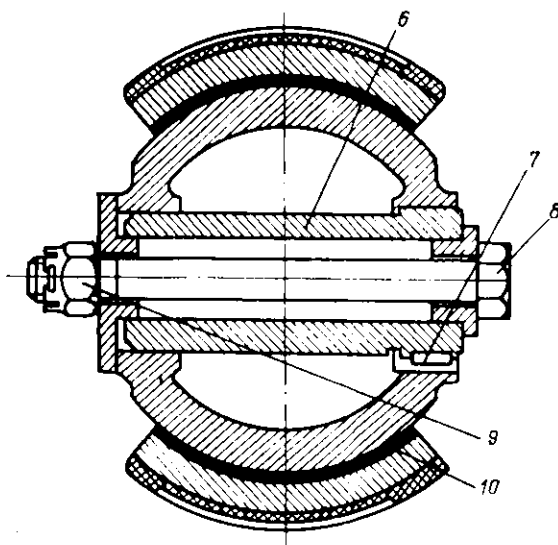
Рис. 6.24. Конструкция закрытого кресткопфа со съемными башмаками:
