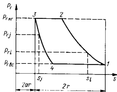
Рис. 5.10. Схематизированная индикаторная диаграмма:
