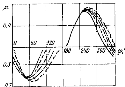
Рис. 11.8. График изменения коэффициента \mu от угла поворота вала \varphi :
