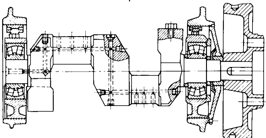
Рис. 6.16. Конструкция двухопорного коленчатого вала многорядного компрессора
