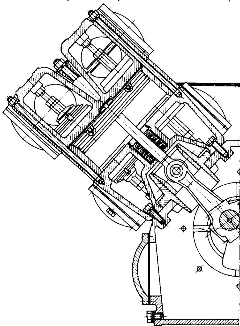
Рис. 12.4. Поперечный разрез У-образного
