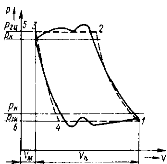
Рис. 2.8. Первая схематизация индикаторной диаграммы:
