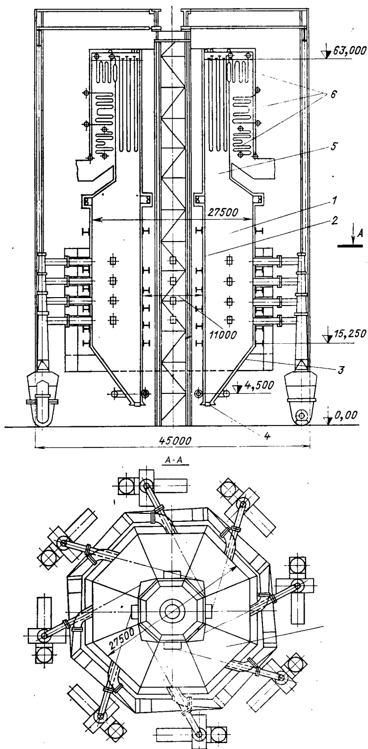
Рис. 27.10. Энергетический котел на 800 МВт с кольцевой топкой
