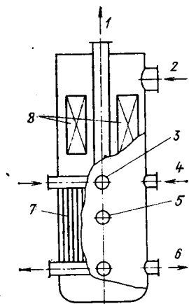
Рис. 31.3. Устройство сепаратора-пароперегревателя (СПП):
