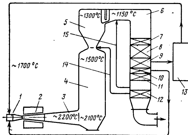
Рис. 27.13. Структурная схема парогенератора МГД электростанции:
