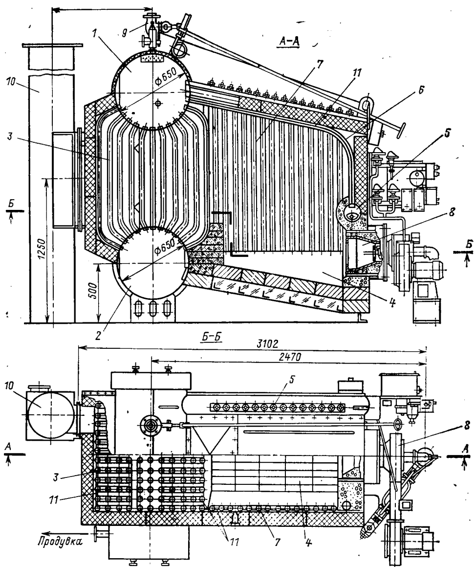
Рис. 26.2. Двухбарабанный вертикальный водотрубный стационарный паровой котел с естественной циркуляцией ПО «Красный котельщик» типа Е-1-9-1 Г:
