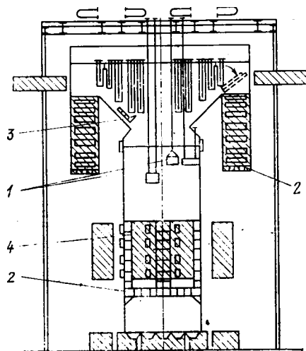
Рис. 28.4. Схема организации ремонтных работ на котле: 1 — установка подвесных площадок; 2 — установка настилов; 3 — установка лестниц-площадок; 4 — установка лесов. Заштрихованы зоны ремонтного обслуживания
