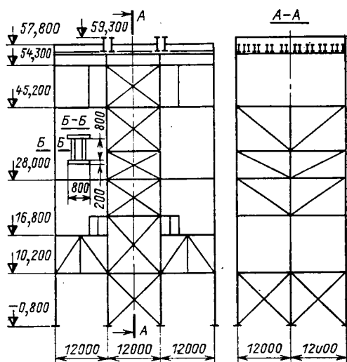
Рис. 24.2. Схема каркаса прямоточного котла на СКД к блоку 500 МВт
