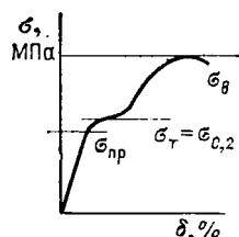
Рис. 23.1. Диаграмма напряжений для стали
