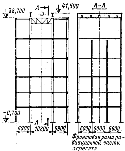
Рис. 24.1. Каркас парового котла ТП-100
