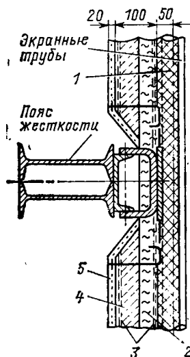
Рис. 24.9. Натрубная обмуровка с поясом жесткости:
