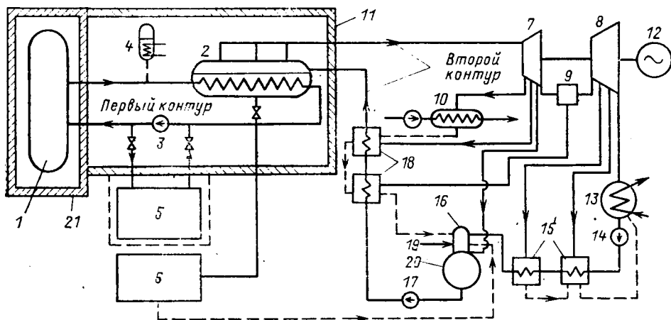
Рис. 31.2. Двухконтурная тепловая схема АЭС с водным теплоносителем:
