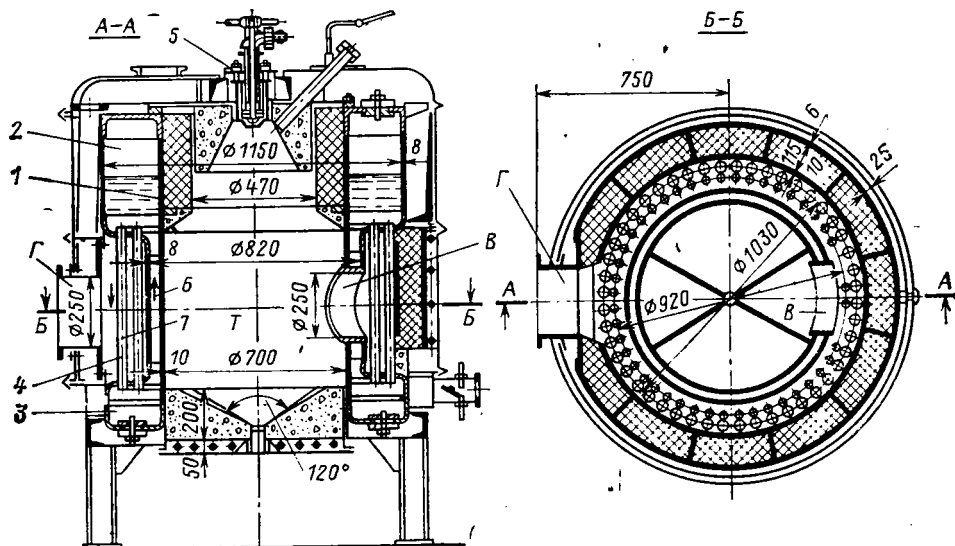
Рис. 26.1. Вертикальный паровой котел с естественной циркуляцией, на газе с наддувом на 0,11 кг/с (0,4 т/ч), 0,9 МПа <
