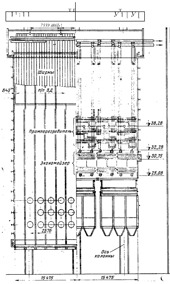
Рис. 27.8. Продольный и поперечный разрезы котла ТГМП-1204 на 1200 МВт
