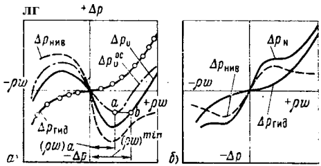
Рис. 15.5. Гидравлические характеристики для панелей из труб:
