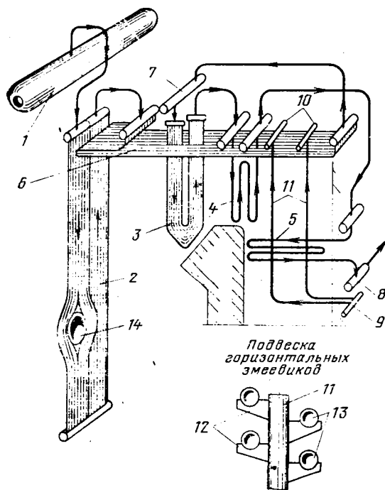
Рис. 2.6. Основные конструктивные элементы пароперегревателя:
