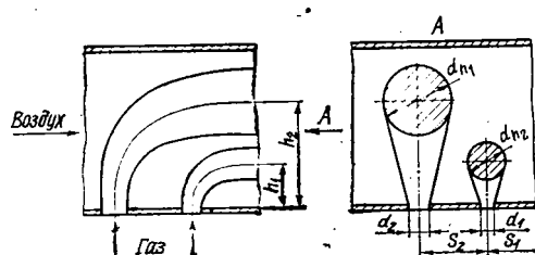
Рис. 9.2. Струйный способ смешения
