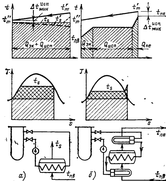
Рис. 31.7. Циклы и параметры парогенераторов в двухконтурных АЭС с ВВЭР
