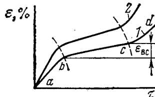
Рис. 23.2. Диаграмма ползучести стали при различных температурах: 1 — при температуре А; 2 — при температуре \langle | \epsilon | \rangle \langle | \epsilon | \rangle / 2
