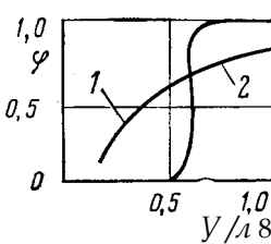
Рис. 13.4. Изменение истинного паросодержания по высоте поперечного сечения горизонтальной трубы: 1 — при \phi_0 = 0,40 ; 2 — при \phi_0 = 0,88 . Примечание: ось y направлена вертикально по диаметру трубы
