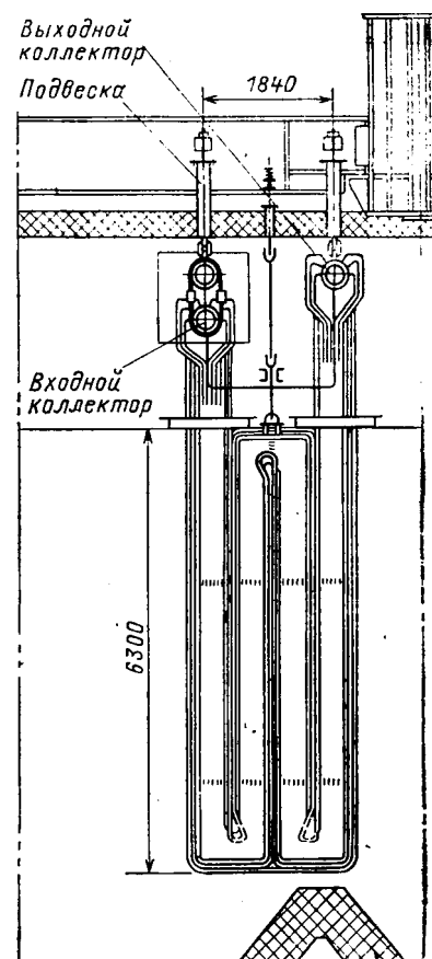
Рис. 17.7. Ширмовый пароперегреватель котла на СКД к блоку 500 МВт
