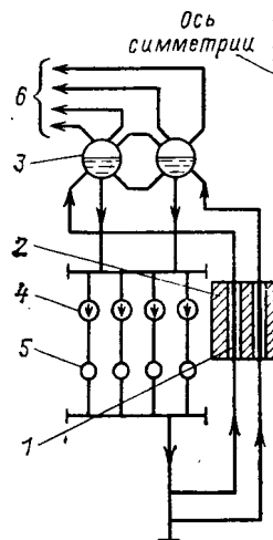
Рис. 31.6. Циркуляционная система кипящего канального реактора РБМК-1000:
