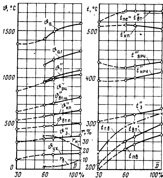
Рис. 28.5. Результаты тепловых расчетов котла П-67 энергоблока 800 МВт для различных нагрузок
