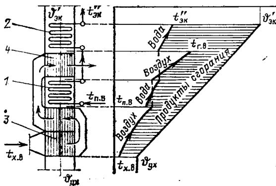
Рис. 17.13. Температурные напоры при двухступенчатой компоновке воздухоподогревателя экономайзера:
