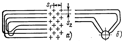
Рис. 17.10. Четырехпетлевая схема включения трубной поверхности:
