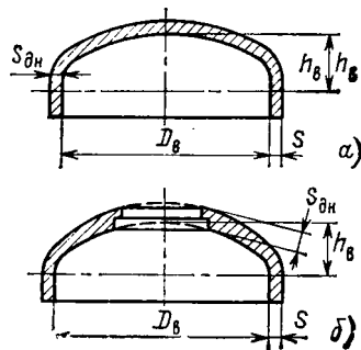
Рис. 23.4. Выпуклые эллиптические днища:
