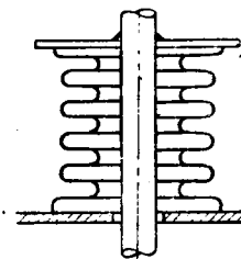
Рис. 24.12. Сильфонное уплотнение при переходе трубопровода через стенку короба
