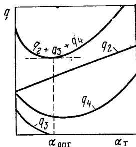
Рис. 5.3. Оптимальное значение a_m для твердых топлив
