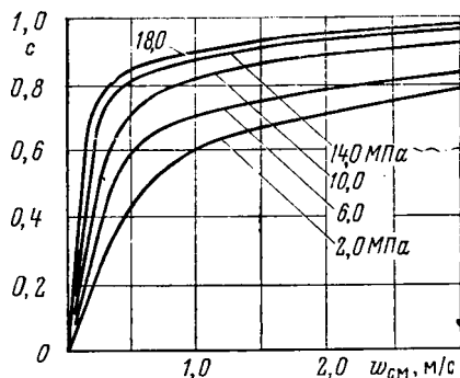
Рис. 13.8. Значение коэффициента c в ления: формуле для Определения \phi у вертикальных подъемных труб
