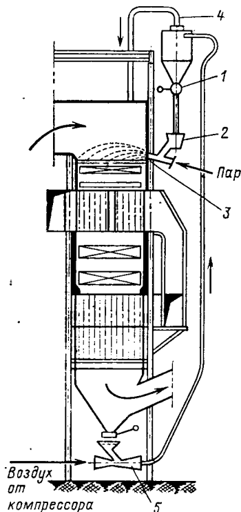
Рис. 20.13. Схема дробеочистки под давлением:
