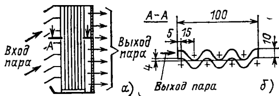
Рис. 19.7. Жалюзийный сепаратор: а — конструкция жалюзийного пакета; б — профиль жалюзи
