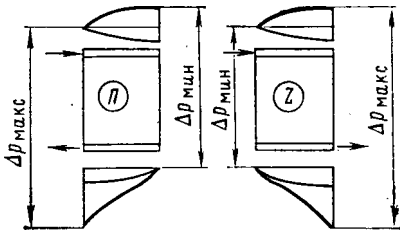
Рис. 15.11. Сравнение перепадов давлений в пароперегревателях с гидравлическими схемами П и I
