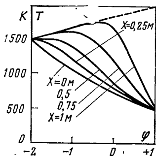
Рис. 6.13. Распределение тем- ператур горящего топлива
