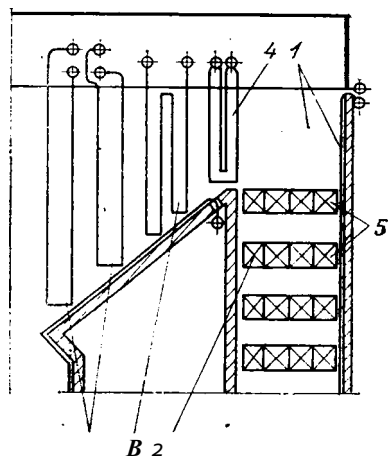
Рис. 15.14. Развернутая гидравлическая схема пароперегревателя прямоточного котла энергоблока 500 МВт (одного потока)
