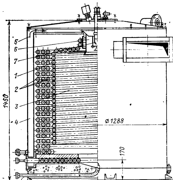
Рис. 26.3. Передвижной прямоточный котел ППК-1600:
