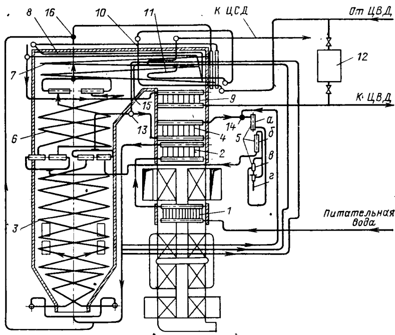
Рис. 27.2. Схема прямооточного котла на 75 кг/с (270 т/ч) с промывочно-сепарационной установкой
