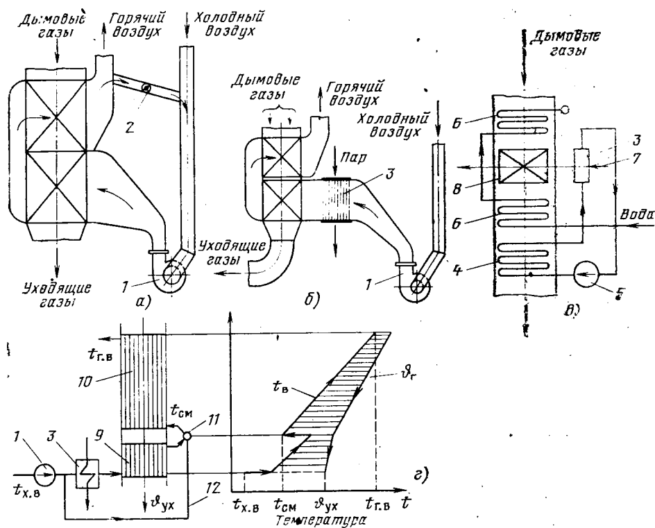
Рис. 17.14. Схемы устройств повышения температуры холодного воздуха в воздухоподогревателе:
