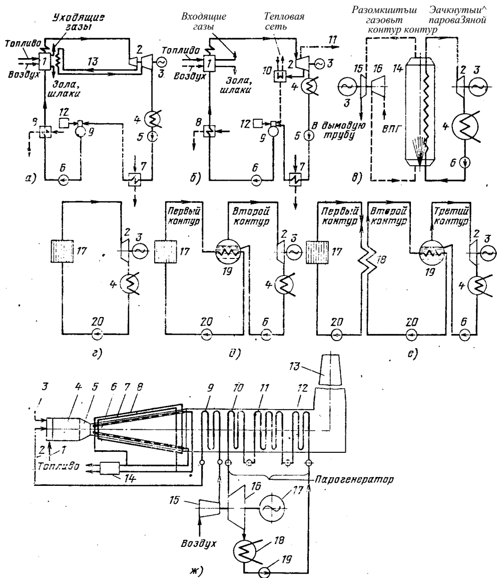
Рис. В.3. Схема использования паропроизводящих аппаратов в энергетике:
