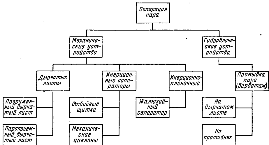
Рис. 19.2. Схема современных паро-сепарационных устройств
