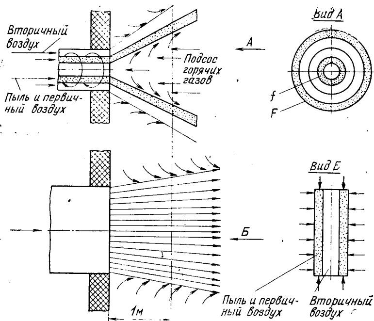
Рис. 9.10. Смесеобразование и зажигание в вихревой и. прямоточной горелках
