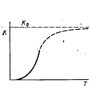
Рис. 6.1. Зависимость константы скорости реакции от температуры
