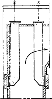
Рис. 17.3. Пример размеще- ния двухсветных поверхностей нагрева в верхней части топки
