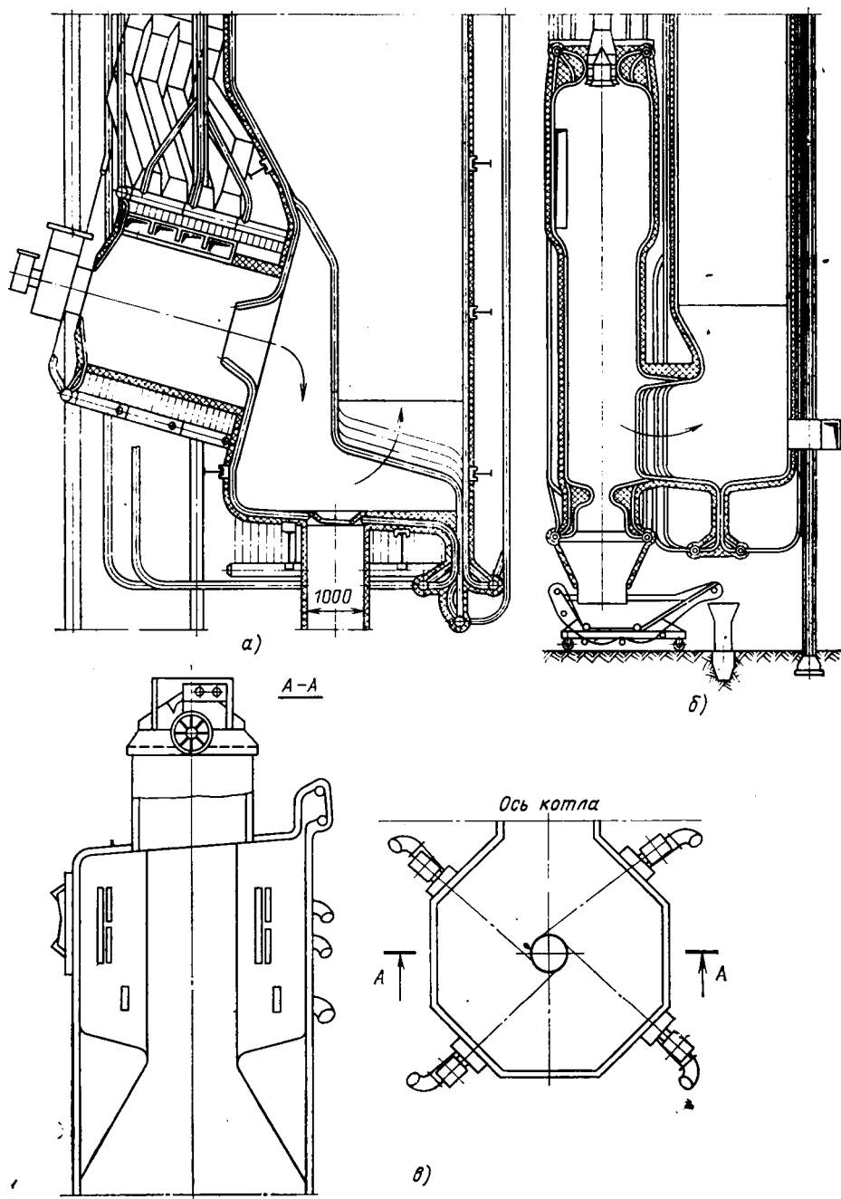
Рис. 9.14. Высокофорсированные камеры сгорания с жидким шлакоудалением
