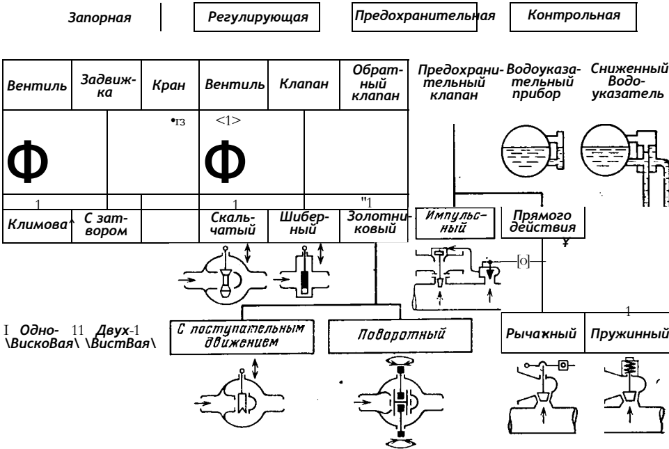
Рис. 25.4. Классификация основных видов арматуры
