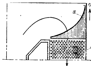
Рис. 20.4. Диаграммы к низкотемпературной коррозии
