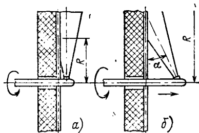
Рис. 20.9. Средства интенсификации паровой (воздушной) обдувки
