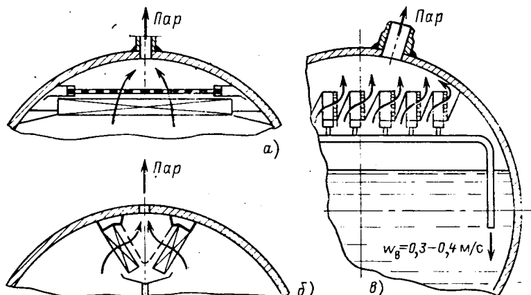
Рис. 19.8. Компонка жалюзийных сепараторов в барабане парового котла я парогенератора АЭС:
