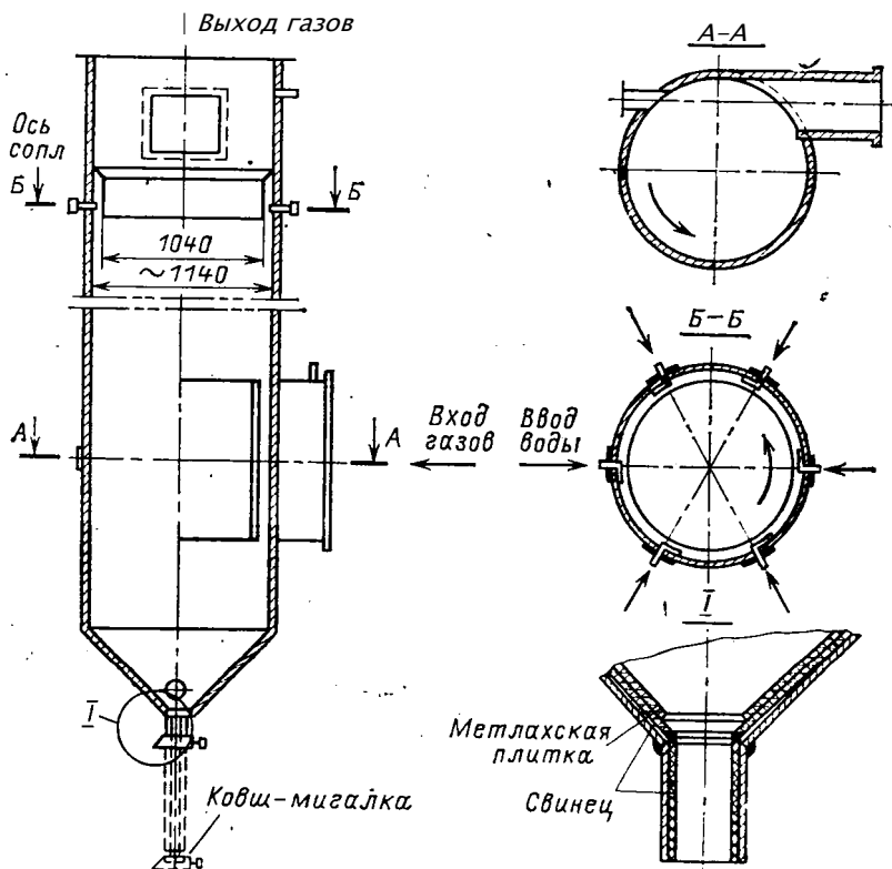
Рис. 30.4. Центробежный скруббер-золоуловитель
