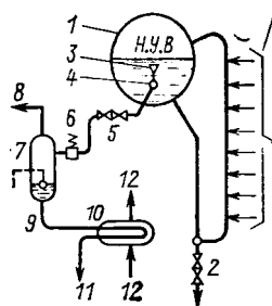
Рис. 18.11. Принципиальная схема устройства продувки барабанного котла:
