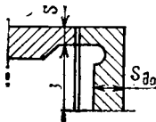
Рис. 23.5. Приварка донышка к коллектору
