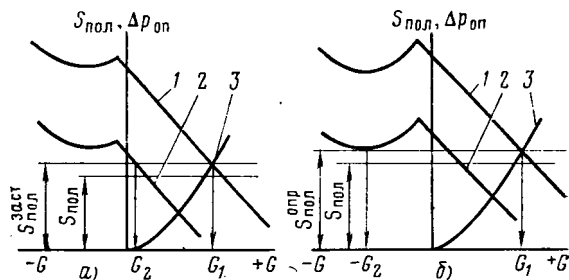
Рис. 14.5. Циркуляционные характеристики:
