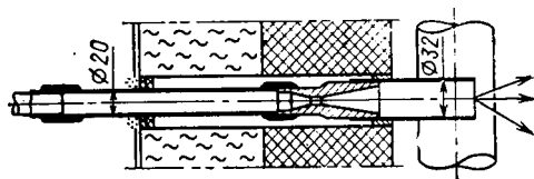
Рис. 20.10. Аппарат для водяной обмывки
