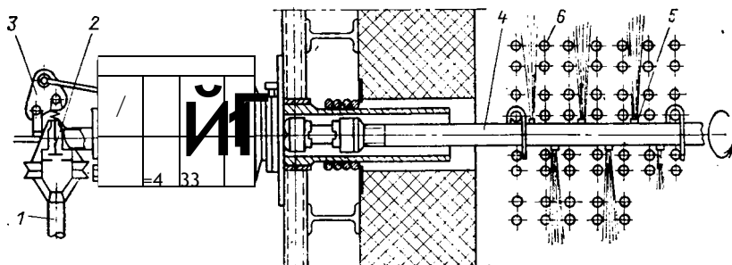
Рис. 20.6. Паровой обдувочный прибор ОПК-7 конвективного перегревателя:
