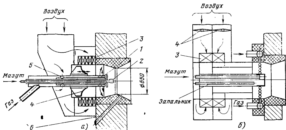
Рис. 9.7. Газомазутные горелки:
