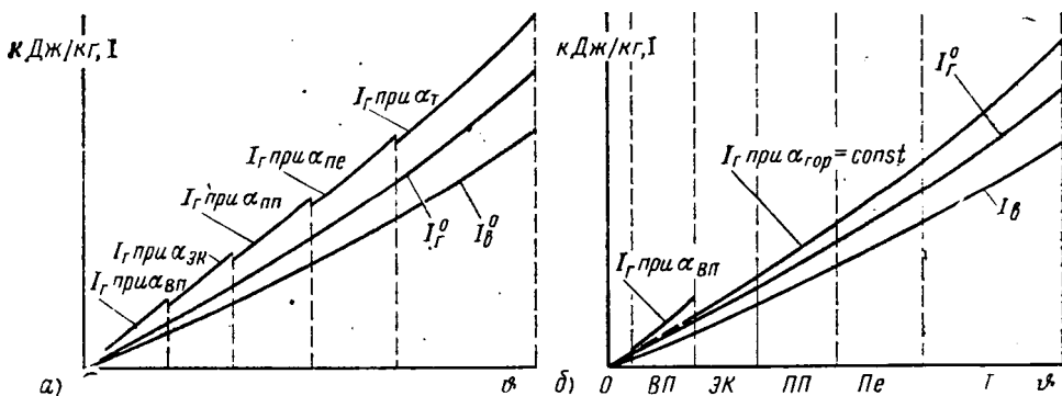
Рис. 4.1. /, -в-диаграмм а для воздуха и продуктов сгорания при уравнишенной тяге (а) и наддуве (б)
