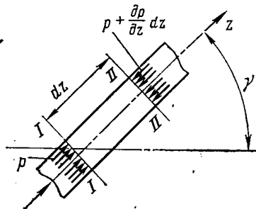
Рис. 13.1. Элемент жидкости, нагруженный силами давления
