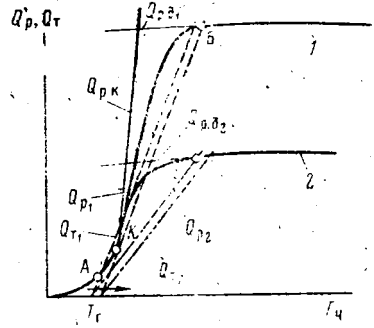
Рис. 6.5. Кинетический и диффузионный режимы горения: 1 — для мелких частиц; 2 — для крупных частиц
