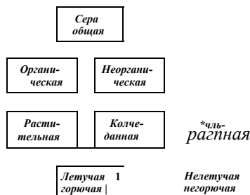
Рис. 3.2. Природа и свойства серы в топливе
