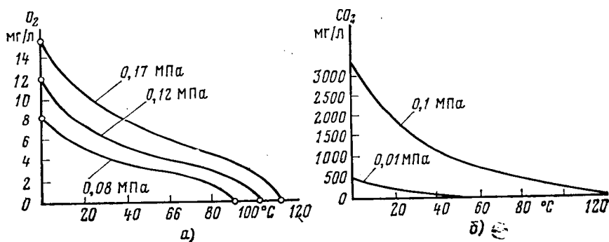
Рис. 18.10. Содержание растворенных в воде газов, определяемое температурой и давлением
