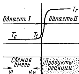
Рис. 6.9. Схема распространения фронта ламинарного пламени
