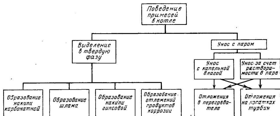
Рис. 18.4. Схема поведения примесей воды в котле
