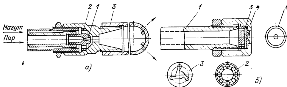
Рис. 9.5. Форсунки с паровым и механическим распыливанием:
