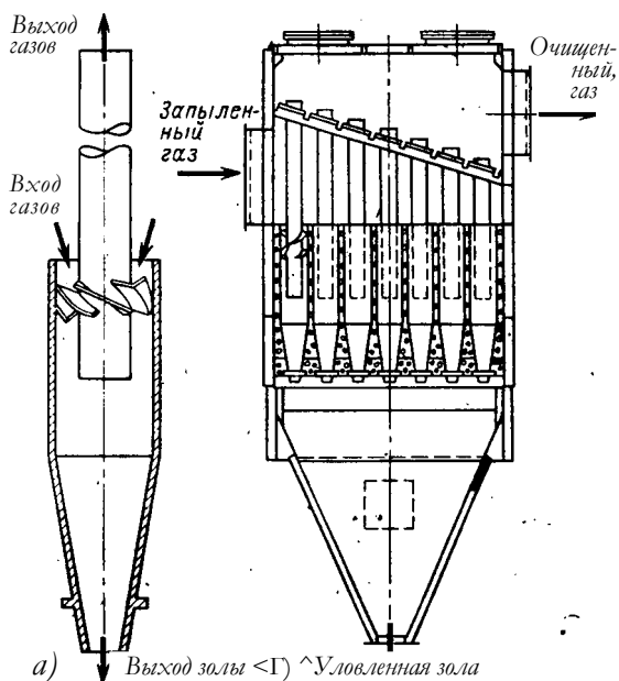
Рис. 30.3. Инерционный батарейный циклон-золоуловитель
