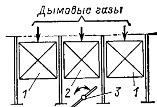
Рис. 21.11. Схема байпасирования газов при регулировании перегрева вторичного пара: 1 — вторичный пароперегреватель; 2 — экономизер; 3 — регулирующий шибер
