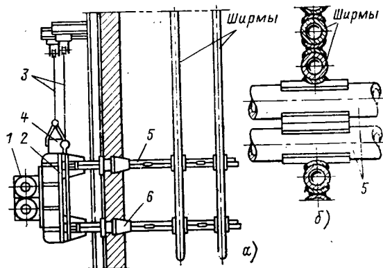
Рис. 20.14. Вибрационное устройство очистки шпирмового перегревателя:
