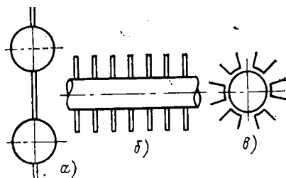
Рис. 27.14. Варианты оребрений конвективных поверхностей: а — мембранное; б — поперечное; в — продольное
