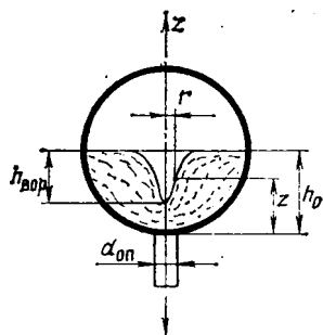
Рис. 14.6. Вихревая воронка при входе воды в опускную трубу
