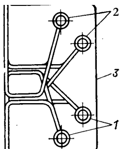
Рис. 24.11. Узел разъема экрана: / — выходные коллекторы; 2 — входные коллекторы; 3 — уплотняющий короб
