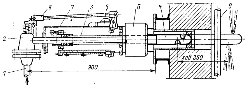
Рис. 20.7. Маловыдвижной обдувочный аппарат типа ОМ-0,35:
