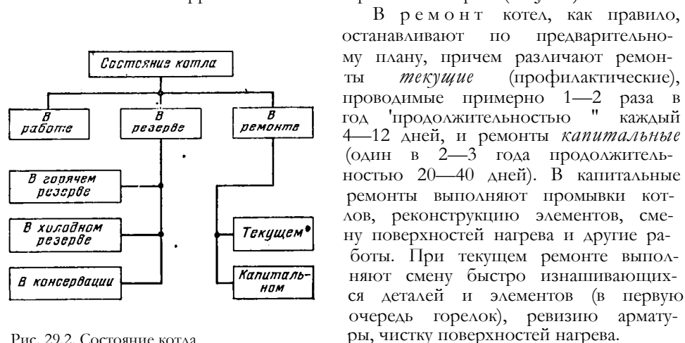
Рис. 29.2. Состояние котла
