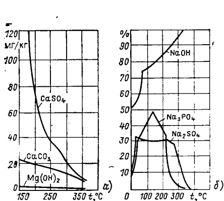
Рис. 18.2. Растворимость основных накипеобразователей (а) и основных легкорастворимых соединений (б) в зависимости от температуры воды.
