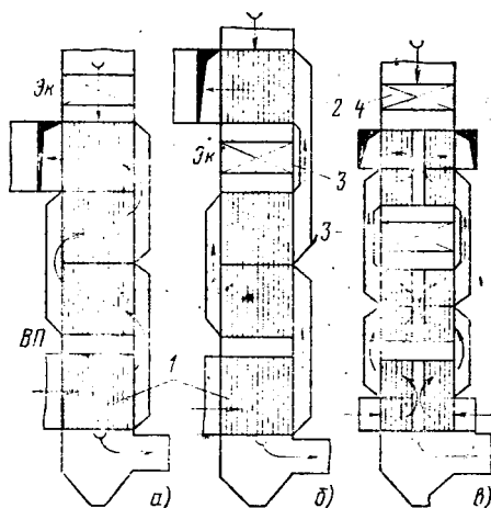
Рис. 2.9. Конструктивные схемы рекуперативных трубчатых воздухоподогревателей в зависимости от \angle T -в и мощности агрегата:
