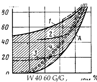
Рис. 12.4. Характеристика эффективности систем регулирования тягодутьевых машин
