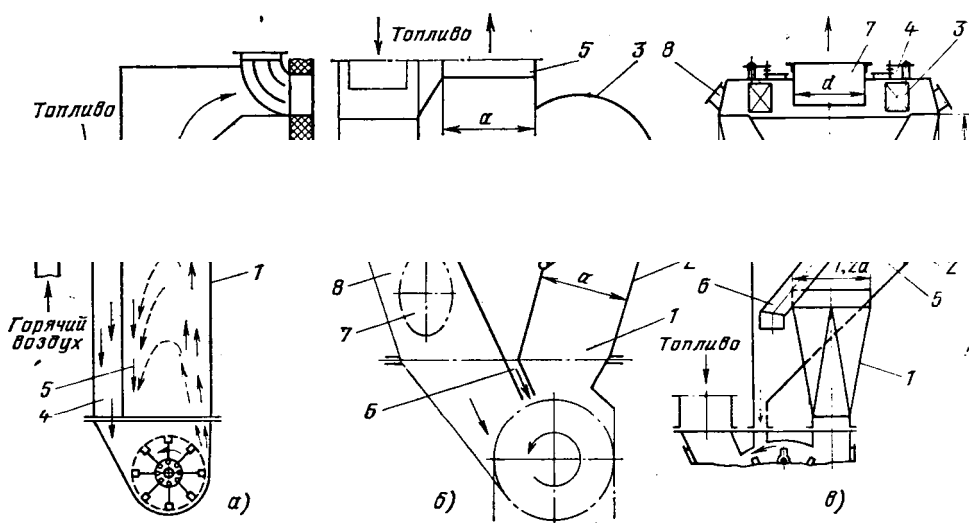
Рис. 8.9. Типы мельничных сепараторов:
