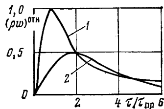
Рис. 21.4. Динамика изменения массовой скорости при тепловом возмущении скачком +X-
