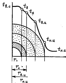
Рис. 25.2. Распределение температур в сечении изолированного трубопровода
