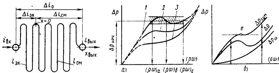
Рис. 15.1. Изменение энтальпии по длине витка проточного котла на докритическое давление; Рис. 15.2. Гидравлические характеристики витков
