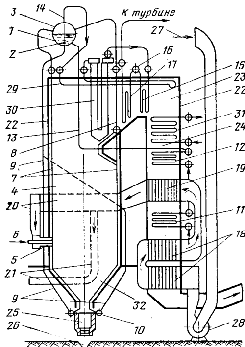
Рис. 1.2. Схема устройства парового котла с естественной циркуляцией
