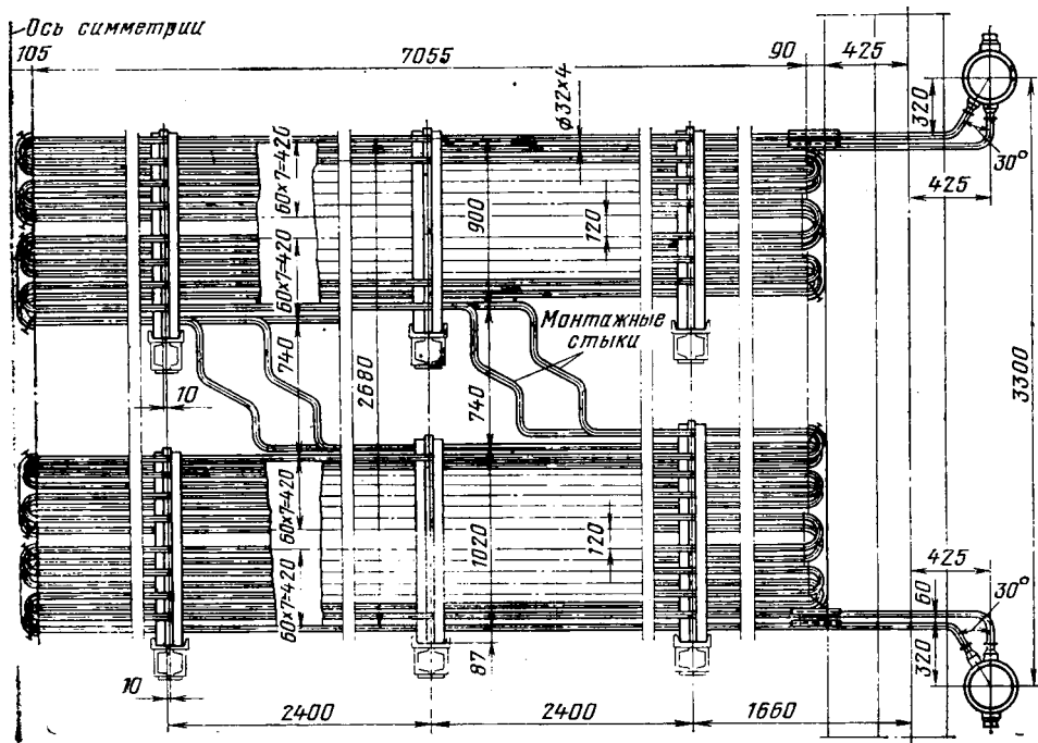
Рис. 17.11. Компоновка экономайзера
