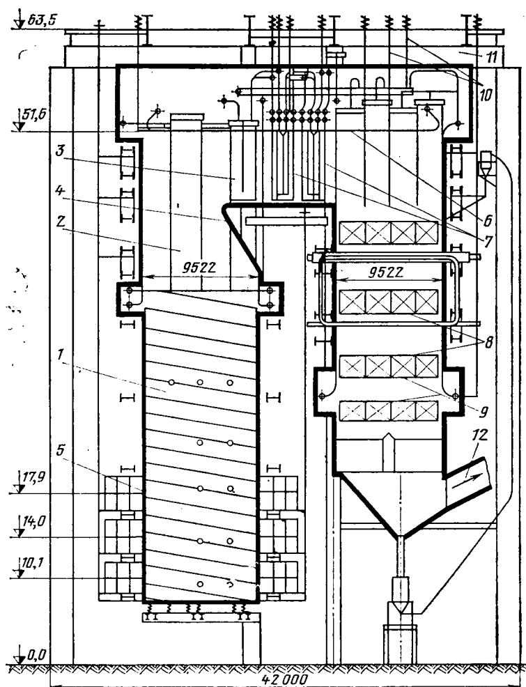
Рис. 27.6. Продольный разрез полуципового котла Пп-1800-140МН на 500 МВт:
