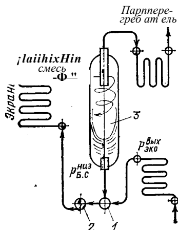
Рис. 15.6. Принцип работы прямо- точного агрегата с дополнительной циркуляцией: 1 — смеситель; 2 — циркуляционный на- сос; 3 — барабан-сепаратор
