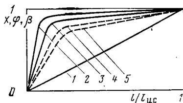
Рис. 13.7. Изменение x , r , \phi на испарительном участке трубы с подъемным движением при \Delta p < \Delta p_{кр} : 1 — x ; 2 — r ; 3 — \phi при p = p_{кр} ; 4 — \phi ; 5 — \phi при p > p_{кр} .
