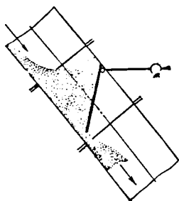
Рис. 8.13. Схема устройства и принцип работы мигалки в прямоугольной топке
