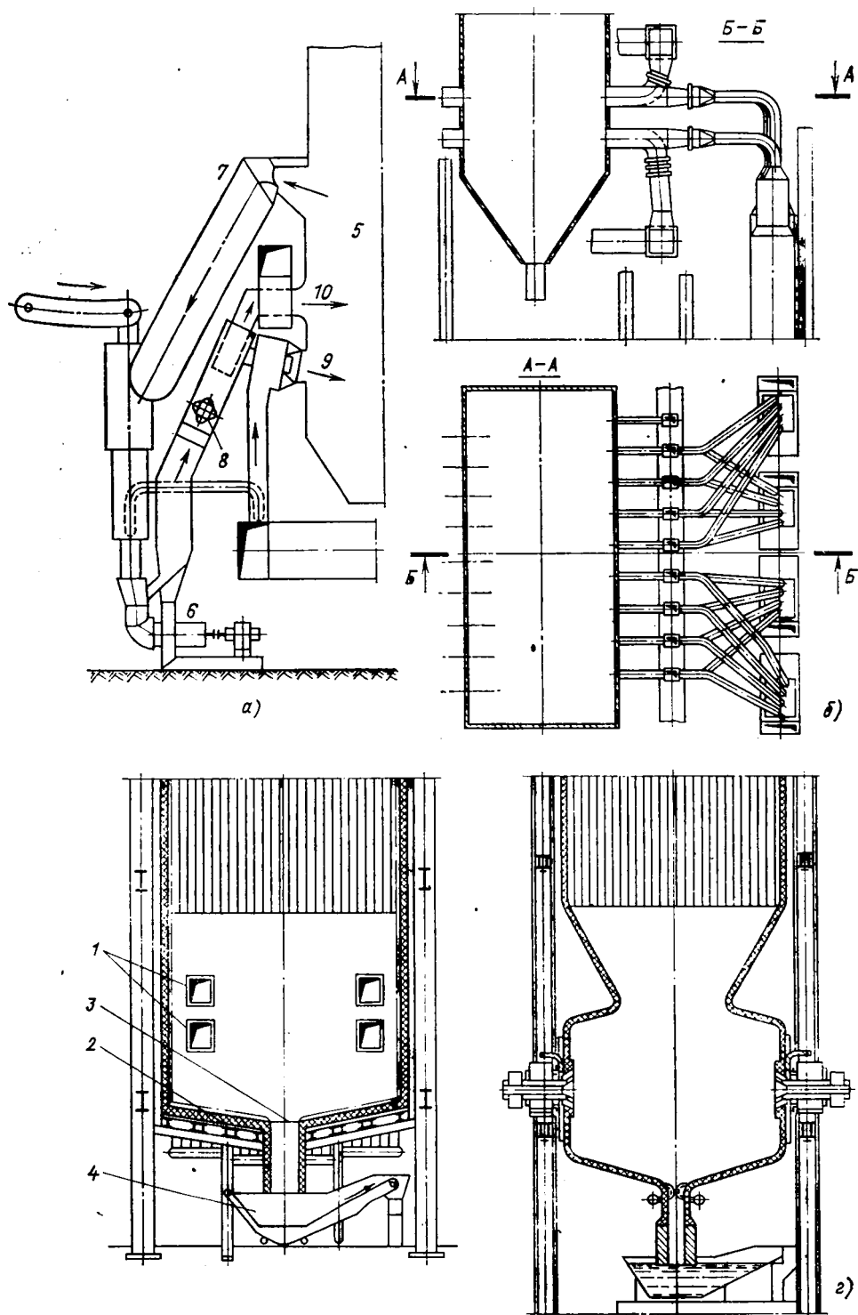
Рис. 9.13. Топко» призматические и с нережимом для сжигания угольной пыли 8—79
