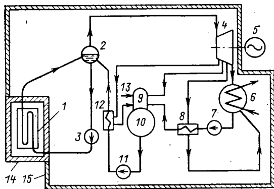
Рис. 31.1. Одноконтурная тепловая АЭС:
