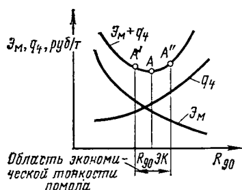
Рис. 8.4. Определение оптимальной тонкости помола
