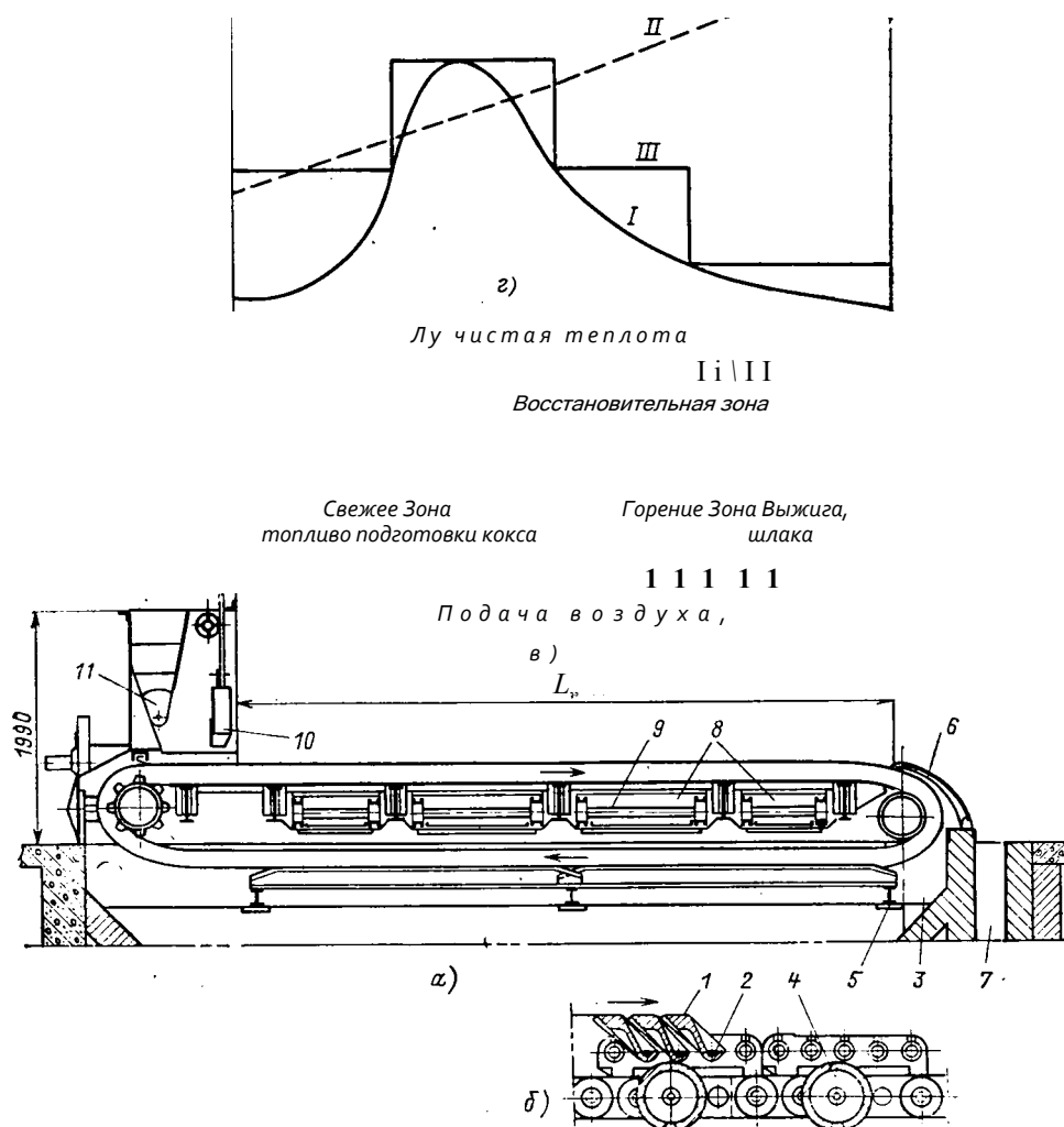
Рис. 7.2. Механическая слоевая топка с решеткой ТЧ и горение на ней топлива
