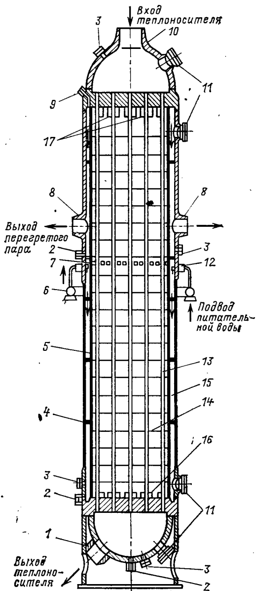
Рис. 31.9. Прямоточный вертикальный парогенератор (США):
