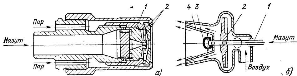
Рис. 9.6. Форсунки комбинированные:
