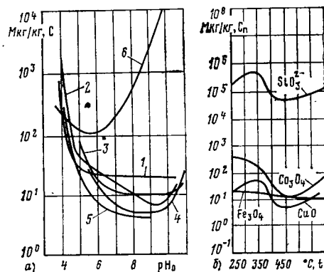
Рис. 18.3. Растворимость окислов металлов в зависимости от рН при температуре кипения воды и давлении 7 МПа (а), изобары растворимости некоторых веществ в рабочей среде СКД при p=25,0 МПа (б):
