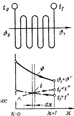
Рис. 11.1. Расчетная схема теплообменника
