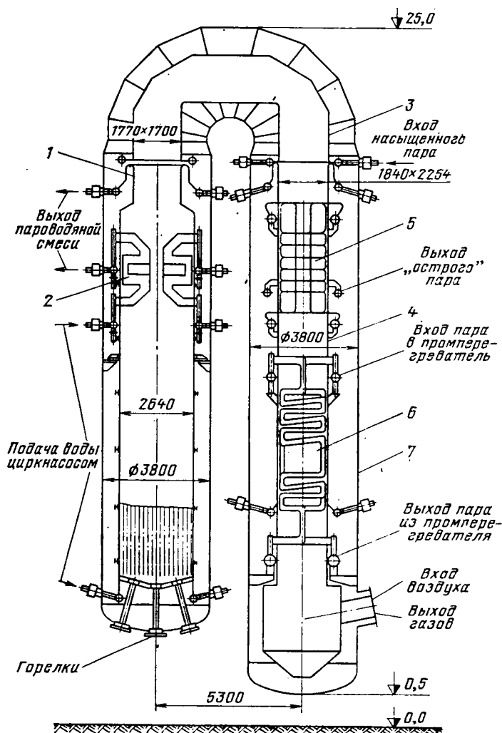
Рис. 27.12. Высоконапорный парогенератор ВПГ-600
