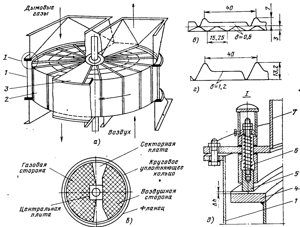
Рис. 2.10. Регенеративный воздухоподогреватель:
