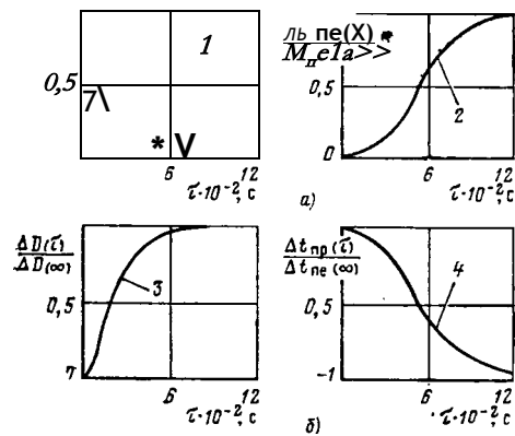
Рис. 21.5. Динамика изменения расхода и температуры перегрева для прямоточного котла СКД при работе на газе:
