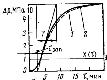
Рис. 22.3. Разгонные кривые котла ТП-87:
