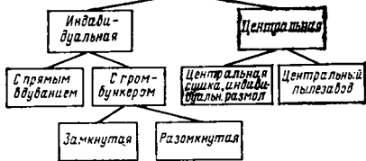
Рис. 8.11. Систематизация применяемых способов пылеприготовления
