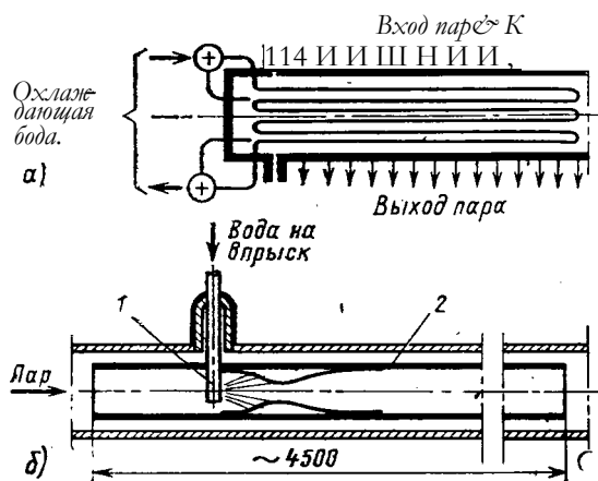
Рис. 21.8. Конструктивная схема пароохладителей: а — поверхностного; б — впрыскивающего; 1 — распыливающая форсунка; 2 — защитные кожух
