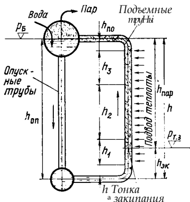
Рис. 14.1. Контур естественной циркуляции
