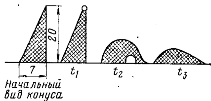
Рис. 3.3. Определение плавкости золы по конусам
