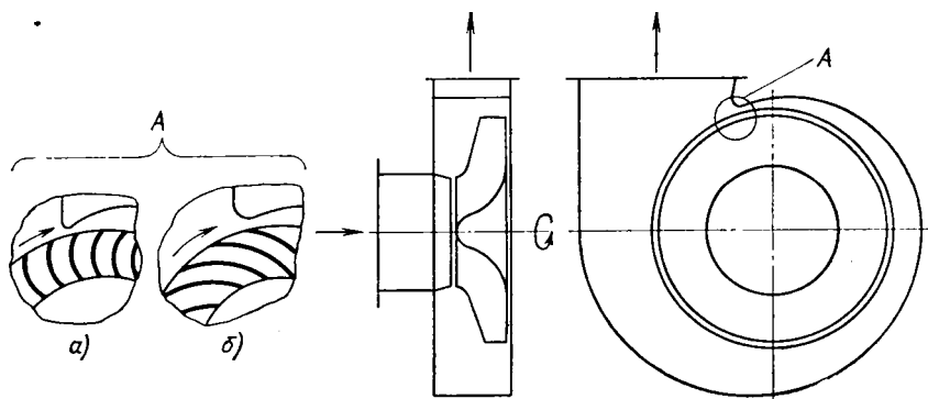
Рис. 12.2. Центробежный (радиальный) вентилятор:
