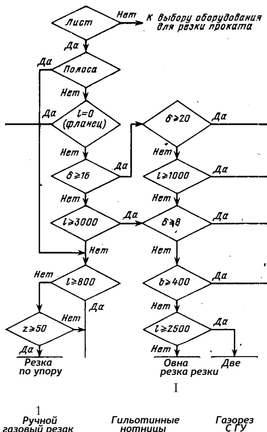
Рис. 28.2. Блок-схема выбора оборудования для резки листовых деталей
