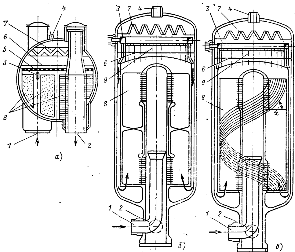
Рис. 31.8. Типы парогенераторов с естественной циркуляцией для ВВЭР:
