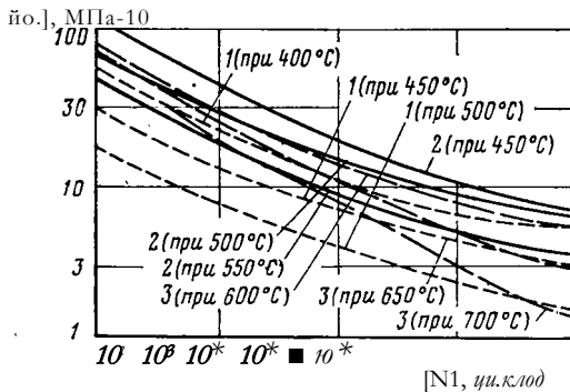
Рис. 23.6. Зависимость [N] от расчетной амплитуды напряжений \sigma_a : / — для углеродистой стали; 2 — для низколегированных сталей; 3 — для аустенитных сталей
