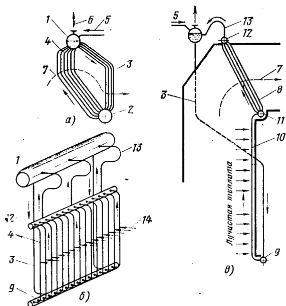
Рис. 2.4. Испарительные поверхности нагрева:
