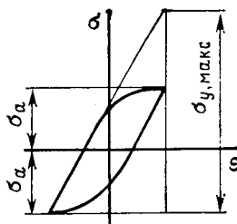
Рис. 25.3. Диаграмма циклического деформирования металла трубопровода
