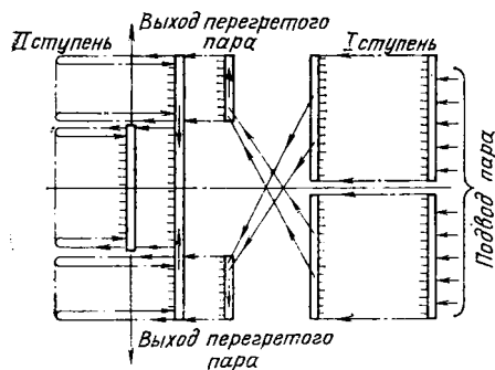
Рис. 15.12. Схема пароперегревателя высокого давления с перебросом
