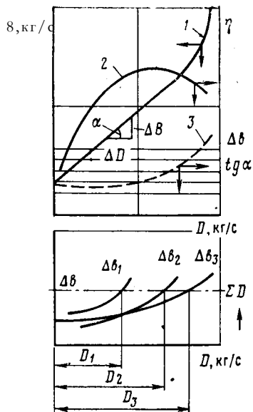
Рис. 29.1. Графическое построение относительного прироста топлива:
