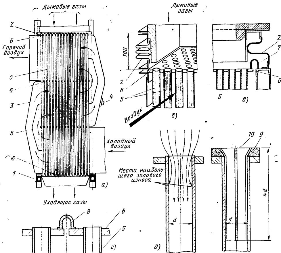
Рис. 2.7. Конструкция стального однопоточного и трехходового по воздуху трубчатого воздухоподогревателя:
