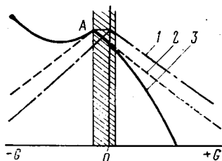
Рис. 14.4. Построение полной циркуляционной характеристики:
