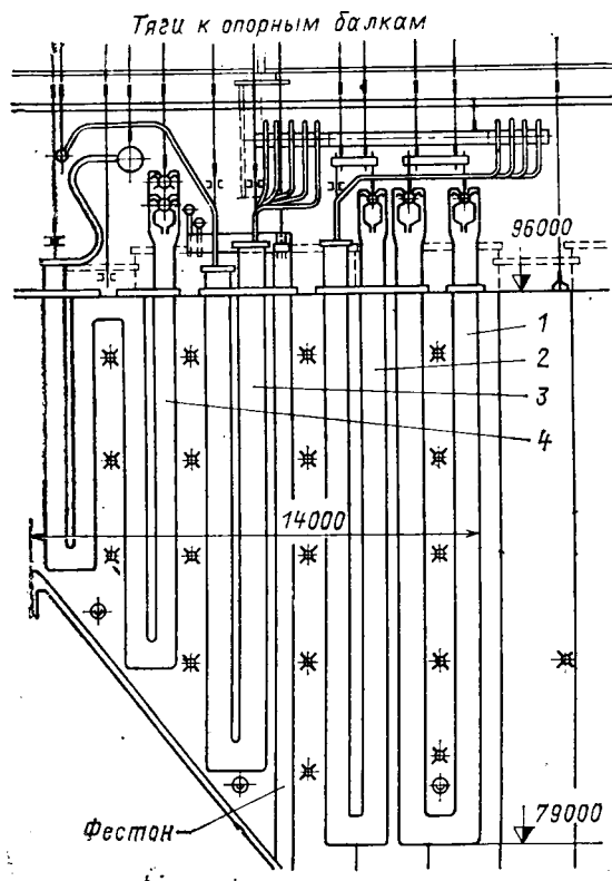
Рис. 17.8. Ширмовые пароперегреватели котла на СКД к блоку 800 МВт:
