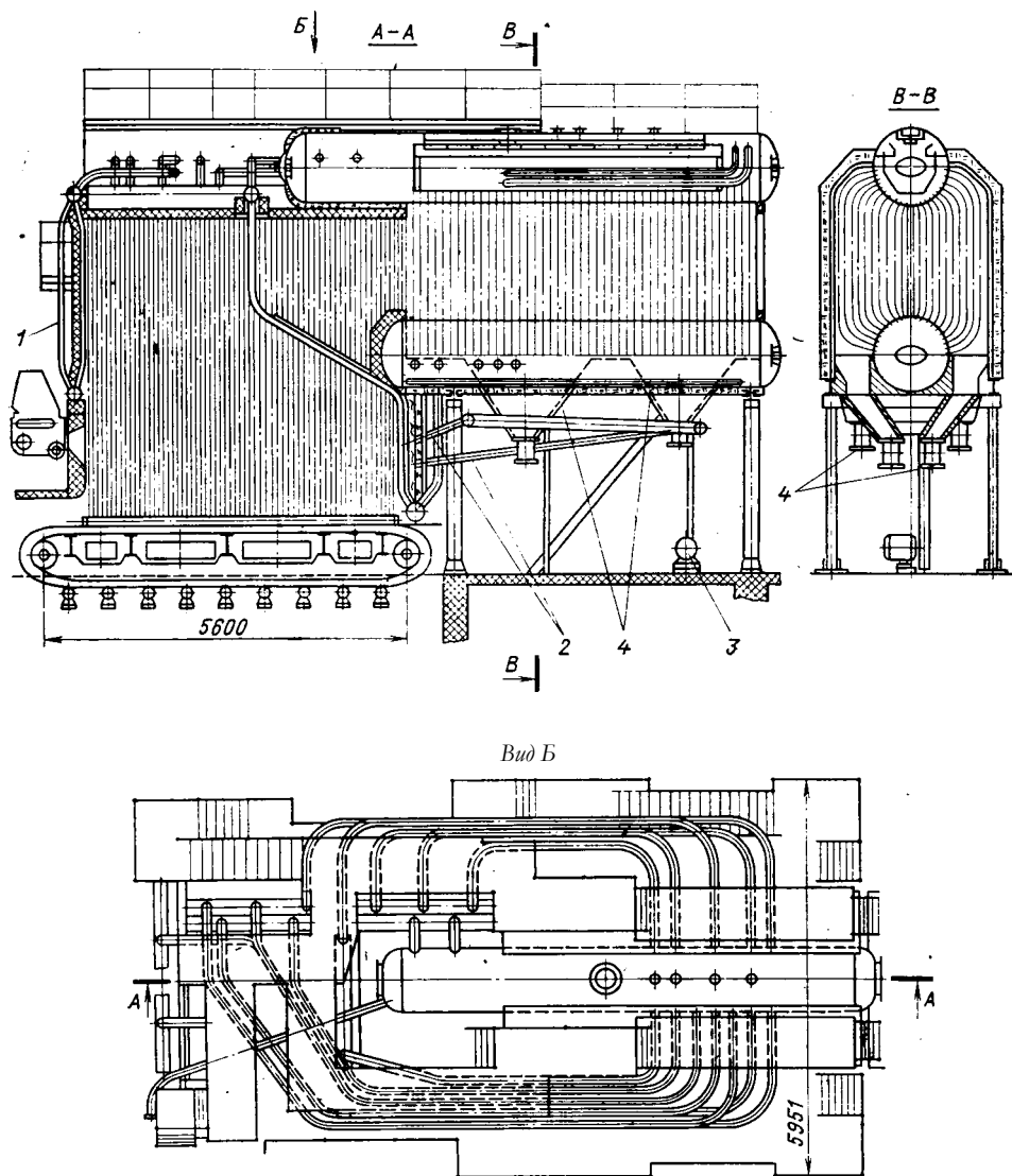
Рис. 26.5. Паровой котел Е-25-14Р (KE-25-14Р)
