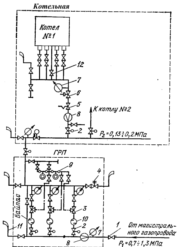
Рис. 8.14. Схема газоснабжения электростанции:
