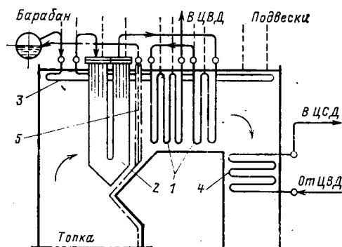
Рис. 17.6. Компоновочная схема пароперегревателей энергетического котла с естественной циркуляцией на большую производительность:
