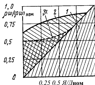
Рис. 15.7. Изменение массовой скорости при переменной нагрузке агрегатов на СКД создает: 1 — питательный насос; 2 — дополнительная циркуляция; 3 — петля естественной циркуляции
