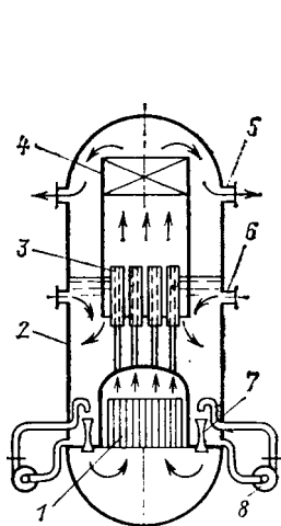
•Рис. 31.5. Элементы кипящего реактора корпусного типа:
