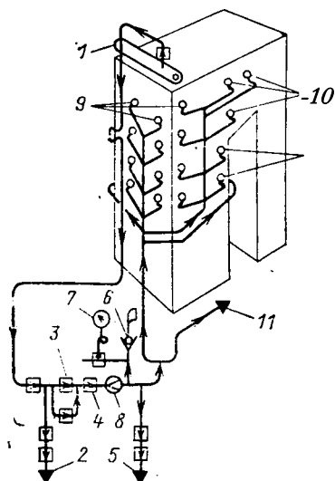
Рис. 20.9. Средства интенсификации паровой (воздушной) обдувки
