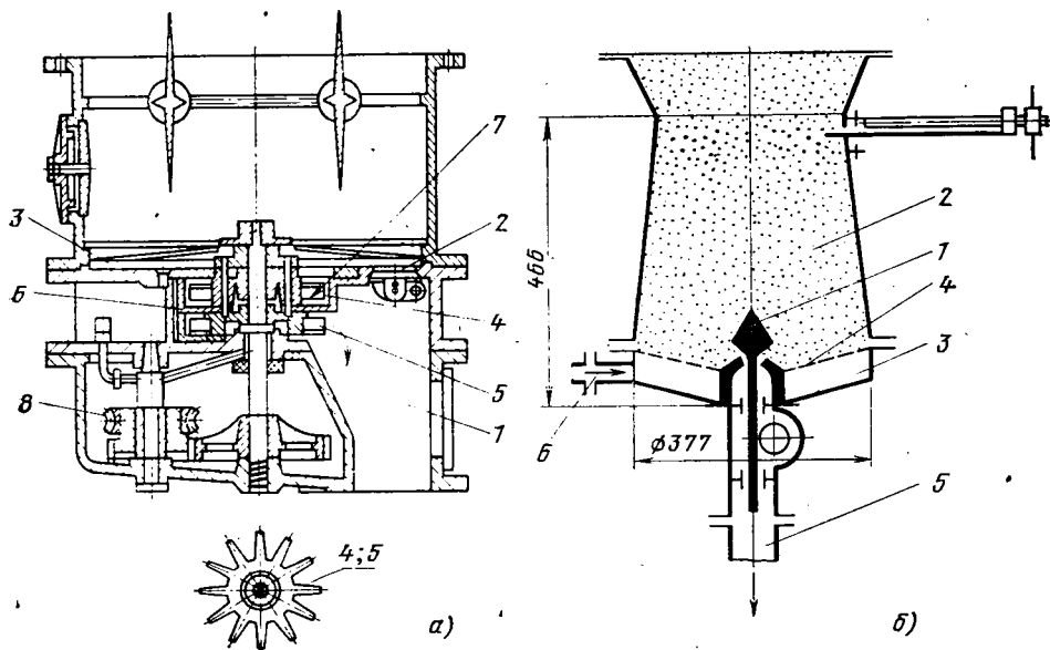
Рис. 8.10. Пылепитатели:
