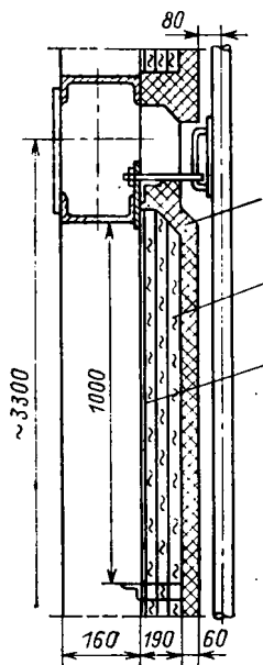
Рис. 24.8. Накаркасная панельная обмуровка:
