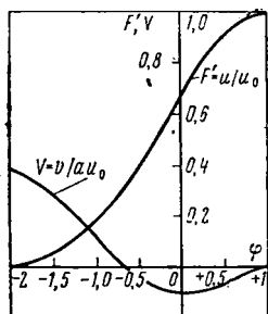
Рис. 6.12. Распределение скоростей в поперечном сечении начального участка струи
