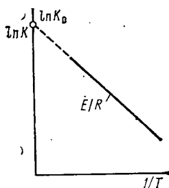
Рис. 6.2. Зависимость \ln K от 1/T
