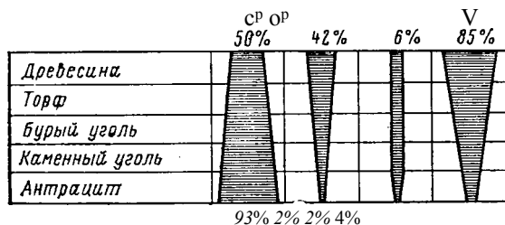
Рис. 3.1. Динамика изменения элементарного состава твердых топлив
