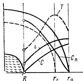
Рис. 6.10. Схема горения капли жидкого топлива
