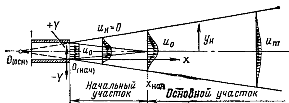
Рис. 6.11. Схема турбулентной струи
