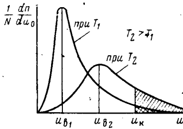
Рис. 6.4. Кривые распределения Максвелла при температурах T_1 и T_2
