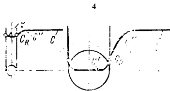
Рис. 6.8. Распределение концентрации кислорода снаружи и внутри мелкой и крупной «с-сжигания» топлива в высокоотурбулированных потоках.
