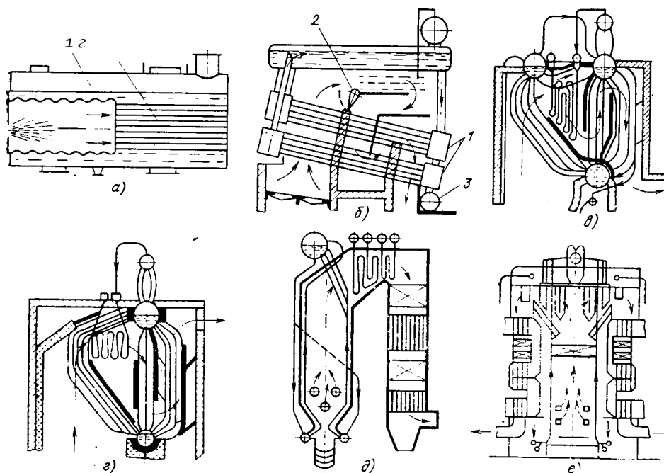
Рис. 1.4. Развитие конструкции котлов с естественной циркуляцией
