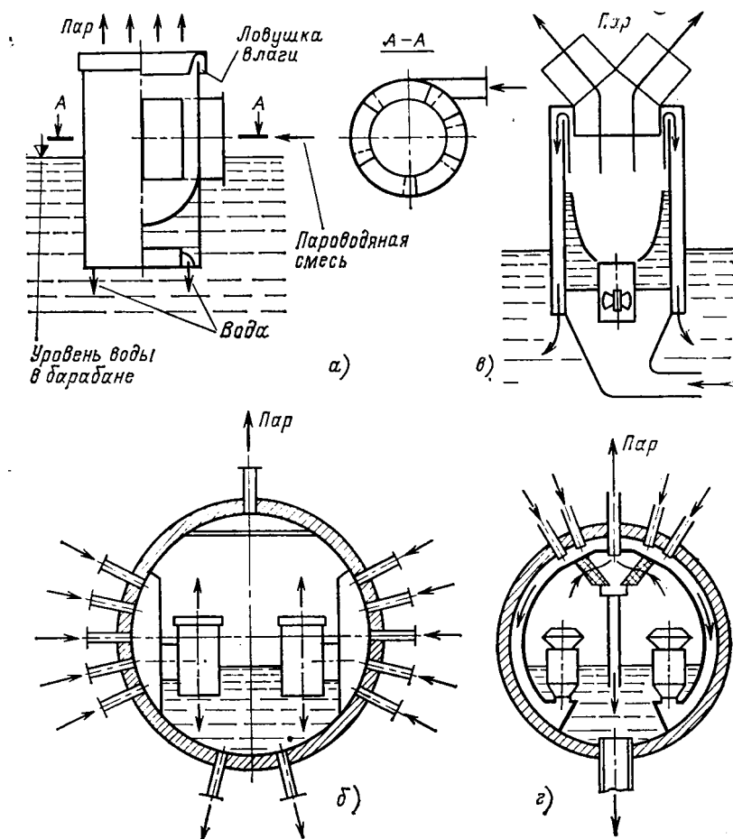
Рис. 19.6. Внутрибарабанные сепарационные циклоны:
