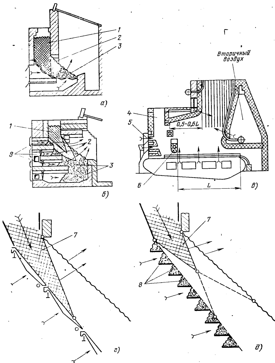
Рис. 7.3. Развитие шахтных топок:
