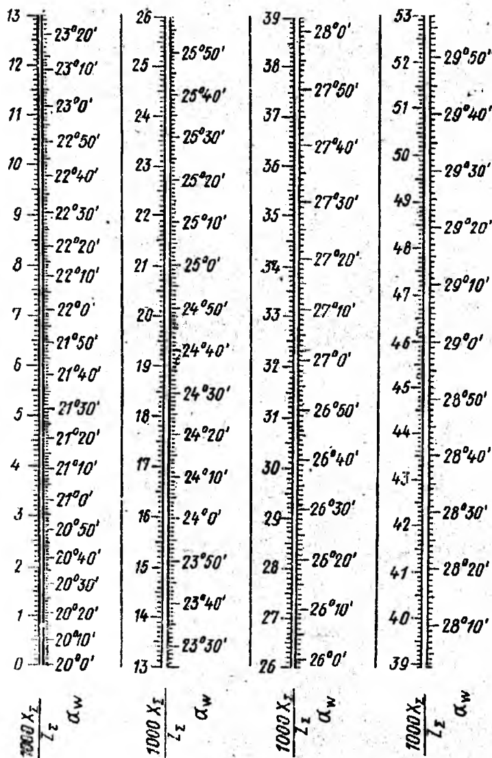
Рис.11 Номограмма для определения угла зацепления \alpha_w
