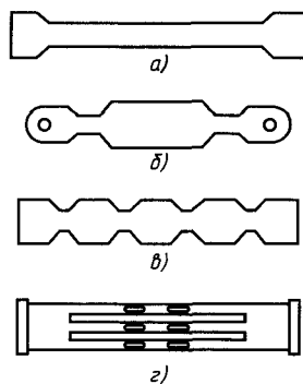
Рис. 14.3. Варианты исполнения плавких вставок:
