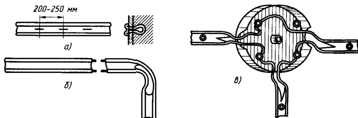
Рис. 2.16. Прокладка проводок АППВ и ППВ:
