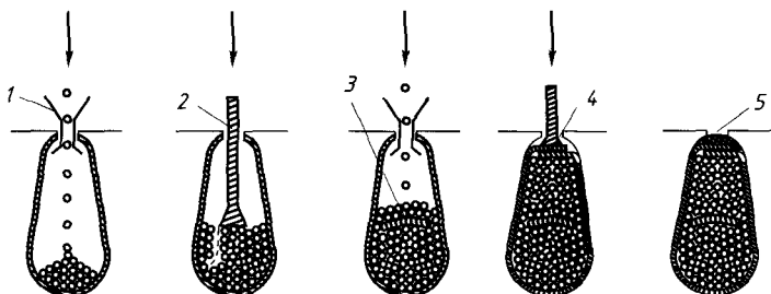
Рис. 10.2. Эскизы паза в процессе «всыпания» витков обмотки
