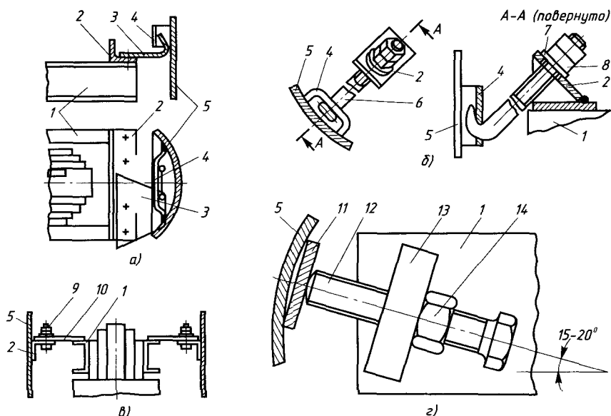
Рис. 11.15. Крепление активной части в баке:
