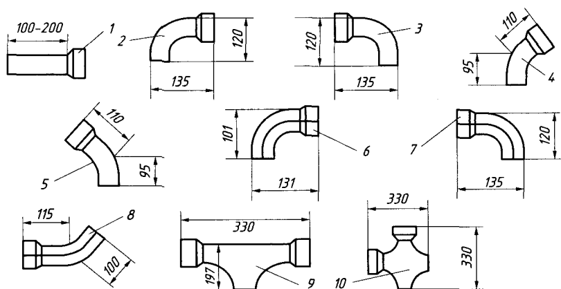
Рис. 2.20. Короба и детали для прокладки осветительных проводов:
