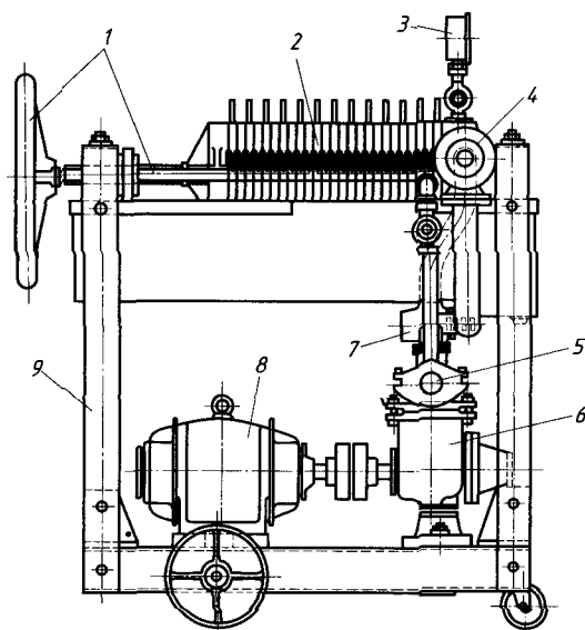
Рис. 12.17. Фильтр-пресс:
