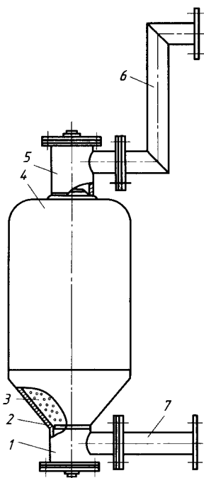
Рис. 6.2. Термосифонный фильтр:
