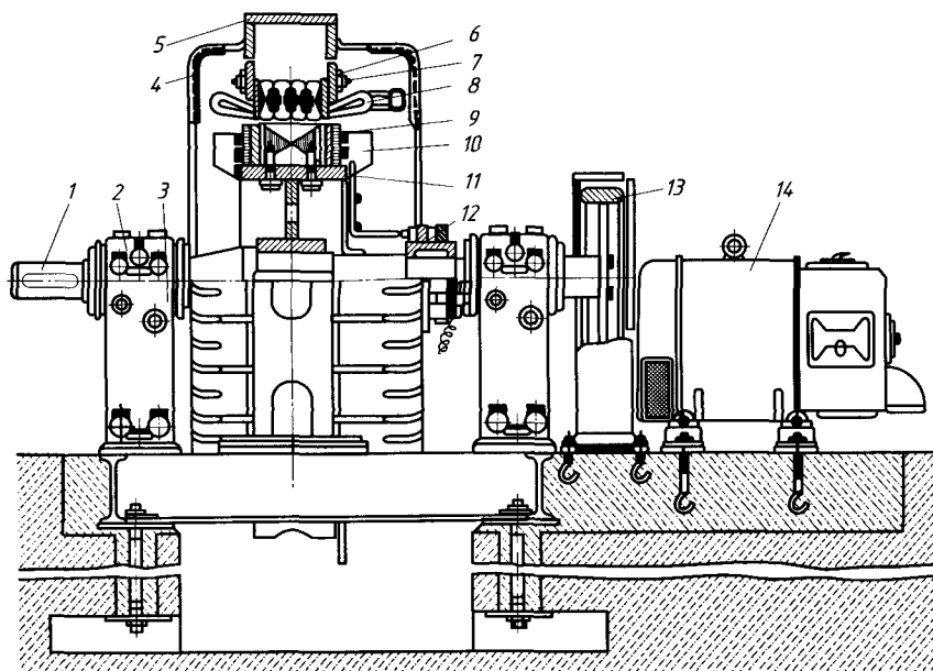
Рис. 1.2. Синхронный генератор (степень защиты IP 22, способ охлаждения IC 01, способ монтажа IM 7312): 1 — вал; 2, 3 — головка и стойка подшипника; 4 — кожух; 5 — корпус; 6, 8 — сердечник и обмотка статора; 7 — шпилька; 9 — полюс; 10 — лопатка вентилятора; 11 — крестовина ротора; 12 — контактные кольца; 13 — клиноременная передача; 14 — возбудитель
