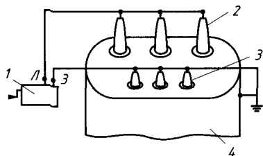
Рис. 12.23. Схема измерения сопротивления изоляции обмоток: 1 — мегомметр; 2 — выводы ВН; 3 — выводы НН; 4 — бак трансформатора
