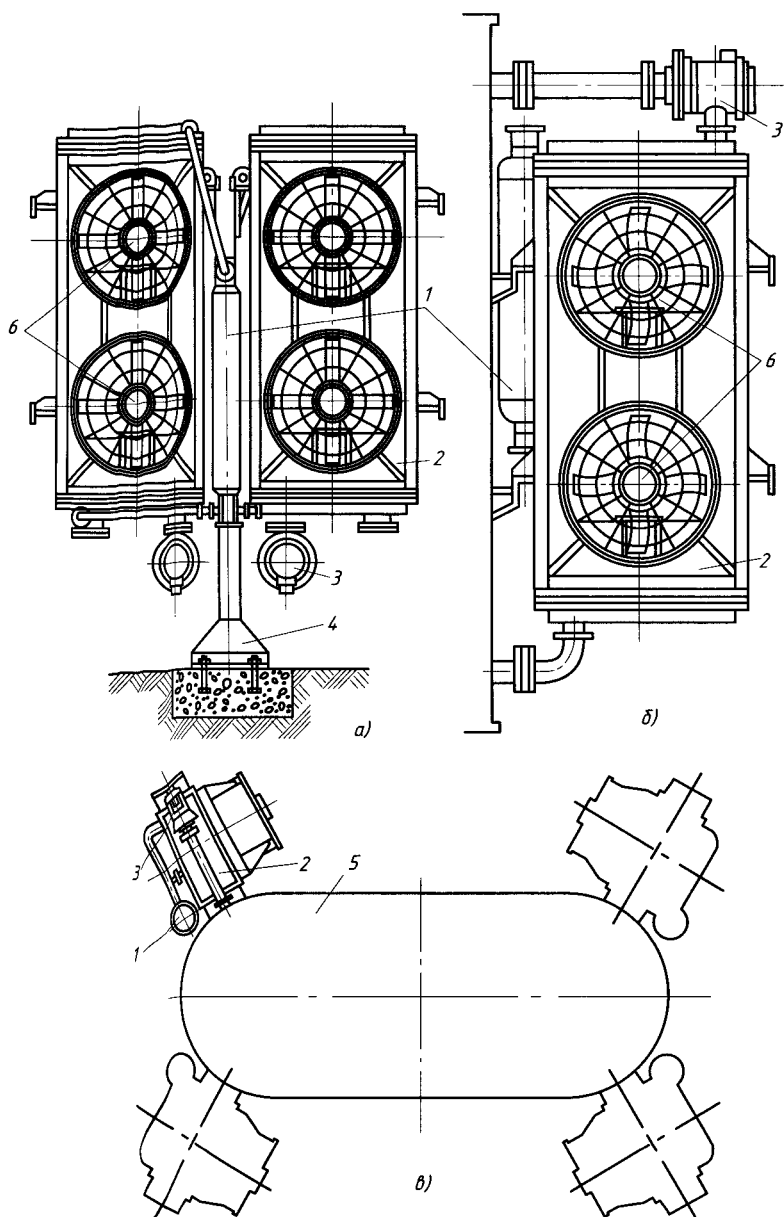
Рис. 3.29. Установка охлаждающих устройств (ОУ) системы ДЦ: а — выносные ОУ; б — навесные ОУ; в — расположение навесных ОУ на баке трансформатора IV габарита (1 — термосифонный фильтр; 2 — охладитель; 3 — масляный насос; 4 — стойка выносных ОУ; 5 — бак трансформатора; 6 — дутьевые вентиляторы)
