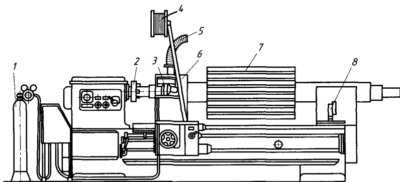
Рис. 9.6. Установка газоплазменного напыления
