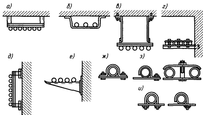
Рис. 2.19. Опорные и крепежные конструкции и детали для трубных электропроводов:
