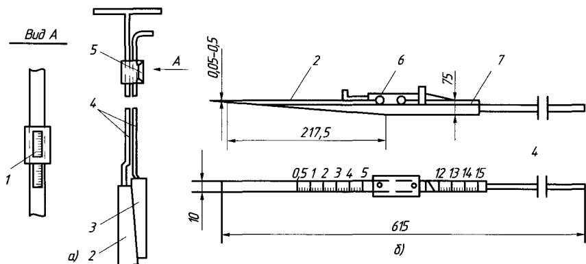
Рис. 3.13. Специальный (а) и клиновой (б) щупы:
