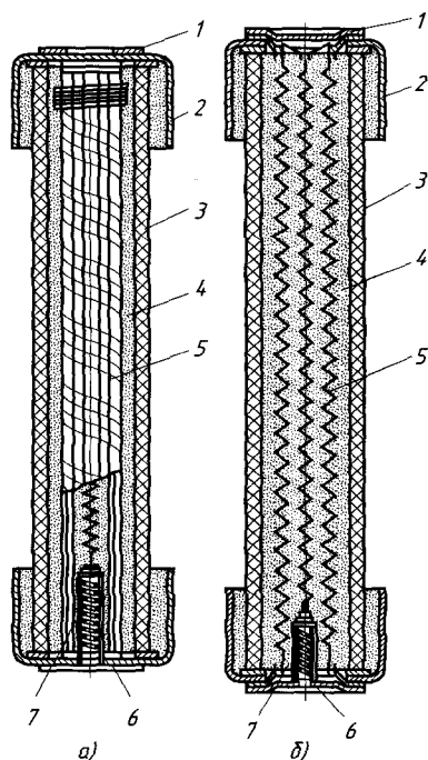
Рис. 14.5. Патроны предохранителей ПК с плавкими вставками на керамическом сердечнике (а) и свитыми в спираль (б):
