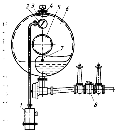
Рис. 6.3. Устройство пленочной защиты:
