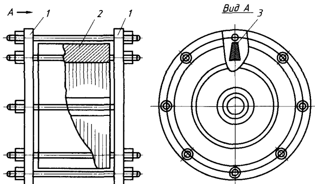
Рис. 9.9. Приспособление для снятия сердечника с вала: 1 — массивные шайбы; 2 — сердечник; 3 — стальной калибр
