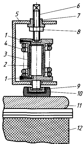
Рис. 11.8. Эскиз гидропружинного запорного устройства
