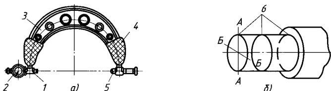
Рис. 3.15. Скоба с отсчетным устройством ( а ) и определение посадочных размеров конца вала ( б ):
