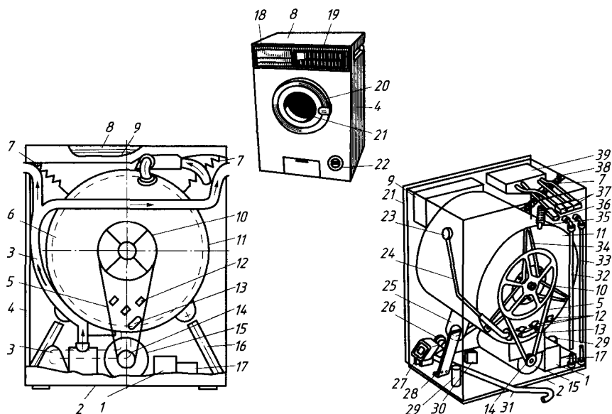
Рис. 5.3. Стиральная машина СМА-4ФБ:
