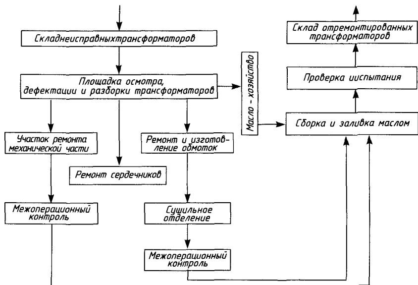
Рис. 7.2. Типовая структурно-технологическая схема ремонта трансформаторов
