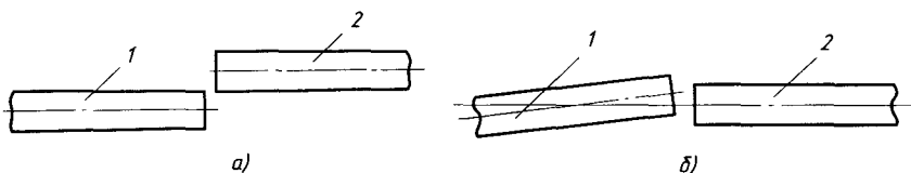
Рис. 3.17. Смещение валов: a — боковое (радиальное); b — угловое (осевое)
