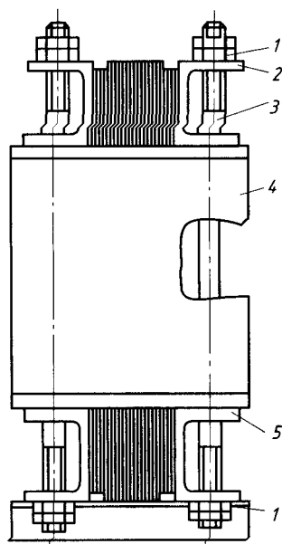
Рис. 11.3. Эскиз активной части трансформатора
