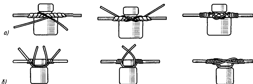
Рис. 2.21. Крепление проводов на изоляторах:
