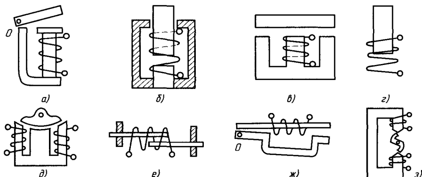
Рис. 4.1. Электромагнитные системы электрических аппаратов:
