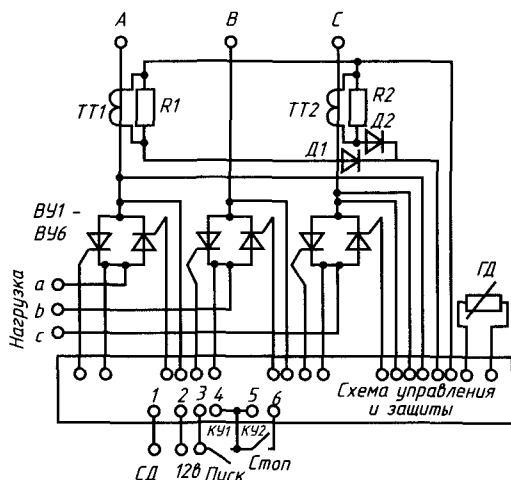
Рис. 14.11. Электрическая схема тиристорного пускателя ПТ40 -380
