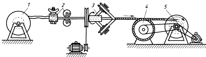
Рис. 12.4. Схема бумагооплеточного станка
