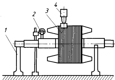
Рис. 9.10. Схема исправления кривизны вала:
