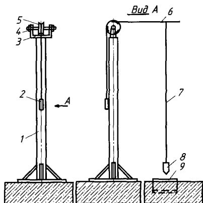
Рис. 3.1. Оседержатель:
