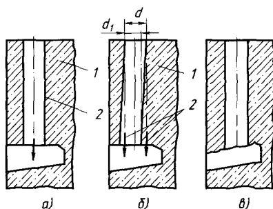
Рис. 3.4. Правильное (а) и неправильное (б, в) выполнение колодцев под фундаментные болты:
