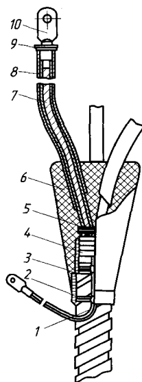
Рис. 2.9. Концевая заделка КВЭн: 1 — провод заземления; 2 — проволоочный бандаж провода заземления; 3 — двухслойная подмотка; 4 — оболочка кабеля; 5 — бандаж из суровых ниток на поясной изоляции; 6 — корпус из эпоксидного компаунда; 7 — токопроводящая жила в заводской изоляции; 8 — трубка из найритовой резины; 9 — бандаж или хомут; 10 — наконечник
