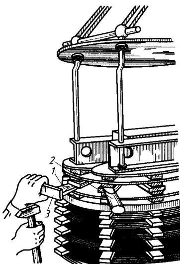
Рис. 11.4. Обмотки трансформатора с прессующими клиньями:
