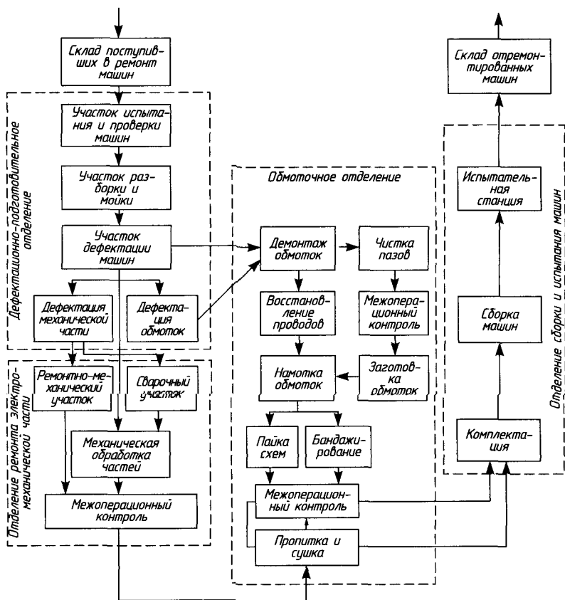
Рис. 7.1. Типовая структурно-технологическая схема ремонта электрических машин
