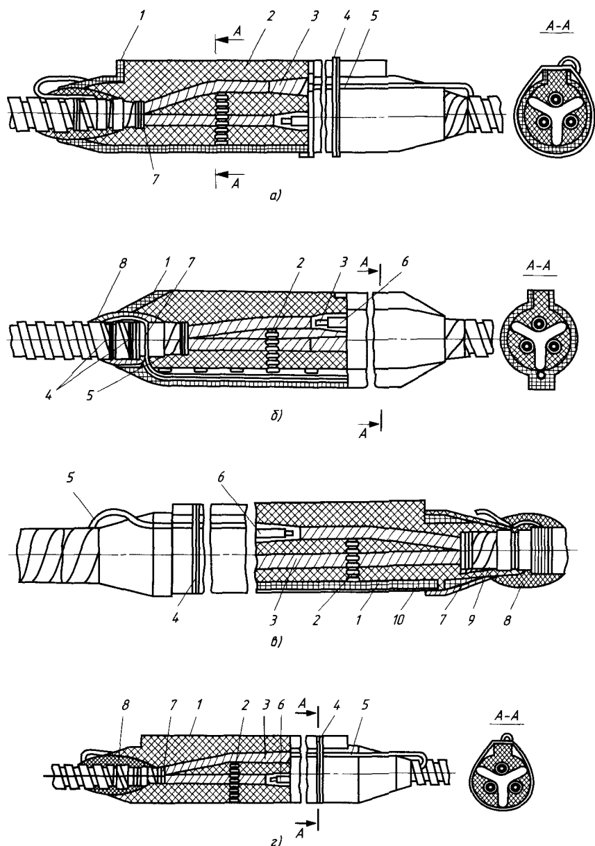
Рис. 2.5. Эпоксидные соединительные муфты (а — СЭп; б — СЭв; в — СЭм; з — СЭс):
