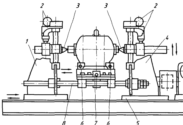
Рис. 8.6. Стенд для разборки электродвигателя:
