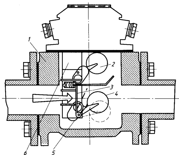
Рис. 6.1. Газовое реле
