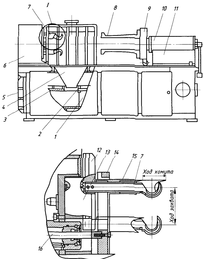
Рис. 8.11. Станок типа УПО-1 для удаления обмотки из статоров: 1 — ползун; 2 — нож; 3 — пакетирующий пресс; 4 — бункер; 5 — шибер; 6, 11 — передняя и задняя бабки; 7 — захват; 8, 12 — кулачки; 9 — патрон; 10 — цилиндр; 13 — самоцентрирующийся патрон; 14 — диск с пазами; 15 — хомуты; 16 — гидроцилиндр
