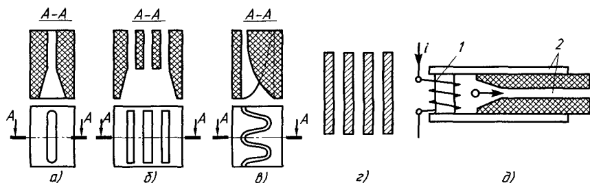
Рис. 4.2. Схемы дугогасительных камер низкого напряжения:
