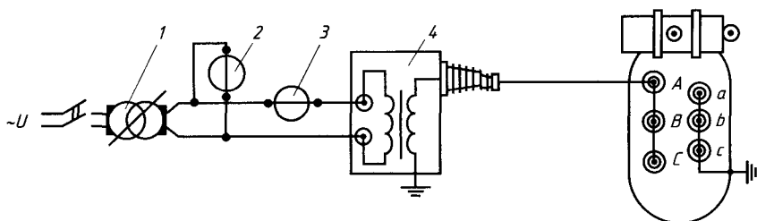
Рис. 12.21. Схема испытания изоляции обмотки ВН приложенным напряжением:
