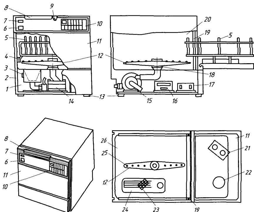
Рис. 5.6. Посудомоечная машина МПА-4:
