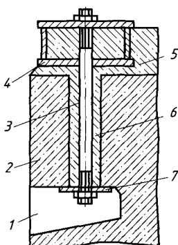
Рис. 3.3. Колодец в фундаменте для установки фундаментных болтов: 1 — ниша; 2 — фундамент; 3 — фундаментный болт; 4 — фундаментная плита; 5 — цементная подливка; 6 — колодец; 7 — анкерная пласка
