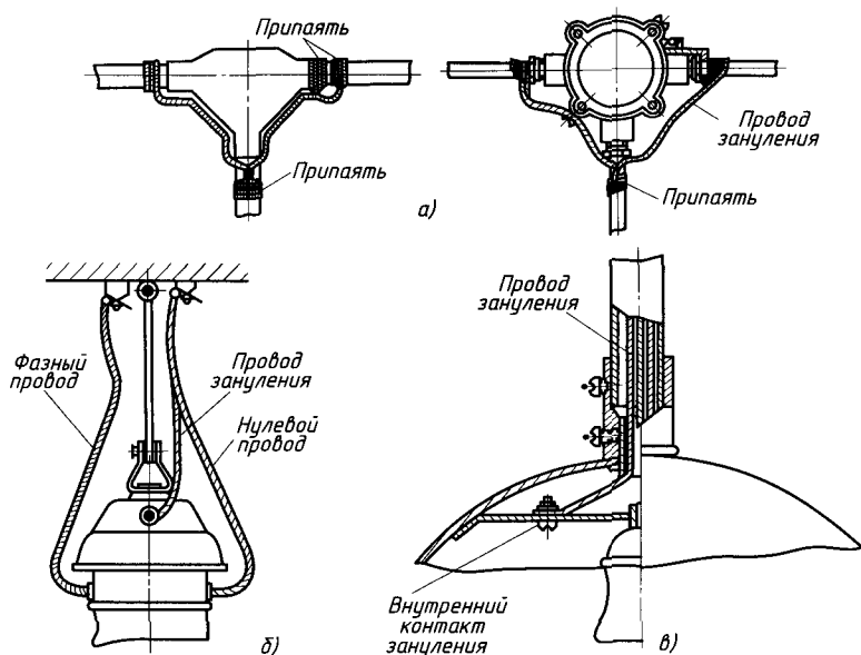
Рис. 2.26. Защитное заземление (зануление) ответственных коробок и металлических оболочек проводов и кабелей (а) и корпуса светильников снаружи (б) и внутри (в)
