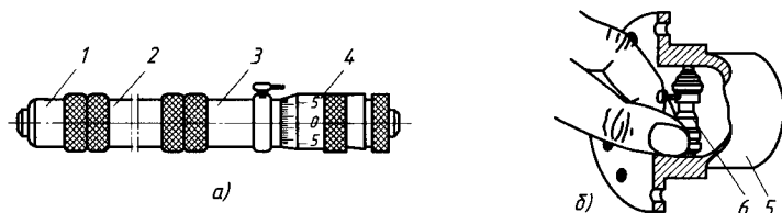
Рис. 3.16. Микрометрический нутромер ( а ) и определение им посадочных размеров конца вала ( б ):
