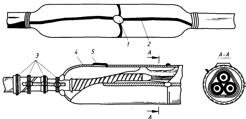
Рис. 2.4. Свинцовая соединительная муфта кабелей напряжением 6 и 10 кВ: 1 — участок присоединения заземляющего провода к корпусу муфты; 2 — заземляющий провод; 3 — проволоочные бандажи; 4 — корпус; 5 — заливочное отверстие, закрытое свинцовой пластиной
