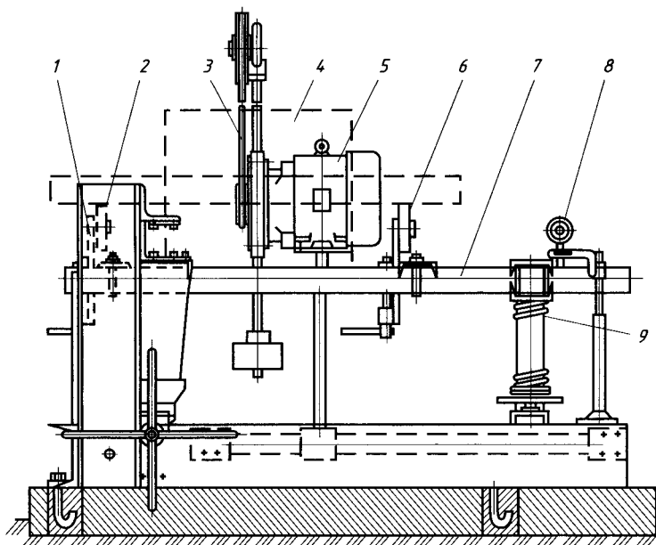
Рис. 10.6. Универсальный балансировочный станок:
