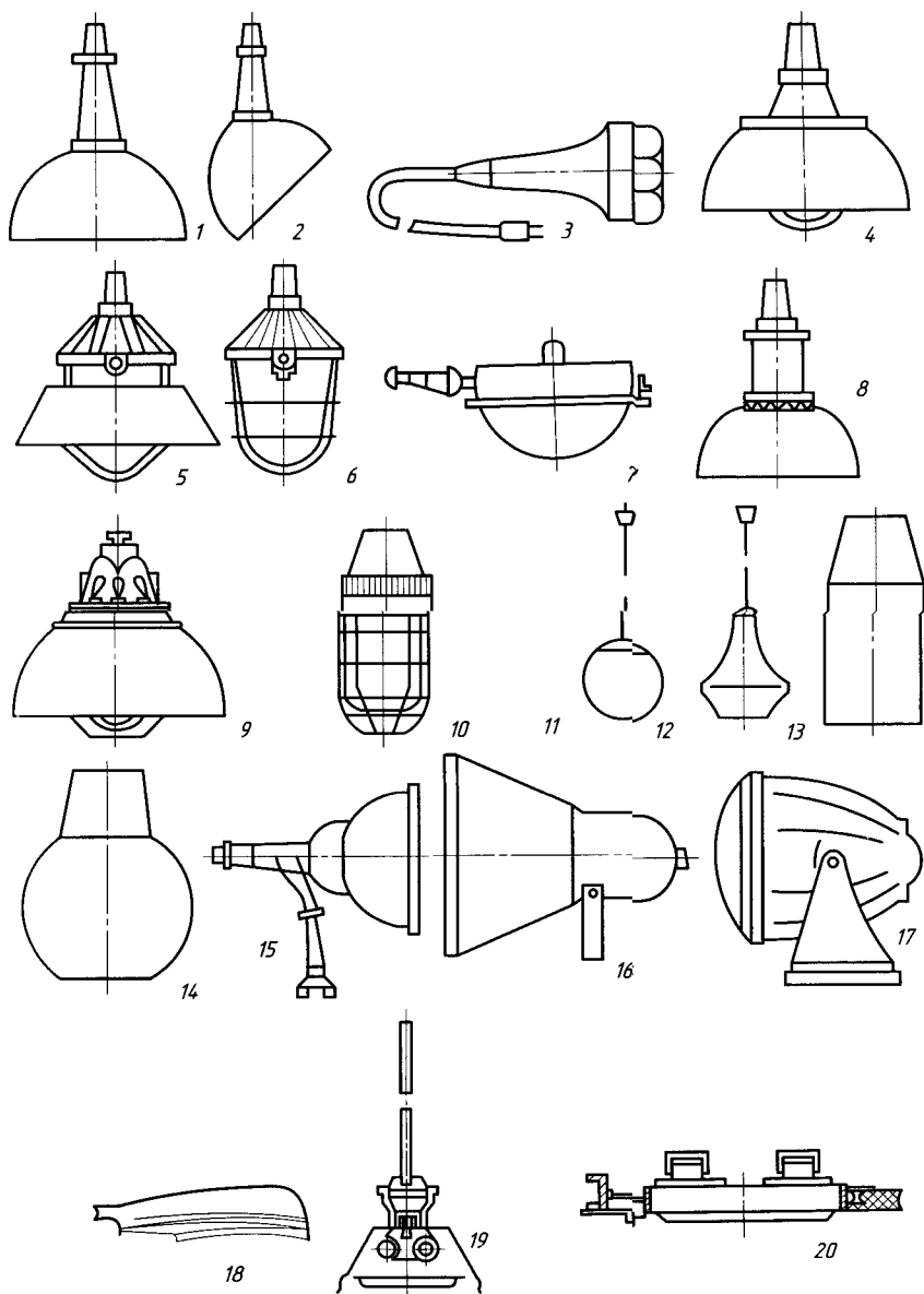
Рис. 2.22. Светильники, применяемые в промышленных помещениях: 1 — ГСМ-500, -1000, -1500, «Астра-11, -12», УПД, ДРЛ; 2 — «Астра-22, -23»; 3 — ГВО-36; 4 — ППД-100, -200; 5 — ППД-500; 6 — ГПР-100, -200, -500; 7 — ППП101; 8 — НСПО7; 9 — Н4БН-1501, -15011; 10 — Н4Т2Н-3001; 11 — НСОО2-150 (шар); 12 — НСОО2-100 (люцетта); 13, 14 — ПУН; 15 — ПСМ30А1, ПСМ50А2; 16, 17 — СЗЛ1; 18 — «Лилия-1, -2»; 19 — ЛДОР; 20 — ПВЛМ
