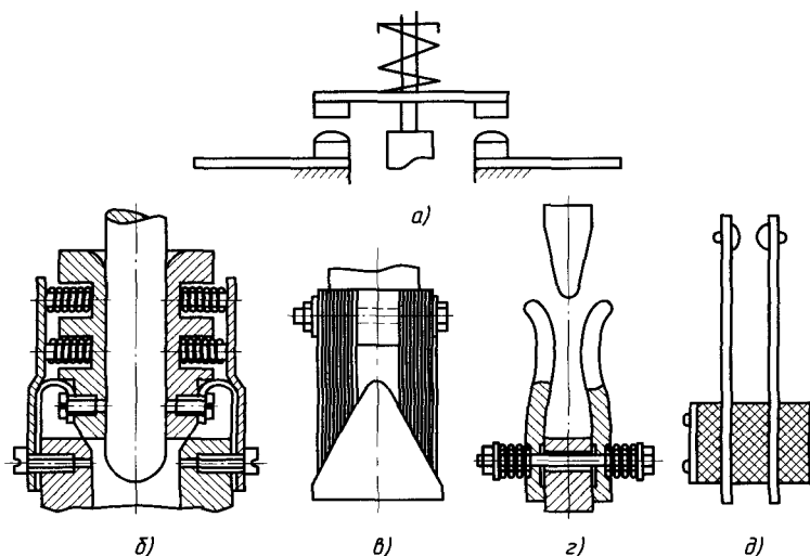
Рис. 4.3. Размыкающие контакты:
