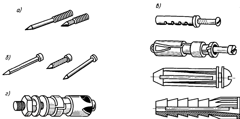
Рис. 2.12. Дюбели:
