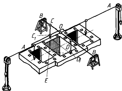
Рис. 3.2. Схема разметки главных осей фундамента:
