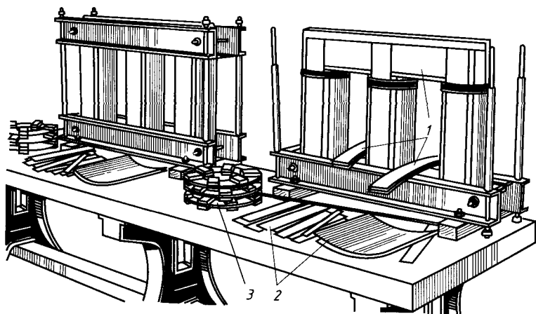
Рис. 12.10. Расшихтовка верхнего ярма трансформатора мощностью 100 кВ·А: 1 — пластины ярма; 2 — детали, подготовленные к сборке; 3 — ярмовая изоляция
