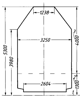
Рис. 3.27. Железнодорожный га-
