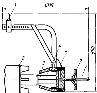
Рис. 8.3. Приспособление для выема и ввода ротора: 1 — серга; 2 — ротор; 3 — вал; 4 — кулачки; 5 — пластина; 6 — рукоятка; 7 — ось
