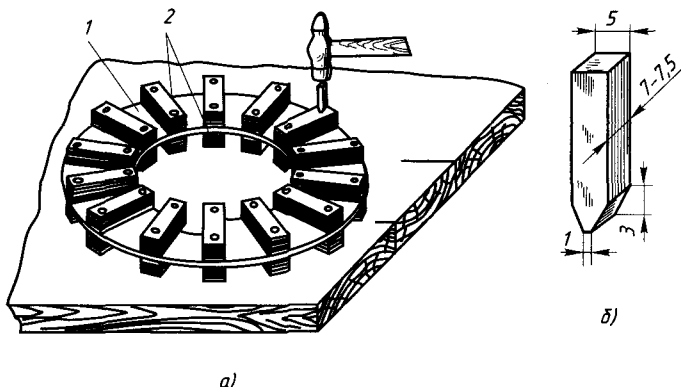
Рис. 12.9. Сборка ярмовой изоляции обмотки трансформатора III габарита: а — ярмовая изоляция; б — заклепка из электрокартона
