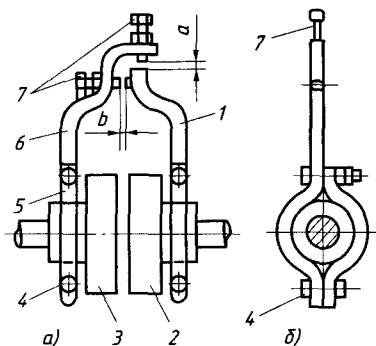
Рис. 3.19. Центровка валов с помощью радиально-осевых скоб:
