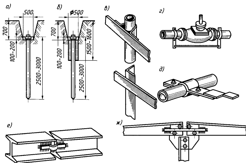
Рис. 2.23. Устройство заземления:
