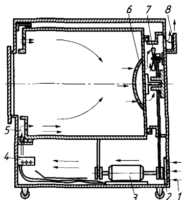
Рис. 5.4. Схема воздушного тракта сушильной машины:
