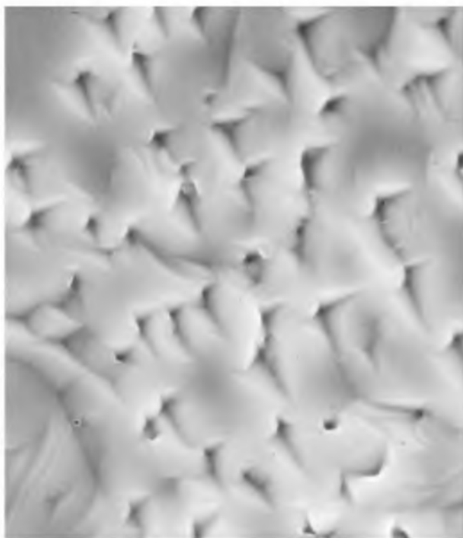
Рис. 2 Рельеф «испарения». Медь, \text{Hg}^+ , 50 эВ, T = 820^\circ\text{C} . Увеличение –1500
