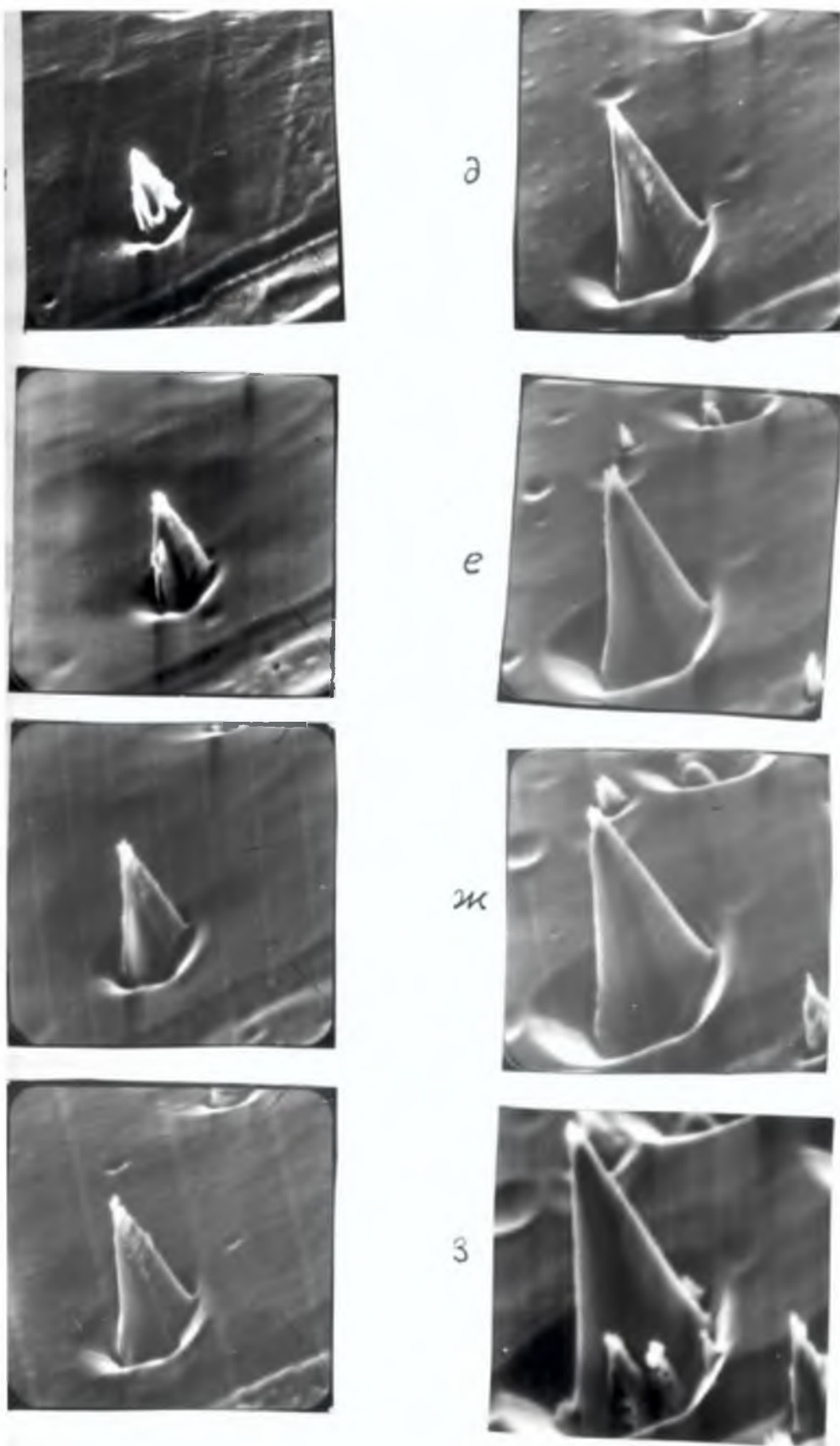
Рис 15. Развитие конуса в период стабилизации. Медь, \text{Ag}^+ , 600 эВ. Увеличение –1000. Время облучения (мин.): а-90; б-110; в-130; г-150; д-170; е-200; ж-230; з-250.
