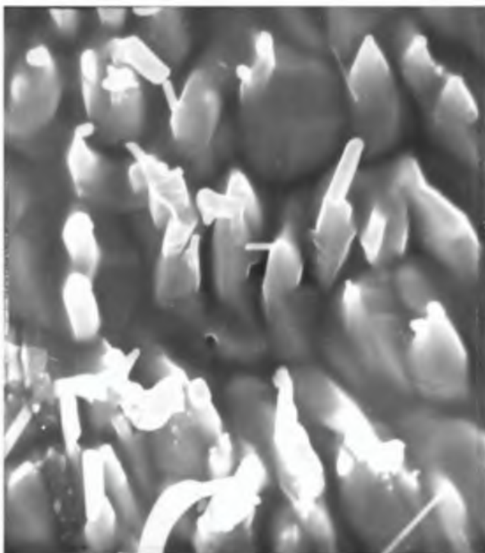
Рис 9. Конусы, наплывающие на кристаллы. Медь, \text{Hg}^+ , 50 эВ. Увеличение –1500.
