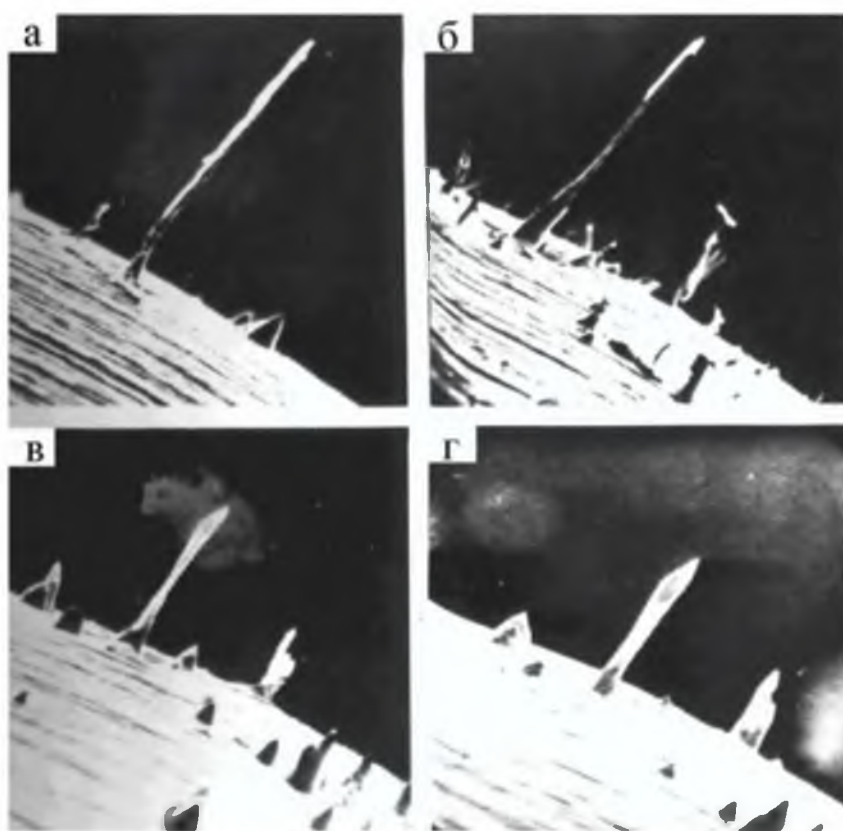
Рис. 10 Динамика развития вискера на поверхности вольфрама. Ионы \text{Ar}^+ , 1000 эВ. Увеличение –270. Доза облучения: а- 3,4 \cdot 10^{20} \text{ см}^{-2} ; б- 4,2 \cdot 10^{20} \text{ см}^{-2} ; в- 5,1 \cdot 10^{20} \text{ см}^{-2} ; г- 6 \cdot 10^{20} \text{ см}^{-2} .
