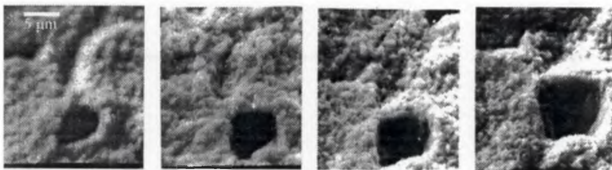
Рис. 23 Развитие поры на поверхности сплава Cu-Ni50at%. \text{He}^+ , 600 эВ. Увеличение \times 4000 .
