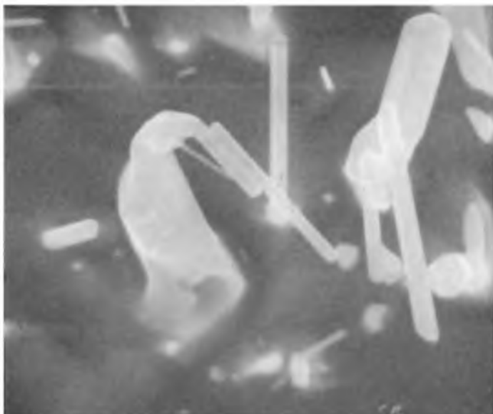
Рис. 7 Сросшиеся вис커ры. Медь, ионы \text{Hg}^+ , 50 эВ. Увеличение –6000
