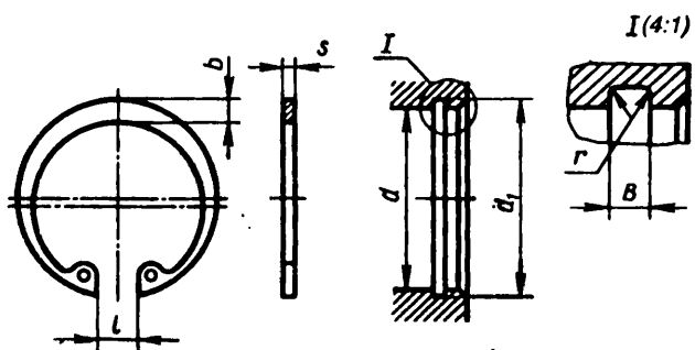
Т а б л и ц а 24.21. Кольца пружинные упорные плоские внутренние эксцентрические (из ГОСТ 13941—86) и канавки для них, мм
