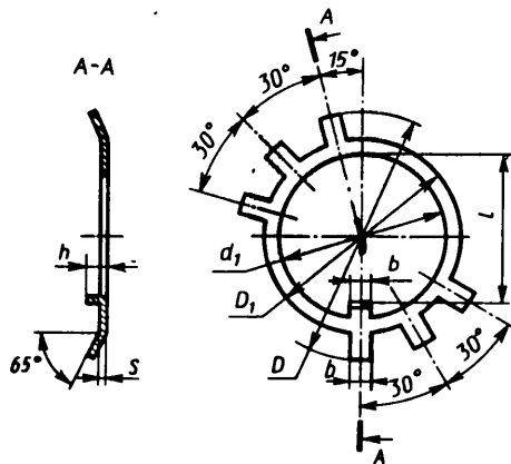
Т а б л и ц а 24.23. Шайбы стопорные многолапчатые (из ГОСТ 11872—89), мм
