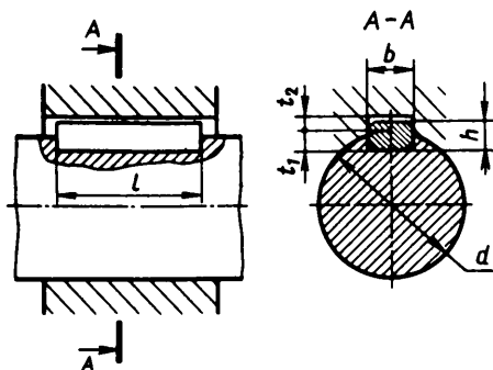
Т а б л и ц а 24.29. Шпонки призматические (из ГОСТ 23360—78)
