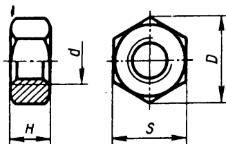
Т а б л и ц а 24.43. Гайки шестигранные с уменьшенным размером «под ключ» класса точности В (из ГОСТ 15521—70), мм
