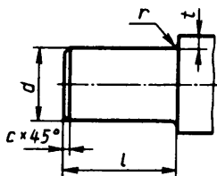
Т а б л и ц а 24.28. Концы валов цилиндрические (из ГОСТ 12080—66), мм
