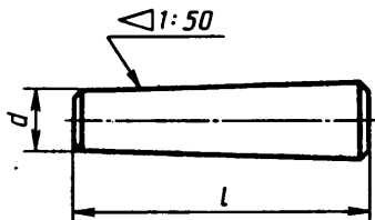
Т а б л и ц а 24.36. Штифты конические (из ГОСТ 3129—70), мм
