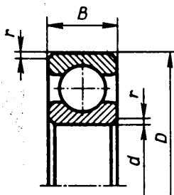
Т а б л и ц а 24.10. Подшипники шариковые радиальные однорядные (из ГОСТ 8338—75)
