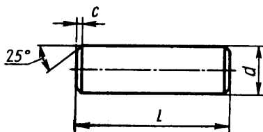
Т а б л и ц а 24.35. Штифты цилиндрические (из ГОСТ 3128—70), мм
