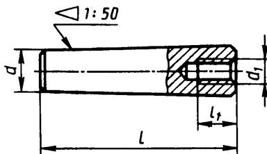
Т а б л и ц а 24.37. Штифты конические с внутренней резьбой класса точности B исполнение 2 (из ГОСТ 9464—79), мм
