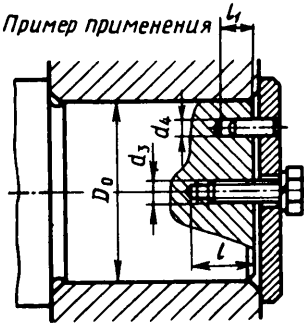
Т а б л и ц а 24.30. Шайбы концевые (из ГОСТ 14734—69), мм
