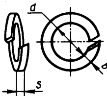
Т а б л и ц а 24.44. Шайбы пружинные (из ГОСТ 6402—70), мм
