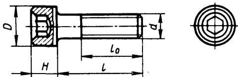
Т а б л и ц а 24.42. Винты с цилиндрической головкой и шестигранным углублением «под ключ» класса точности А (из ГОСТ 11738—84), мм
