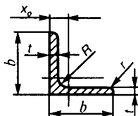
Т а б л и ц а 24.48. Прокатная угловая равнополочная сталь (из ГОСТ 8509—93)
