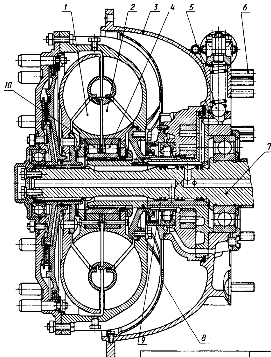
Гидротрансформатор ЛГ-340б
