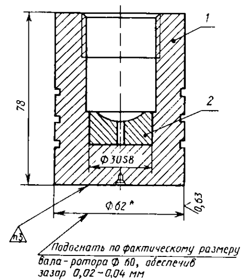
Обозначения: 1-поршень; 2-втулка.
