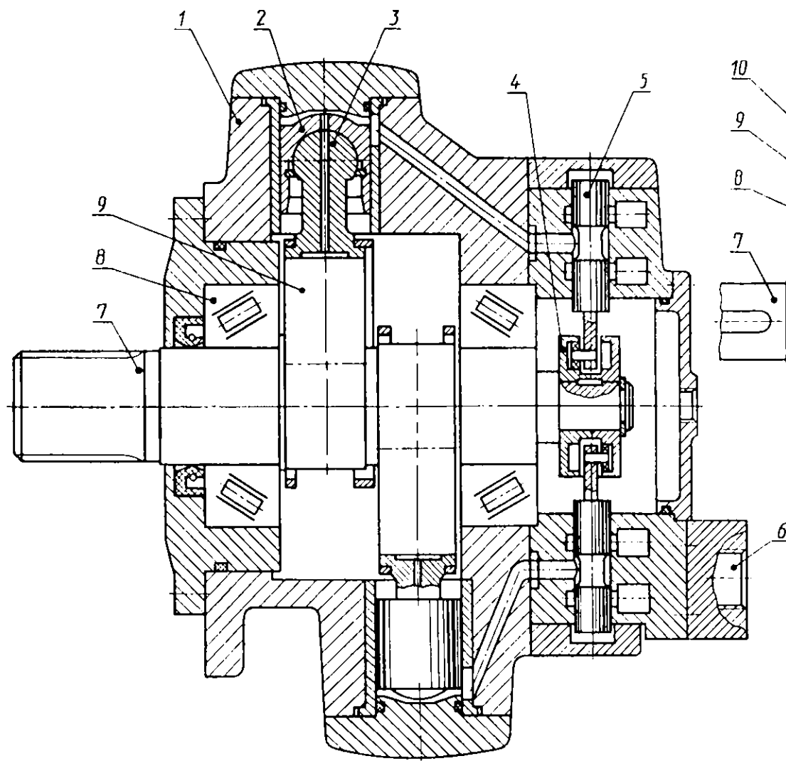
Исполнение с гидростатической разгрузкой шатуна
