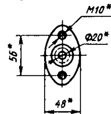
Вид Г уменьшено
