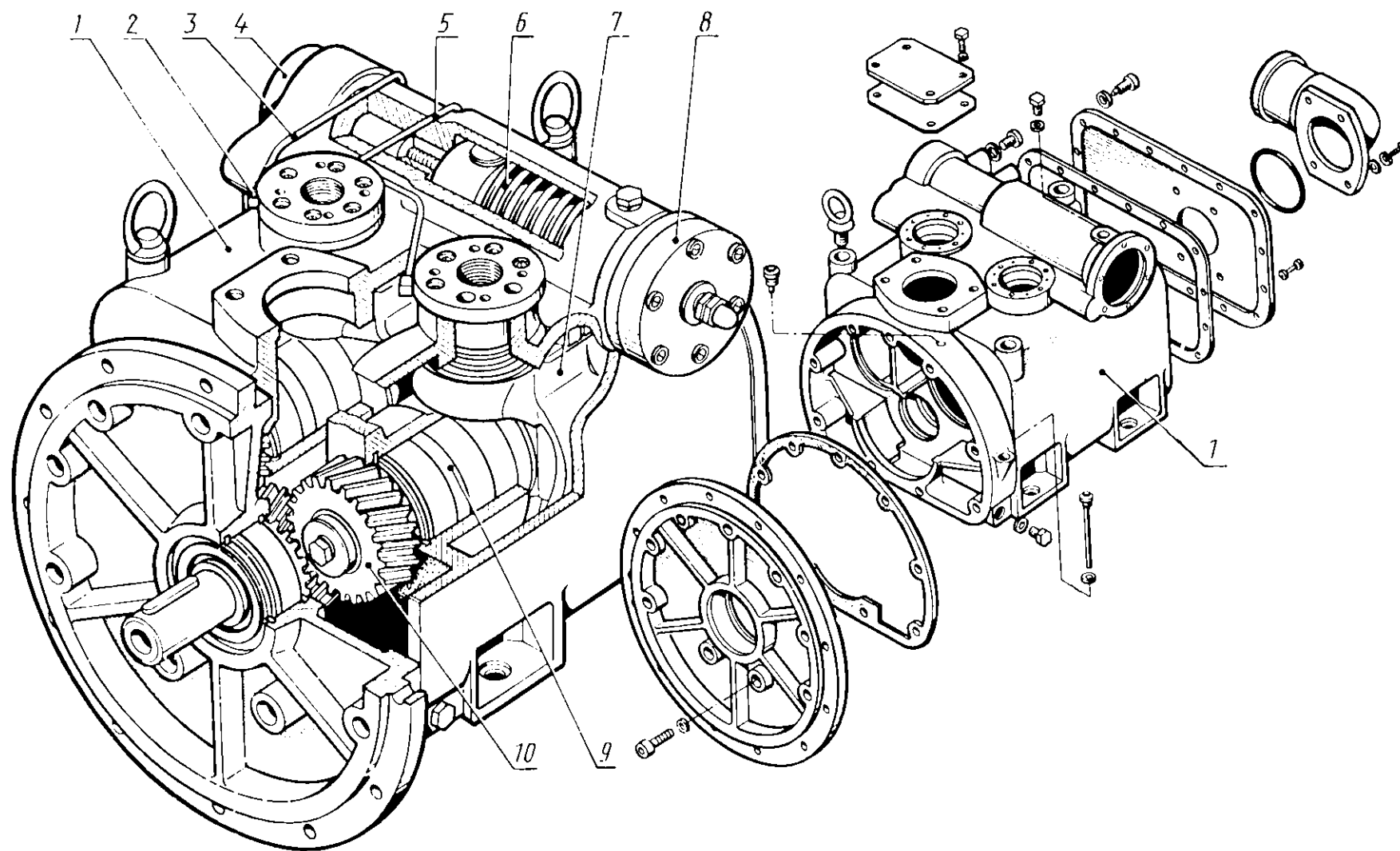
Общий вид насоса
