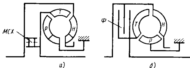
Рис. 12. Конструктивные схемы блокируемых ГДТ: а — с муфтой свободного хода; б — с фрикционом
