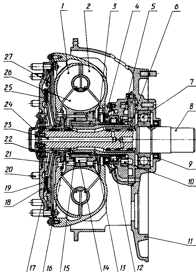
Гидротрансформатор ЛГ-340а
