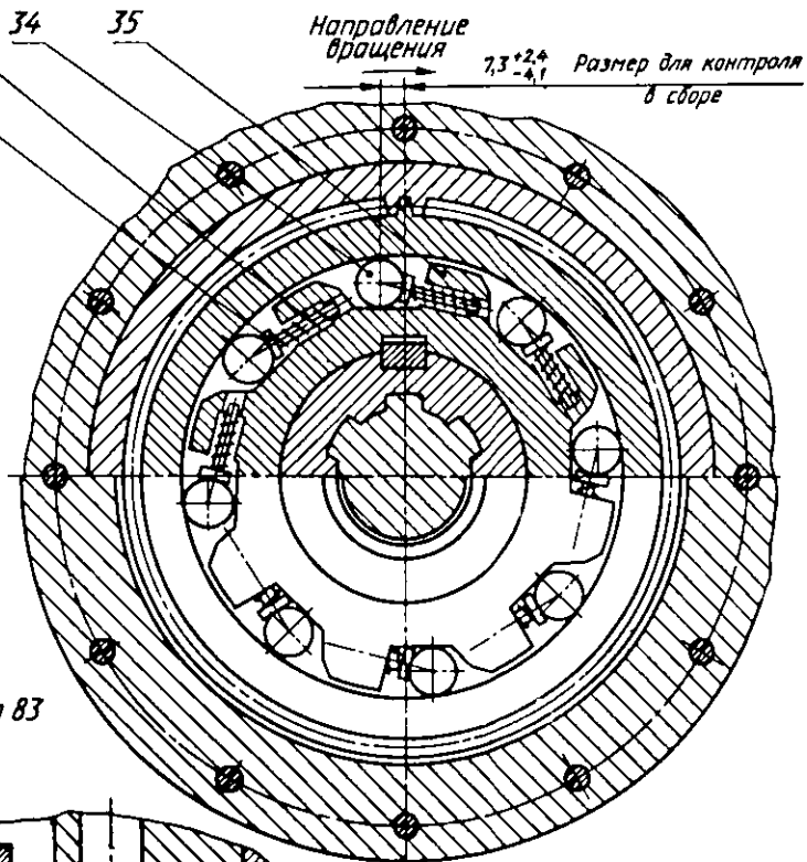
Вид Г уменьшено
