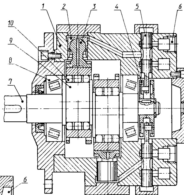
Исполнение с опорой шатуна на подшипник качения
