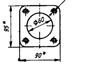
Д-Д уменьшено
