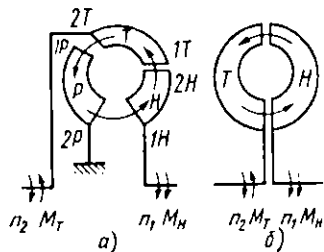
Рис. 8. Схема движения жидкости в гидродинамических передачах:
