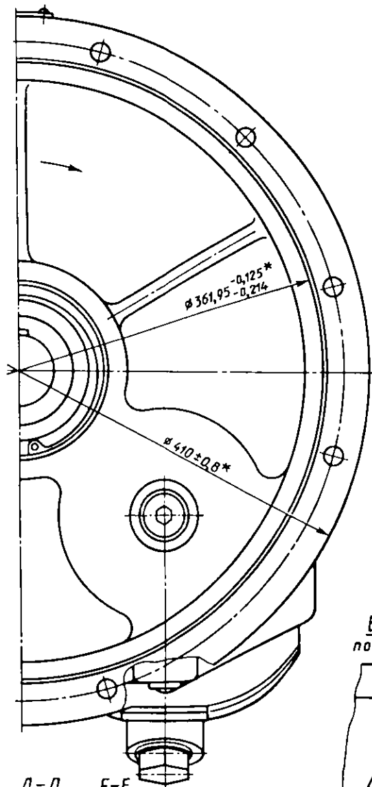
Вид А лист 21
