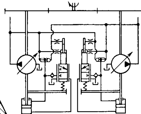
Схема насоса
