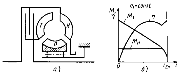
Рис. 14. Конструктивная схема и внешняя харак- теристика комплексно- блокируемого ГДТ: а — схема; б — характеристика
