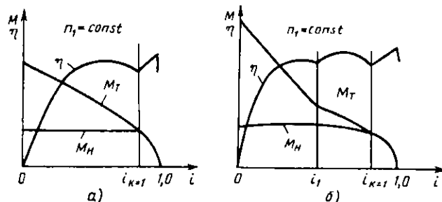
Рис. 11. Внешние характеристики комплексных ГДТ: а — с одним реактором; б — с двумя реакторами
