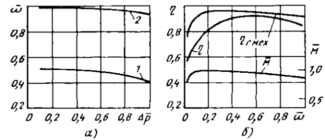
Рис. 3. Типовые относительные характеристики объемного гидромотора:
