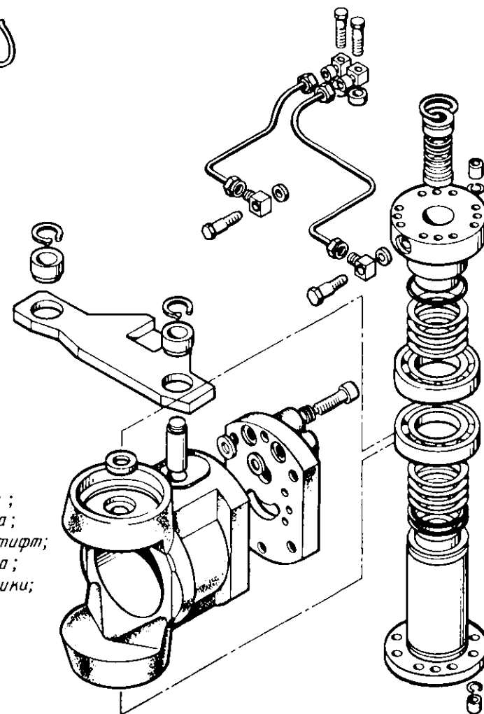
Схема сборки деталей поворотного корпуса
