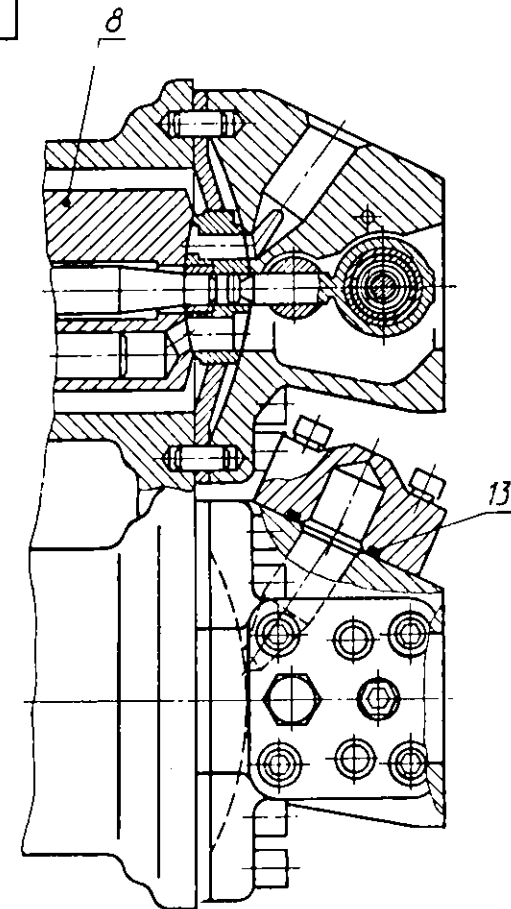
A-A повернуто
