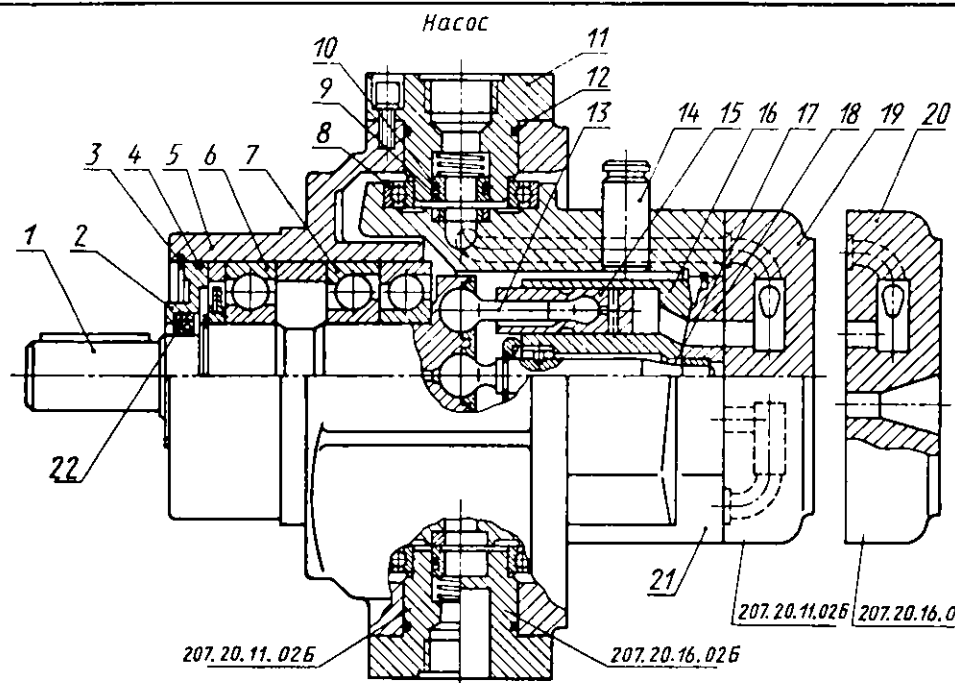
Насос с гидроусилителем
