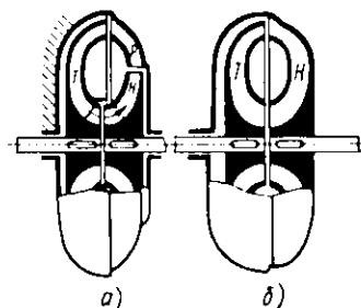
Рис. 5. Гидродинамические передачи Феттингера:
