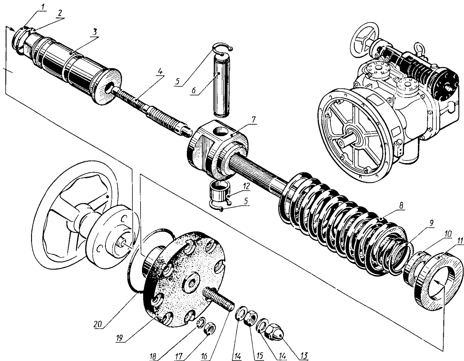
Регулятор мощности в сборе 1,2,5,20 - кольца; 3,12 - втулки; 4 - золотник; 6 - палец; 7 - штанга; 8,9 - пружины; 10,11,18 шайбы; 13,15,17 - гайки; 14 - прокладка; 16 - винт; 19 - крышка
