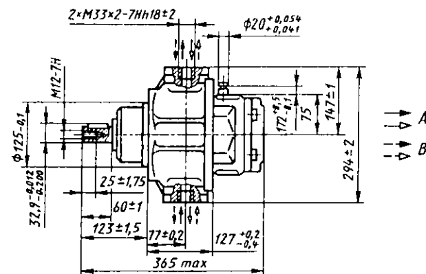
Модель 207.20.16.02Б
