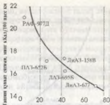
7-рasm. Ташиш қуввати сифимининг шаҳар автобусларида сифдирувчан-лик билан боғлиқлиги.
