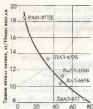
8 - р а с м . Ташишга тўғри келувчи металл сифимининг қ. билан боғлиқлиғи.
