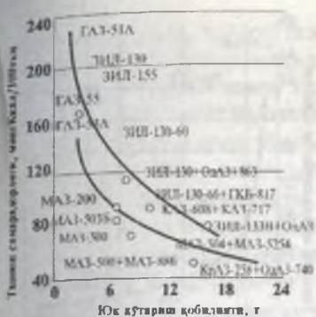
6-рasm. Ташиш қуввати сифими-нинг q_n билан боғлиқлиги.
