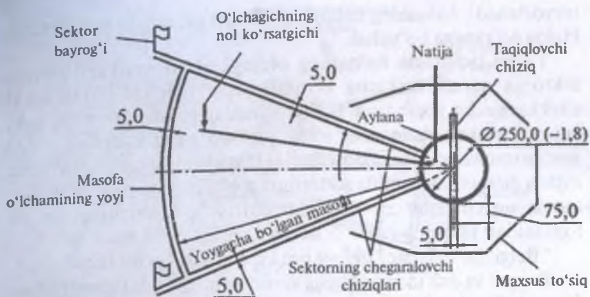
9-rasm. Disk uloqtirish joyi (o'lchamlar sm larda).
