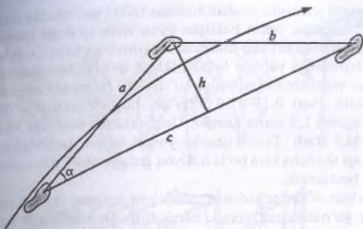
64-rasm. Yugurish uchburchagi, a va b — oxiridan oldingi va oxirgi qadamlar; h — uchburchak balandligi.
