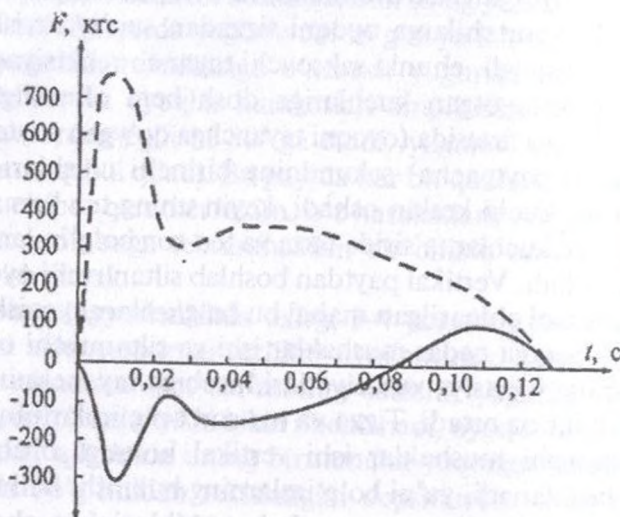
51-рasm. Yugurib kelib uzunlikka sakrashda depsinish dinamogrammasi (vertikal va gorizontol holati).
